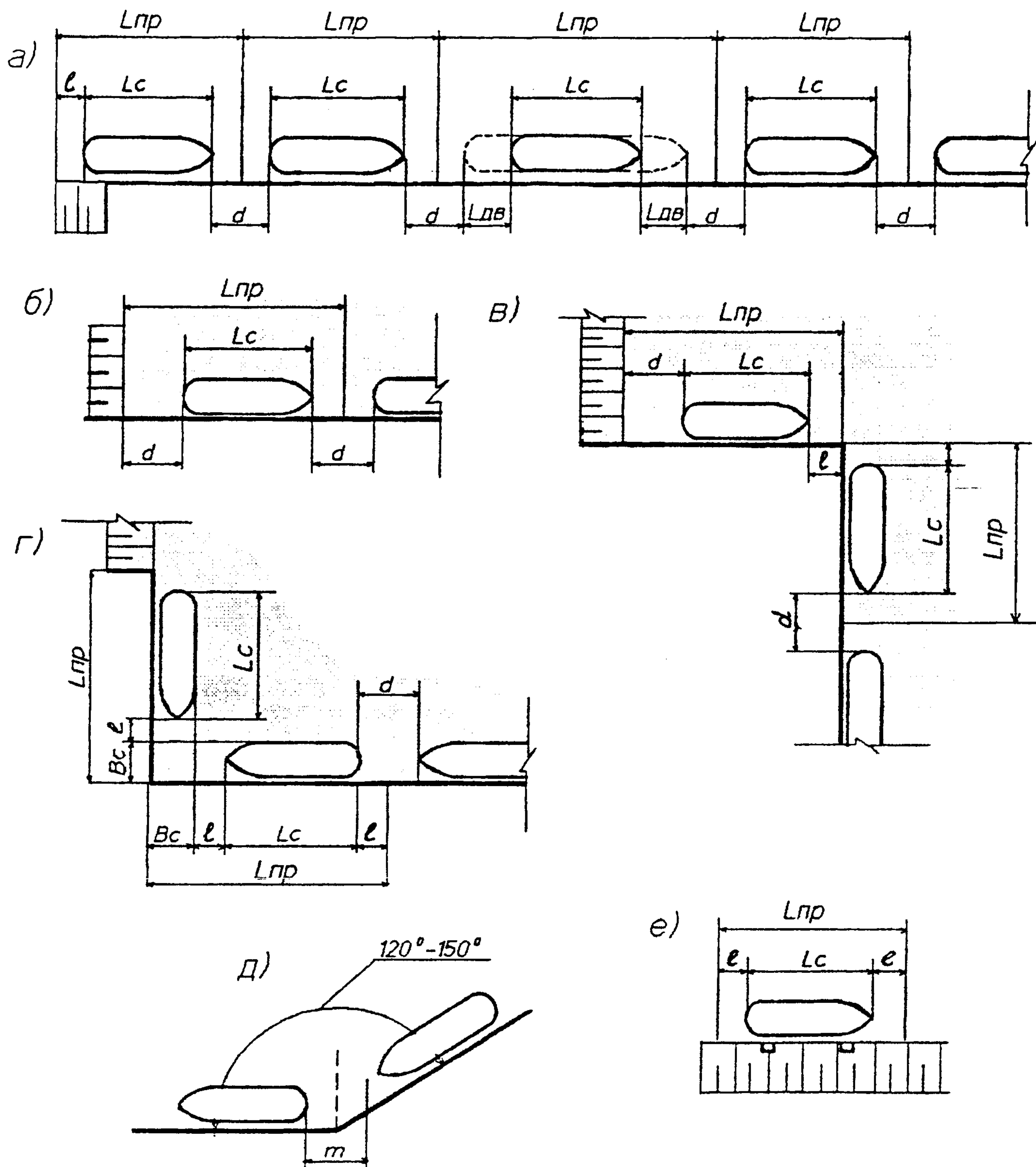
Рисунок 4.5.1 - Схемы размещения судов у причала
