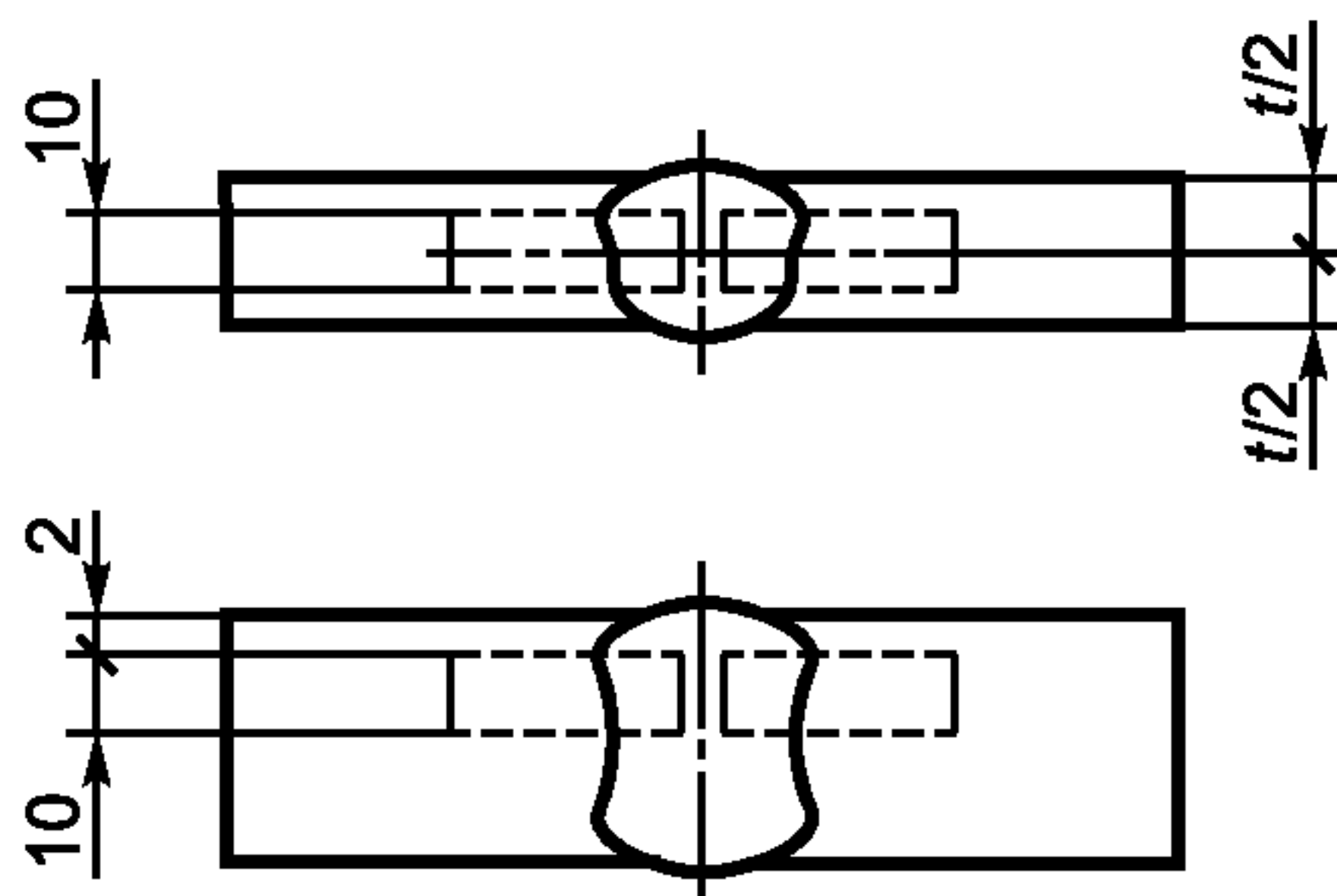
Рисунок 2 — Расположение образцов для испытаний на ударный изгиб
