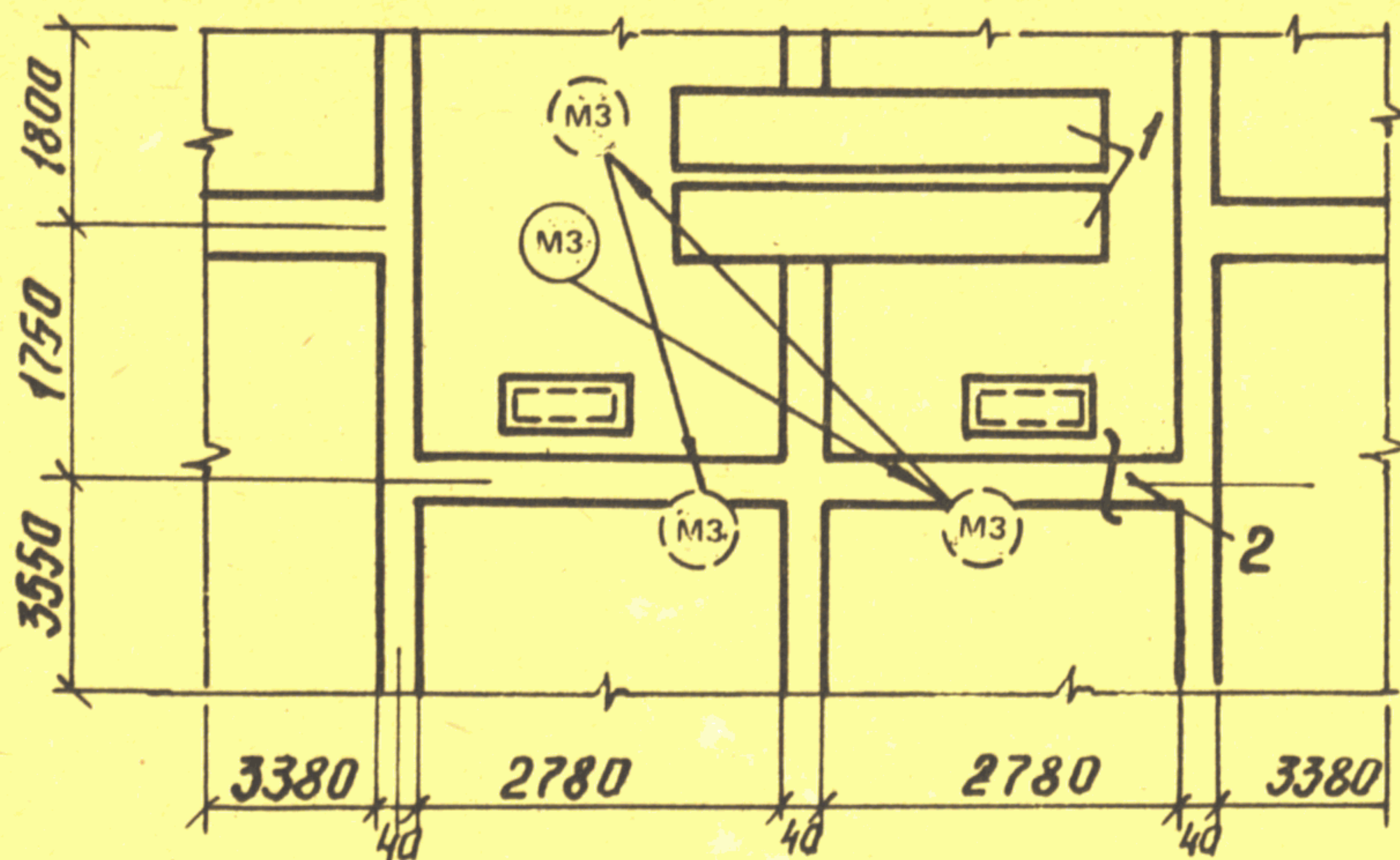
Схема организации рабочего места
