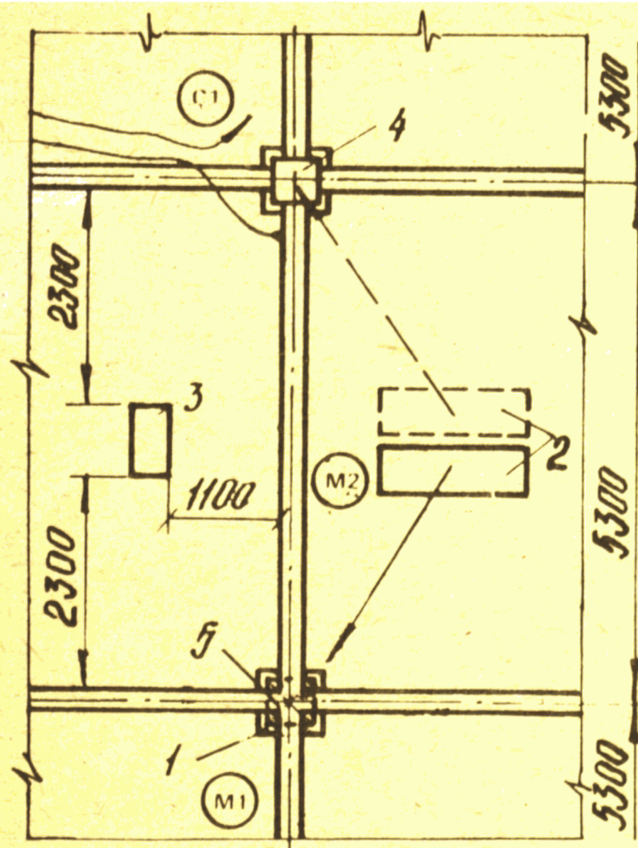
Схема организации рабочего места
