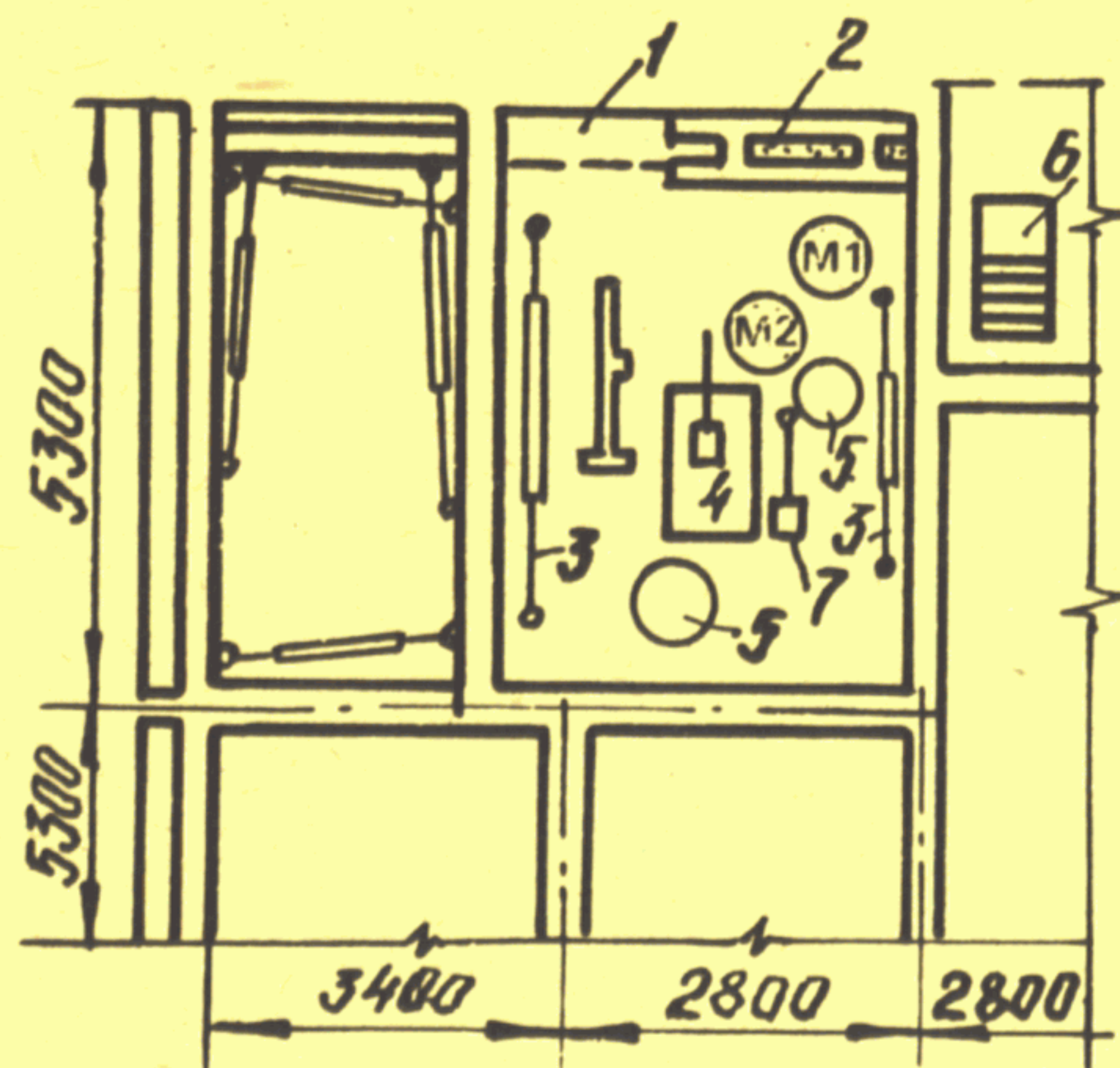
Схема организации рабочего места
