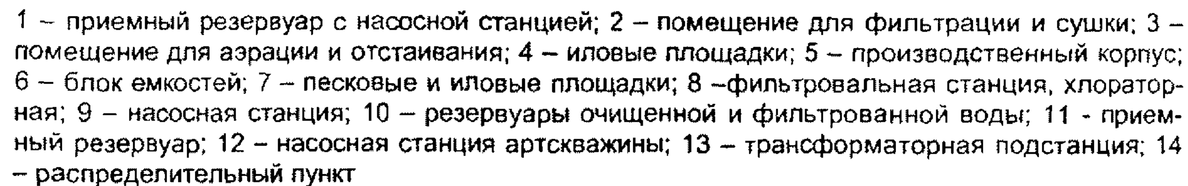
Рисунок Д.6 – Генеральный план сектора обработки навоза на свинокомплексе «Кузнецовский» Московской области
