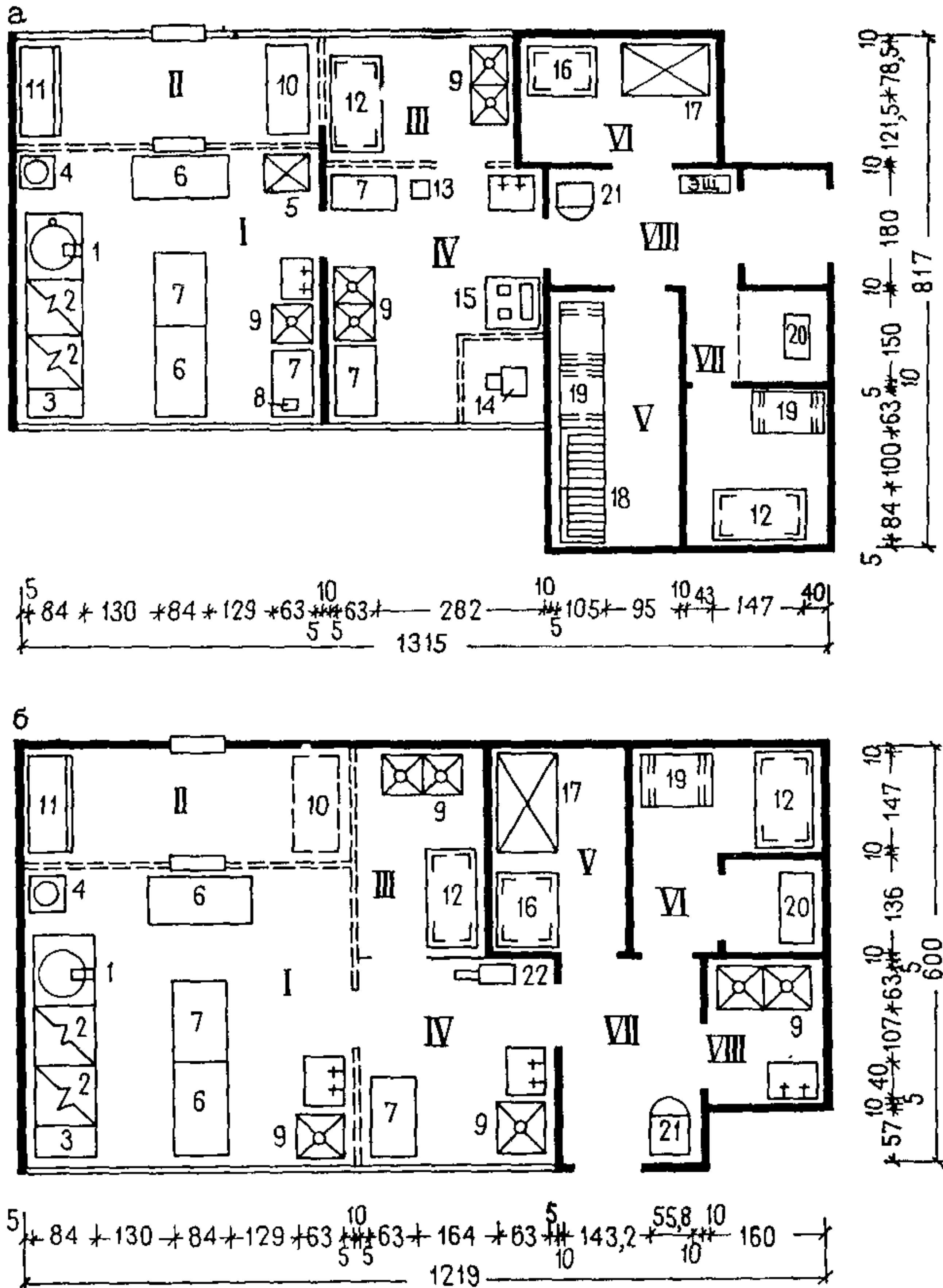
Рис. 31. Функционально-технологическая схема пищеблока яслей-сада на 320 мест
