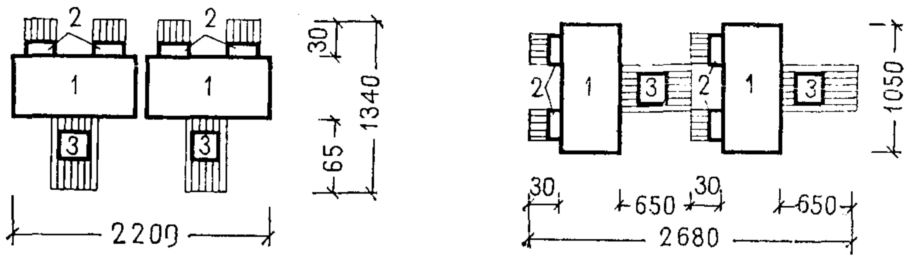
Рис. 22. Примеры расположения столов для кормления детей 1—2 лет
