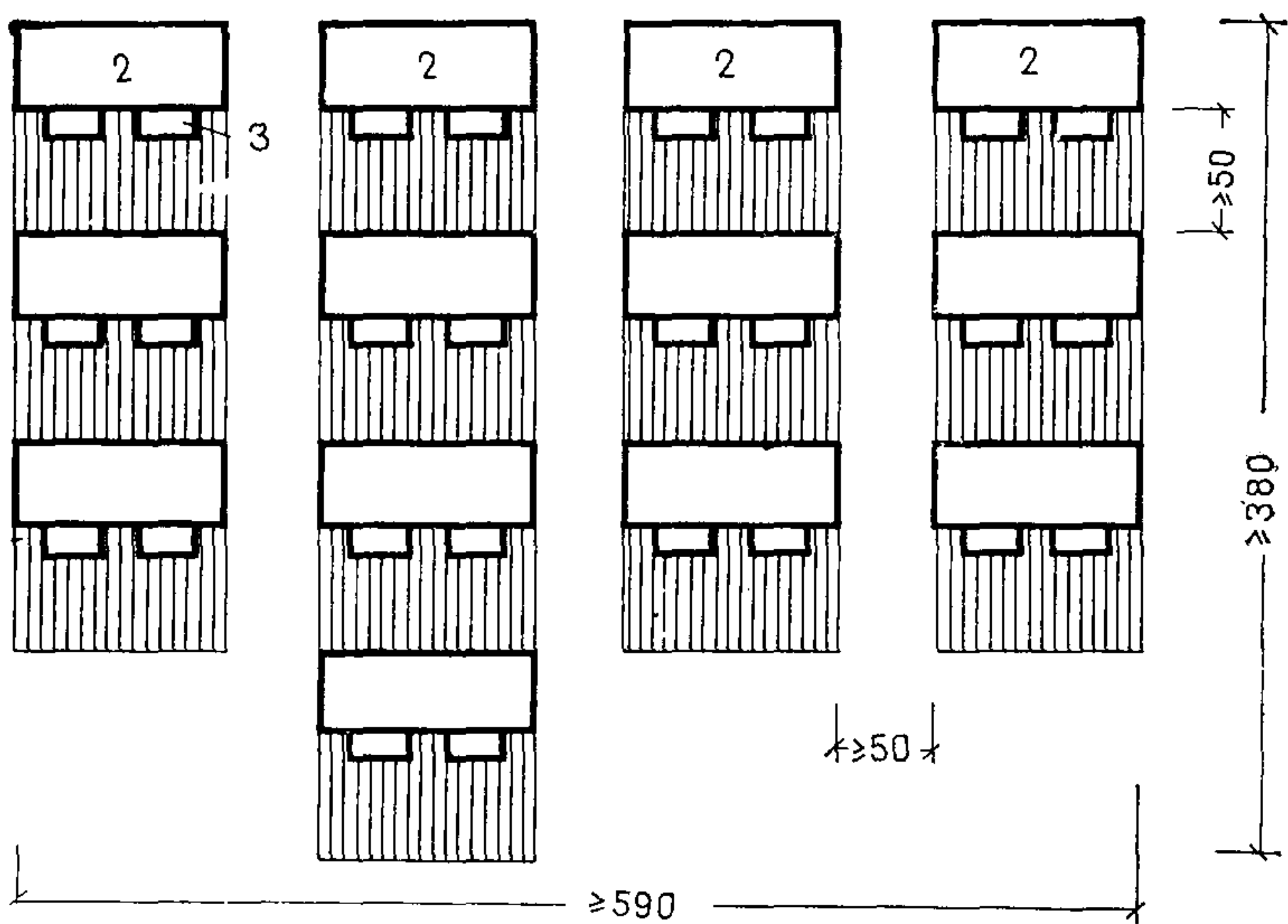
Рис. 23. Варианты размещения детских столов в игральных и групповых помещениях
