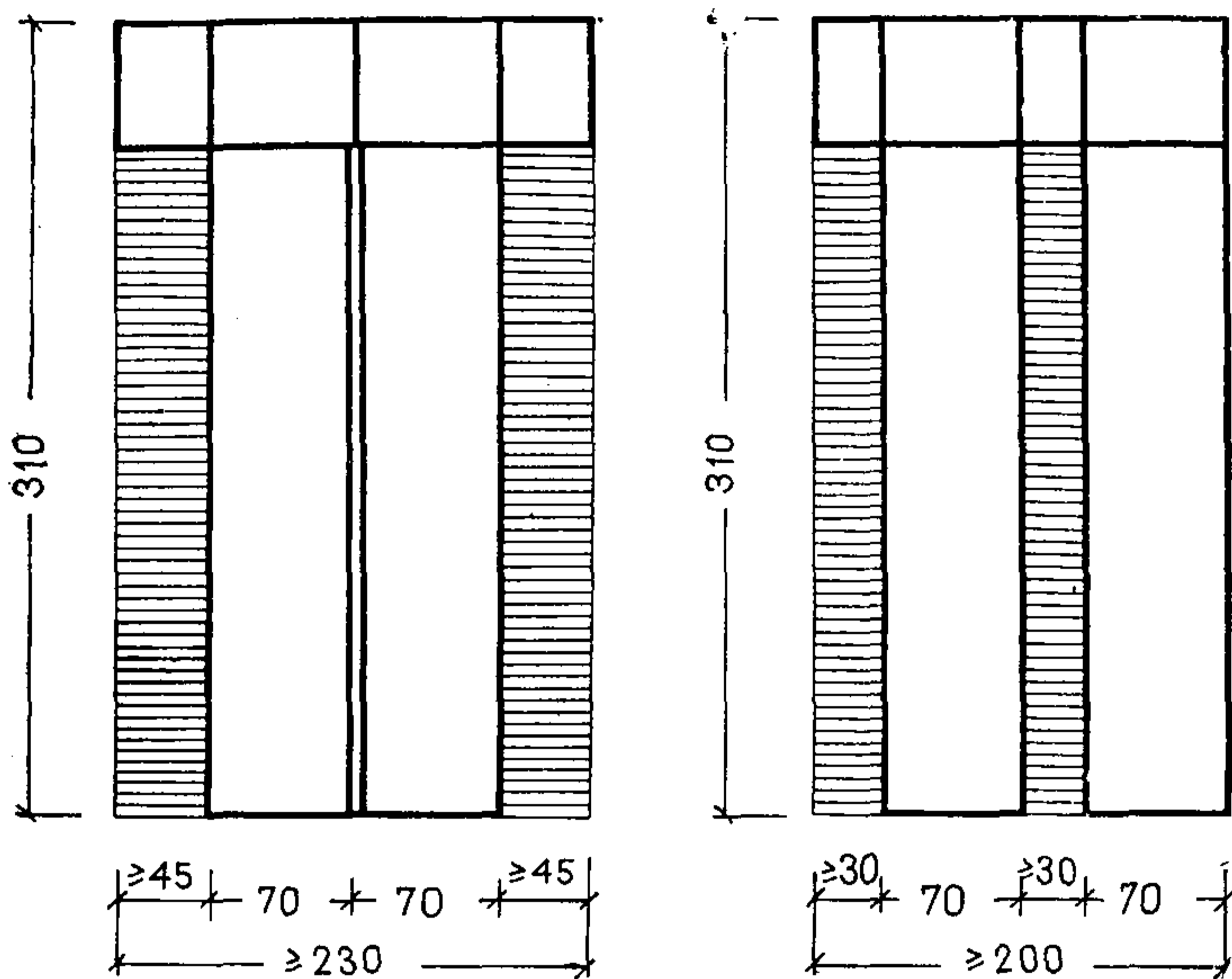
Рис. 27. Функциональные зоны шкафов с откидными кроватями
