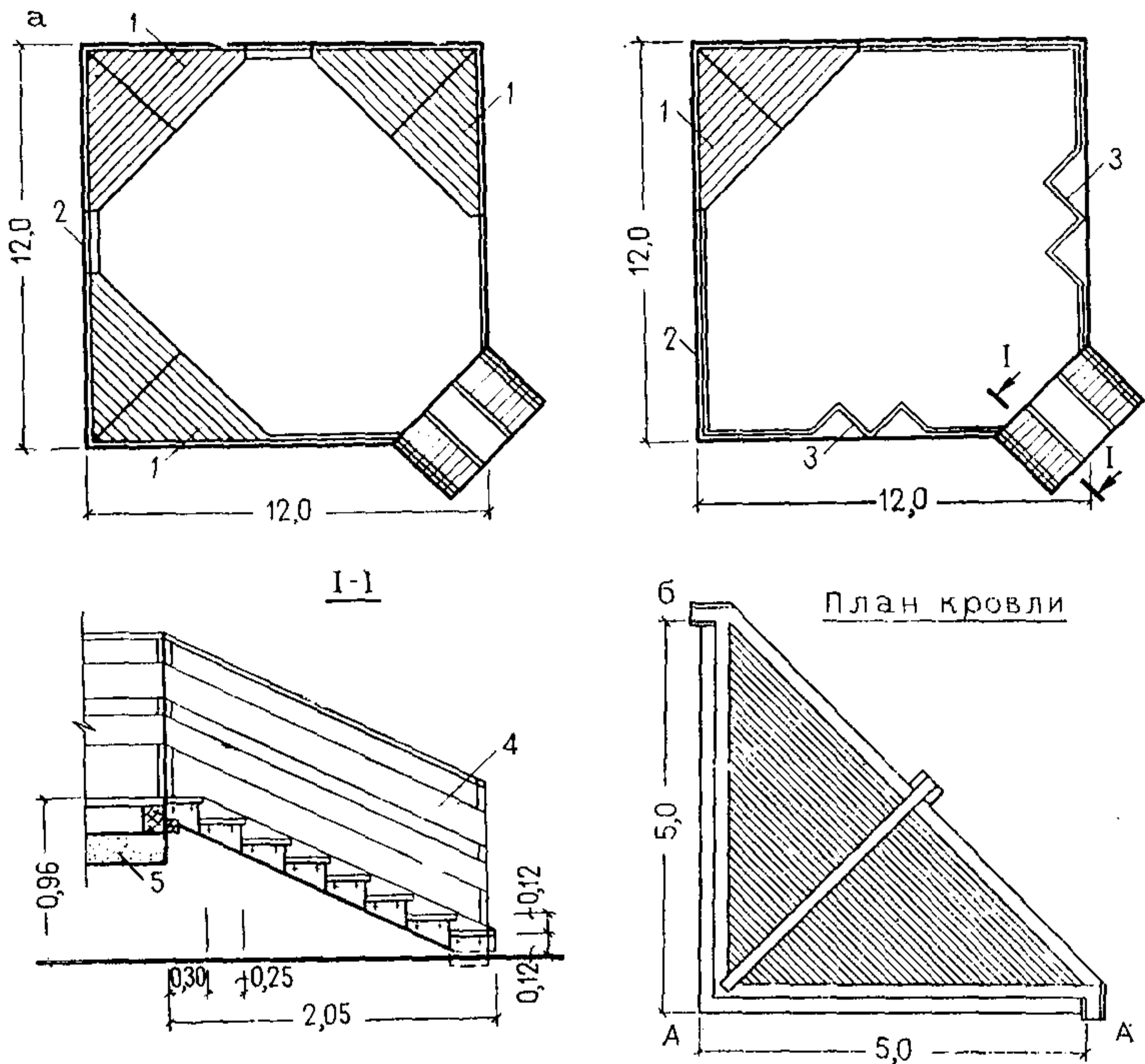
Рис. 6. Примеры решения групповых площадок-платформ для яслей-садов, проектируемых в районах с вечномёрзлыми грунтами
