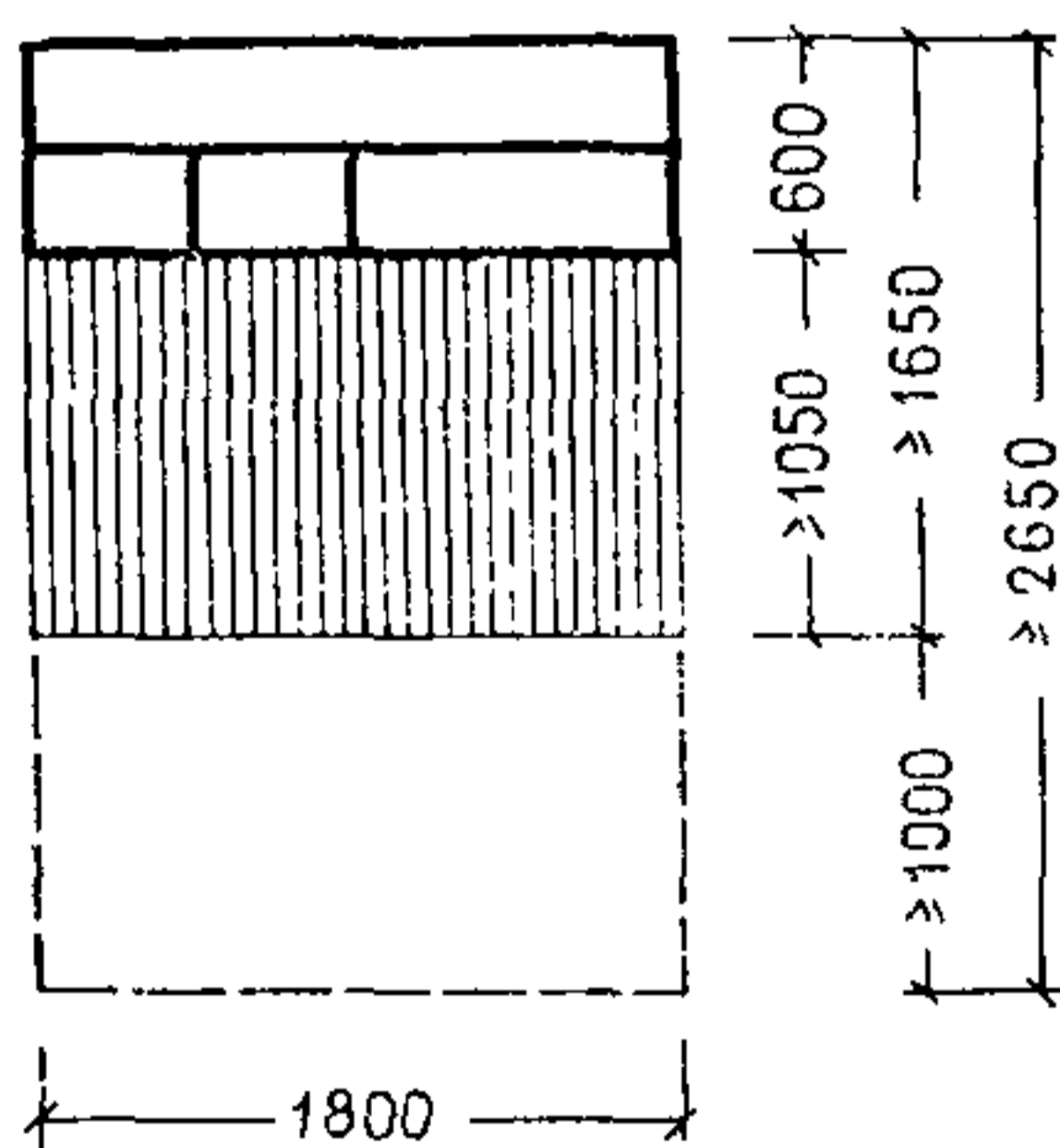
Рис. 25. Функциональная зона буфетной
