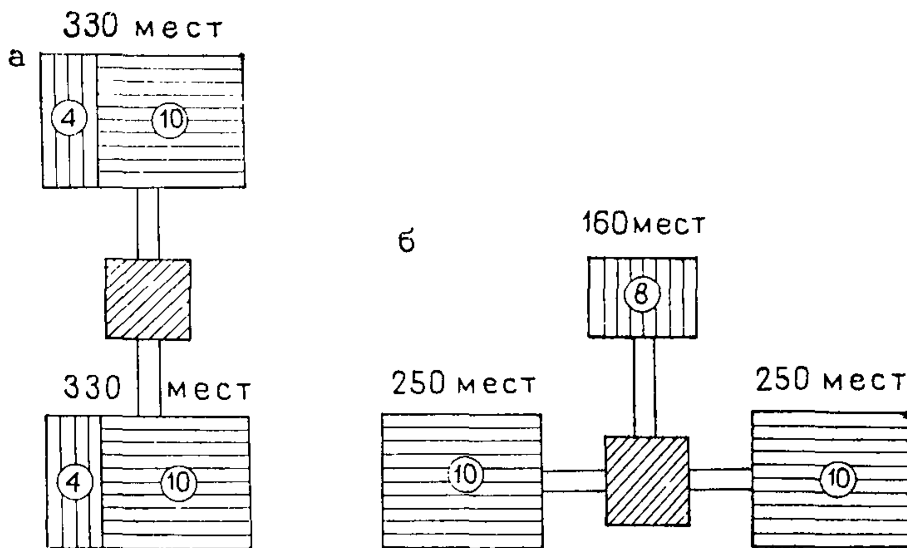
Рис. 13. Схемы комплекса яслей-сада на 660 мест
