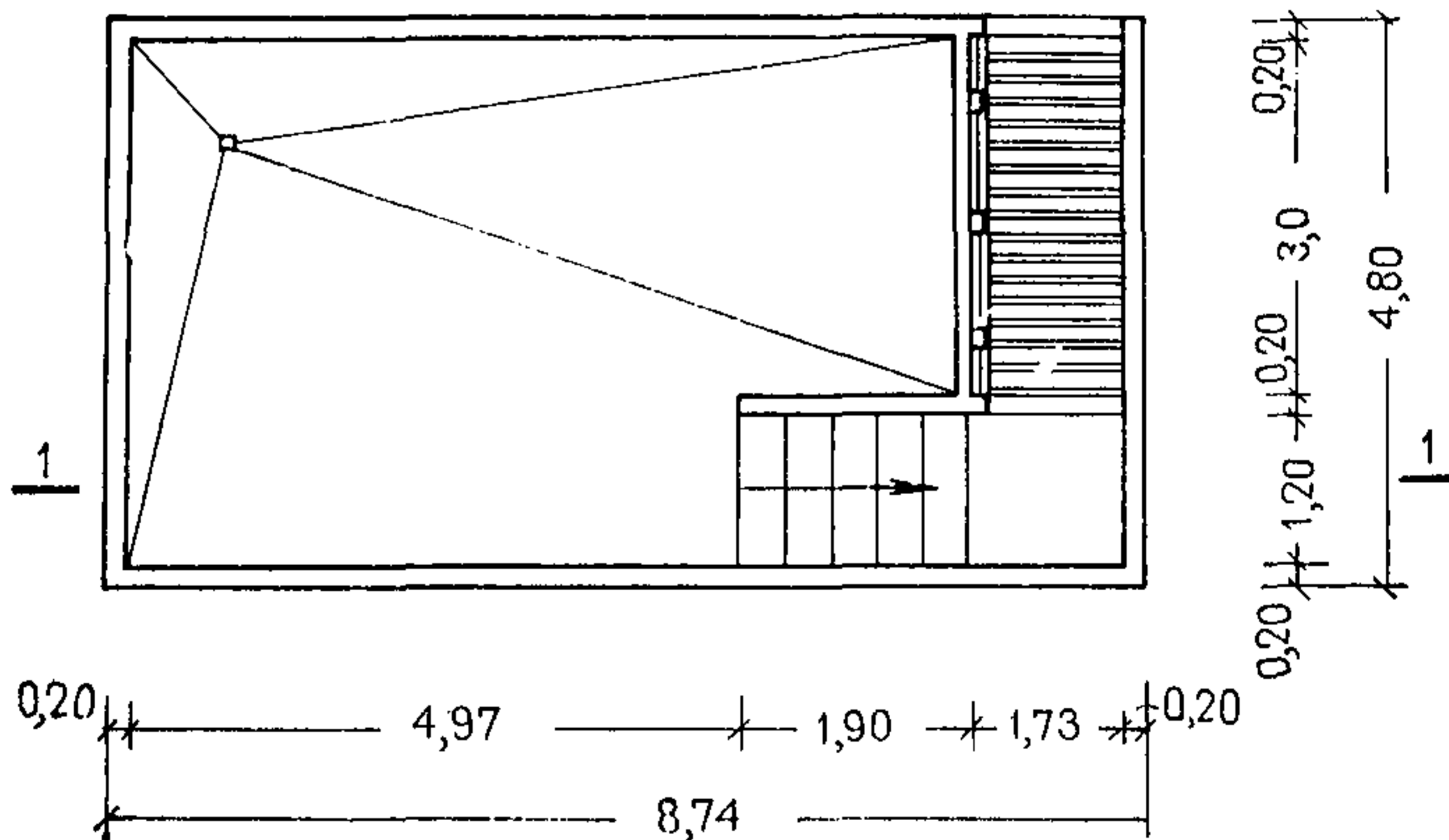
Рис. 9. Пример решения плавательного бассейна
