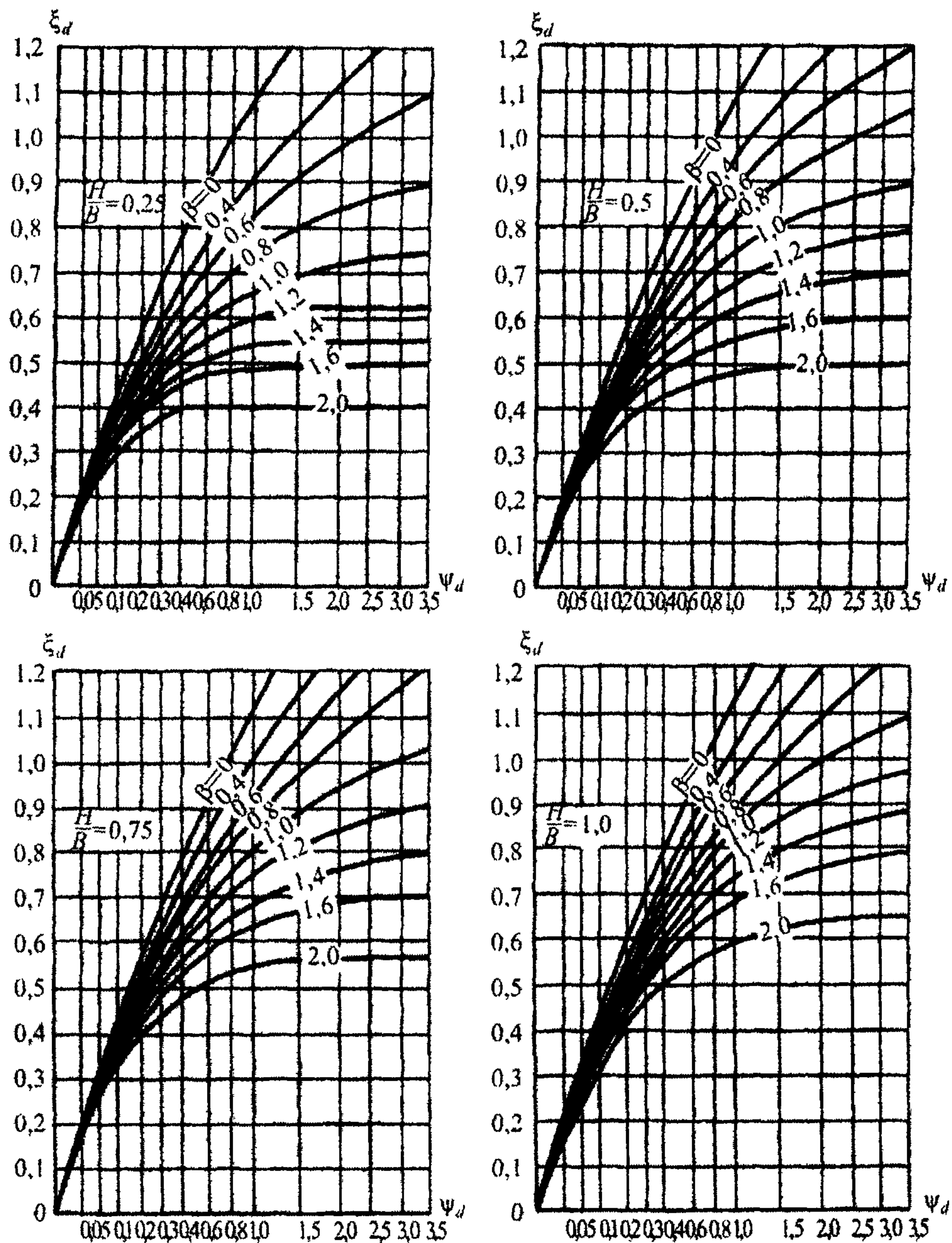
Рисунок К.4 – Графики для определения коэффициента \xi_d
