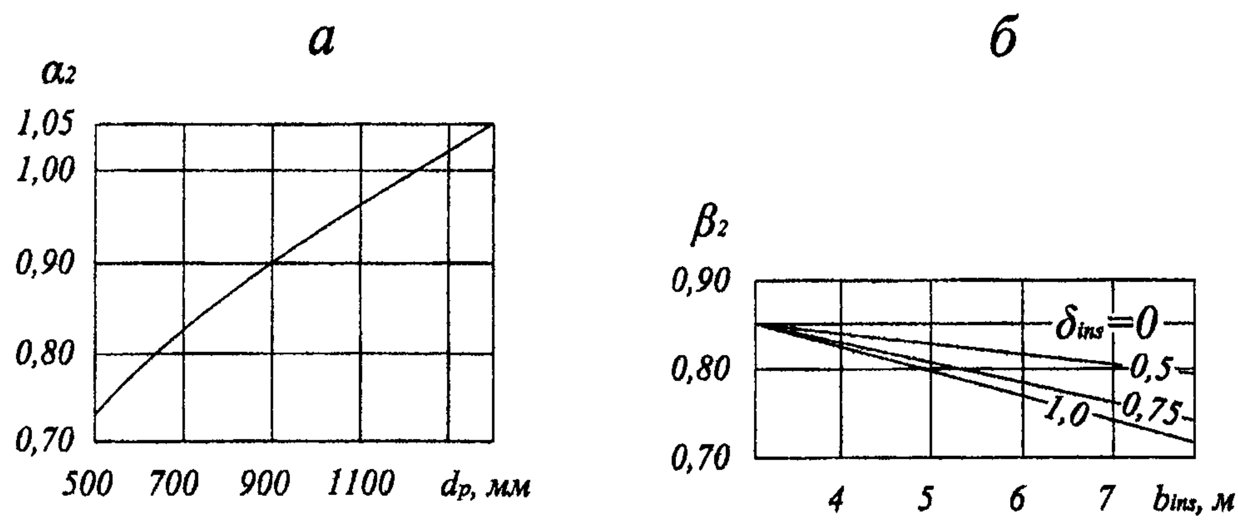
Рисунок Н.4 – Графики для определения коэффициентов \alpha_2 (а) и \beta_2 (б) при расчете многолетнего оттаивания ММГ под теплыми и горячими трубопроводами
