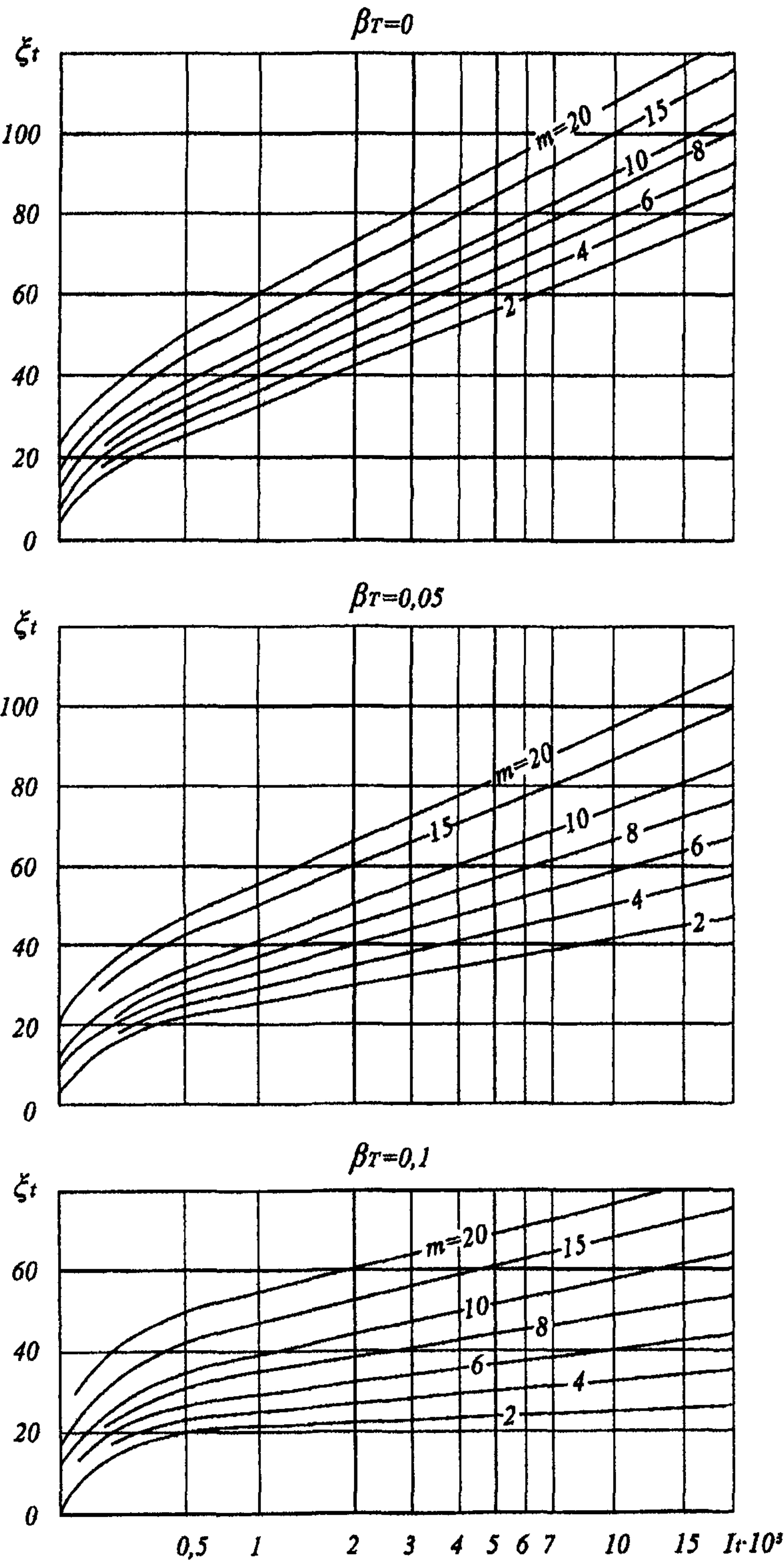
Рисунок Н.2 – Номограмма для определения многолетнего оттаивания ММГ вокруг теплого и горячего трубопроводов
