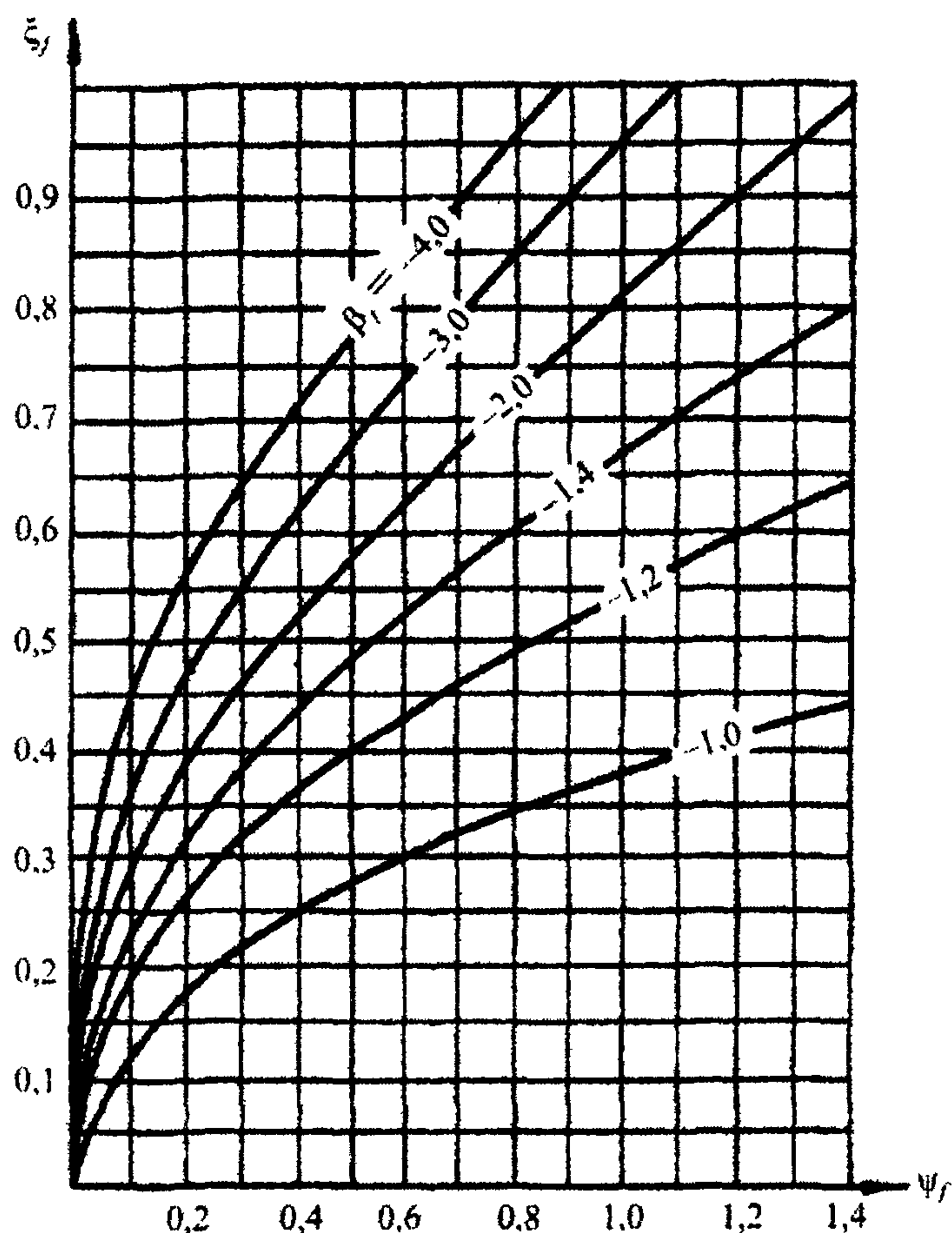
Рисунок Е.1 – Графики для определения коэффициента \beta_f
