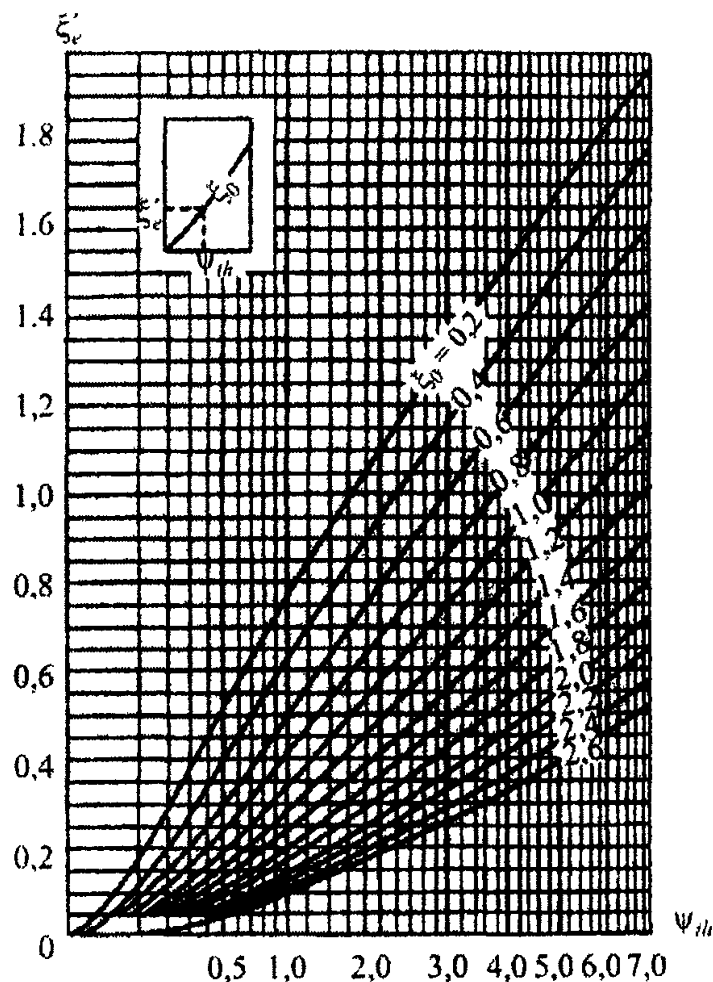
Рисунок К.6 – Графики для определения коэффициента \xi'_e
