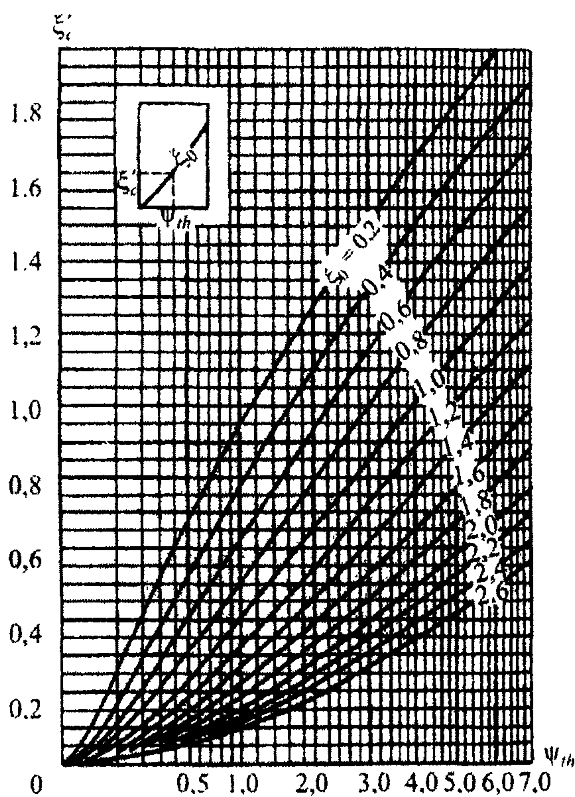
Рисунок К.5 – Графики для определения коэффициента \xi'_c
