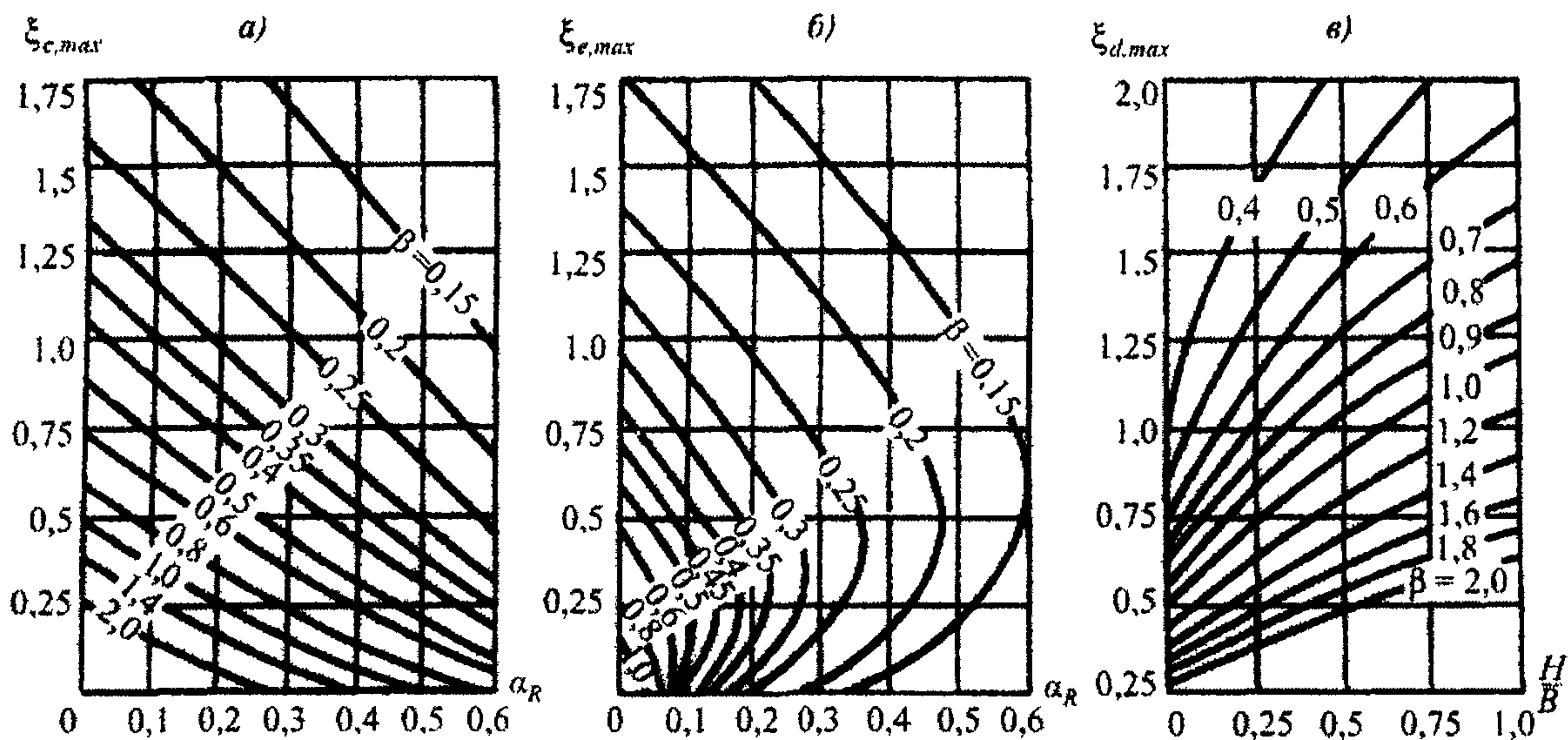
Рисунок К.3 – Графики для определения коэффициентов: а – \xi_{с, max} ; б – \xi_{е, max} ; в – \xi_{d, max}
