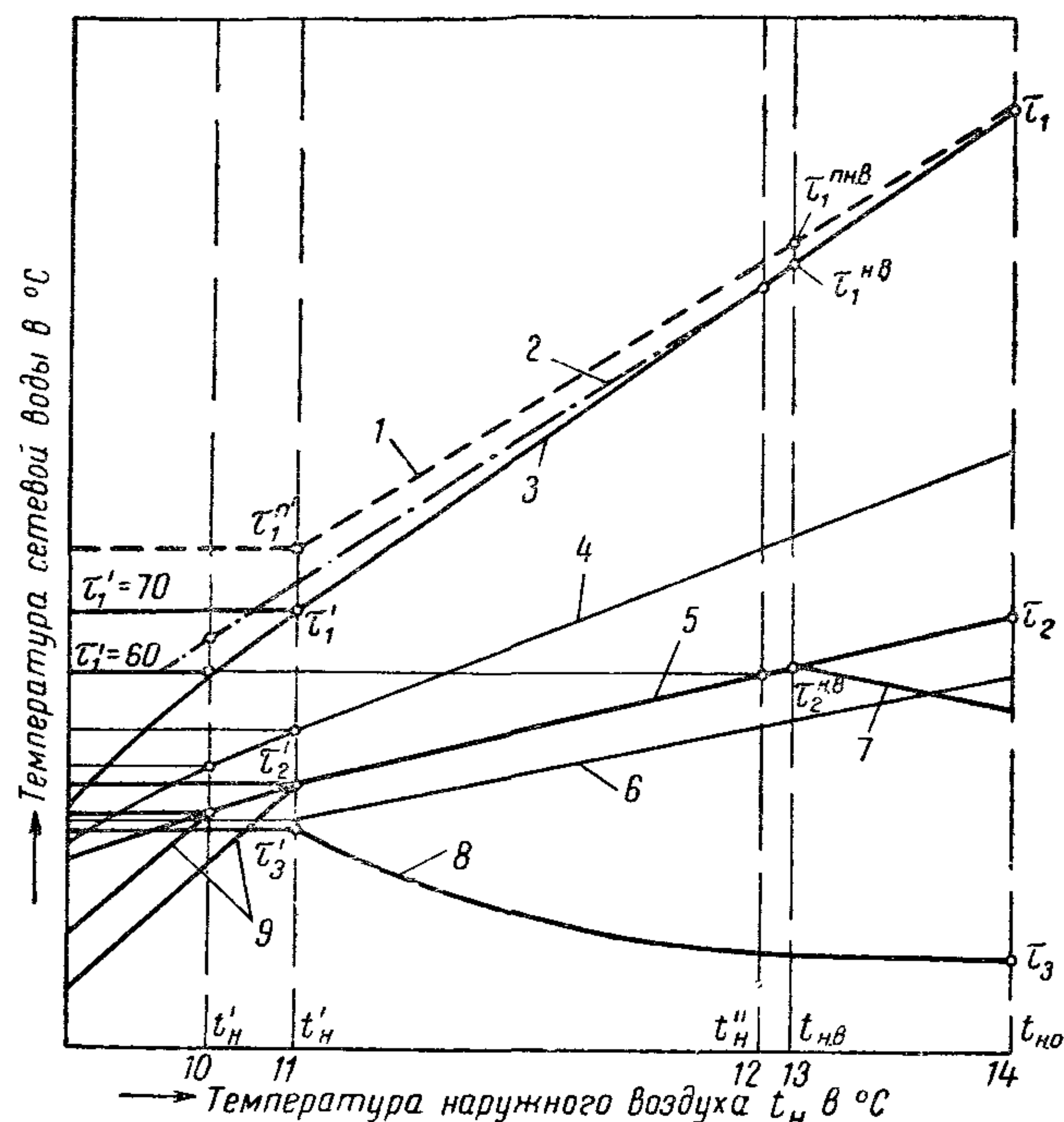
Рис. 1. Графики температур воды в тепловых сетях
