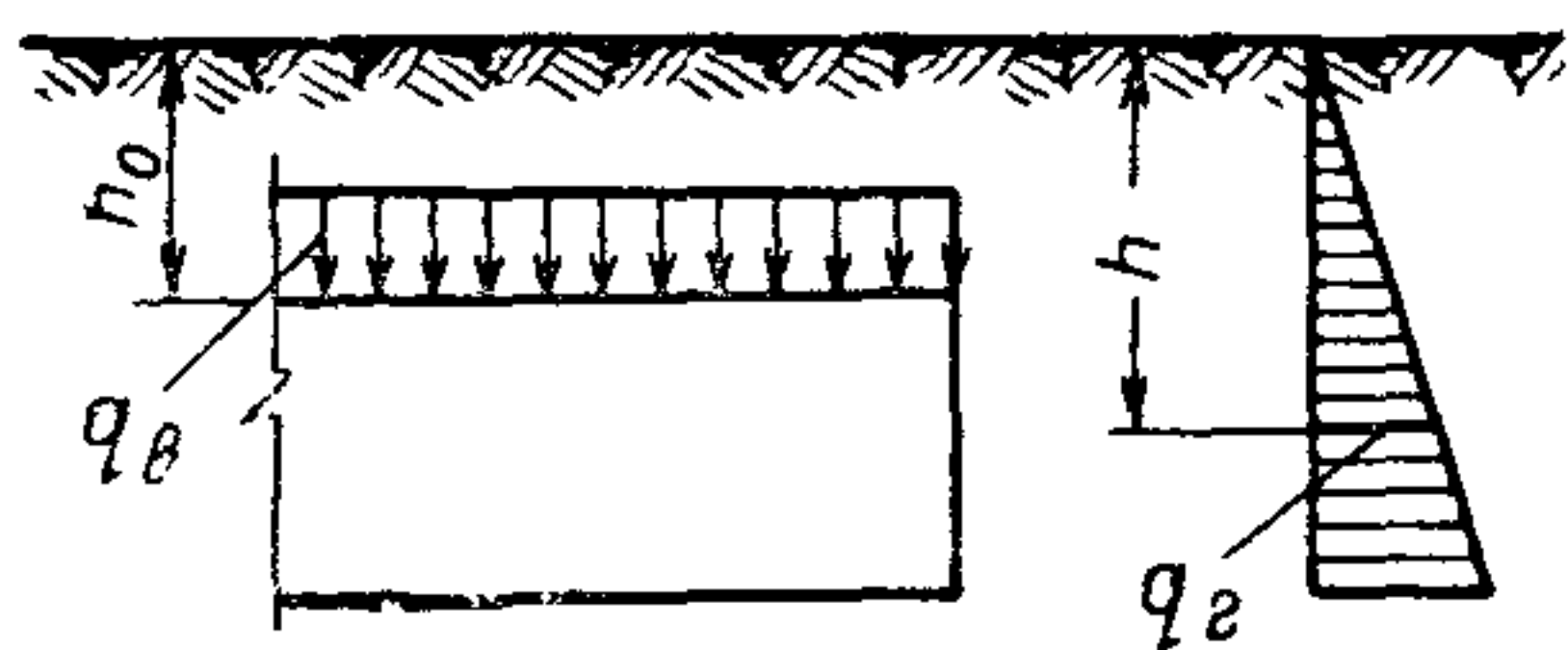
Рис. 4. Схема нагрузок от грунта
