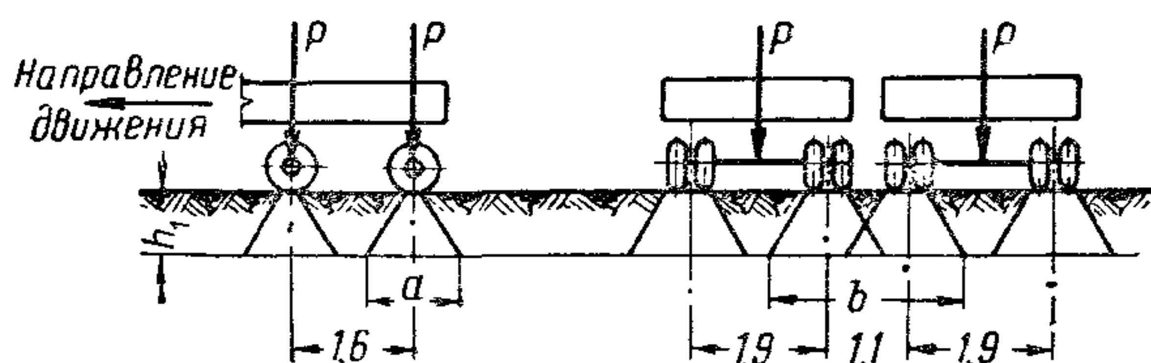
Рис. 2. Схема распределения вертикальной нагрузки от колес автомобилей
