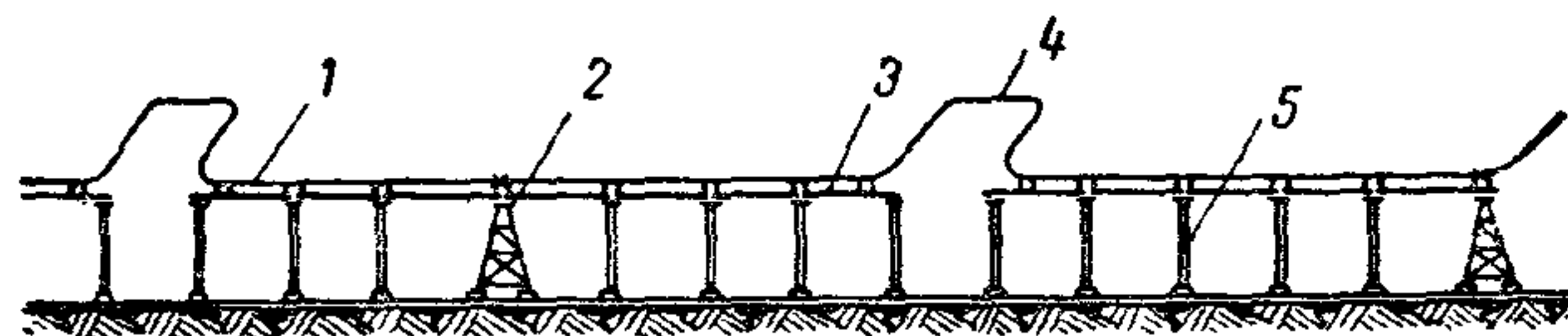
Рис. 5. Схема расстановки компенсаторов
