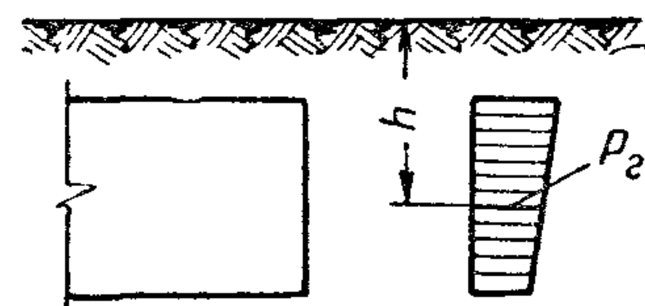
Рис. 3. Схема горизонтальных нагрузок от транспортных единиц
