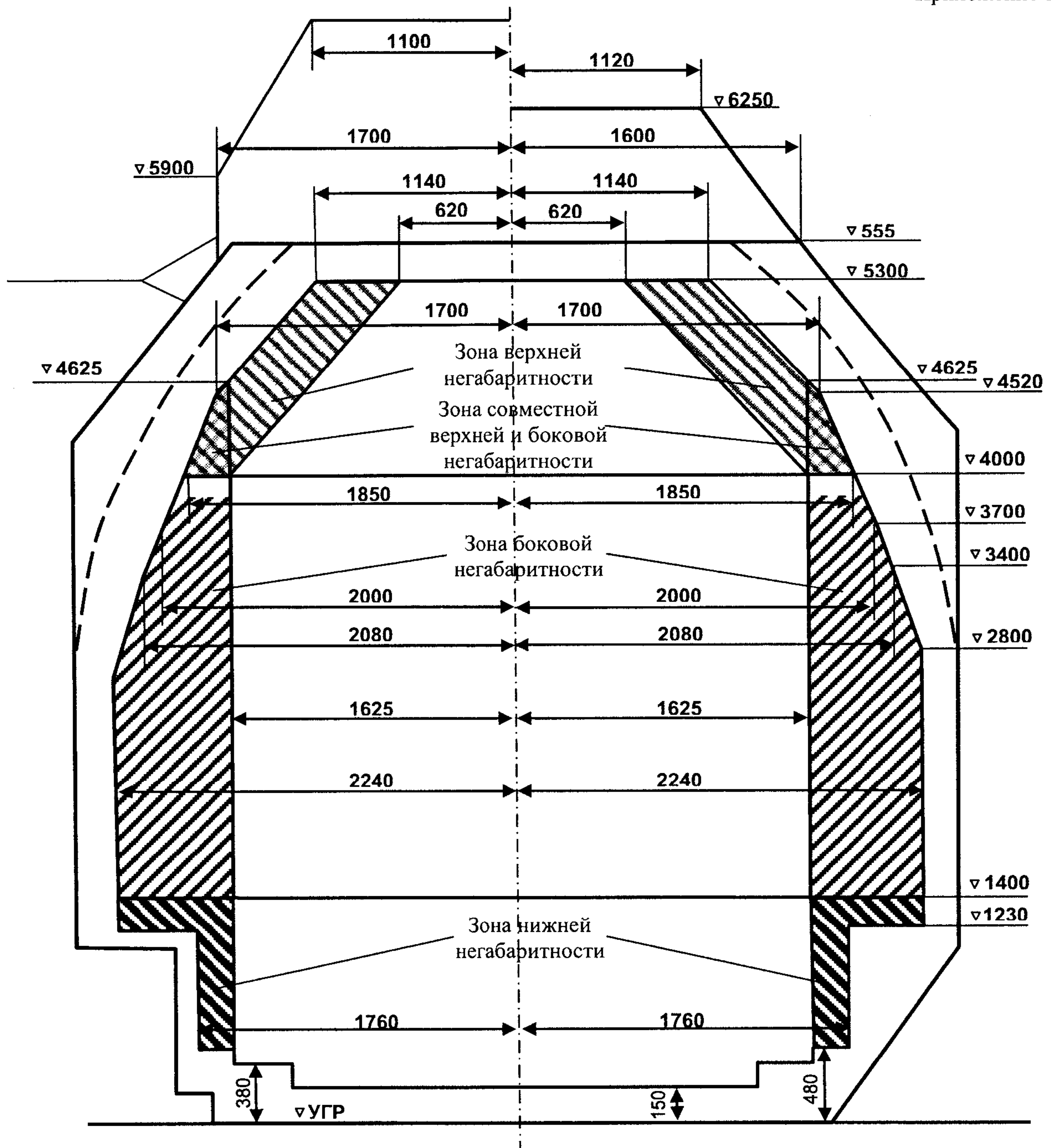
Рис.1. Зоны негабаритности груза
