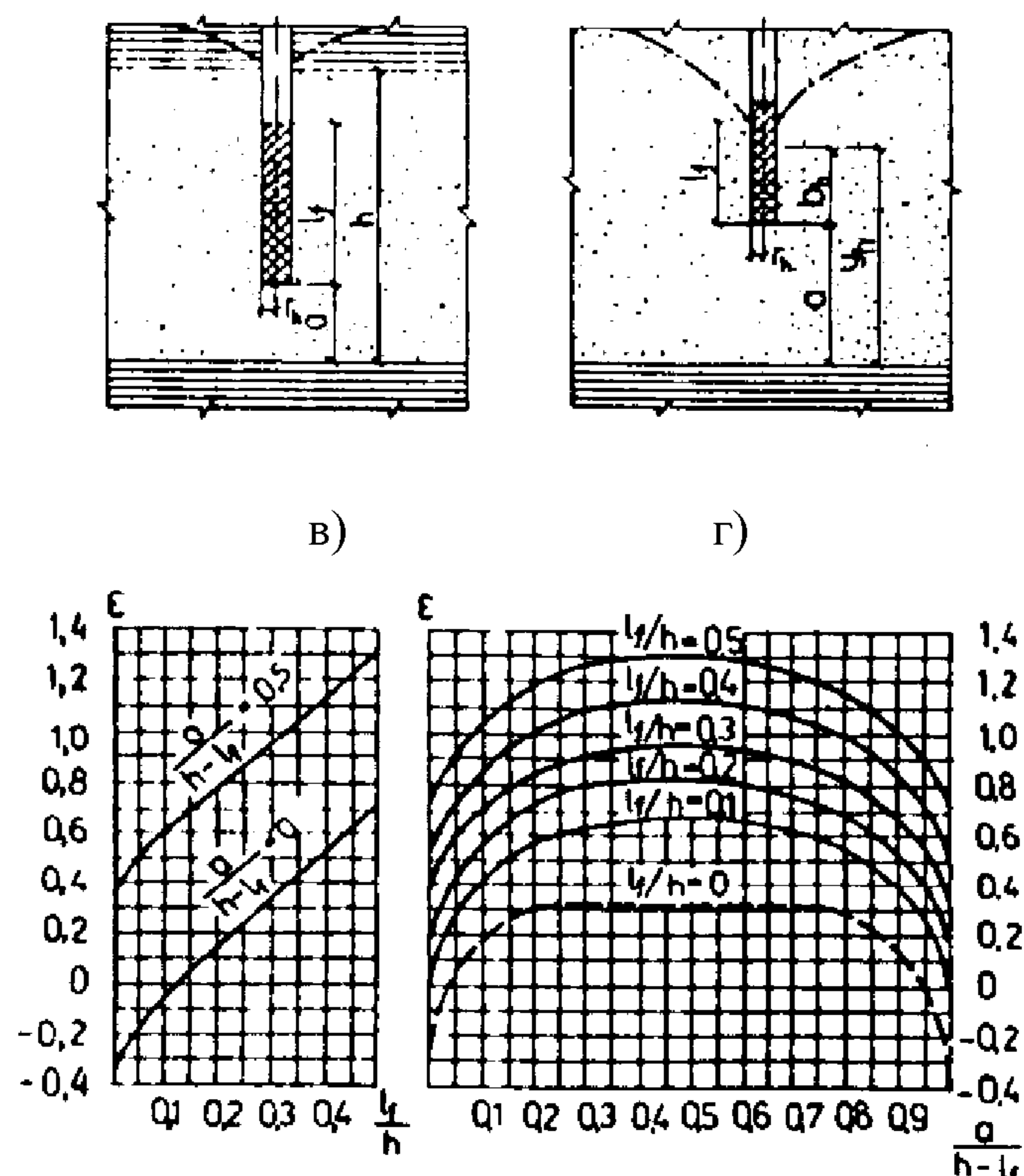
Черт. 3. К расчету сопротивления скважин на гидрологическое несовершенство а, б - схемы несовершенных скважин в напорном и безнапорном пластах; а, г - графики для определения \epsilon
