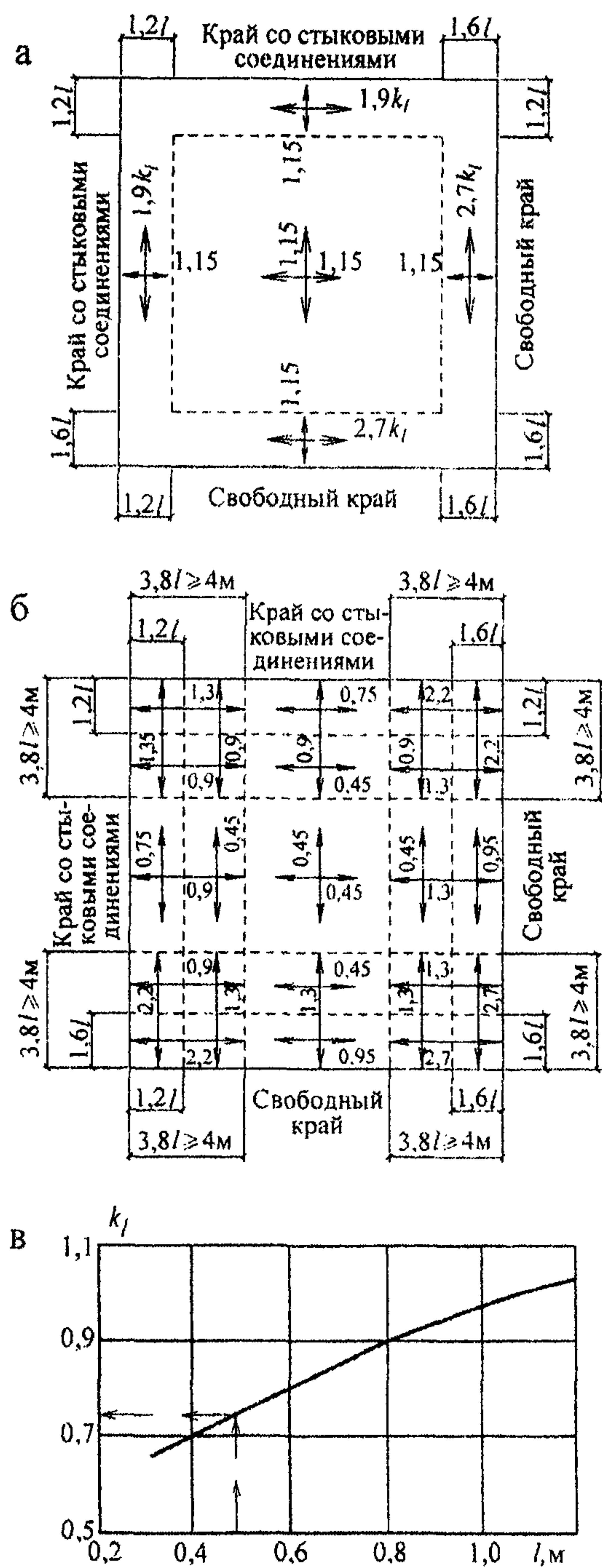
а – для положительных изгибающих моментов; б – для отрицательных изгибающих моментов; в – график для определения поправочного коэффициента k_l к переходному коэффициенту k
