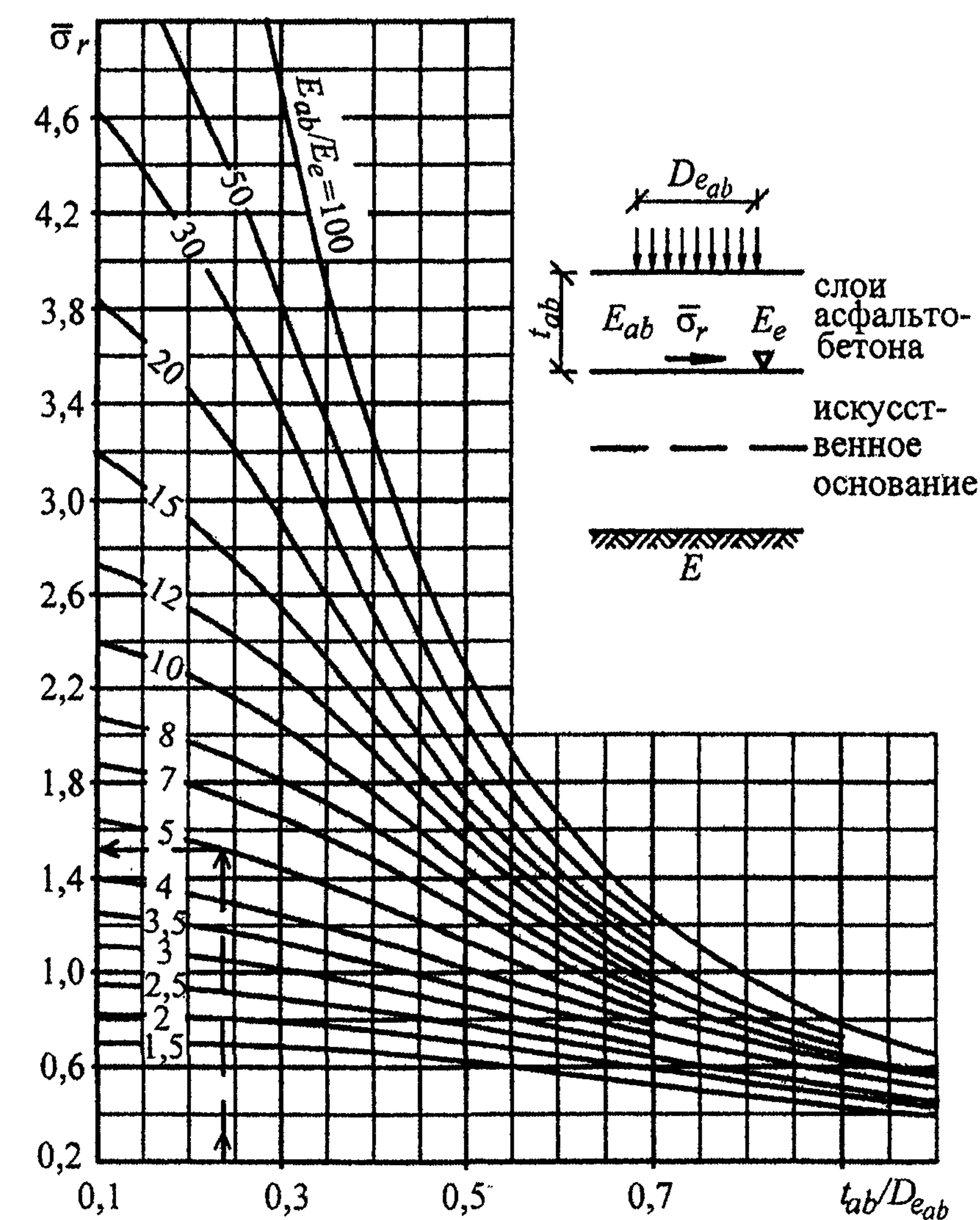
Рисунок К.6 – Номограмма для определения удельных растягивающих напряжений при изгибе \bar{\sigma}_r в асфальтобетоне
