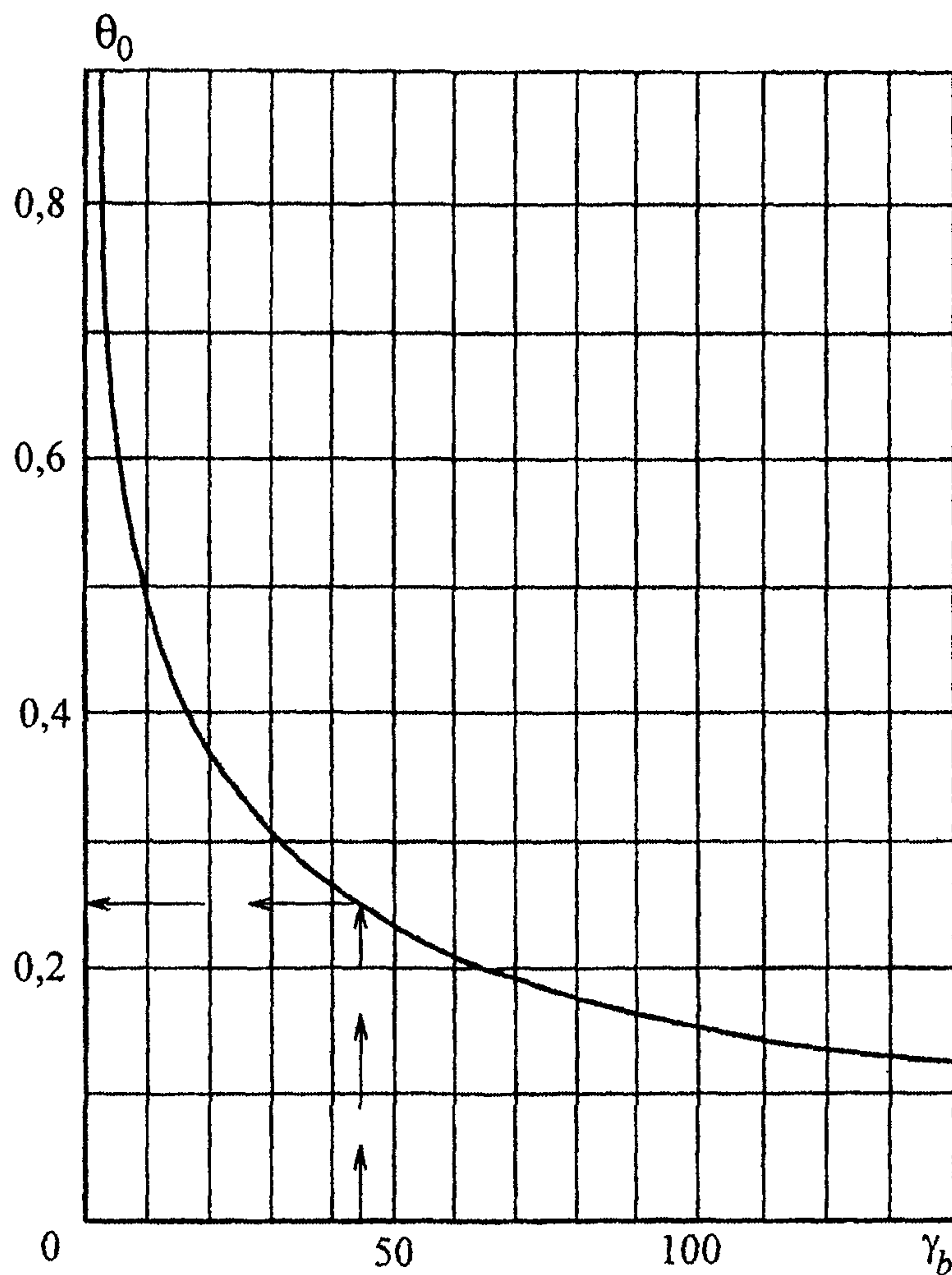
Рисунок М.1 – График для определения \theta_0
