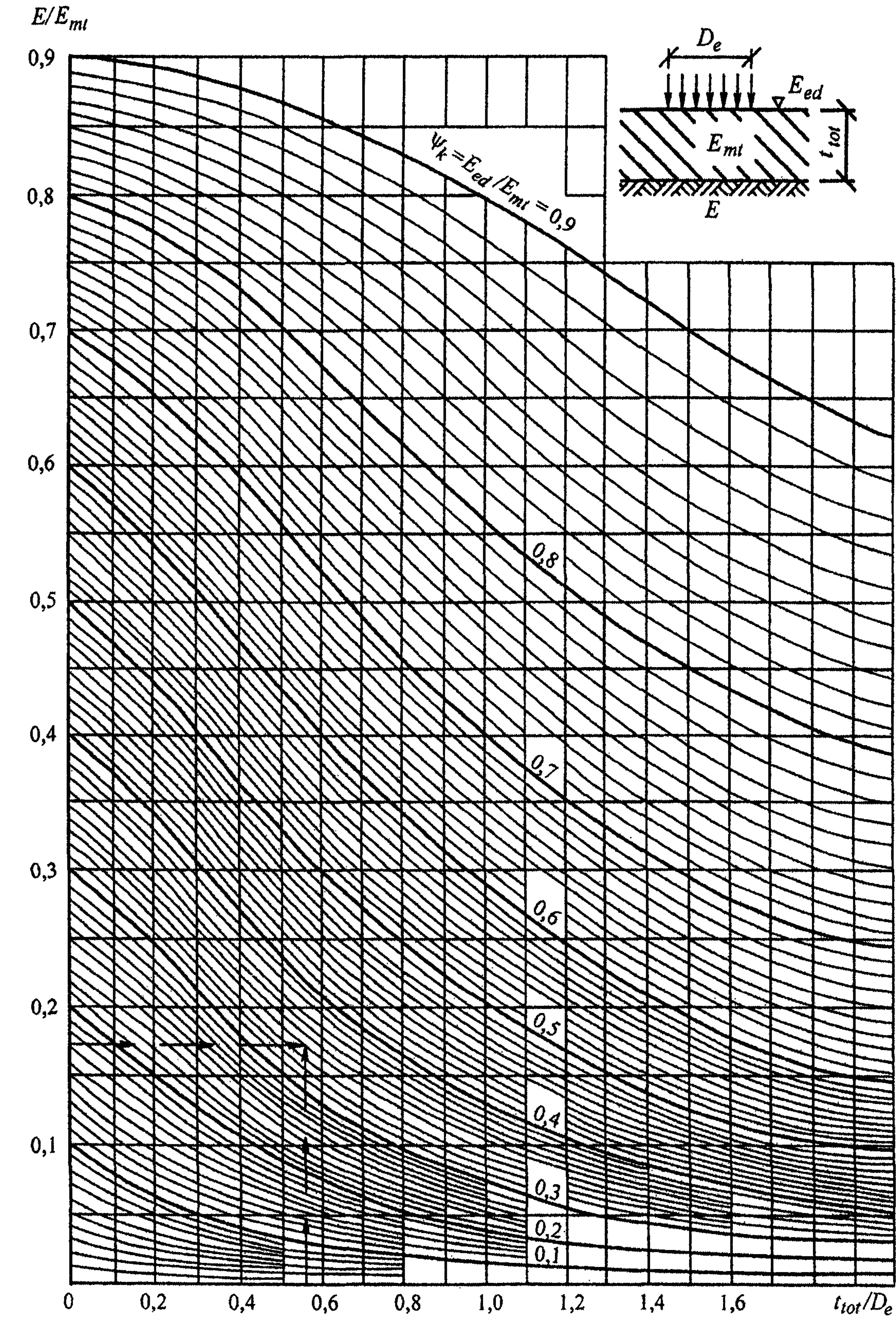
Рисунок К.4 – Номограмма для определения коэффициента \Psi_k
