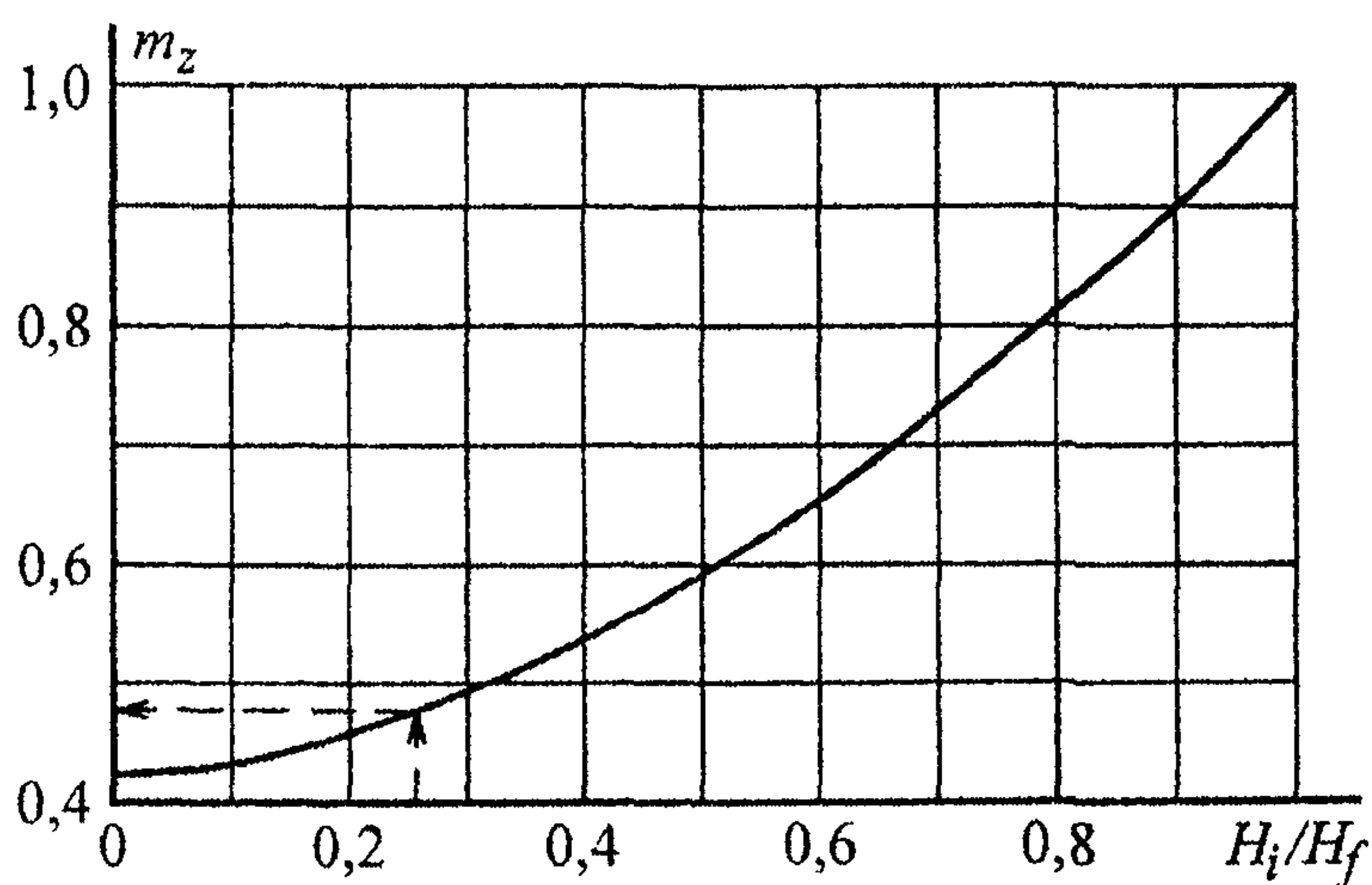
Рисунок Е.2 – График для определения коэффициента m_z
