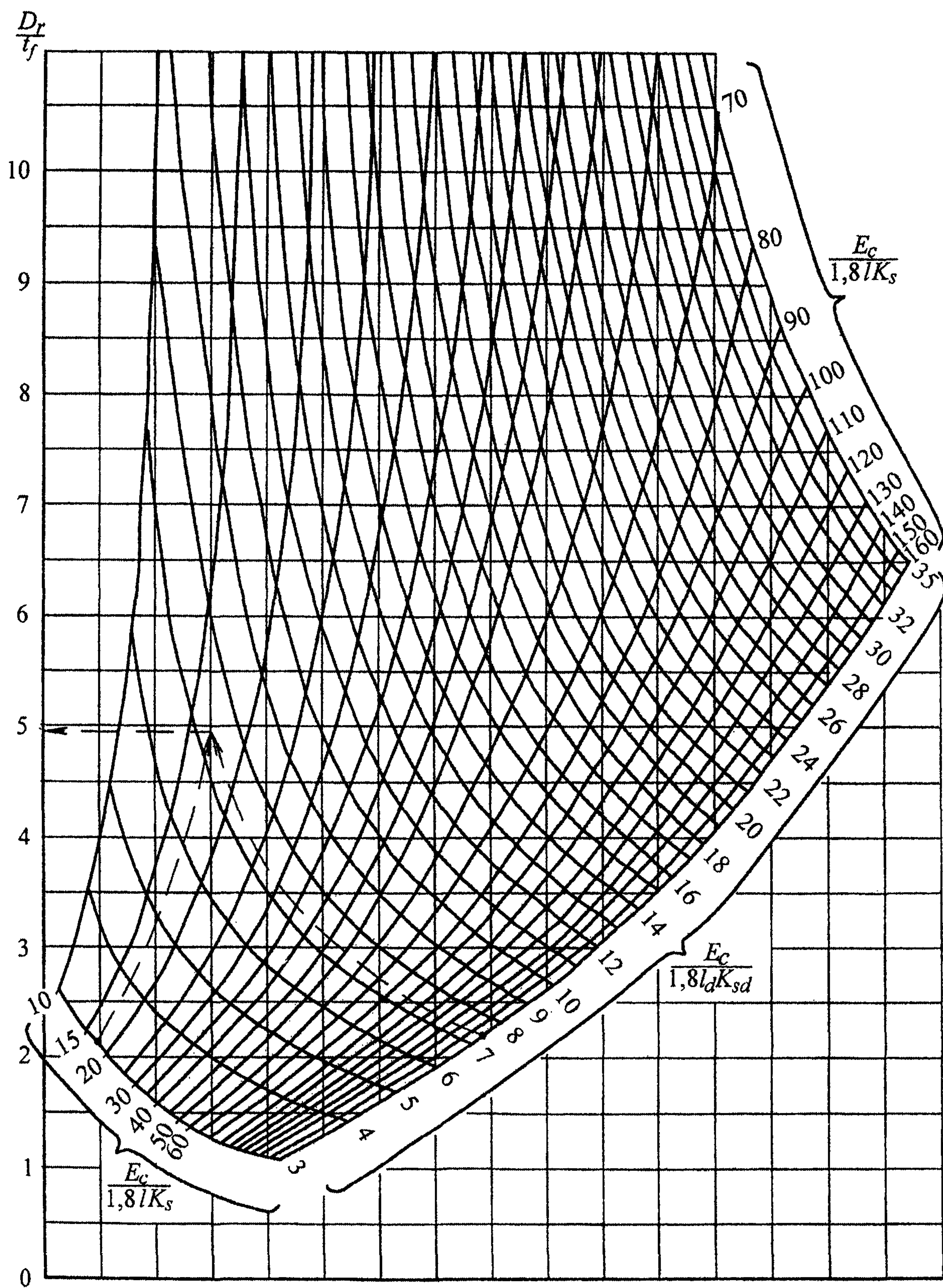
Рисунок М.2 – Номограмма для определения соотношения \frac{D_r}{t_f}
