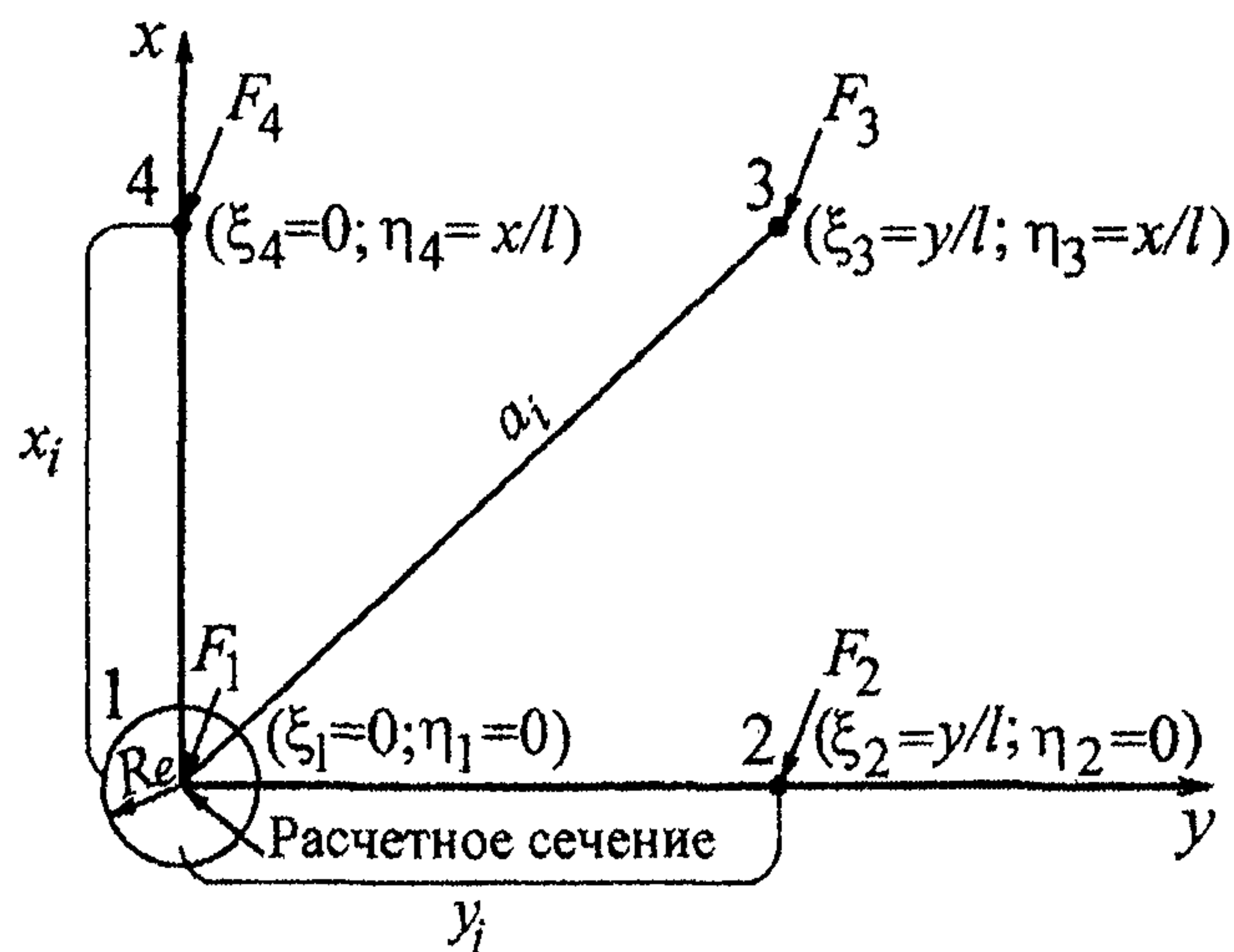
Рисунок 7.2 – Расчетная схема параметров загрузки опор воздушного судна
