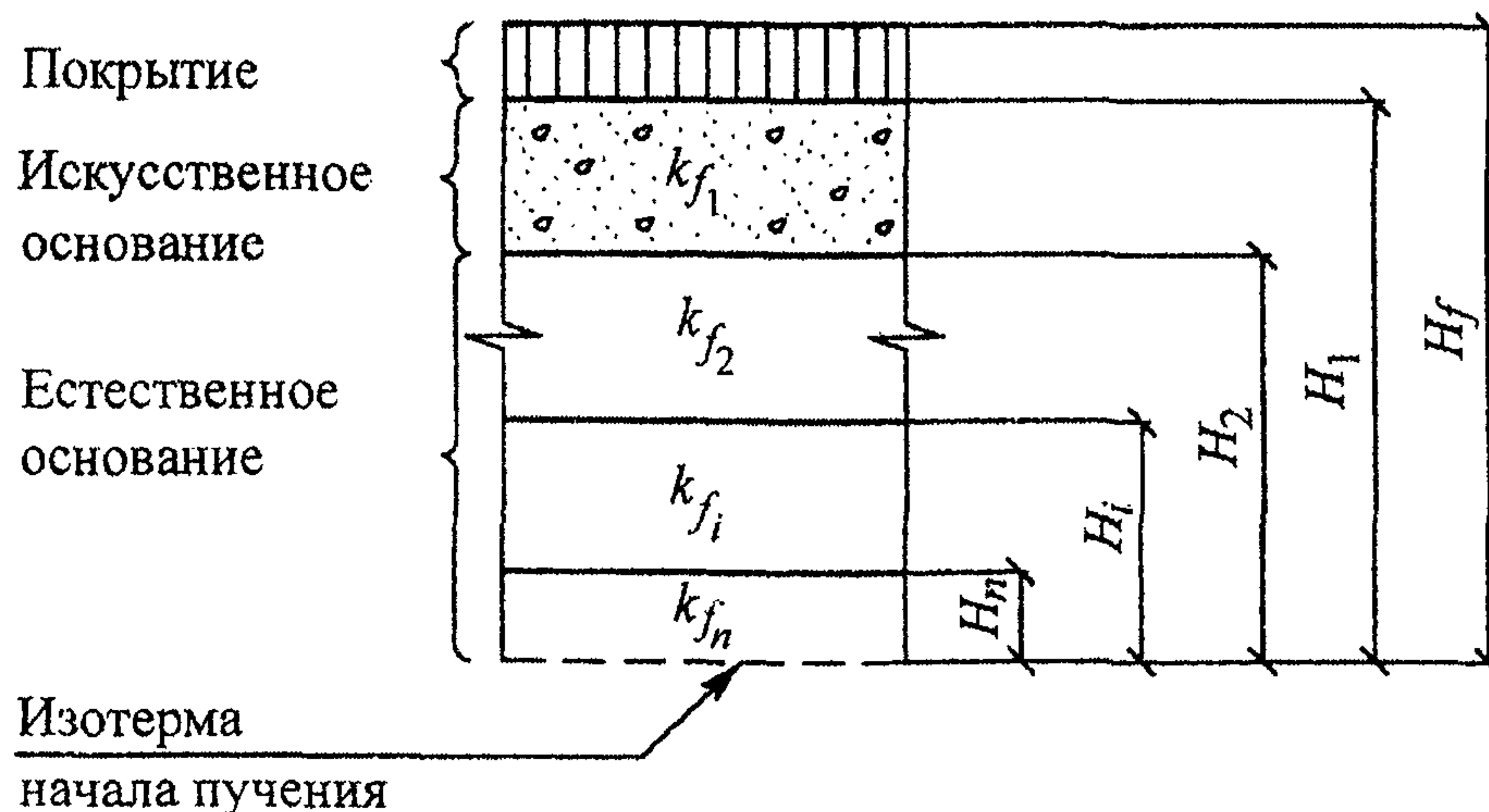
Рисунок Е.1 – Расчетная схема слоистого основания
