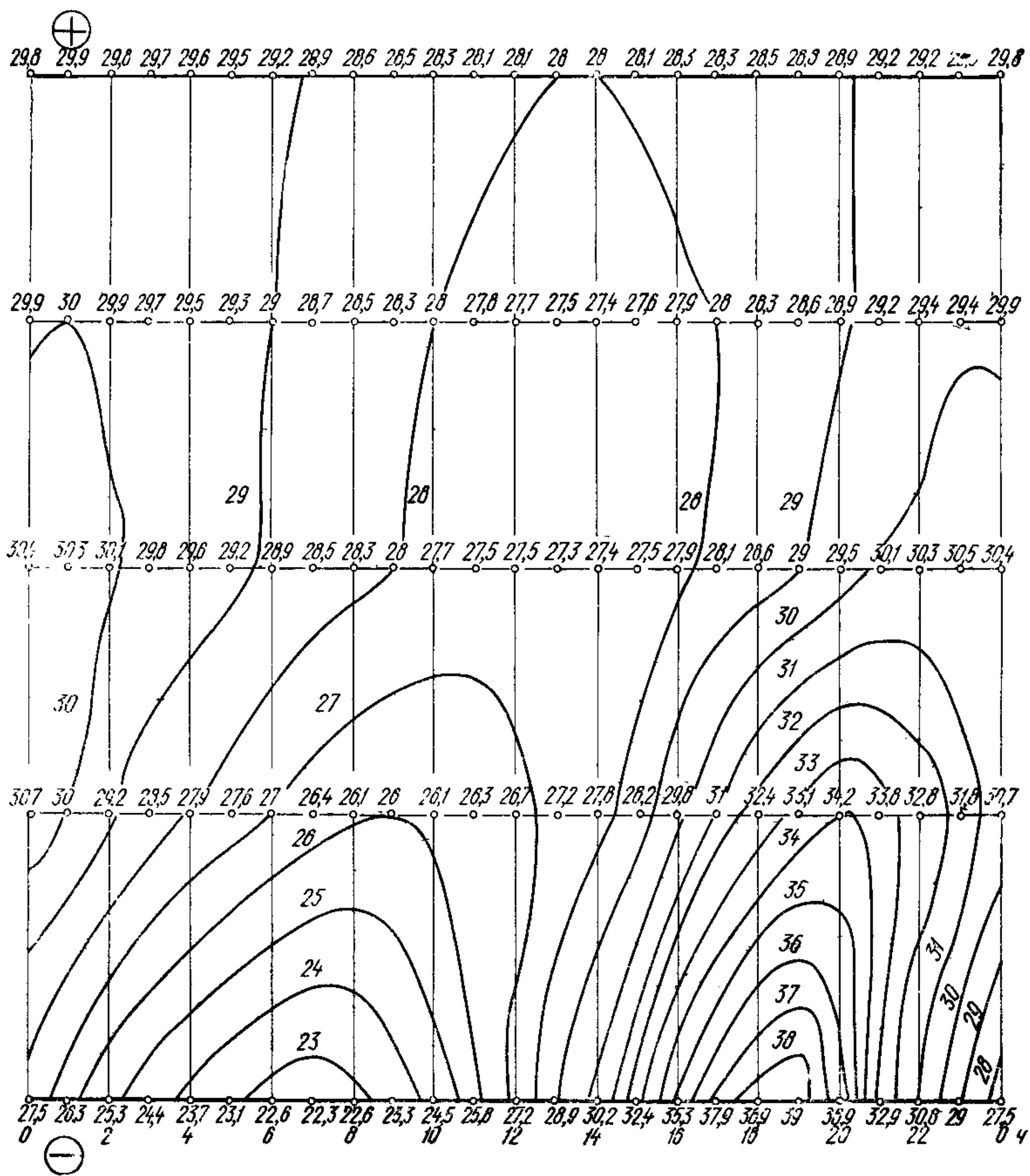
Рис. 7. Термоизоплеты стены
