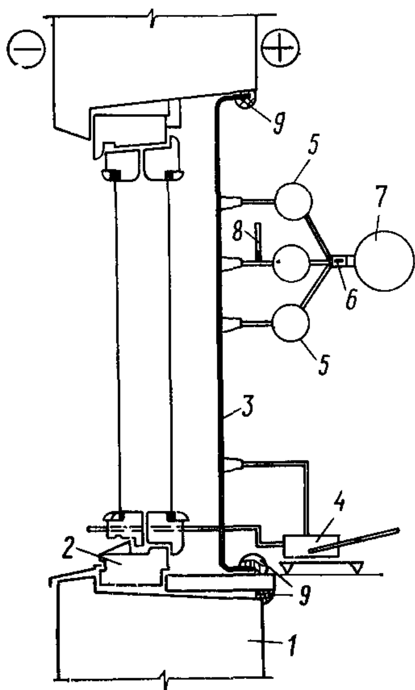
Рис. 11. Схема установки для испытания окна на воздухопроницаемость
