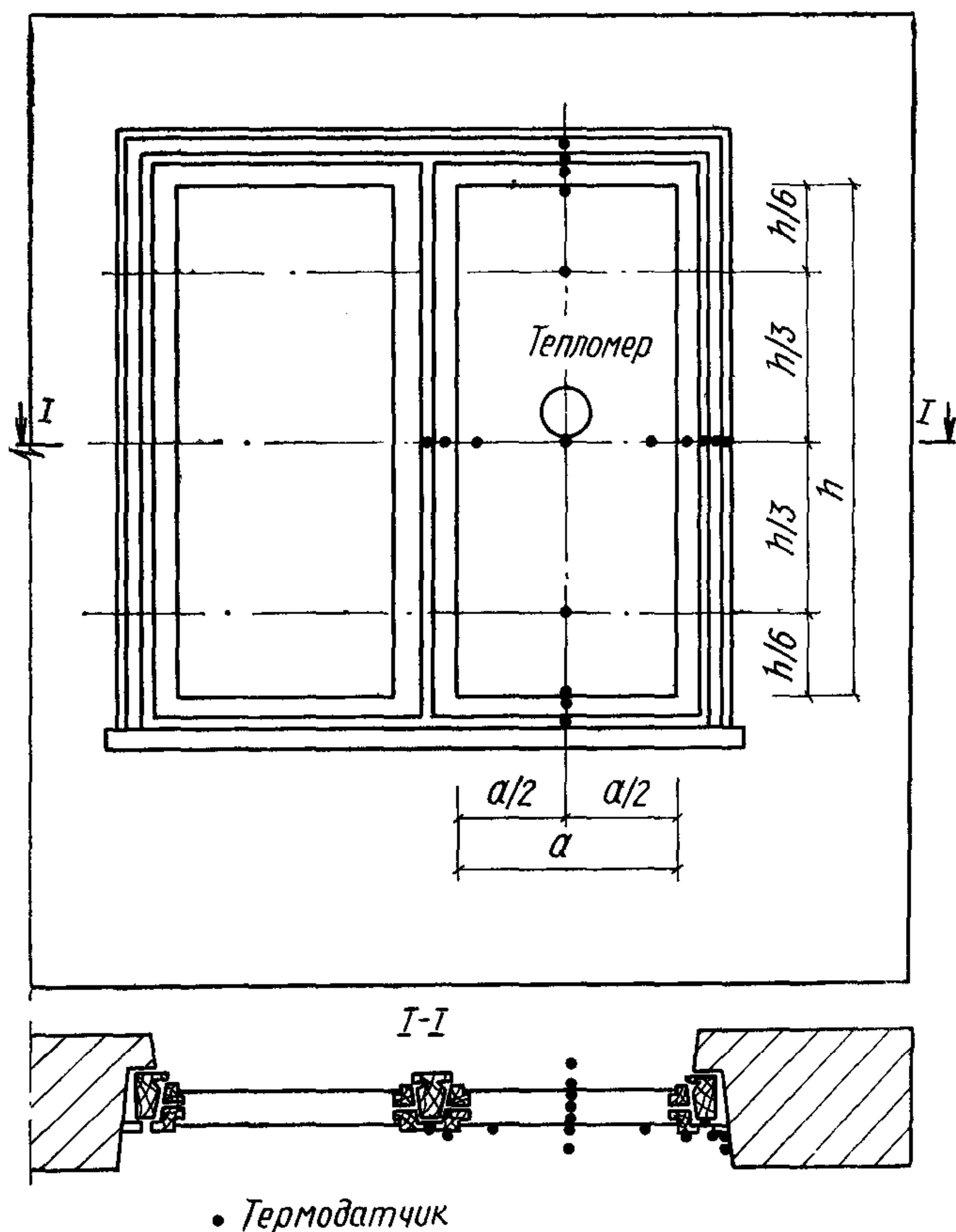
Рис. 2. Размещение датчиков на окне
