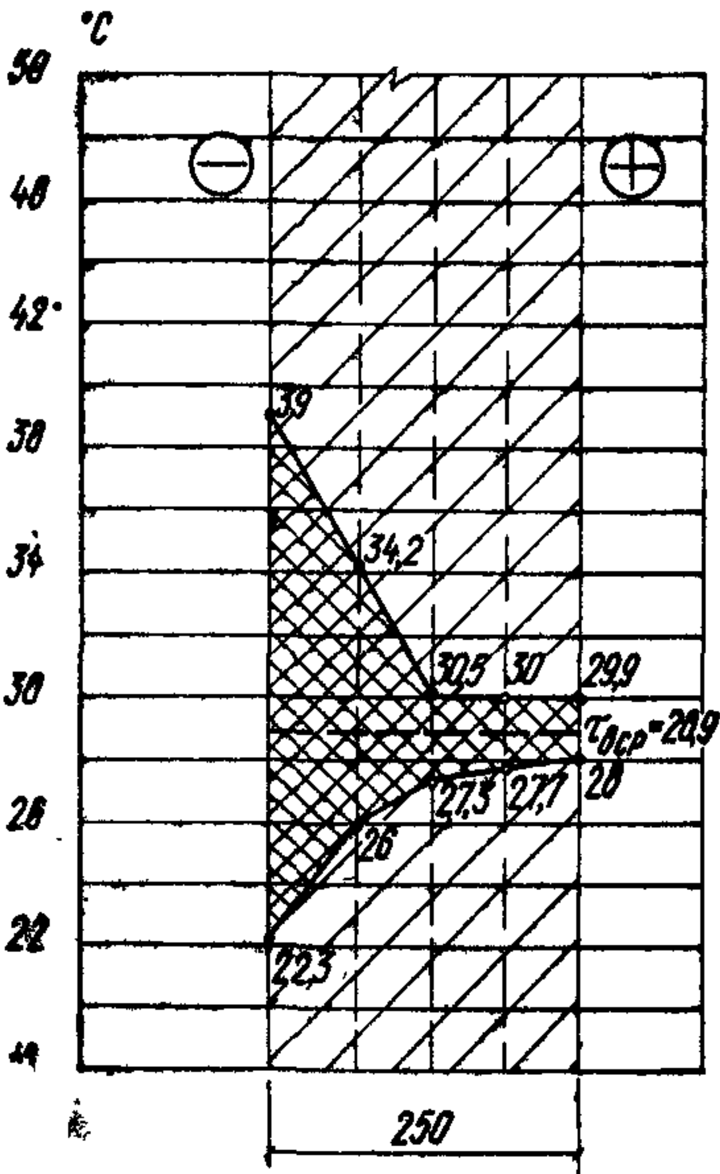
Рис. 8. Колебания температур в толще стены
