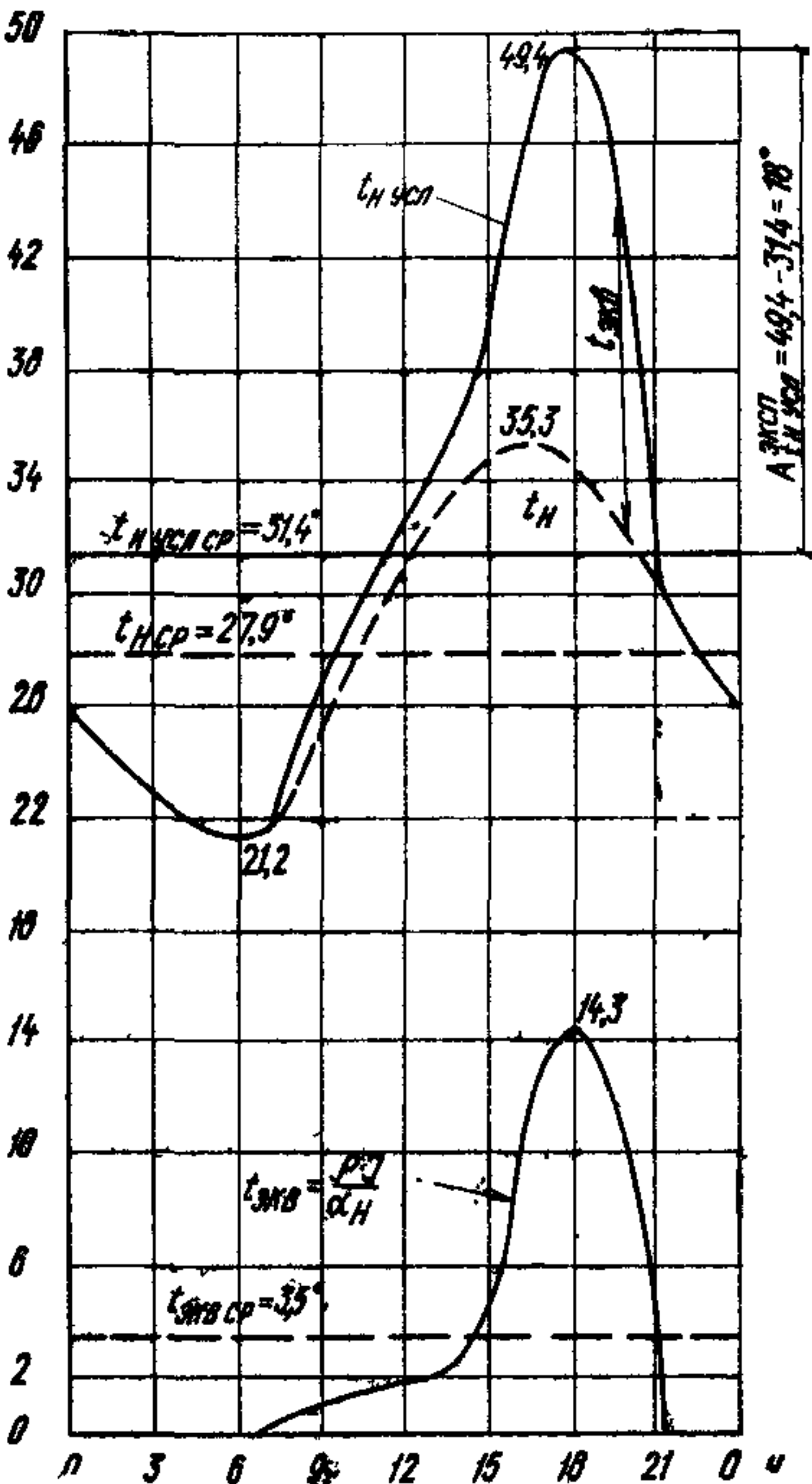
Рис. 9. Графическое определение амплитуды колебания температуры наружного воздуха с учетом солнечной радиации A_{\text{эксп}} t_{\text{н,ср}}
