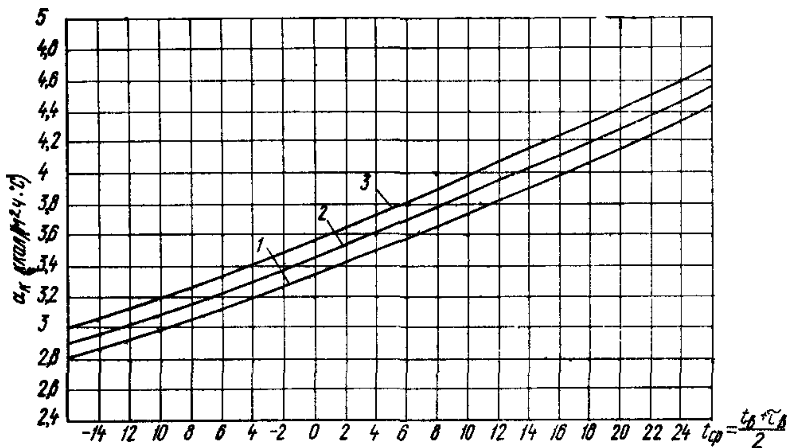
Рис. 5. График для определения \alpha_l
