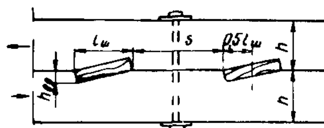
Рис. 3. Схема соединения на деревянных наклонных прямоугольных шпонках
