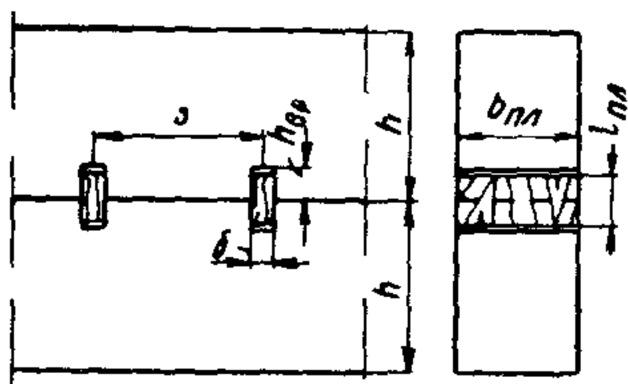
Рис 5. Схема соединения на пластинчатых нагелях
