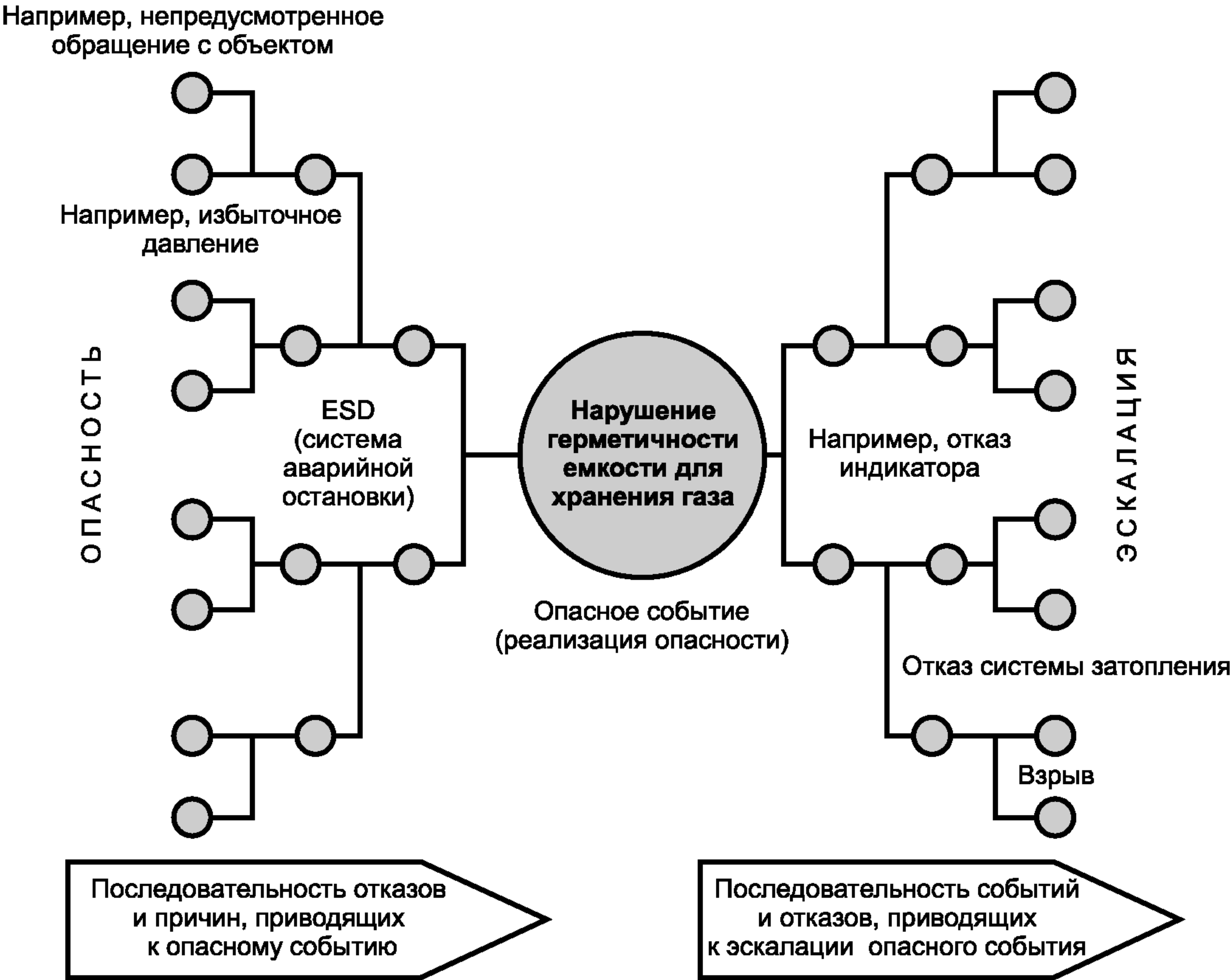
Рисунок А.1 — Схематическое представление опасного события и связанных с ним событий с помощью дерева неисправностей и дерева событий
