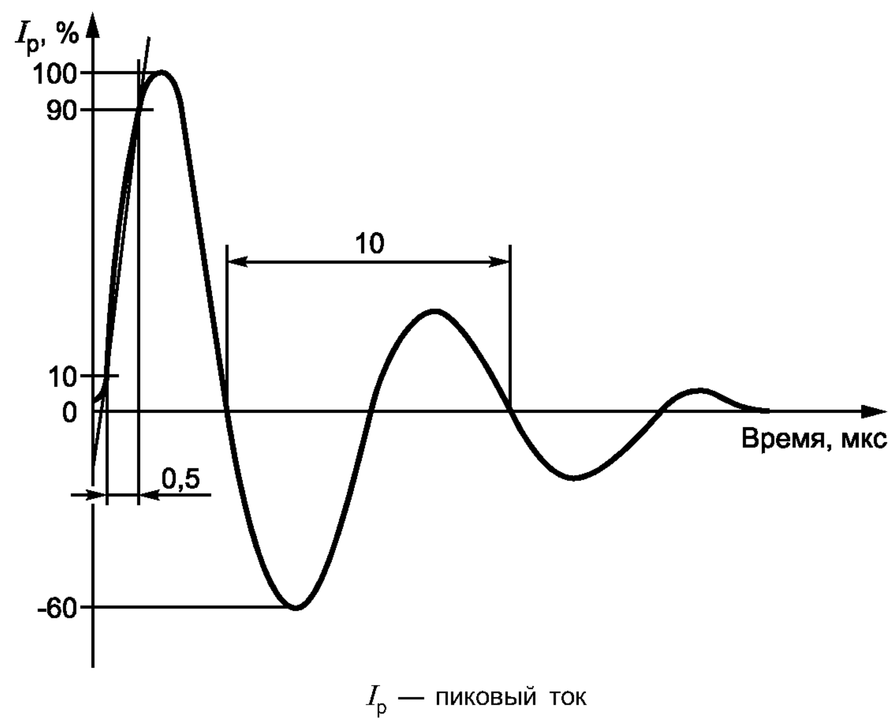
Рисунок 23 — Ток звенящей волны 0,5 мкс/100 кГц
