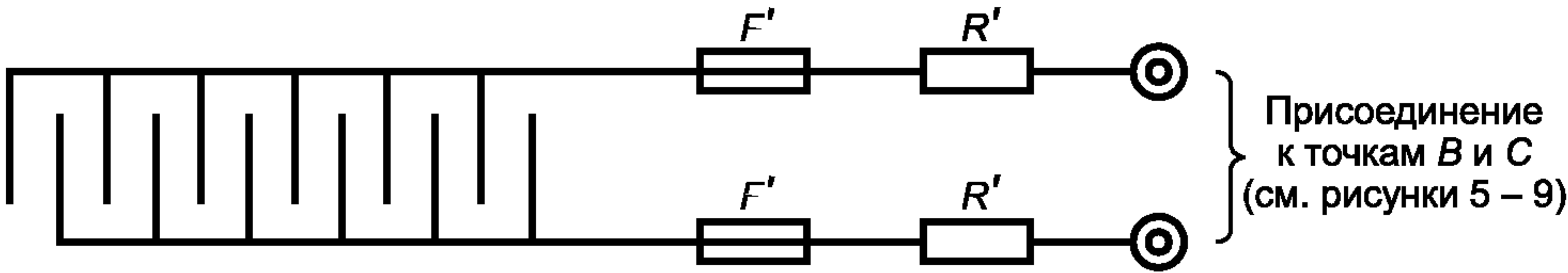
F' — плавкий предохранитель; R' — сопротивление
