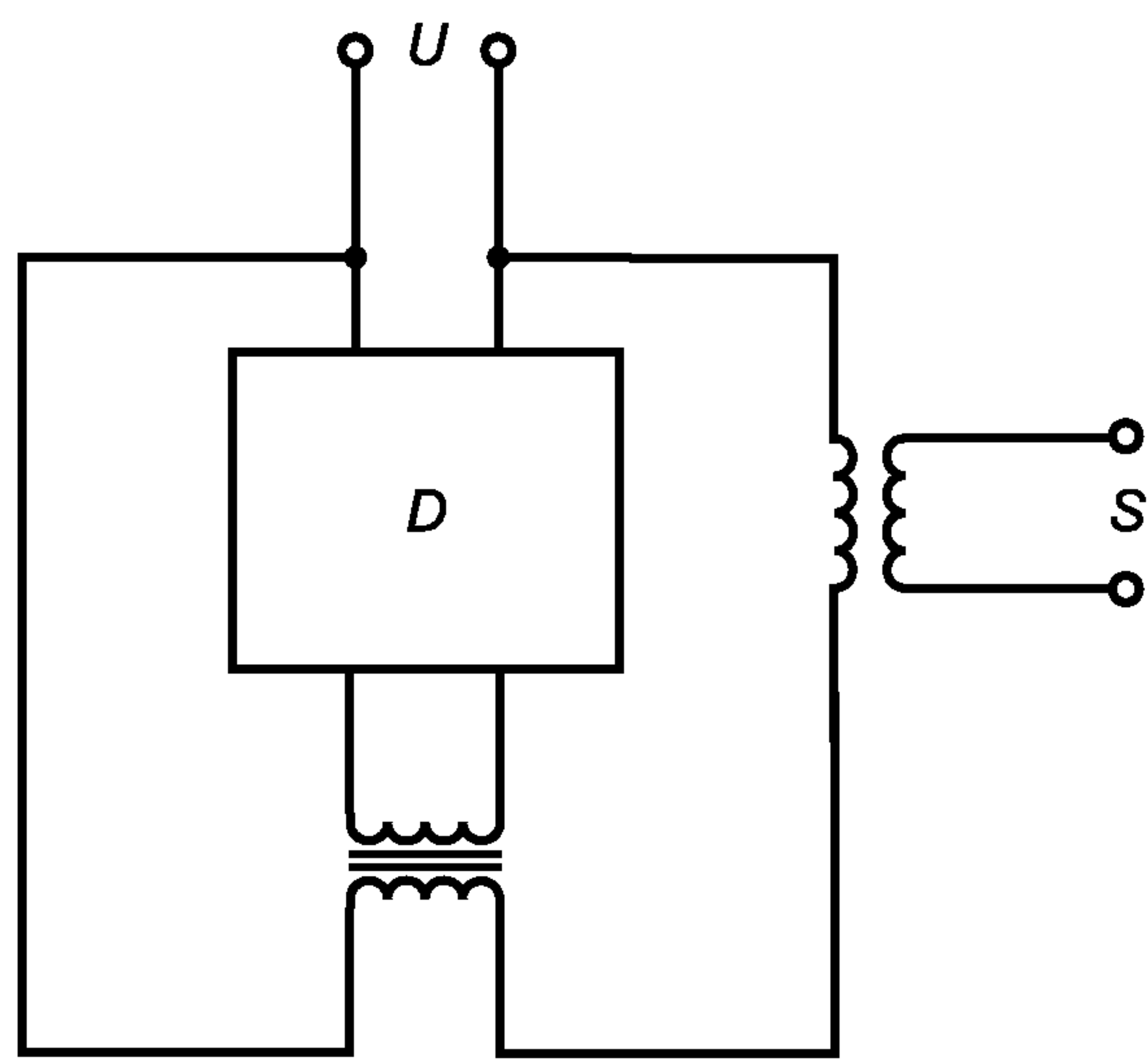
U — источник напряжения 1,1U_n ; D — испытуемый АВДТ
