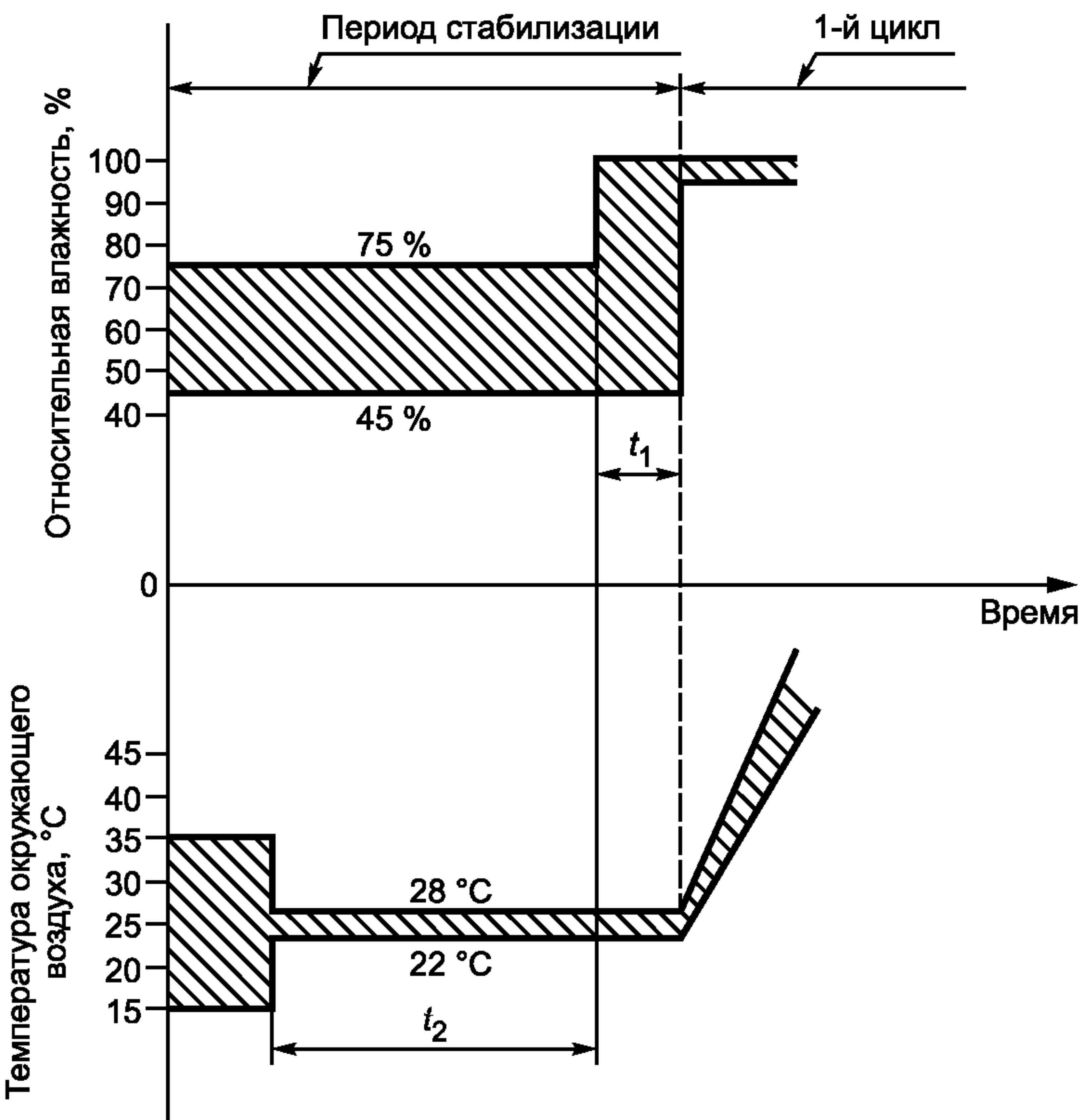
t_1 — время, требуемое для достижения 95 %—100 % относительной влажности (не превышающее 1 ч); t_2 — время, требуемое испытуемому образцу, чтобы достичь температурной стабилизации
