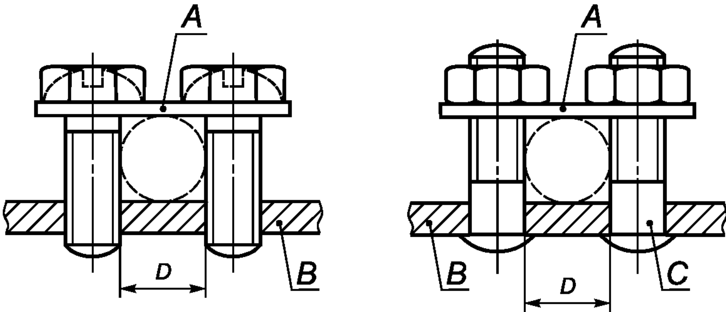
Рисунок IC.2 — Пример винтовых и штыревых выводов
