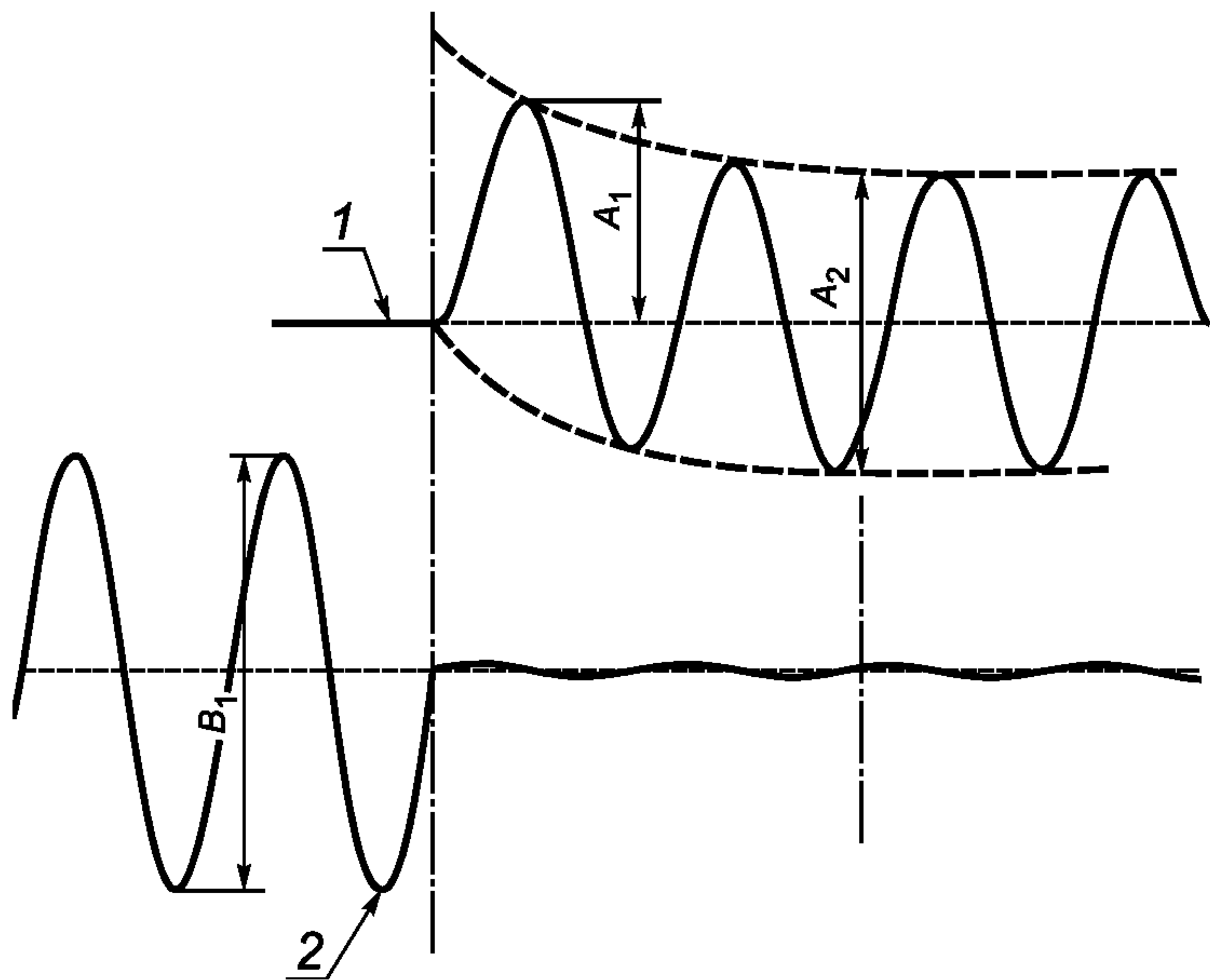
1 — напряжение; 2 — ток
