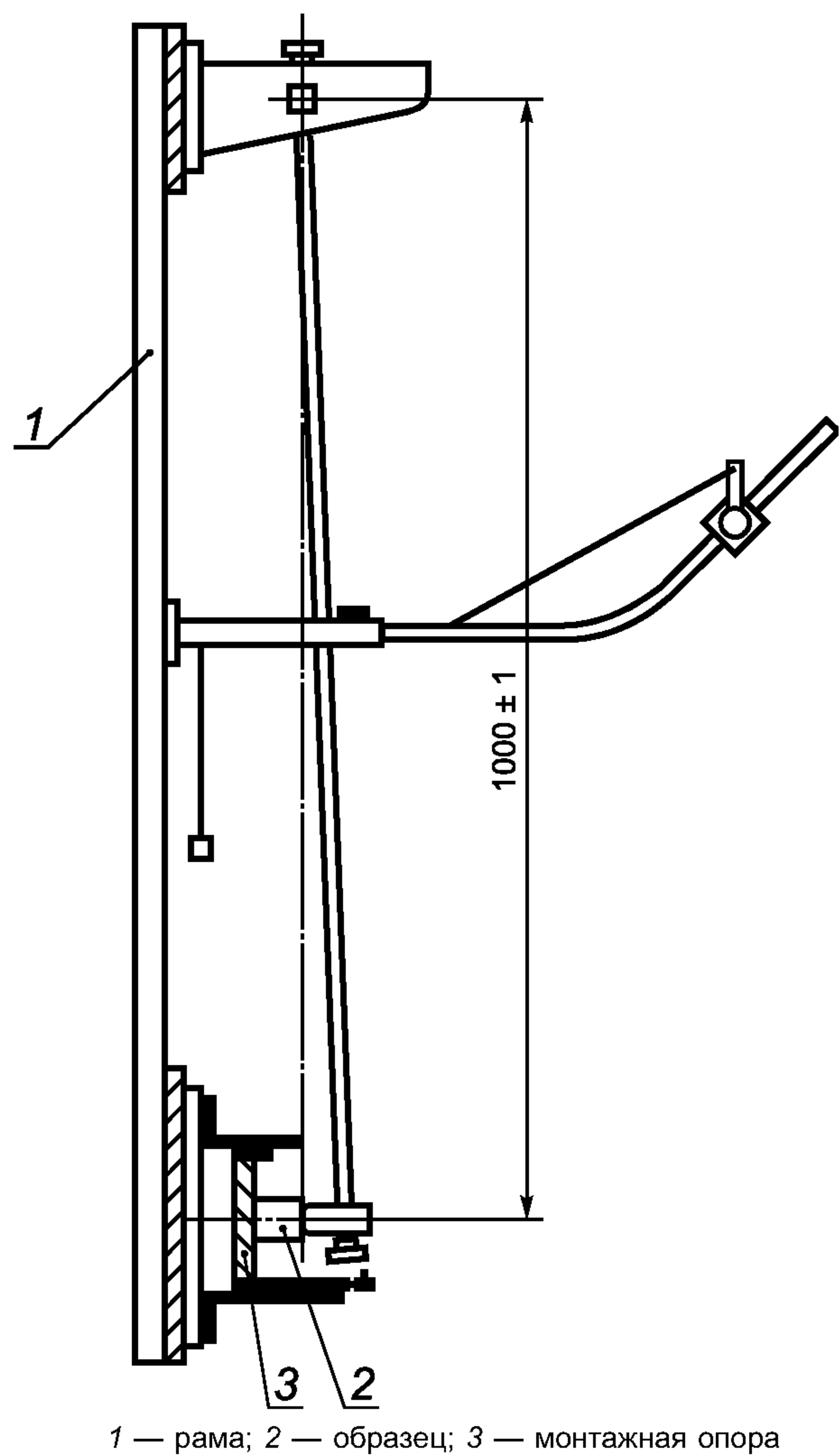
Рисунок 12 — Устройство для испытаний на механический удар (9.13.2.1)
