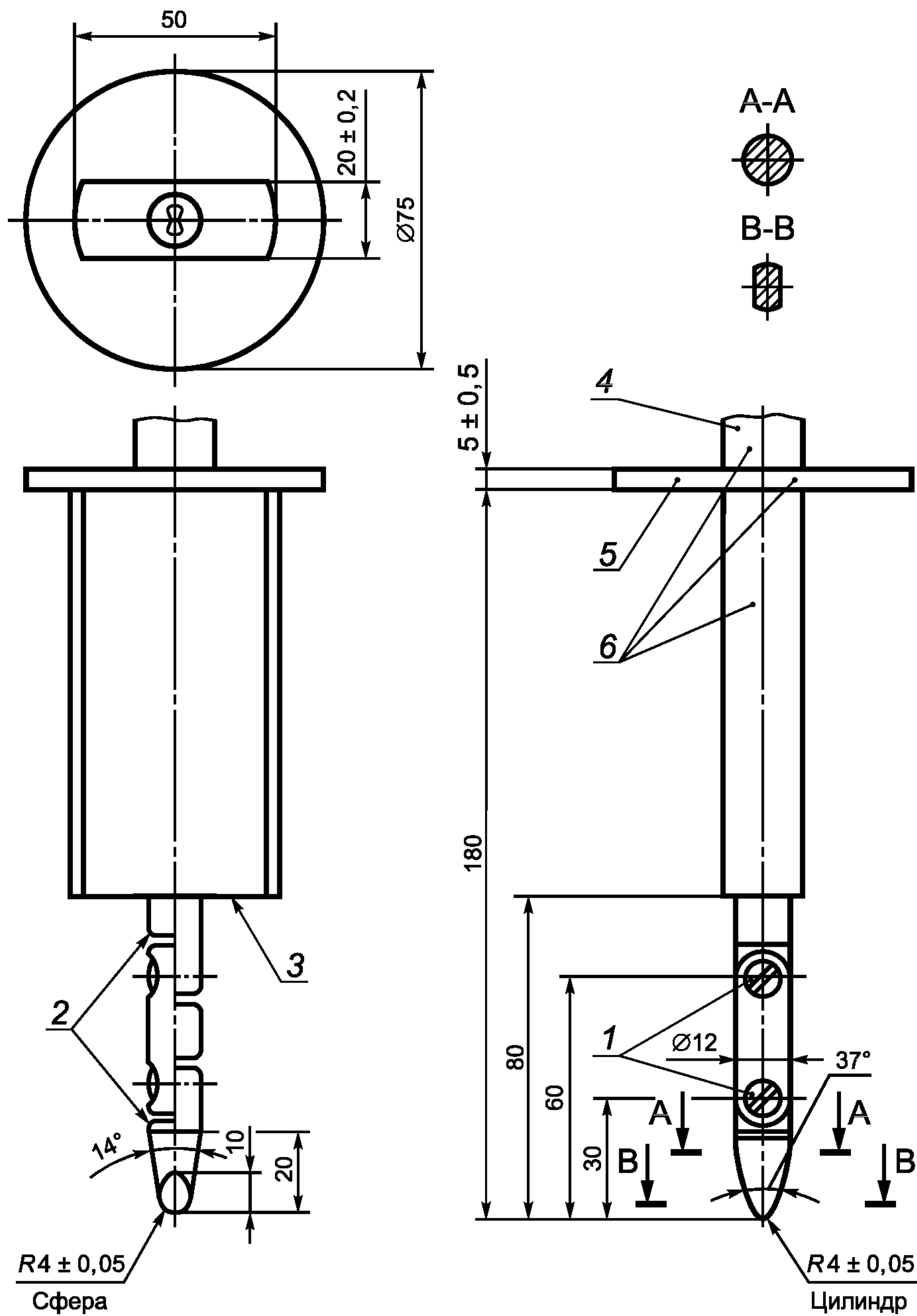
1 — шарниры; 2 — фаски; 3 — упорная поверхность; 4 — ручки; 5 — защитная шайба; 6 — изоляционный материал Материал: металл, если не указано иное Линейные размеры в мм Неуказанные допуски на размеры: - угловые: 0—10 - линейные: до 25 мм 0—0,05 мм св. 25 мм ± 0,2 мм Оба шарнира должны позволять движение в одной плоскости и в одном направлении на угол 90° с допуском 0° + 10°
