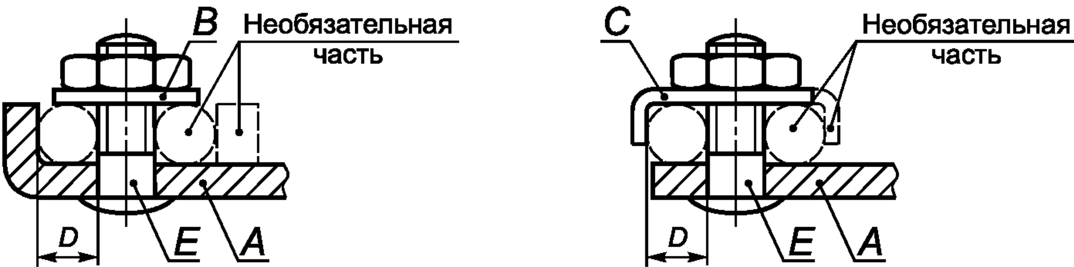
Штыревые выводы
