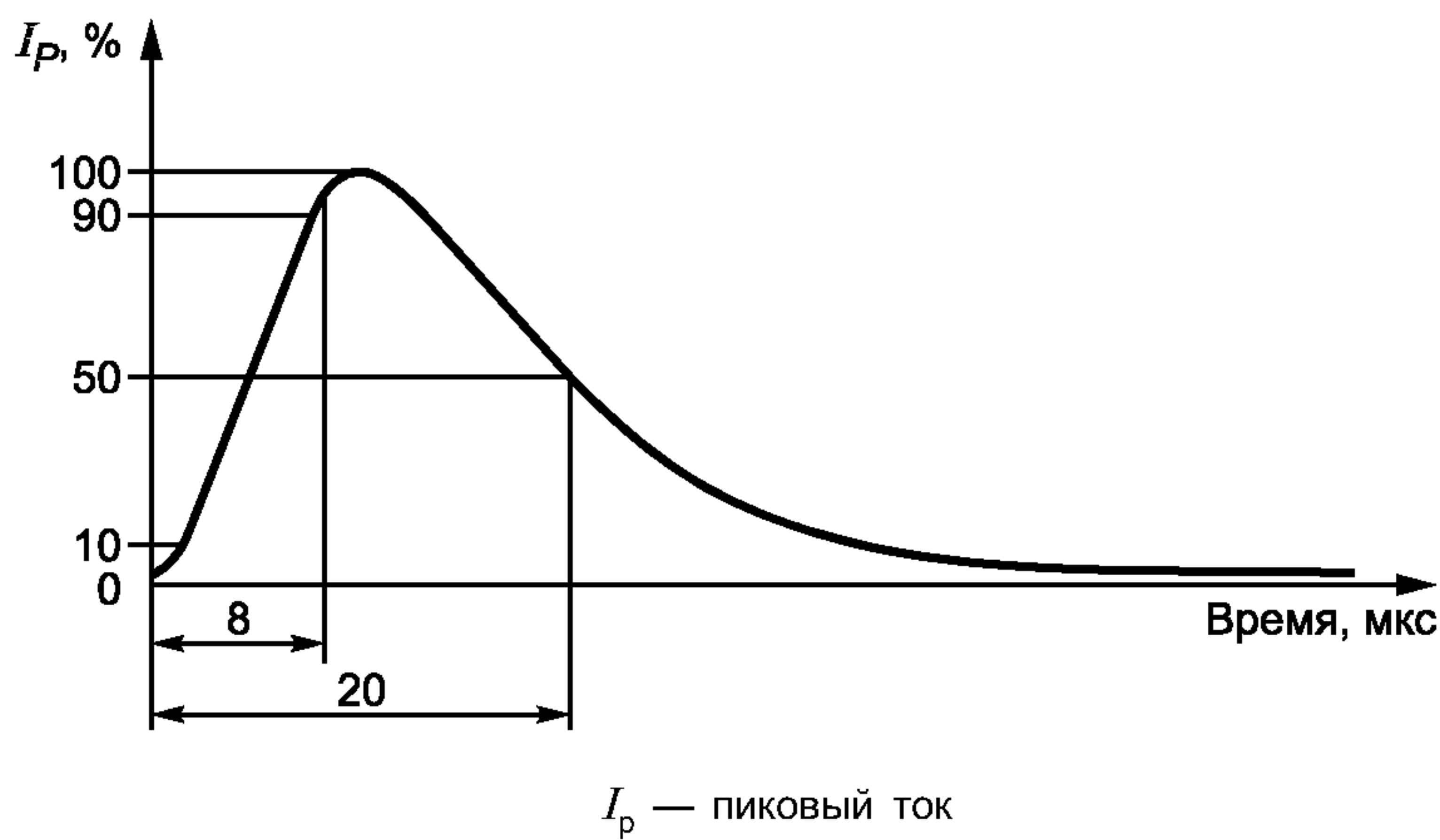
Рисунок 25 — Звонящая волна 8/20 мкс
