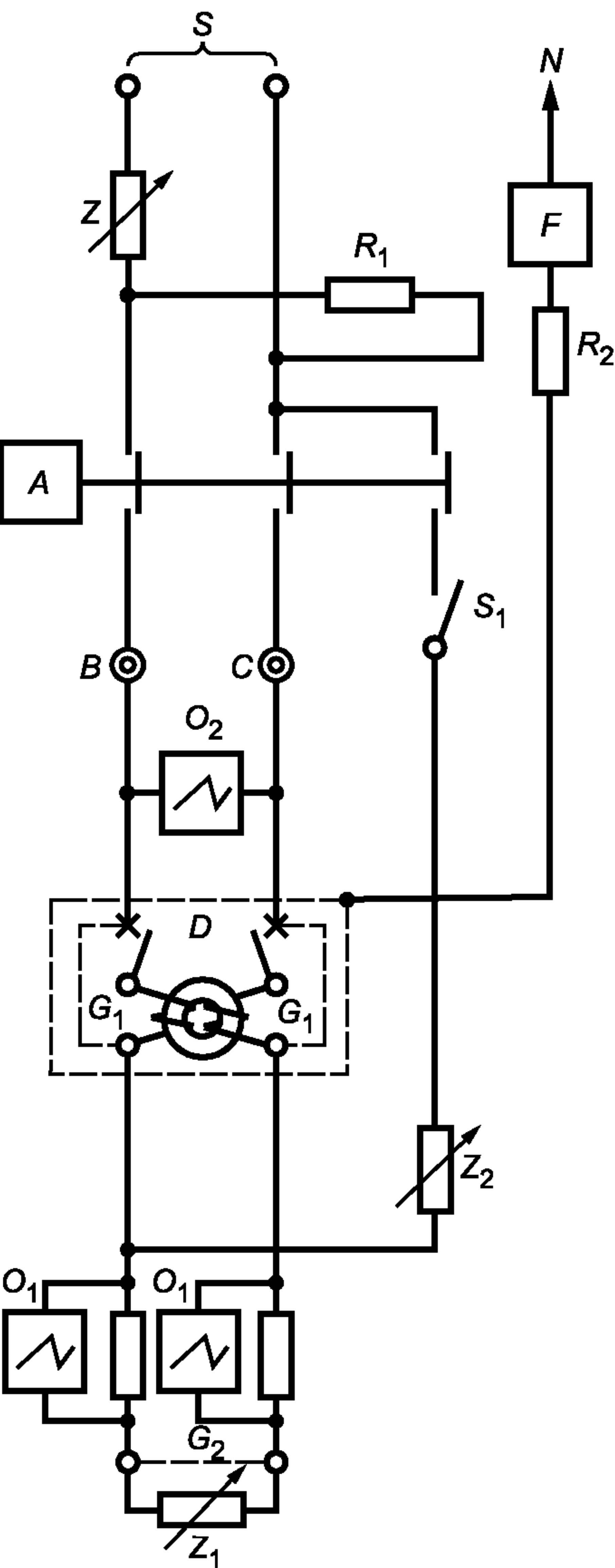
Рисунок 6 — Испытательная цепь для проверки номинальной наибольшей отключающей способности двухполюсного АВДТ в однофазной сети (9.12)
