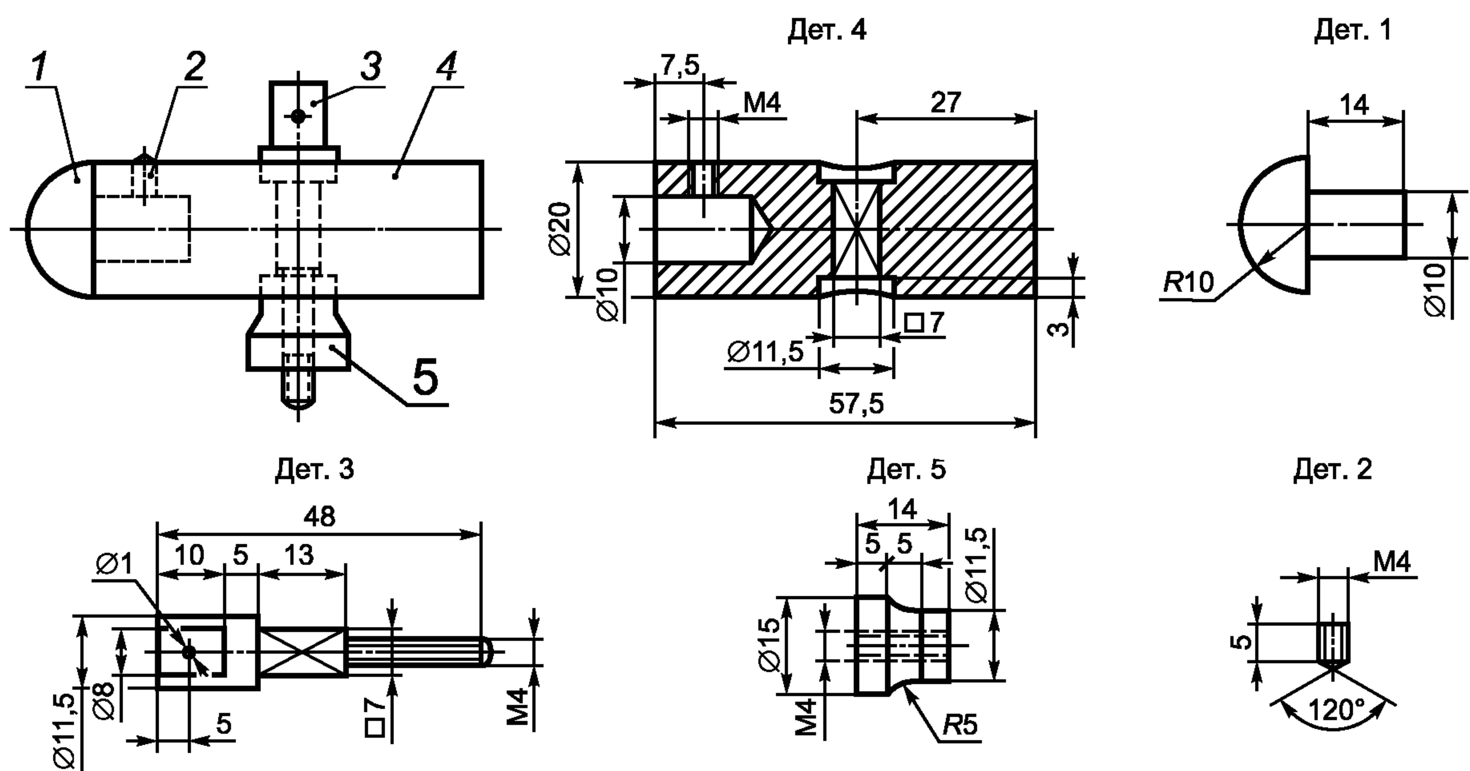
Материал деталей: 1 — полиамид; 2 — 5 — сталь 35
