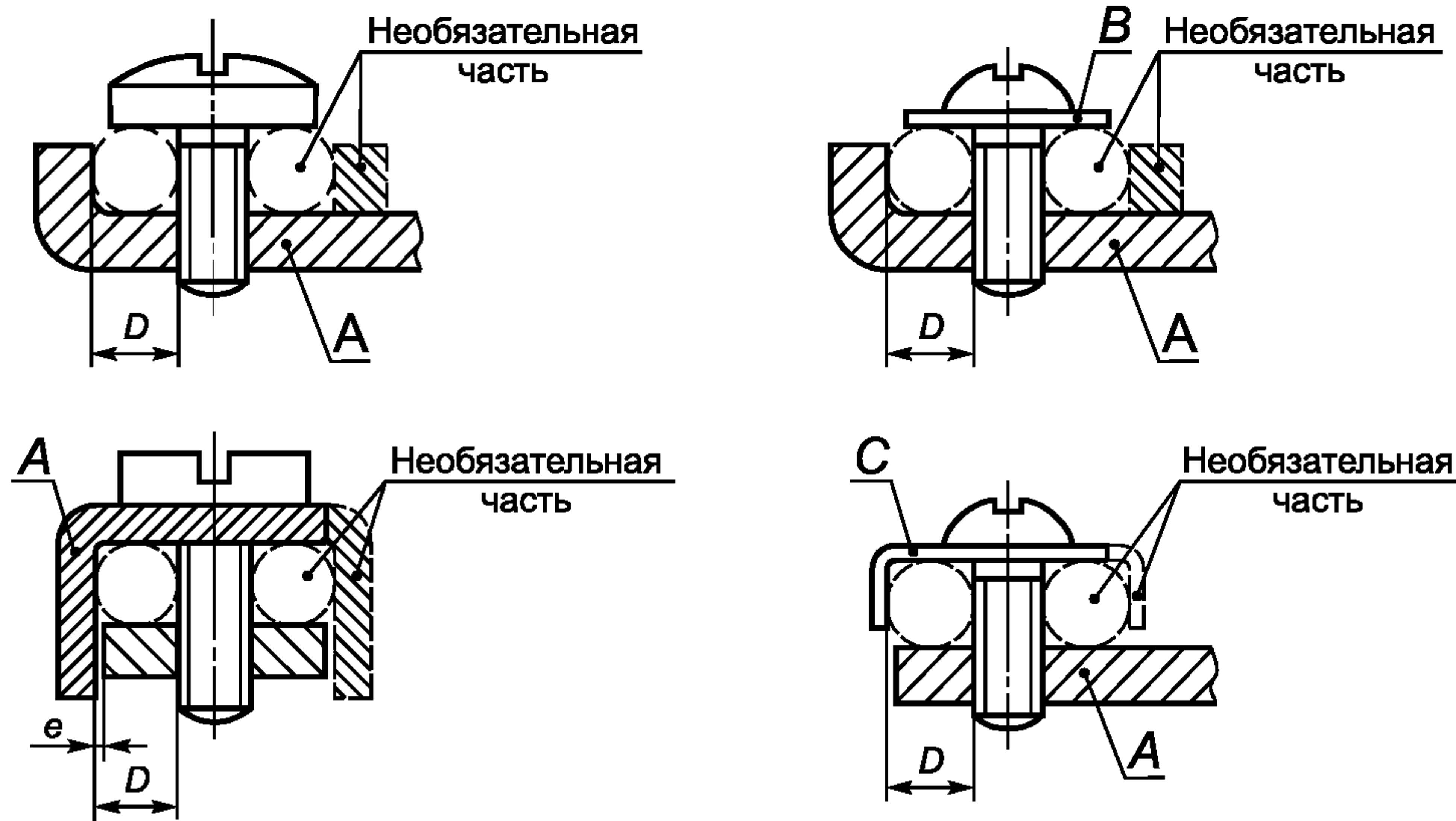
Винтовые выводы
