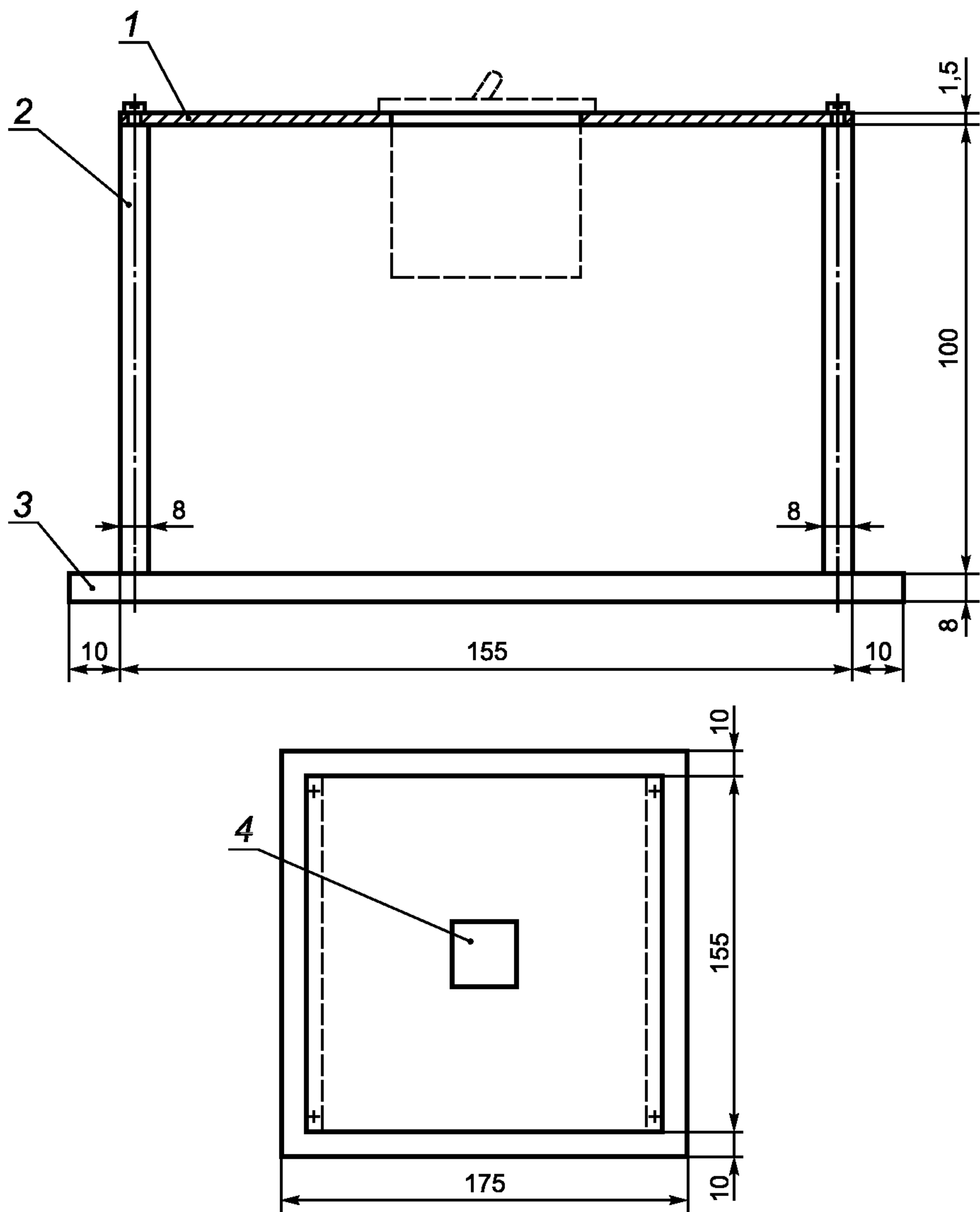
1 — съемная стальная пластина толщиной 1,5 мм; 2 — алюминиевая пластина толщиной 8 мм; 3 — монтажная плита; 4 — окно для АВДТ в стальной пластине
