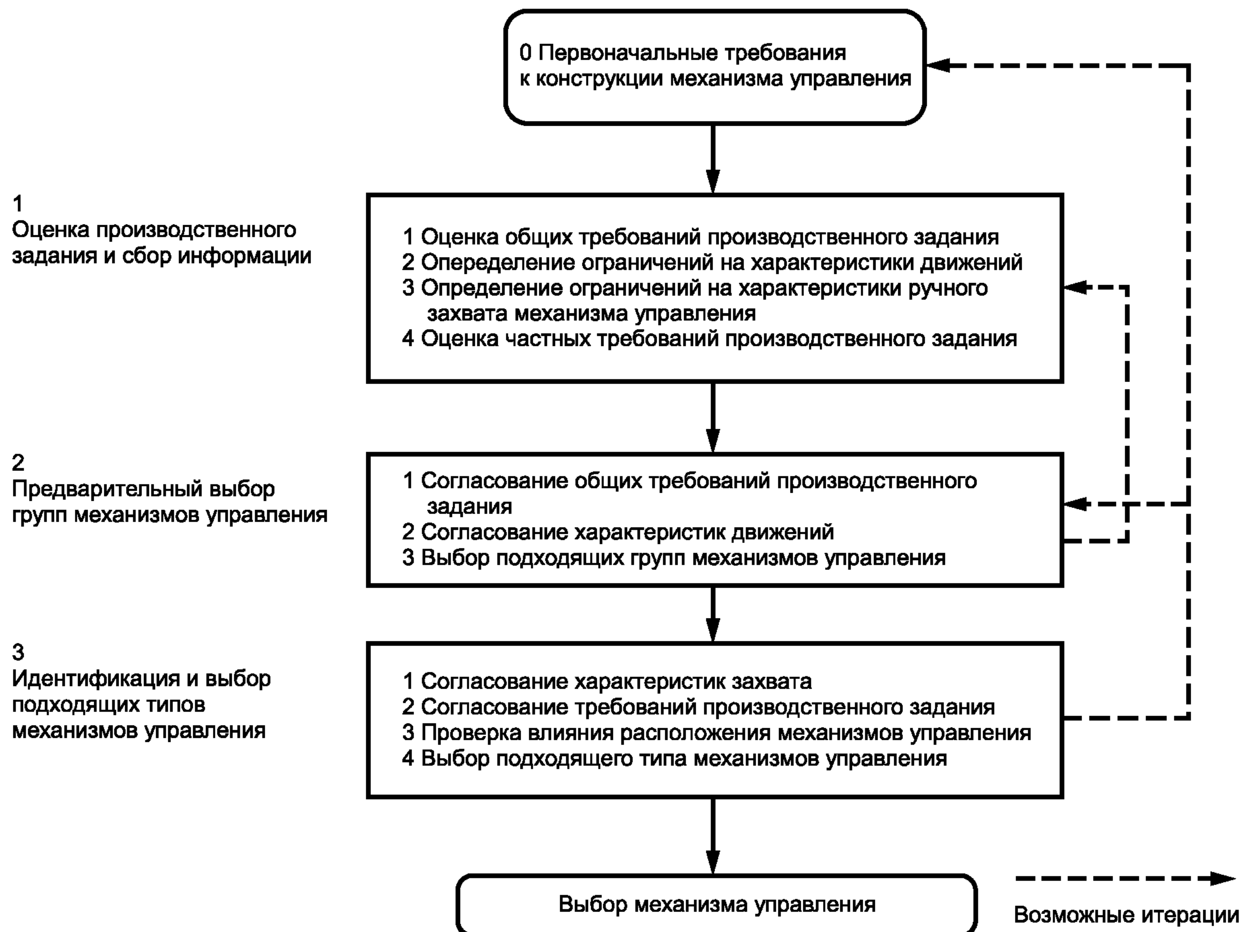
Рисунок 1 — Схема общей процедуры выбора ручного механизма управления
