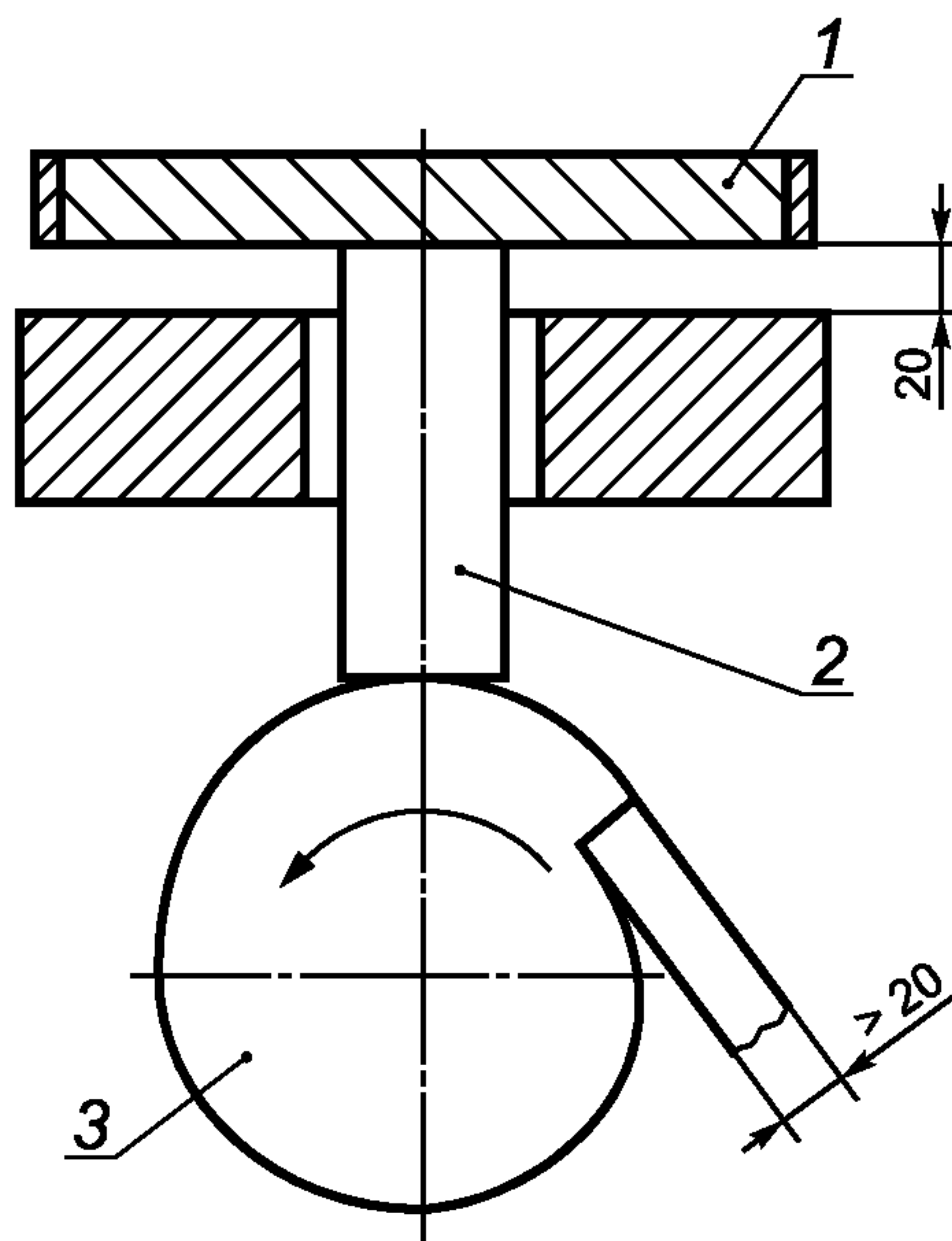
1 — подставка для крепления; 2 — опорный шток; 3 — эксцентрик
