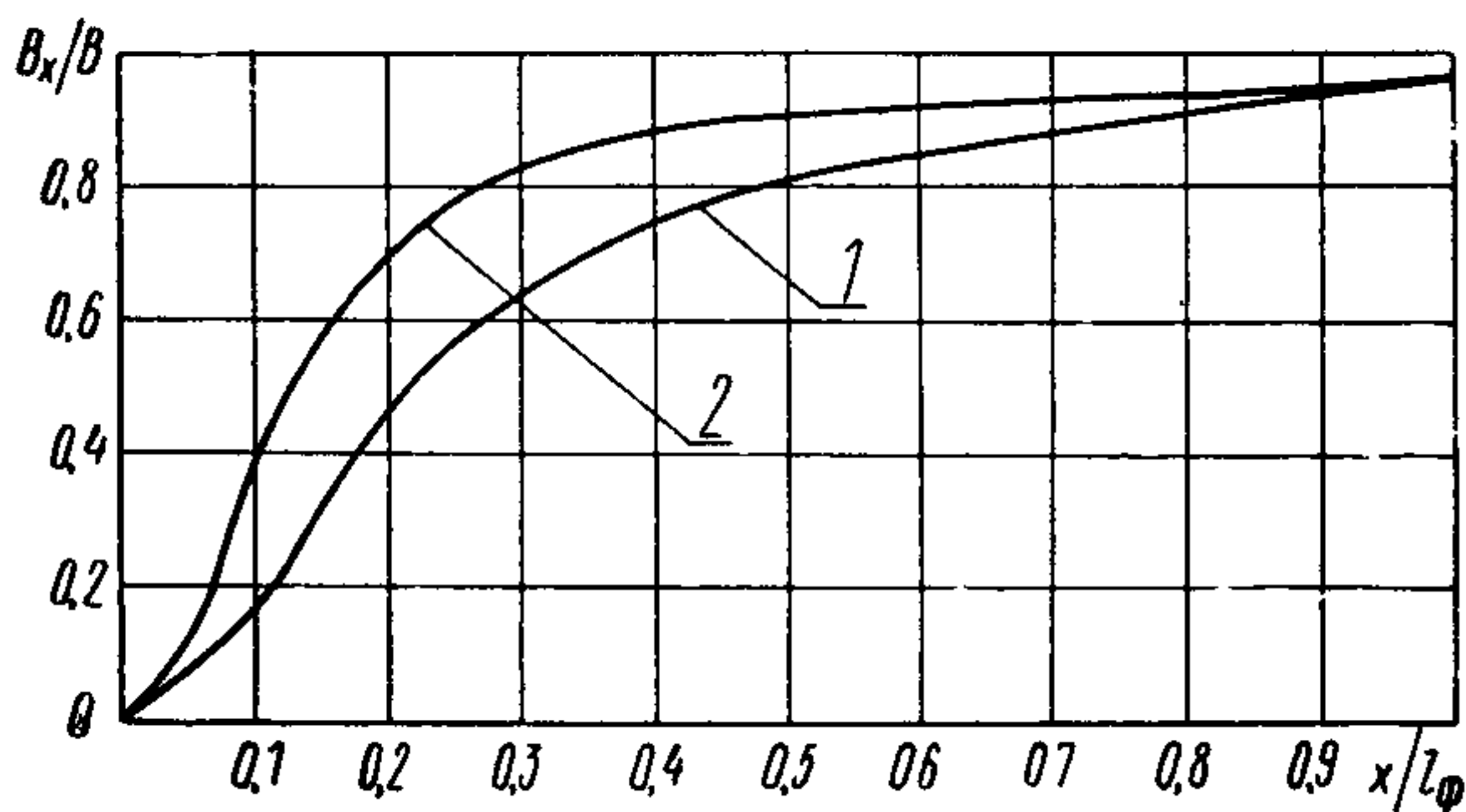
Выгорание топлива по длине факела
