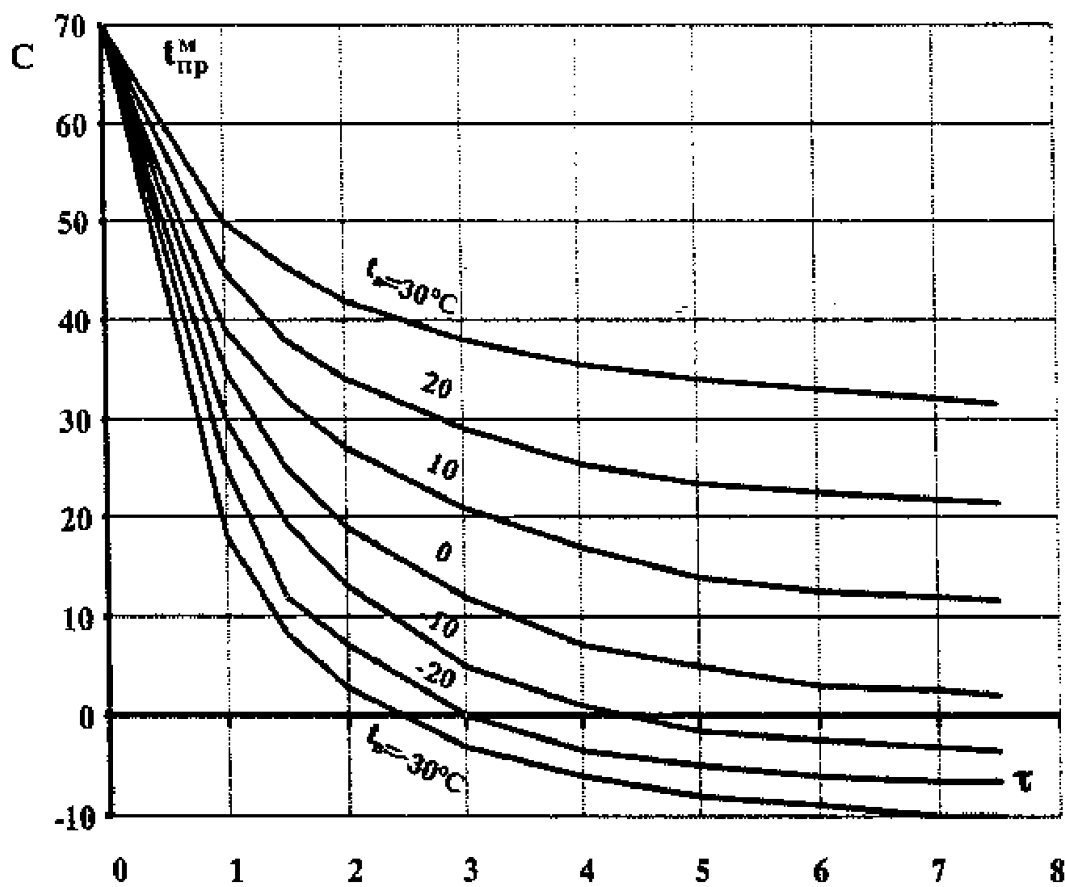
Рисунок Б.3 – Температура мазута в цистернах при транспортировке в зависимости от температуры окружающего воздуха и времени нахождения в пути
