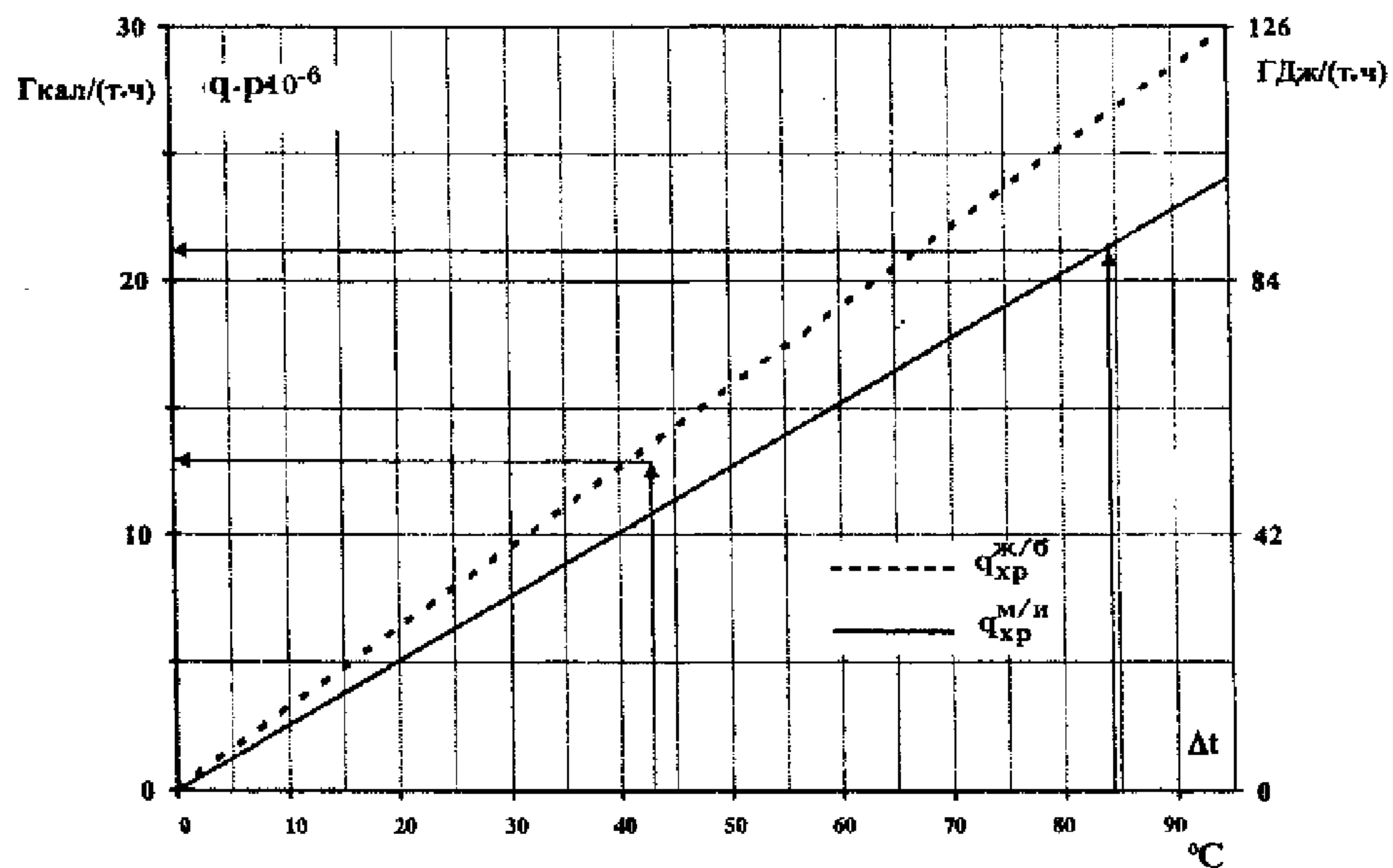
Рисунок Б.6 – Нормы удельного расхода тепла при хранении мазута в железобетонных ( q_{хр}^{ж/б} ), металлических с изоляцией ( q_{хр}^{м/и} ) емкостях, учитываемые при эксплуатации
