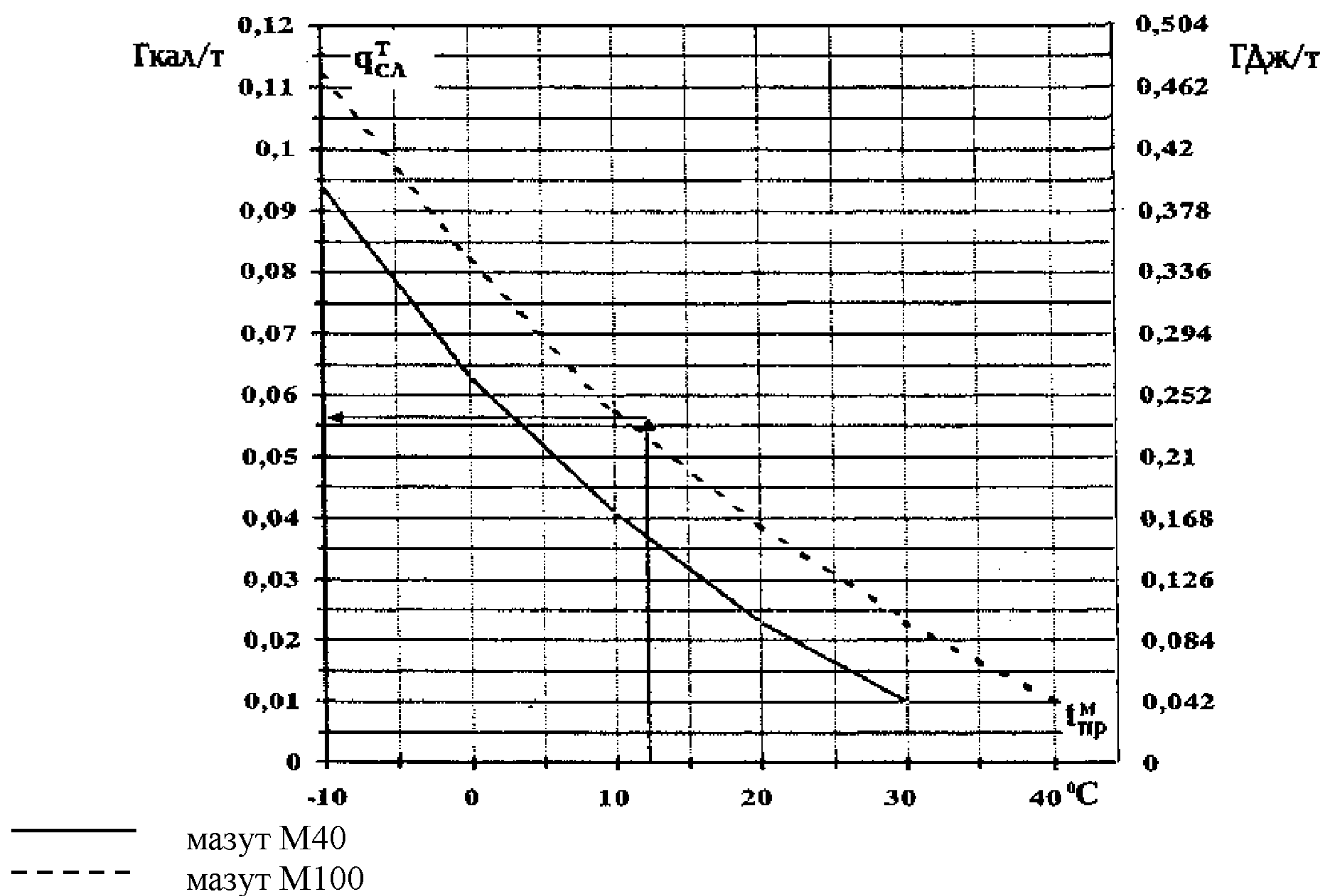
Рисунок Б.2 – Нормы удельного расхода тепла при сливе мазута ( q_{сл}^T ), учитываемые при эксплуатации ХЖКТ
