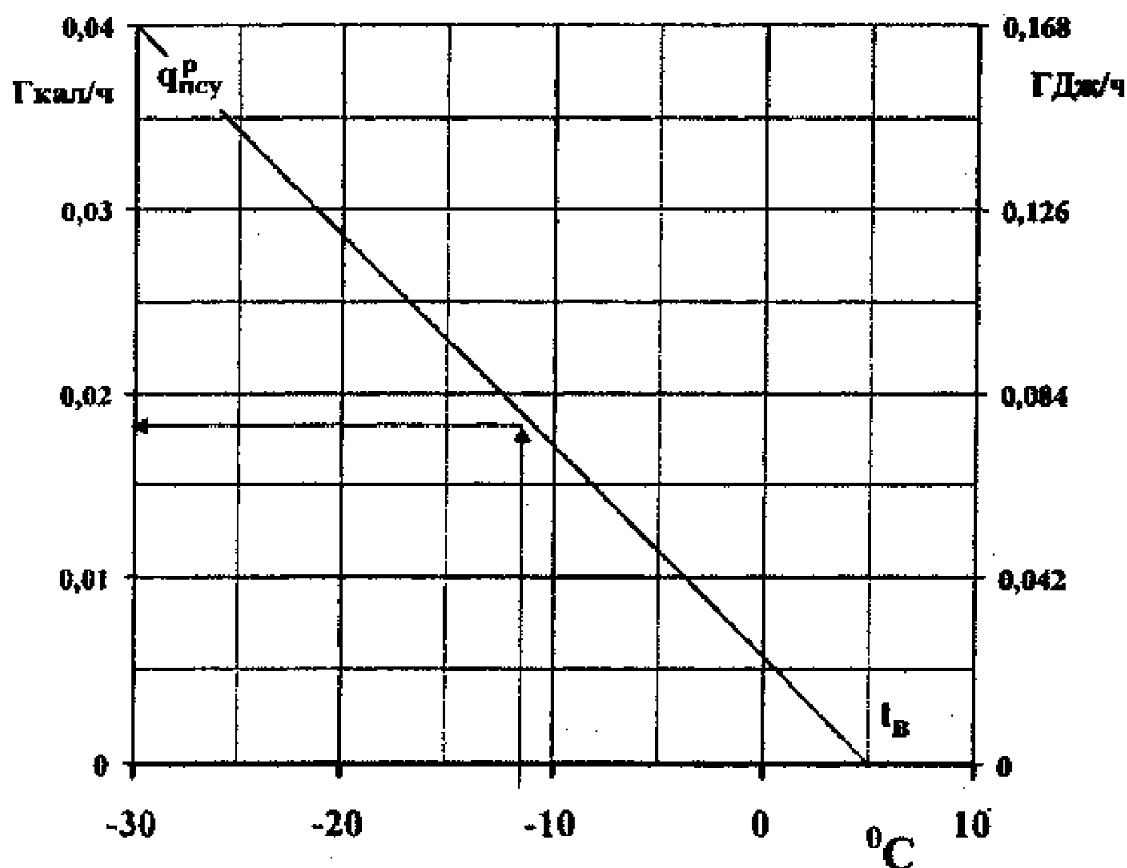
Рисунок Б.8 Нормы удельного расхода тепла на поддержание одного парового «гусака» приемно-сливного устройства в резерве ( q_{\text{псу}}^{\text{р}} ), учитываемые при эксплуатации
