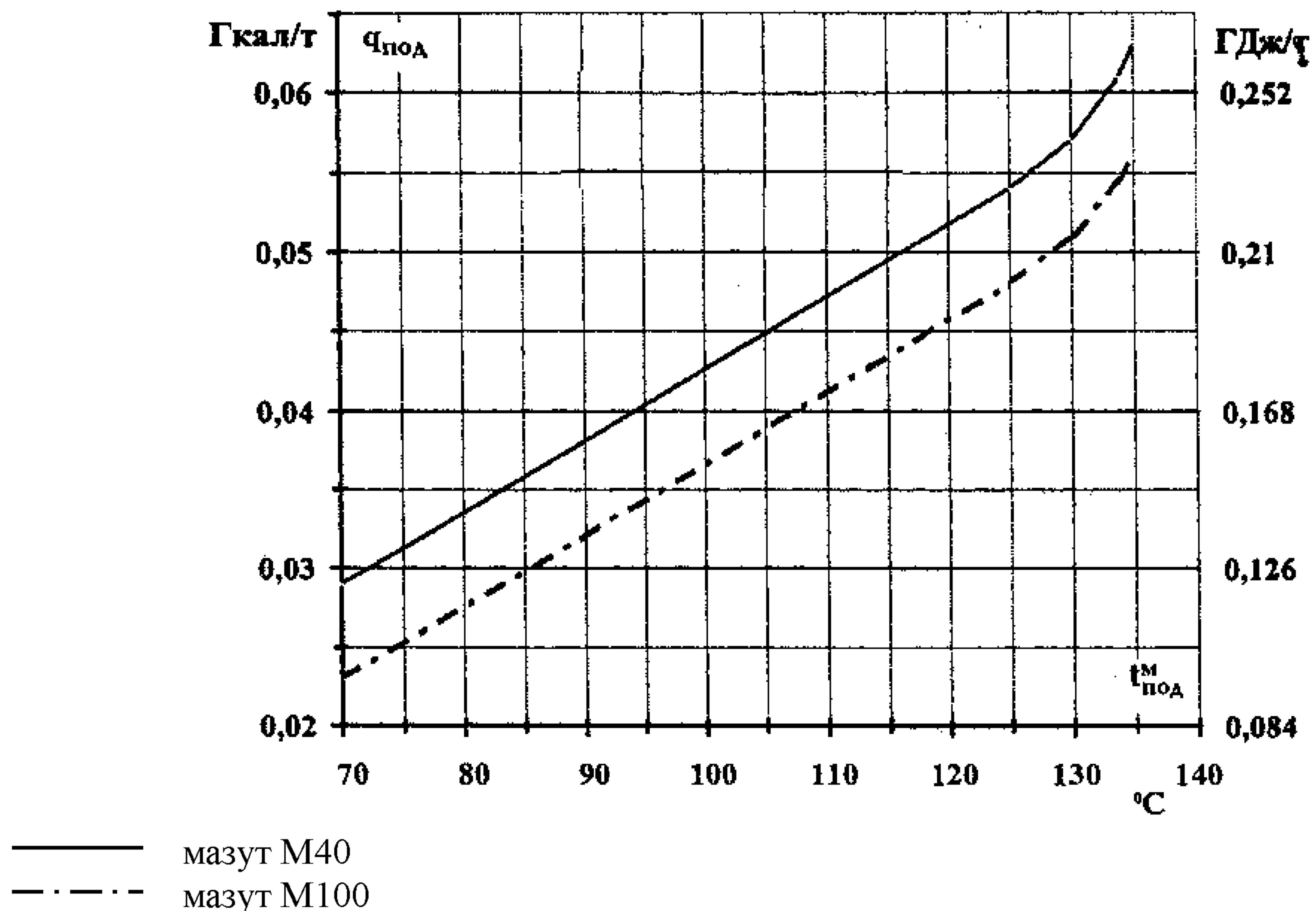
Рисунок Б.4 – Нормы удельного расхода тепла на подогрев мазута в подогревателях ( q_{\text{под}} ), учитываемые при проектировании эксплуатации ХЖКТ
