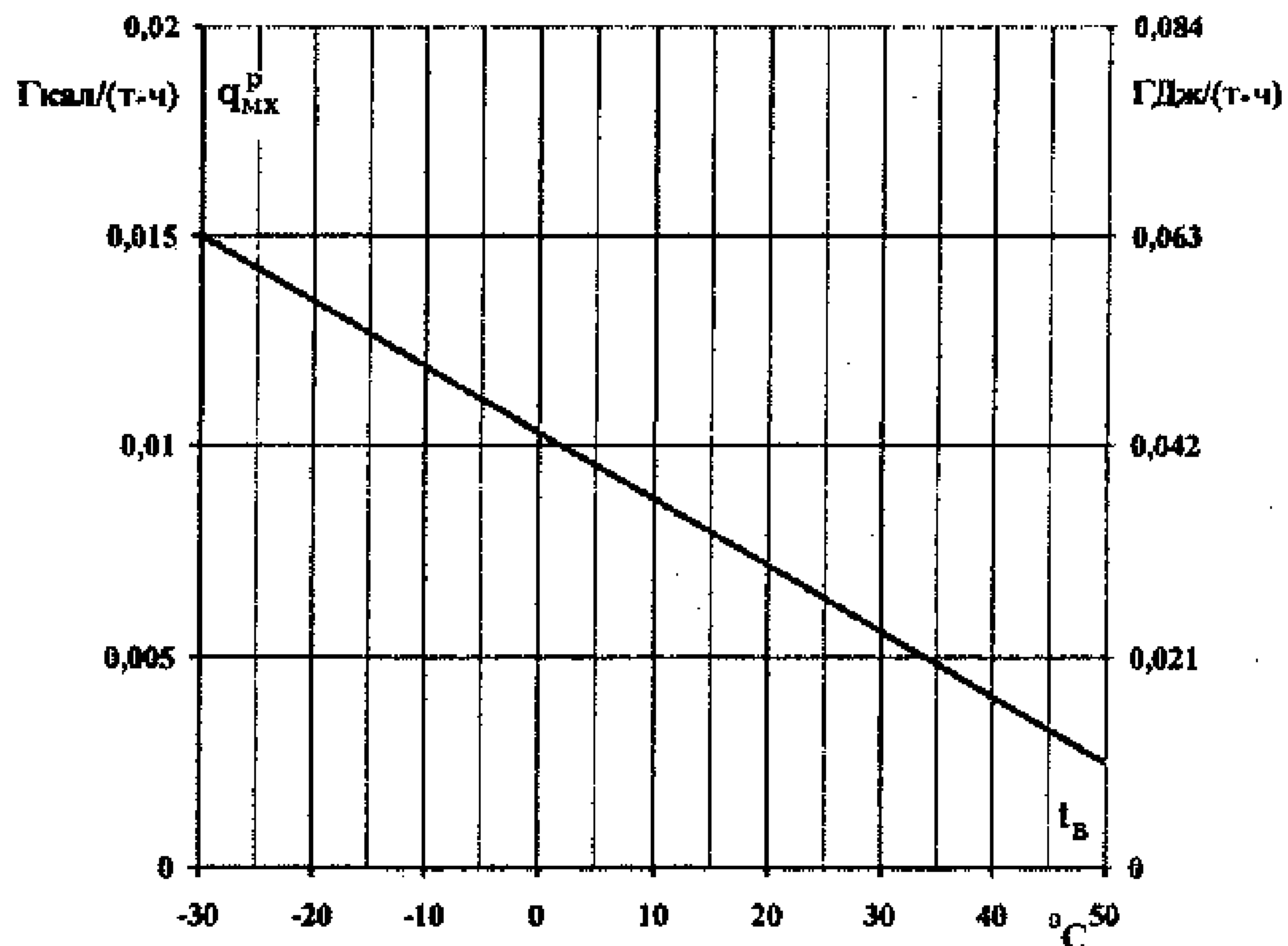
Рисунок Б.7 – Нормы удельного расхода тепла на поддержание ХЖКТ в «горячем режиме» ( q_{мх}^p ), учитываемые при эксплуатации
