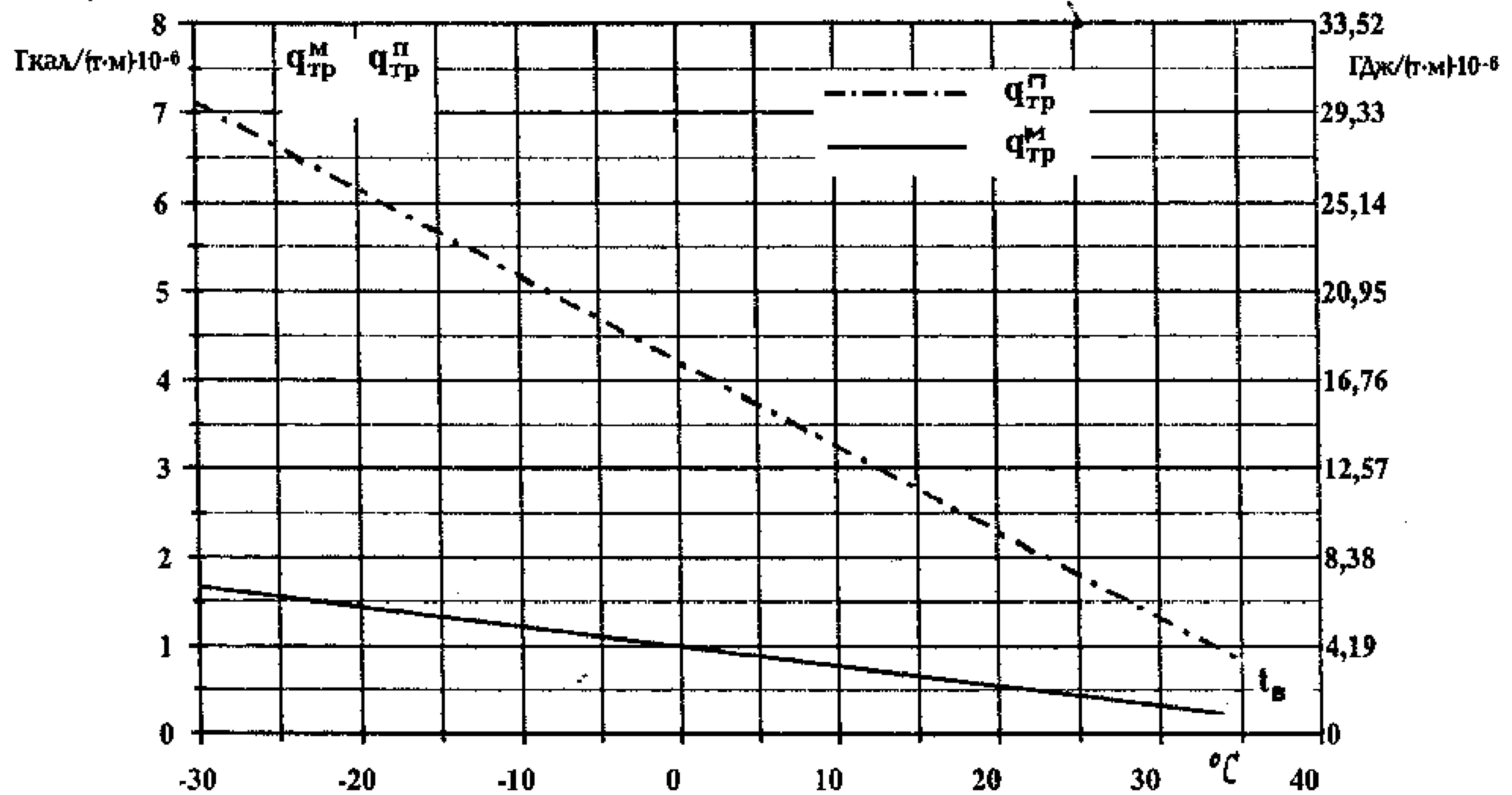
Рисунок Б.5 – Нормы удельного расхода тепла при транспортировке мазута ( q_{тр}^m ) и пара ( q_{тр}^p ) по трубопроводам, учитываемые при проектировании и эксплуатации ХЖКТ
