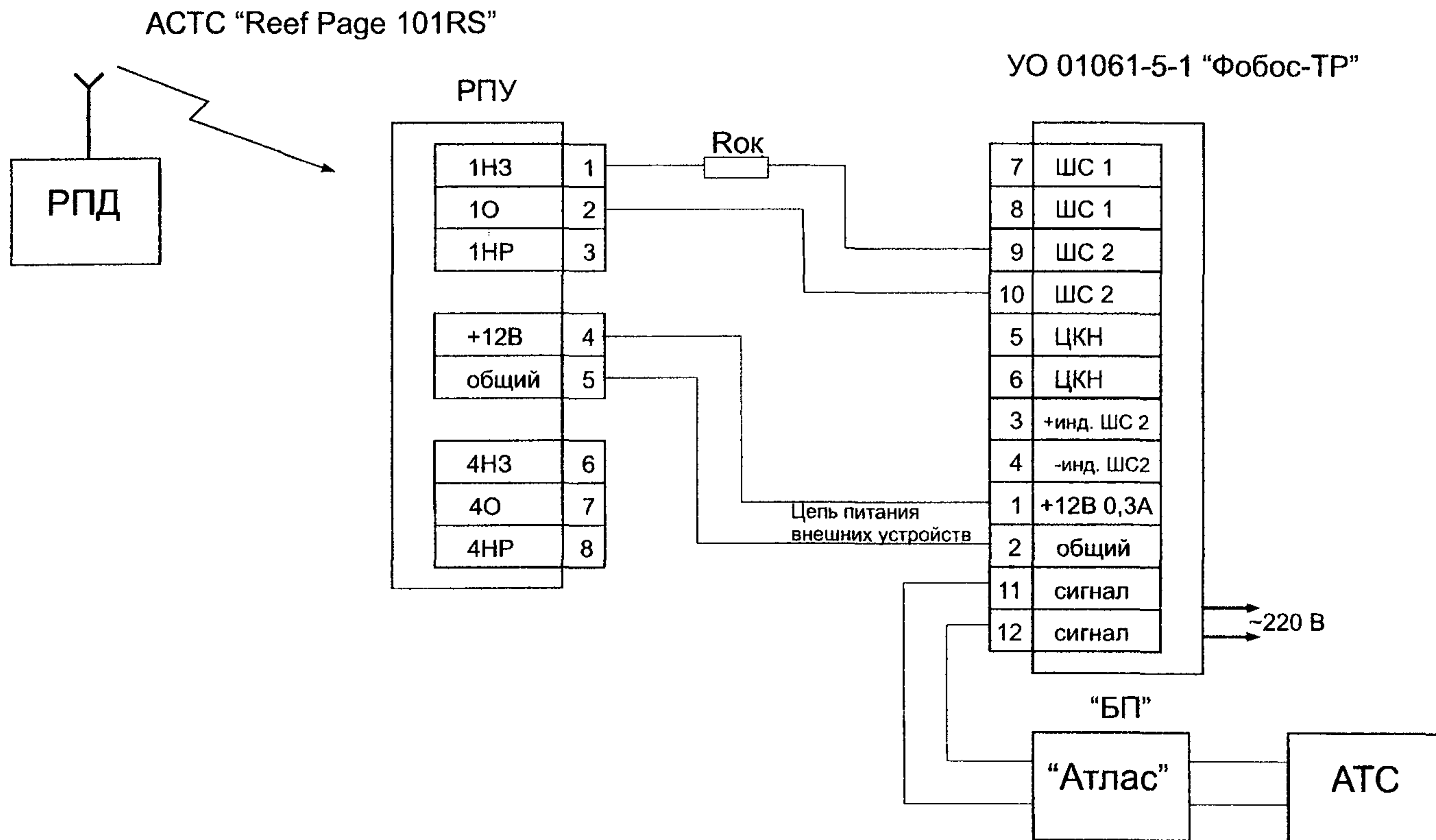
Рис. 4 - Схема подключения ACTC "Reef Page 101RS" к УО 01061-2-1 "Фобос-ТР"
