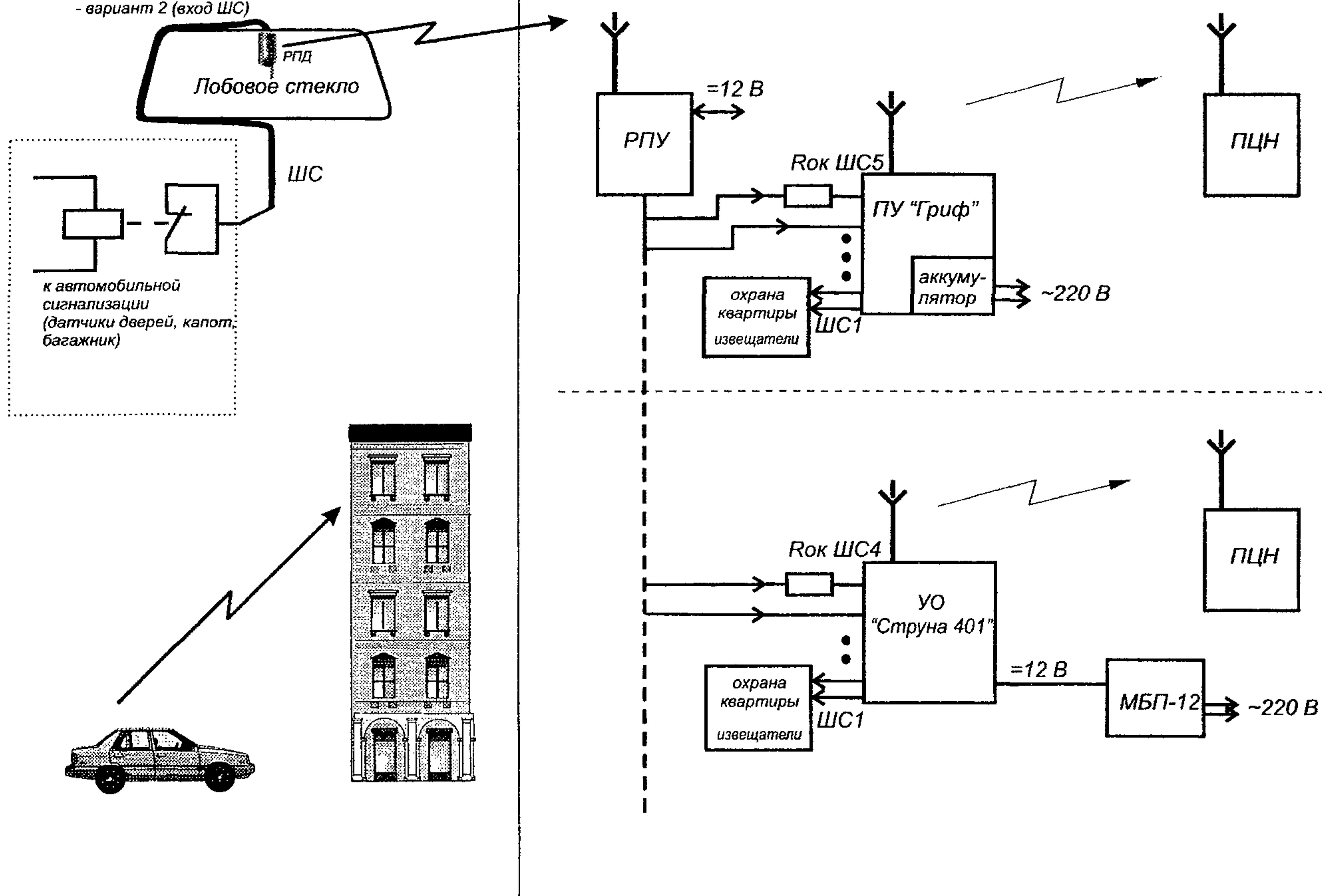
Рис. 9 - Схема подключения РТС "Радиокнопка" к РСПИ "Струна-3М"
