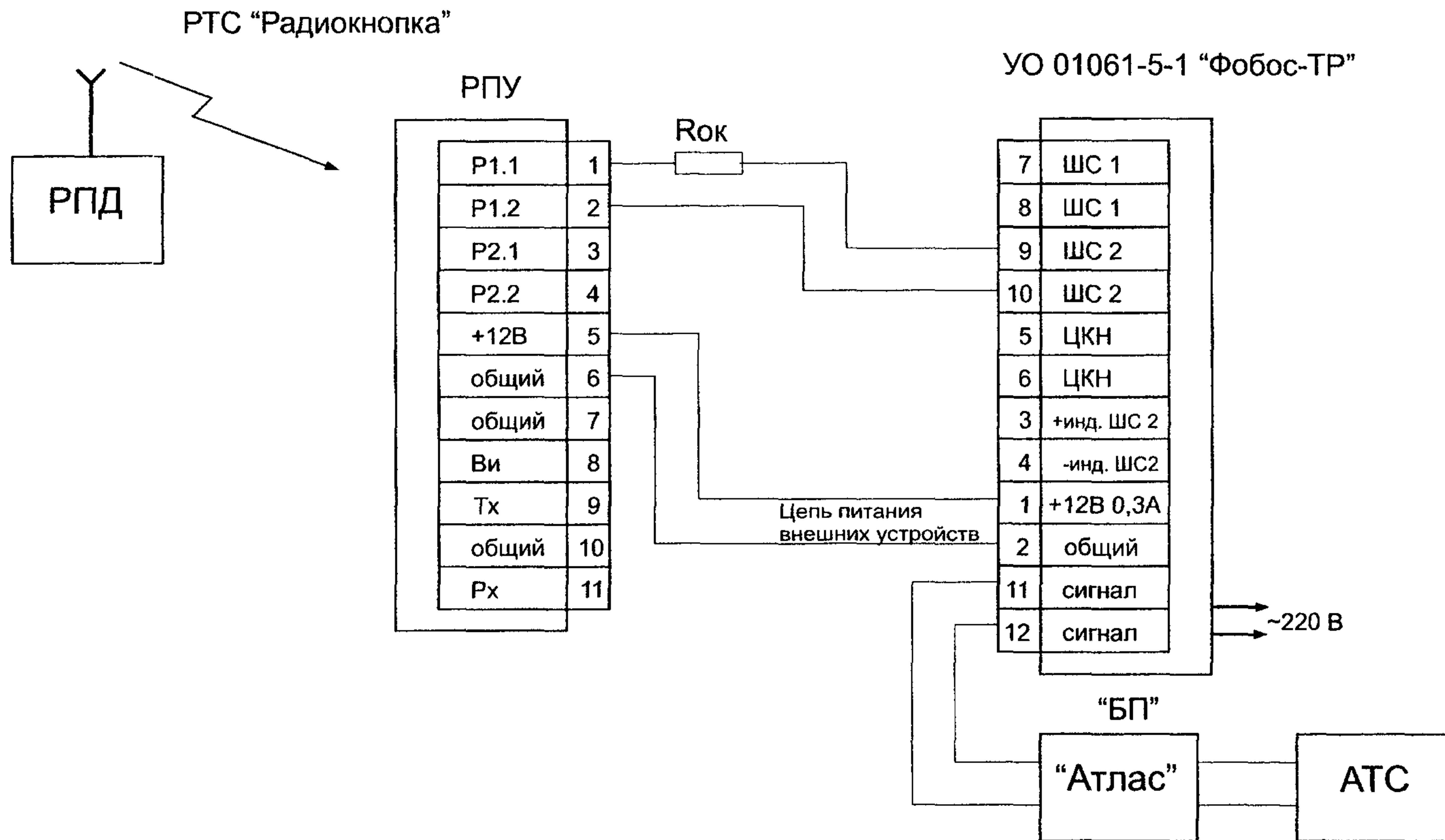
Рис. 4 - Схема подключения РТС "Радиокнопка" к УО 01061-2-1 "Фобос-ТР"
