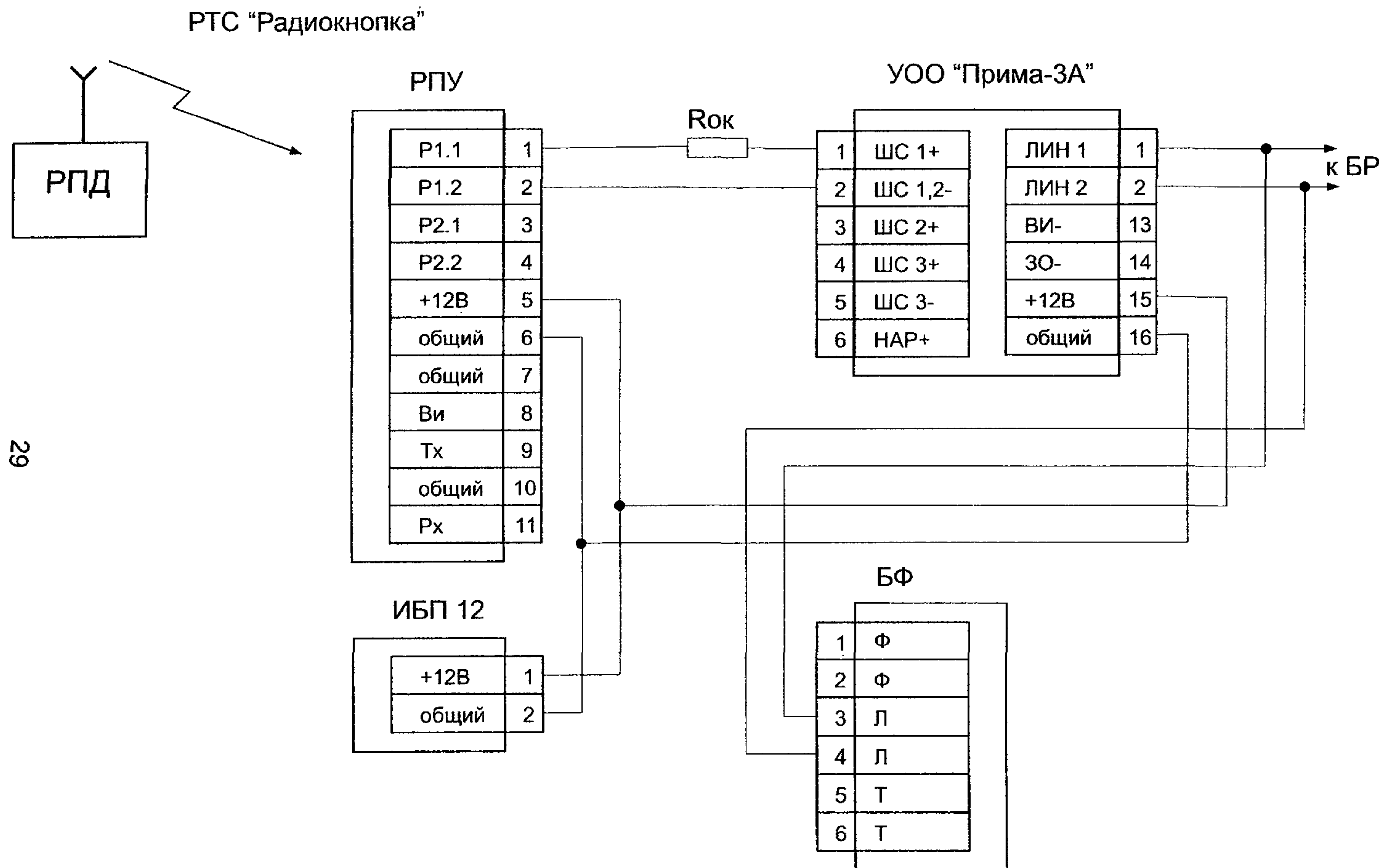
Рис. 7 - Схема подключения РТС "Радиокнопка" к УОО "Прима-3А"
