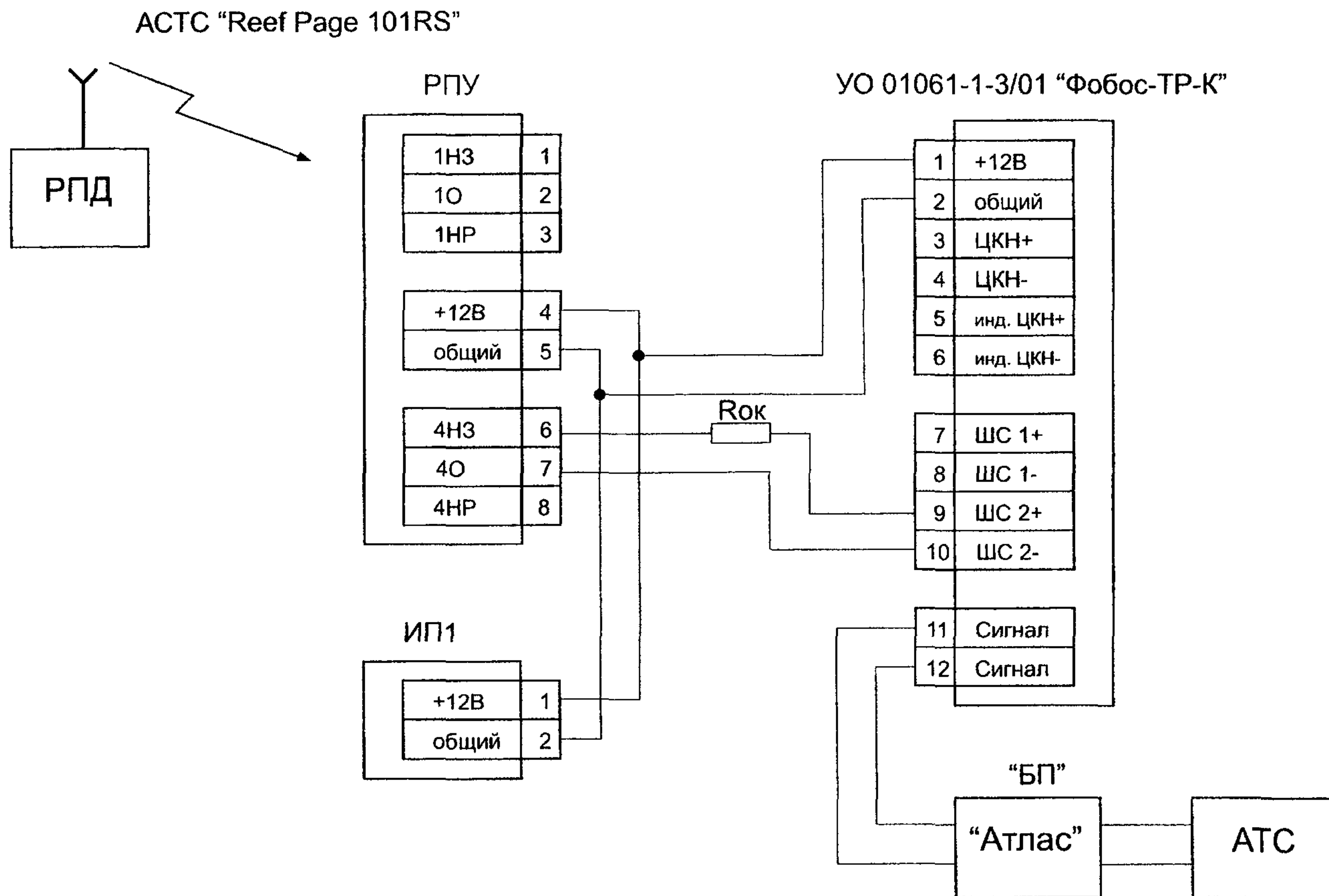
Рис. 2 - Схема подключения АСТС "Reef Page 101RS" к УО 01061-1-3/01 "Фобос-ТР-К"
