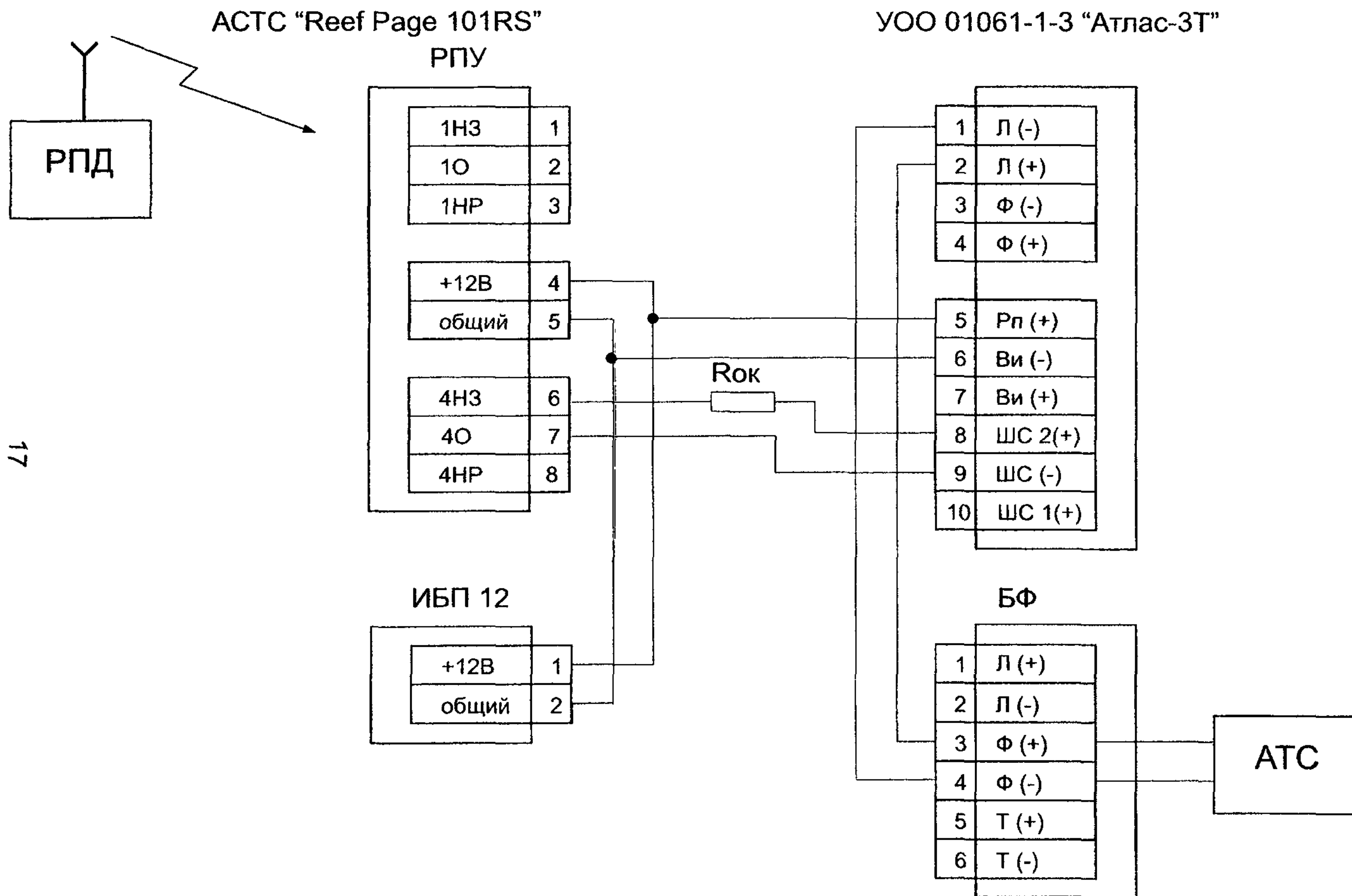
Рис 6 - Схема подключения АСТС "Reef Page 101RS" к YOO 01061-1-3 "Атлас-3Т"
