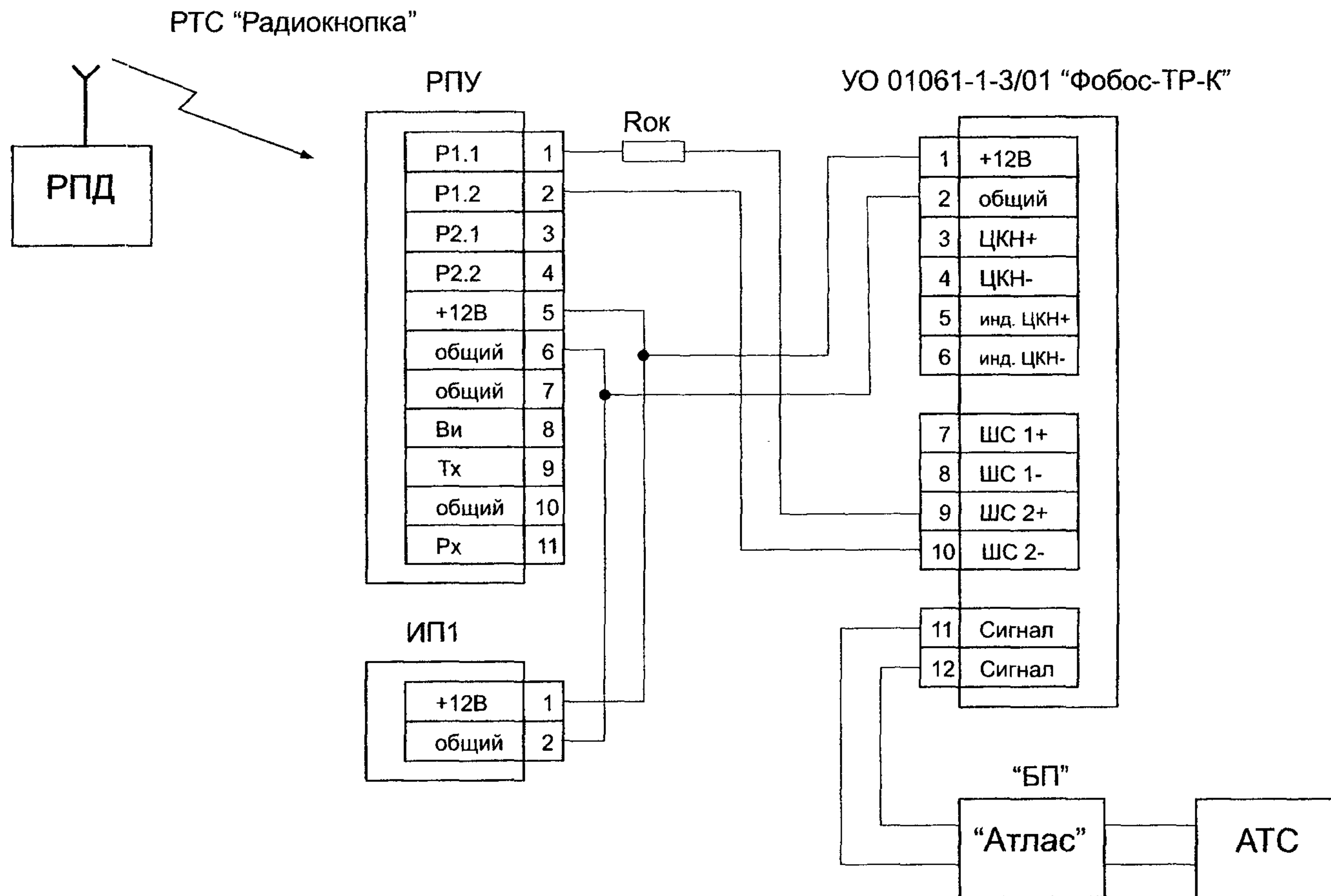
Рис 2 - Схема подключения РТС "Радиокнопка" к УО 01061-1-3/01 "Фобос-ТР-К"
