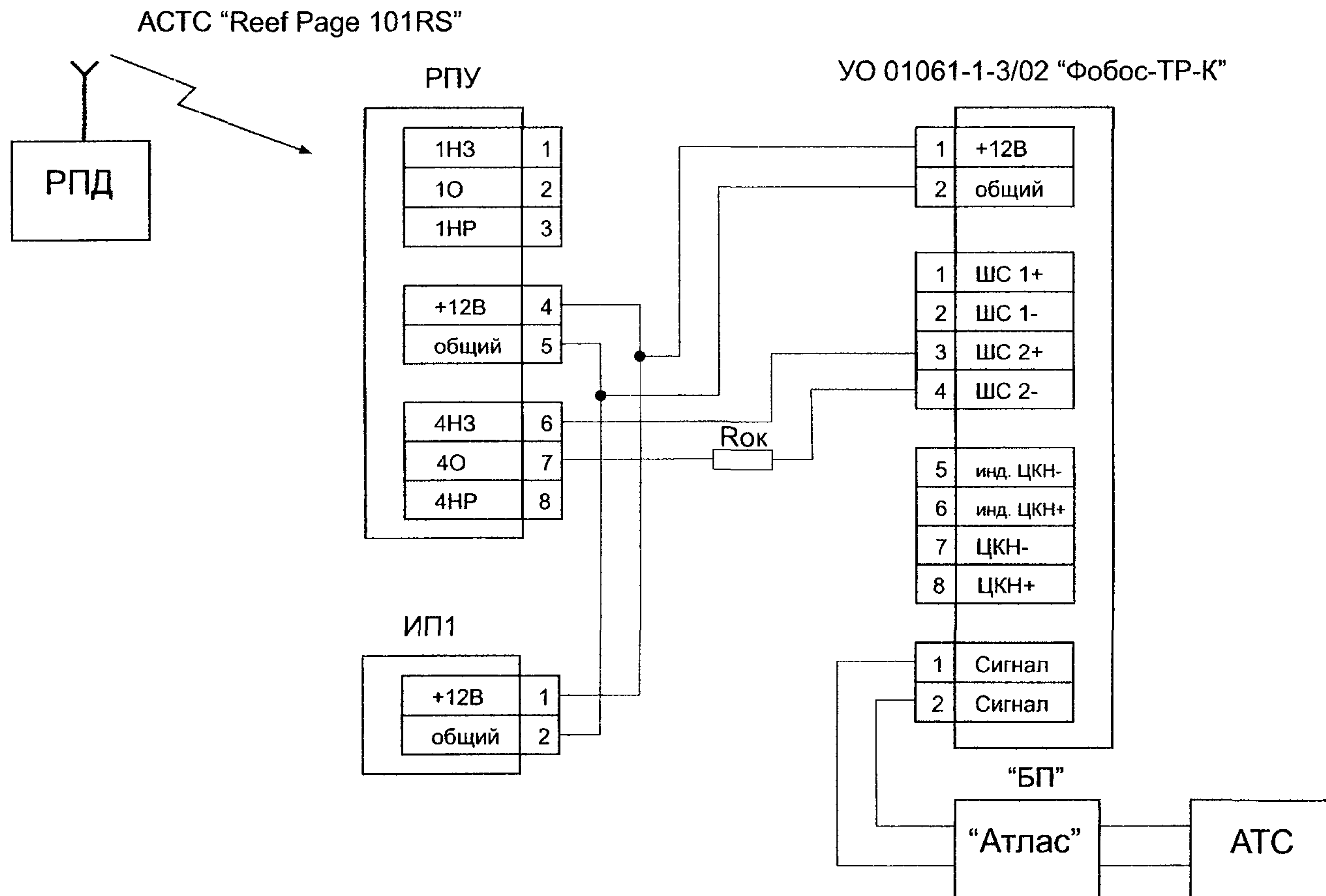
Рис. 3 - Схема подключения АСТС "Reef Page 101RS" к УО 01061-1-3/02 "Фобос-ТР-К"
