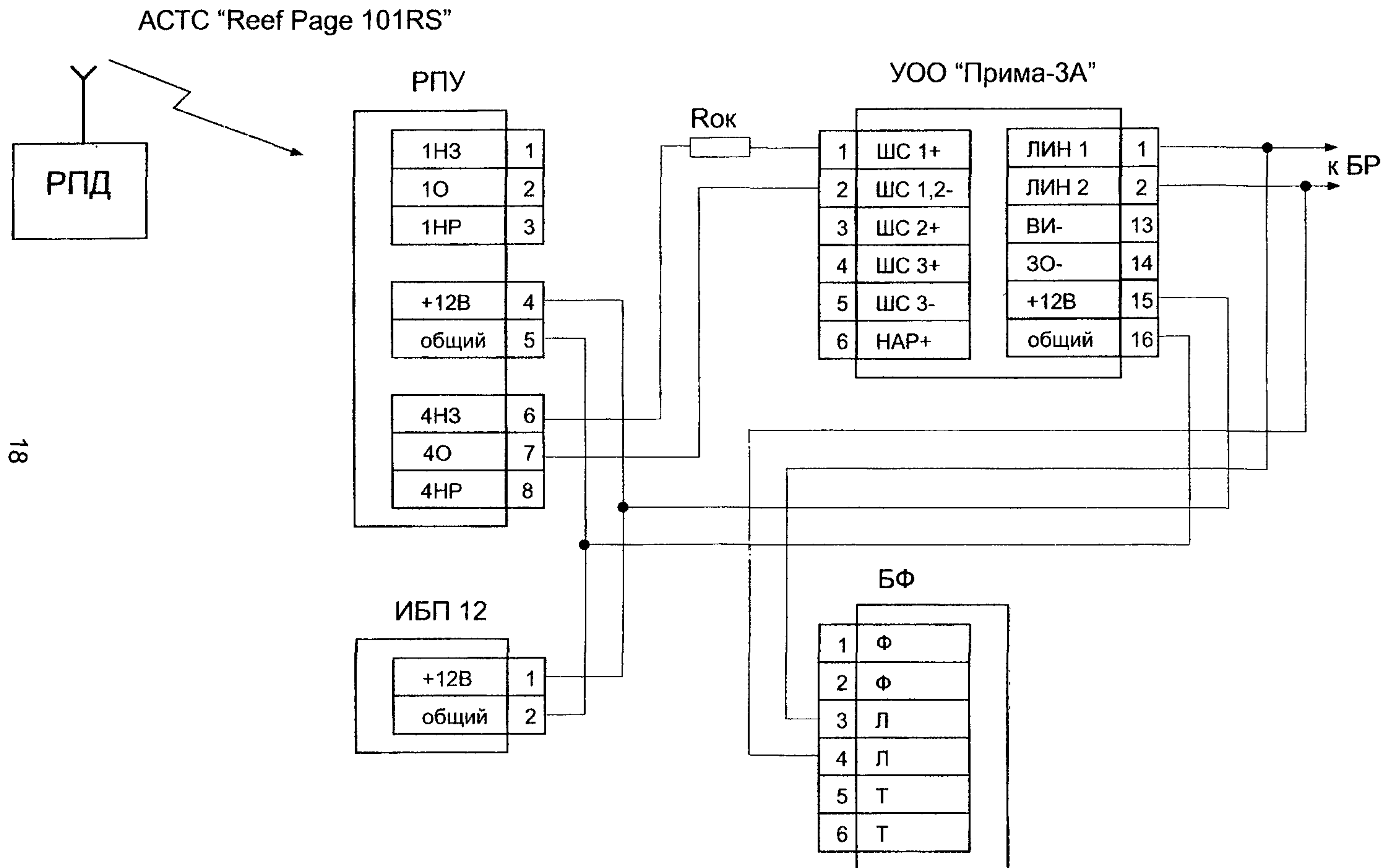
Рис. 7 - Схема подключения АСТС "Reef Page 101RS" к УОО "Прима-3А"
