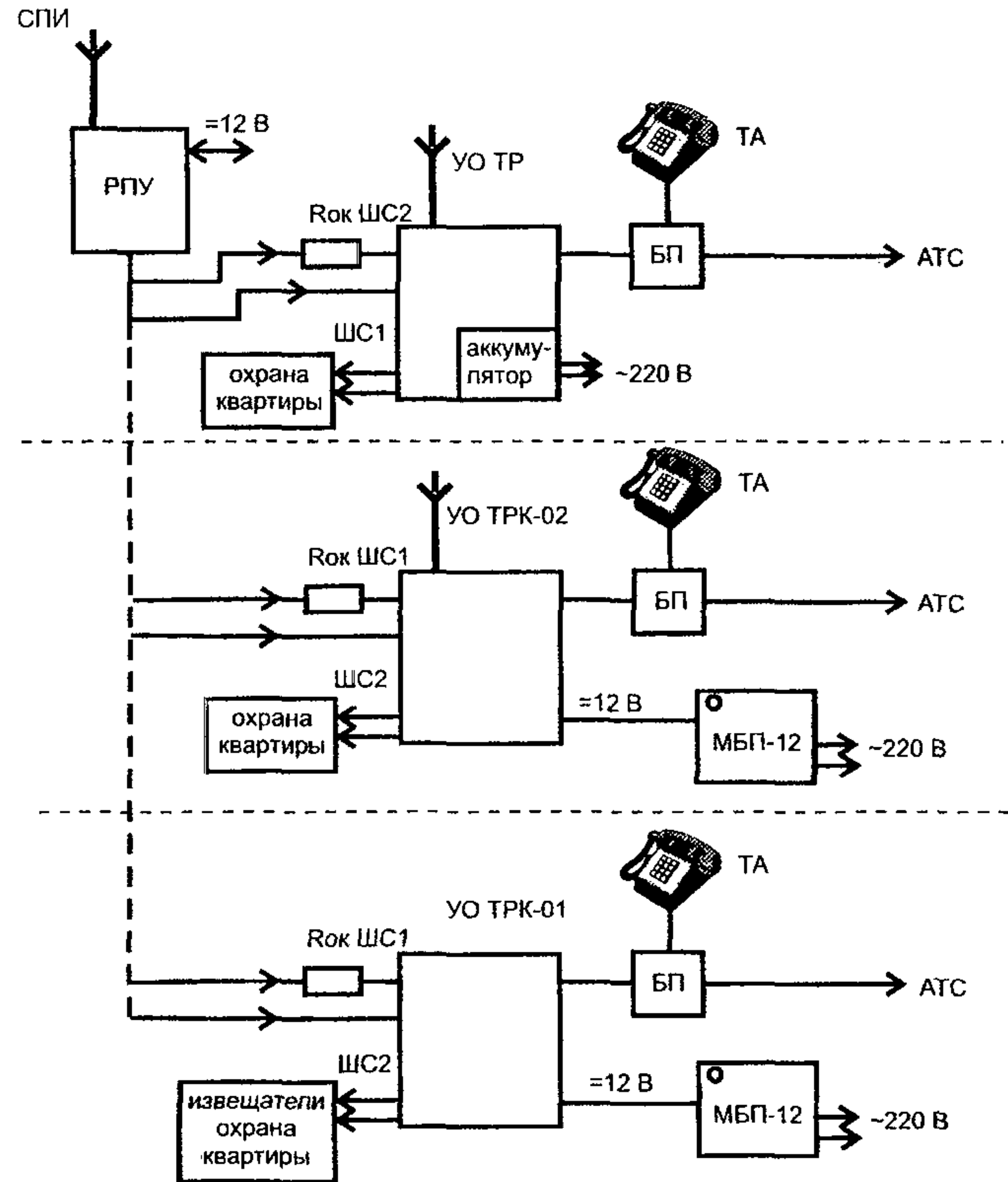
Рис. 1 - Схема подключения АСТС "Reef Page 101RS" к СПИ "Фобос-ТР", "Фобос-3"
