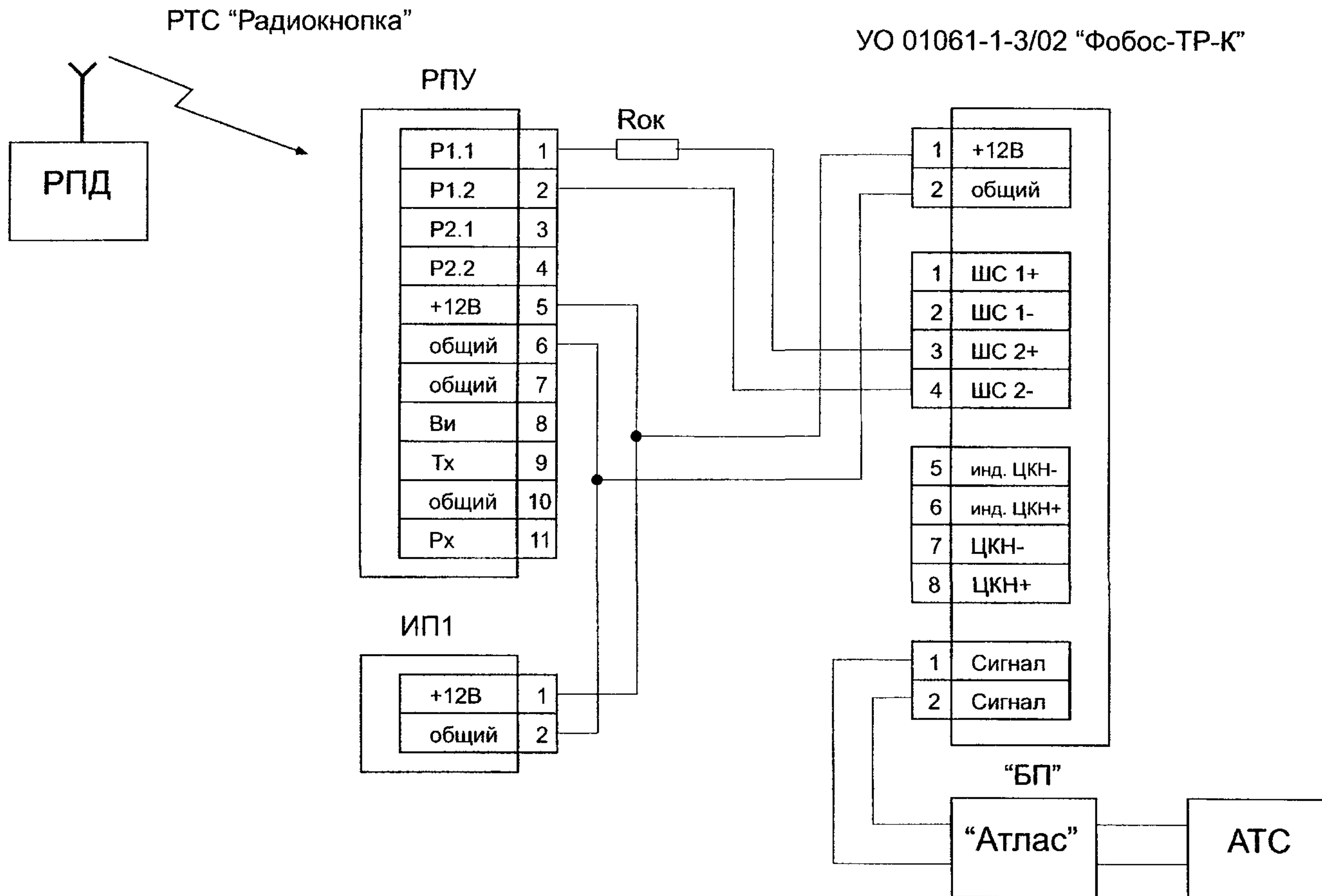
Рис. 3 - Схема подключения РТС "Радиокнопка" к УО 01061-1-3/02 "Фобос-ТР-К"
