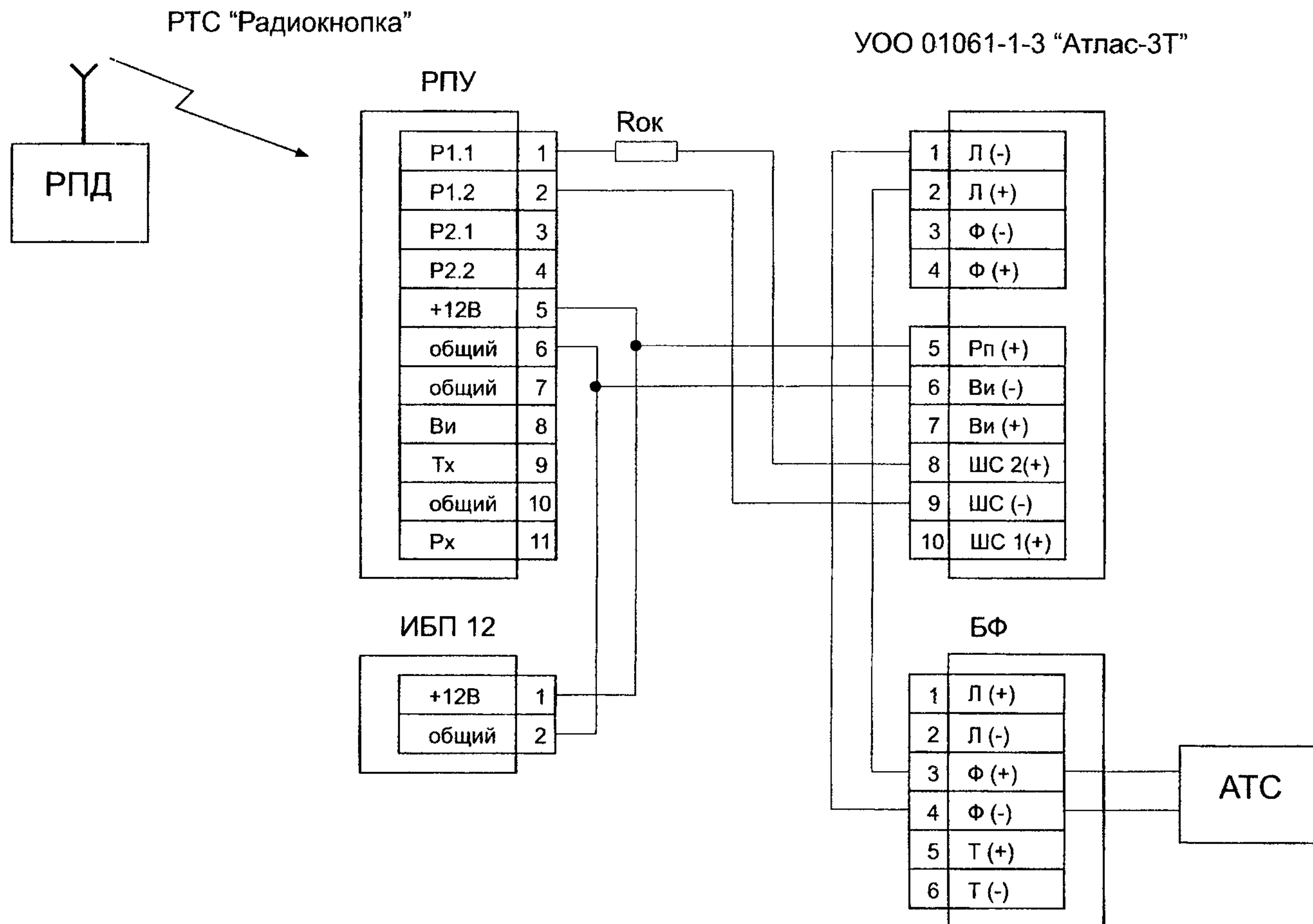
Рис. 6 - Схема подключения РТС "Радиокнопка" к УОО 01061-1-3 "Атлас-3Т"
