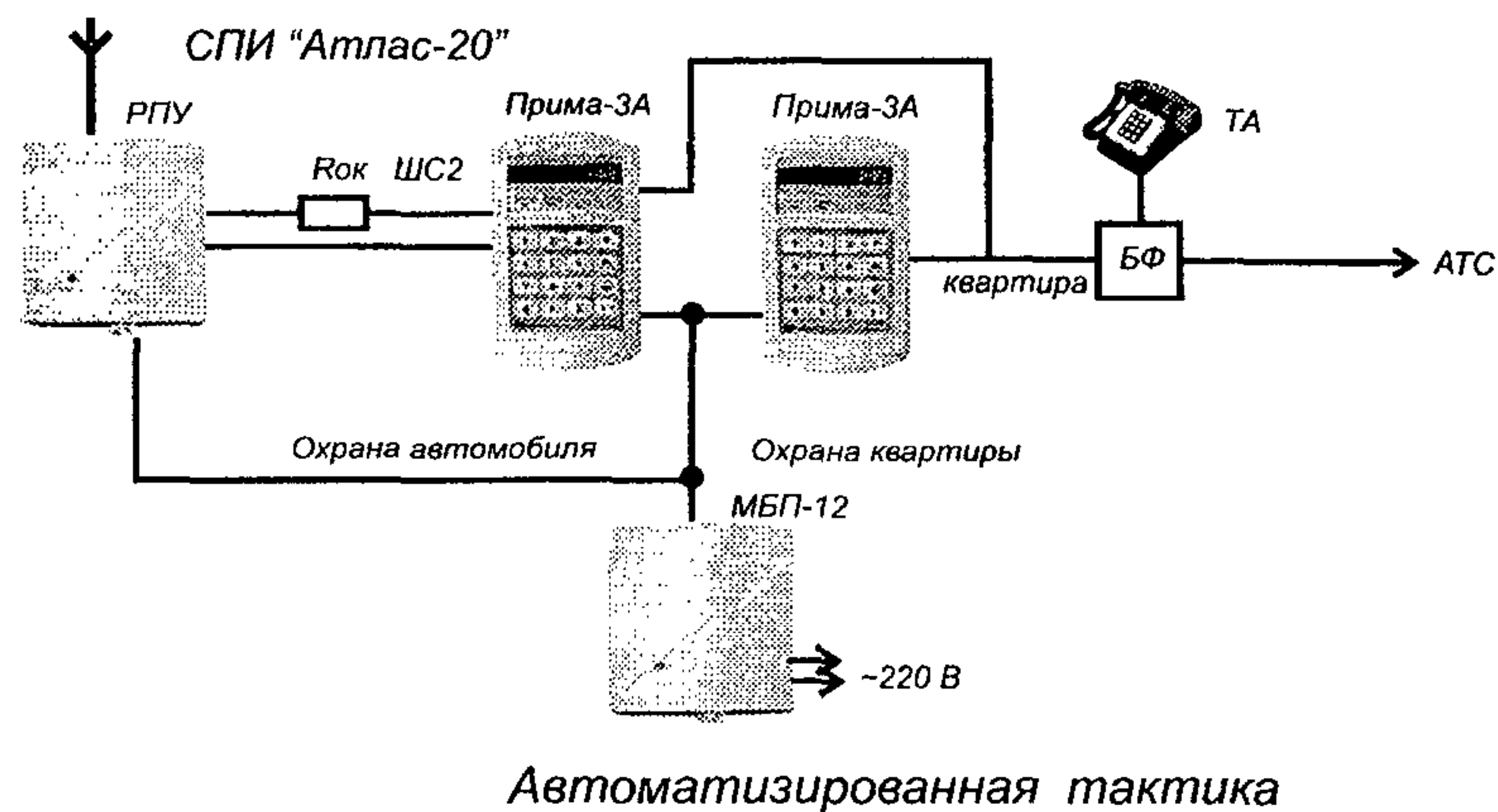
Рис. 5 - Схема подключения РТС “Радиокнопка” к СПИ “Атлас-20”
