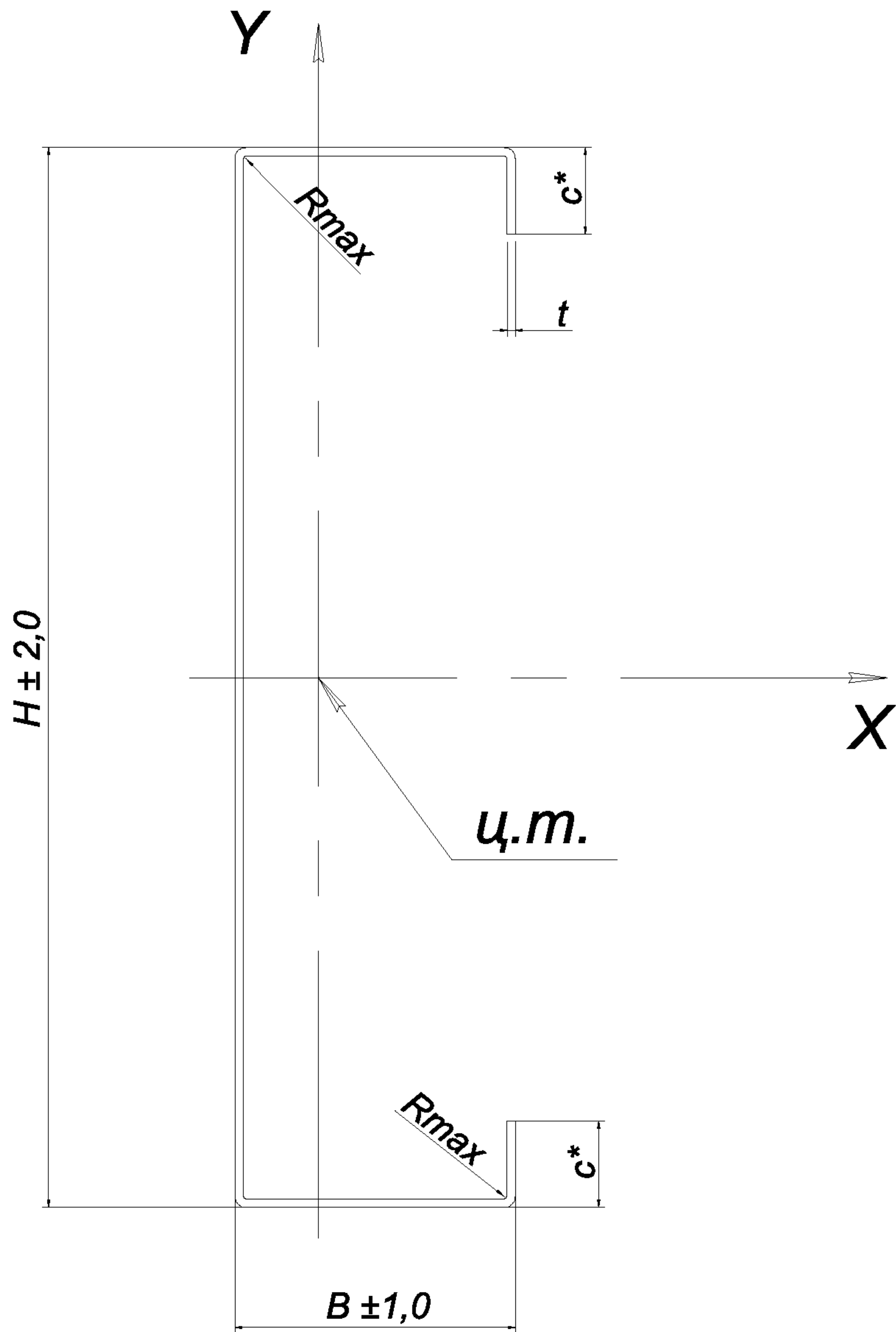
Примечание: 1. * -размер для справок Рисунок 4. Профили ПГС
