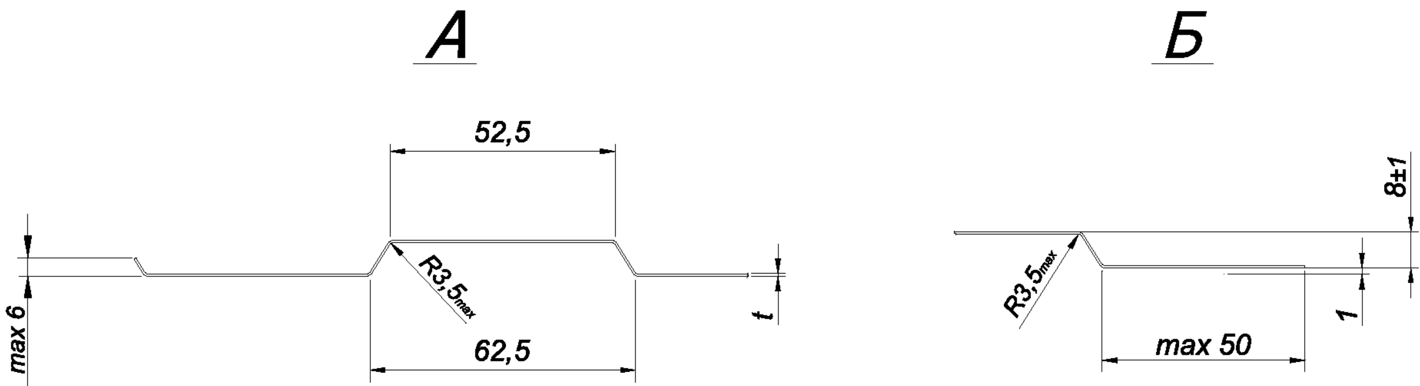
Рисунок 1 – Профилированный лист С8-1150
