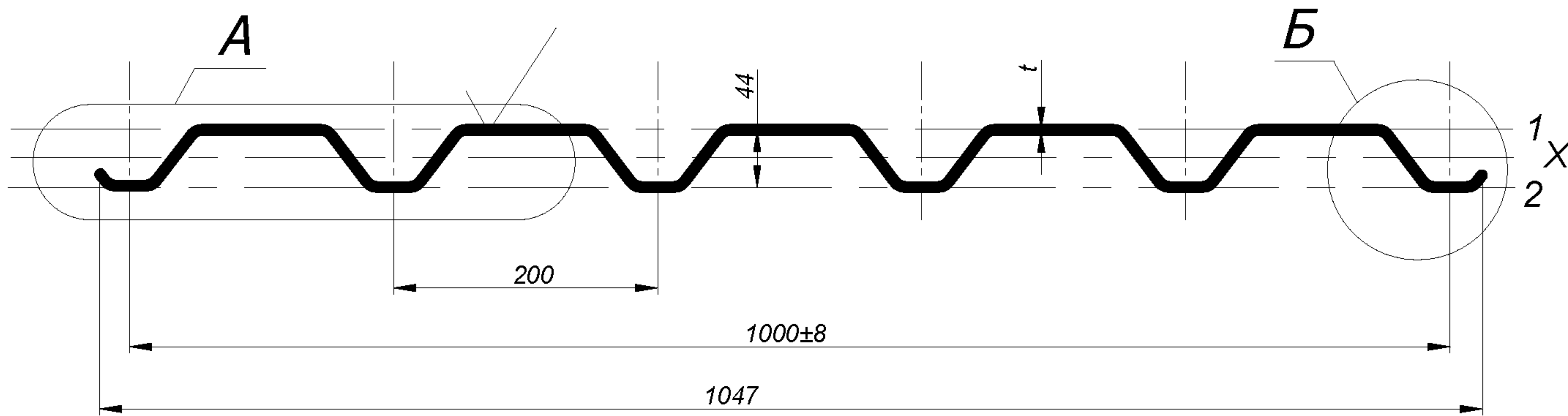
Рисунок 5.1 – Профилированный лист С44-1000 Вид1.
