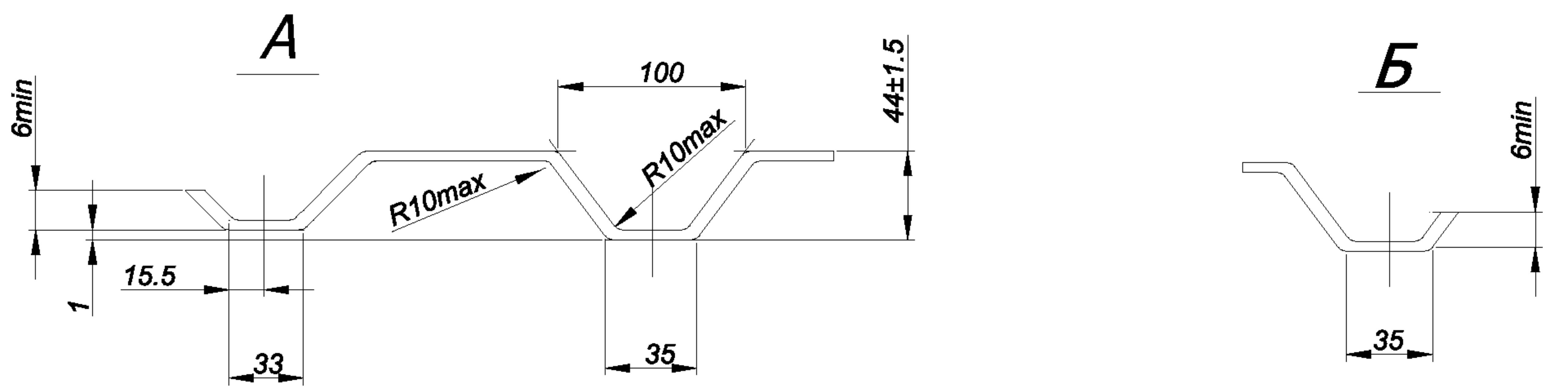
Рисунок 5.2 – Профилированный лист С44-1000 Вид2.
