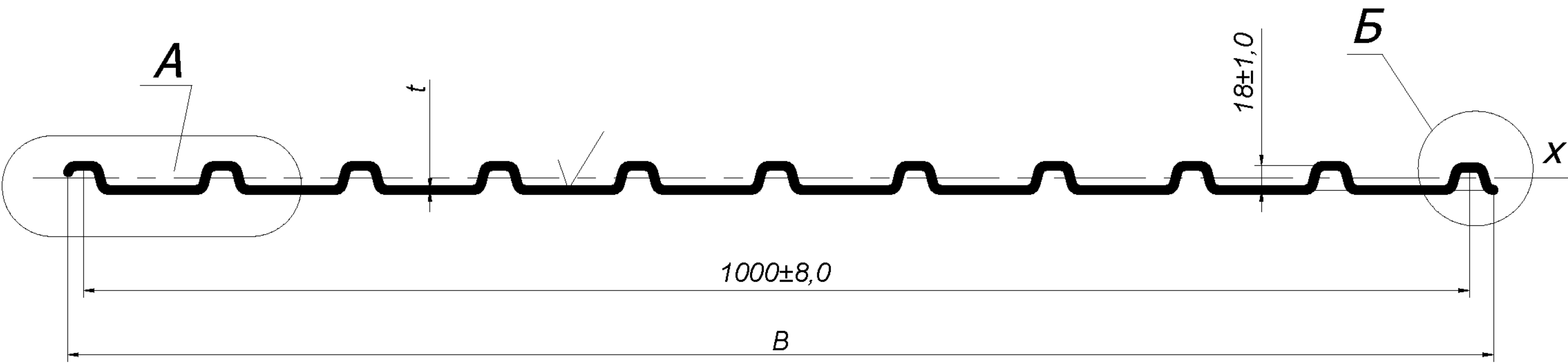
Рисунок 8 – Профилированный лист С18-1000.
