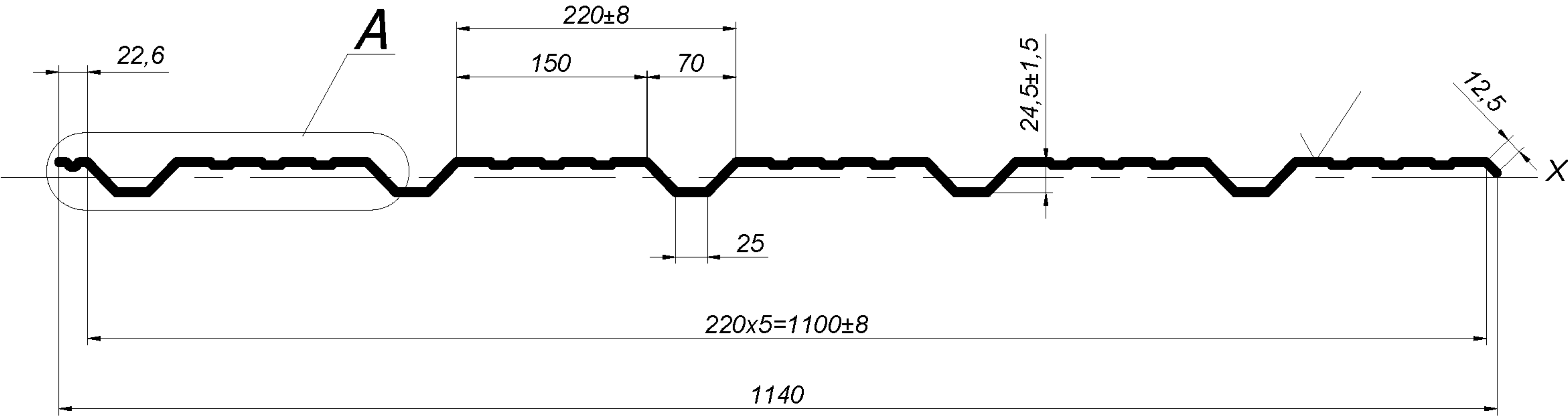
Рисунок 4.1 – Профилированный лист С25-1100. Вид 1
