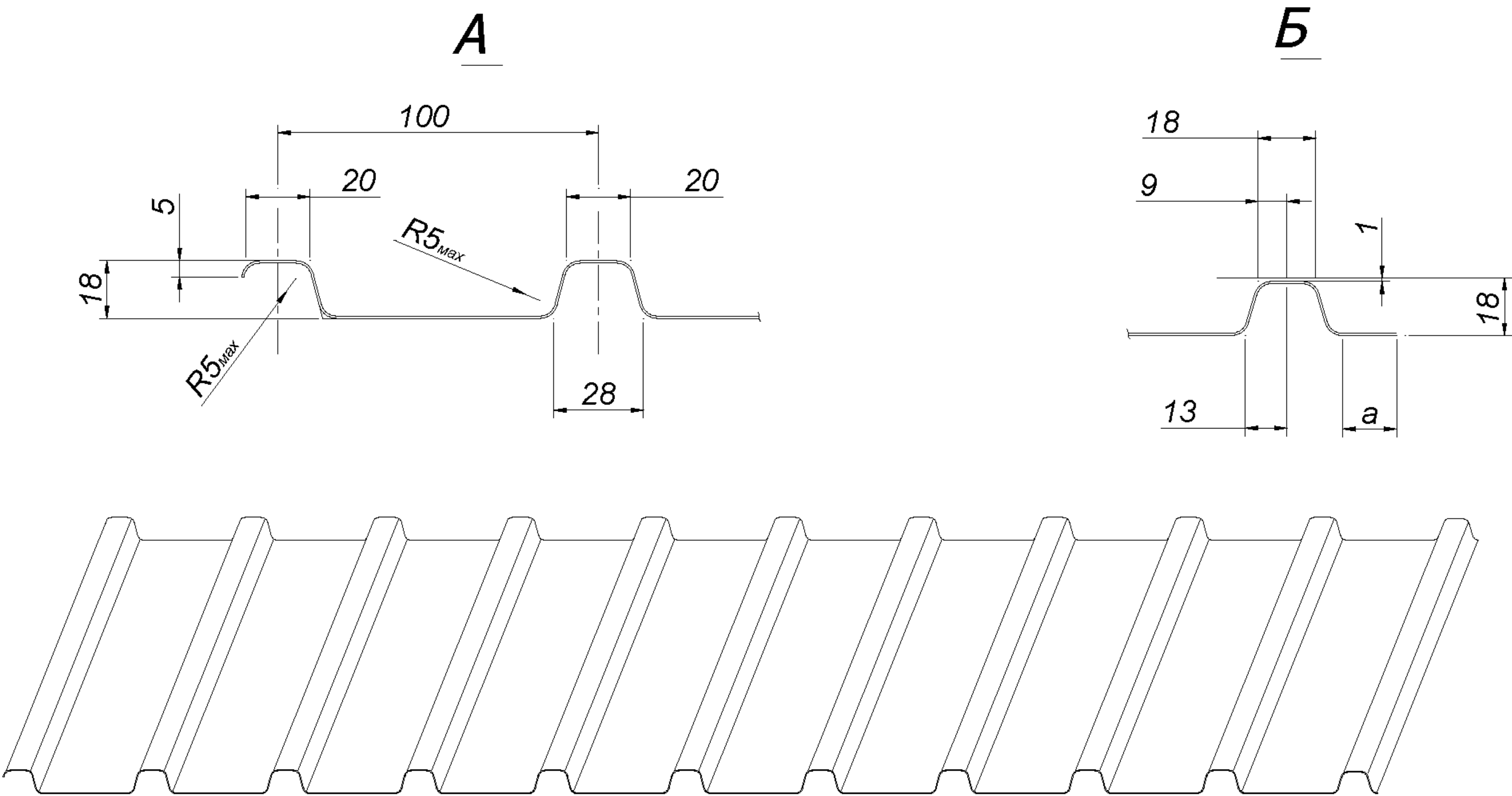
Рисунок 8 – Профилированный лист С18-1000.
