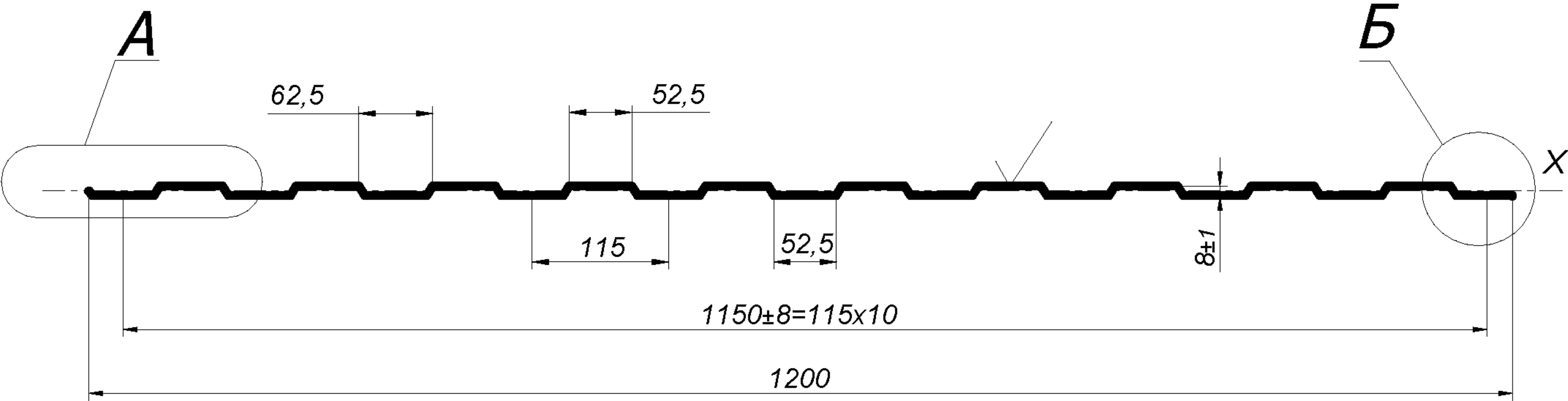
Рисунок 1 – Профилированный лист С8-1150
