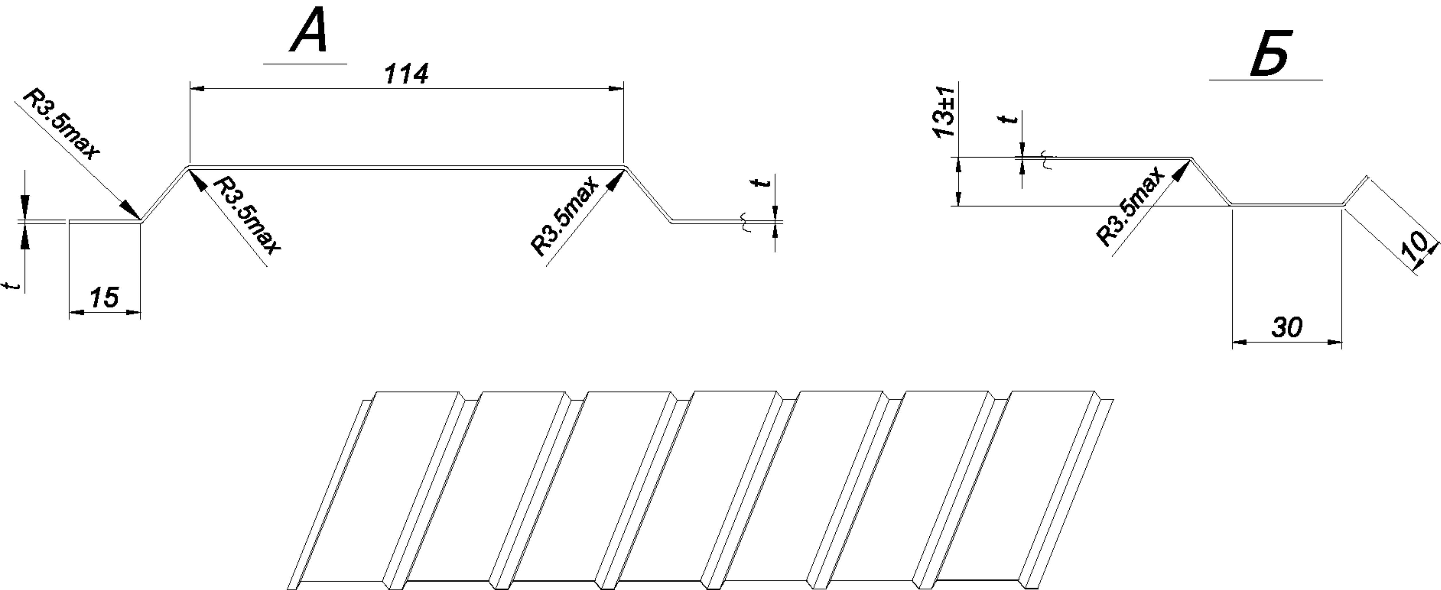
Рисунок 2.2 – Профилированный лист С13-А-1150 тип А. Вид 2
