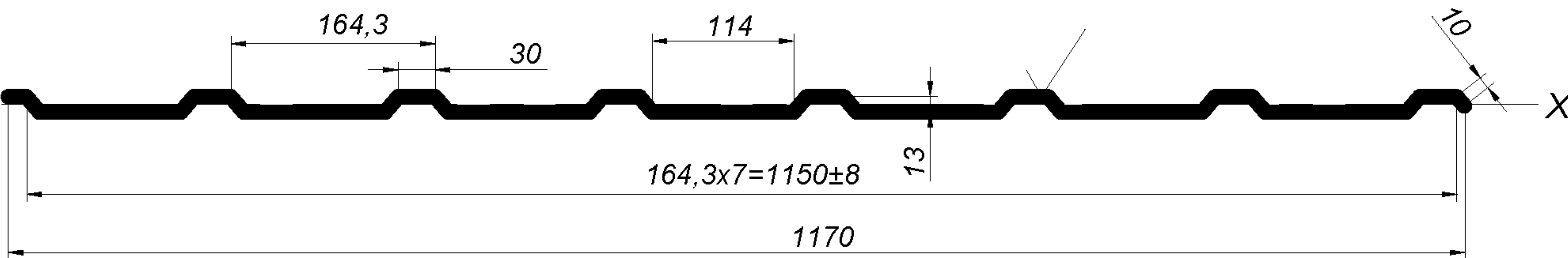
Рисунок 2.2 – Профилированный лист С13-А-1150 тип А. Вид 2
