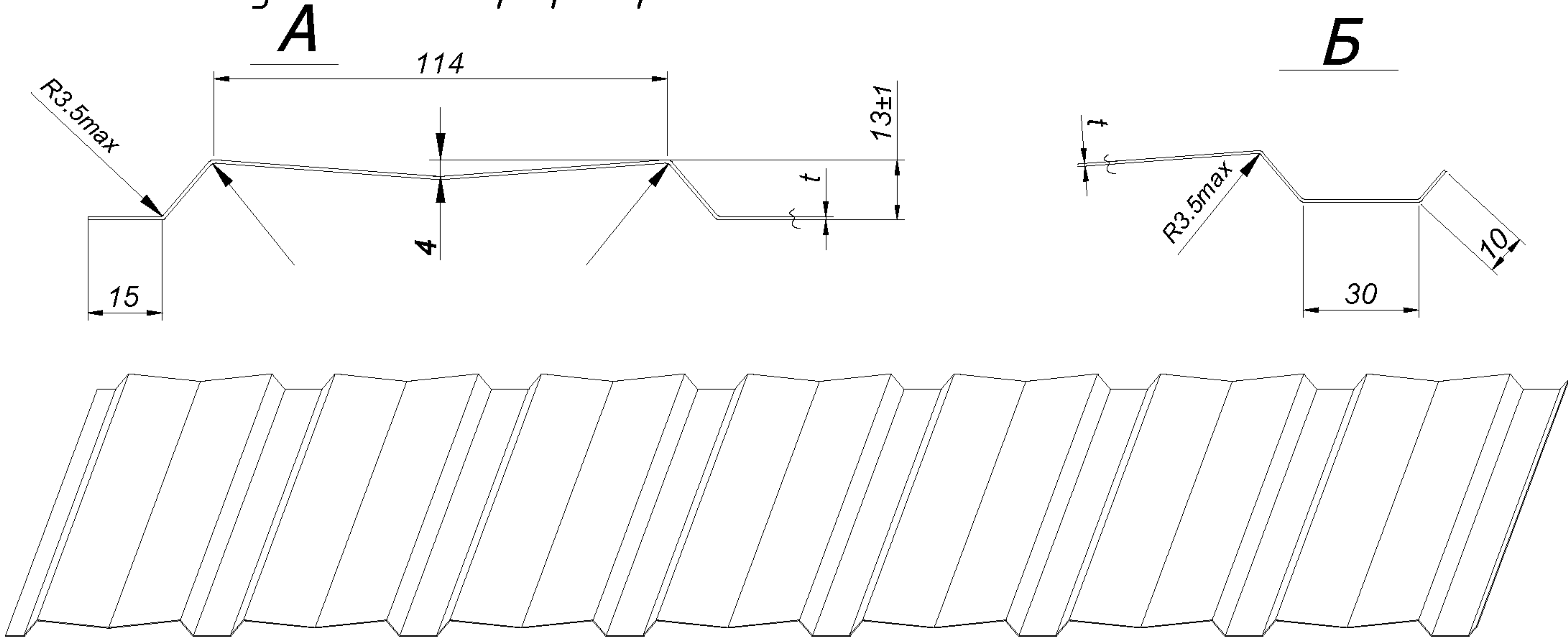
Рисунок 3.1 – Профилированный лист С13-Б-1150 тип Б. Вид 2
