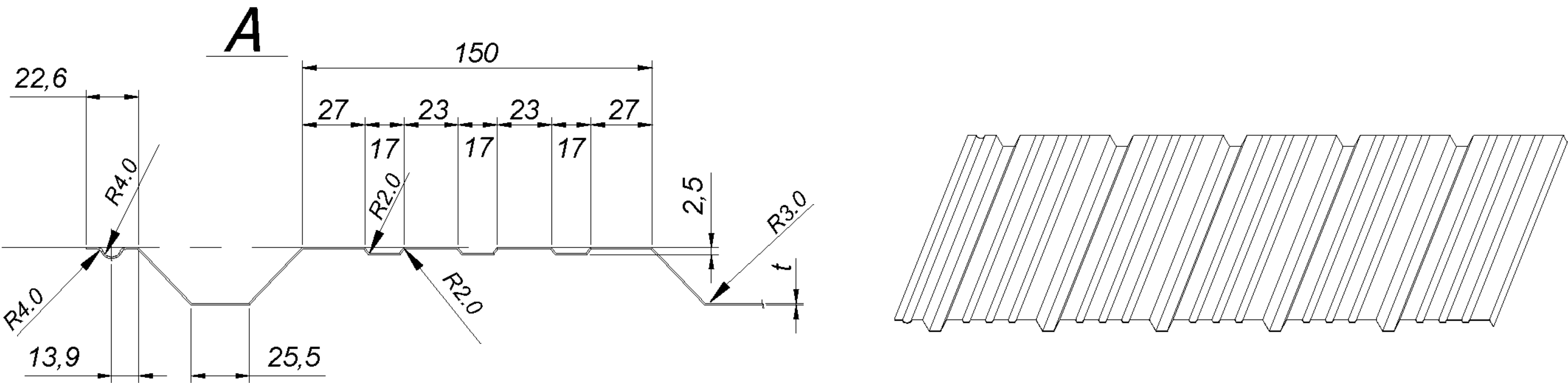
Рисунок 4.2 – Профилированный лист С25-1100. Вид 2
