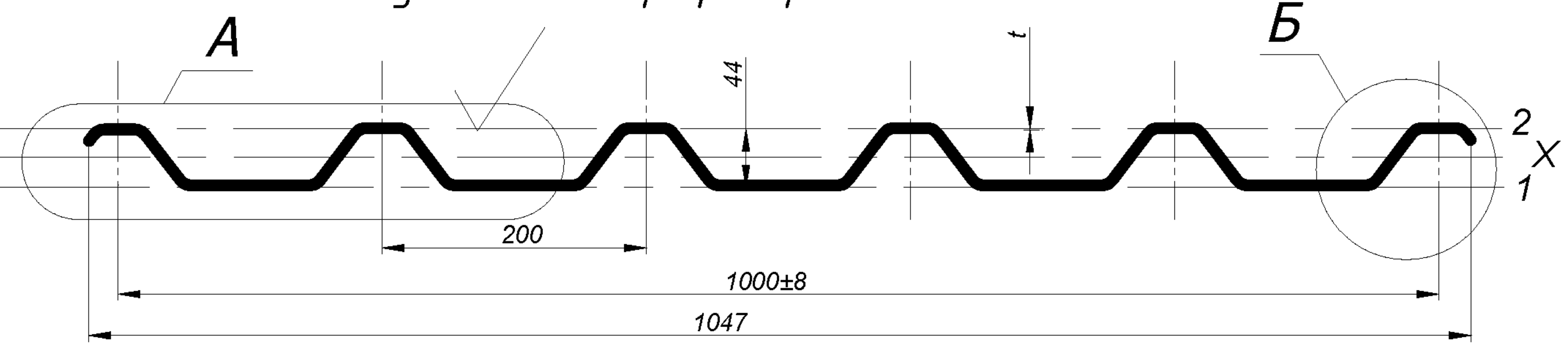
Рисунок 5.2 – Профилированный лист С44-1000 Вид2.
