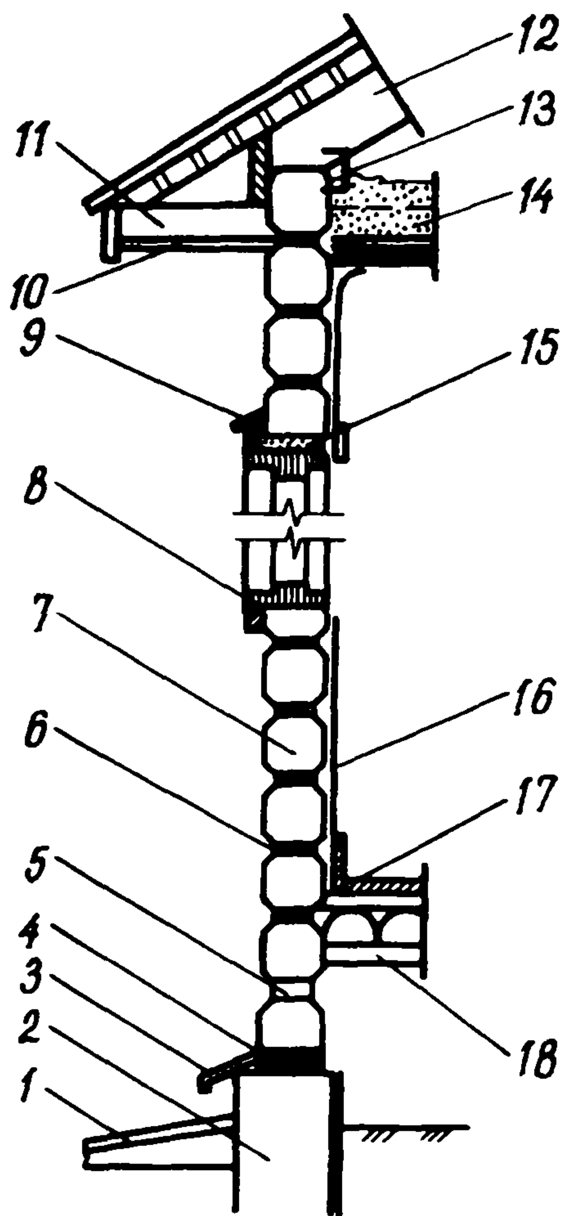
Рис. 5. Разрез брусчатой стены:
