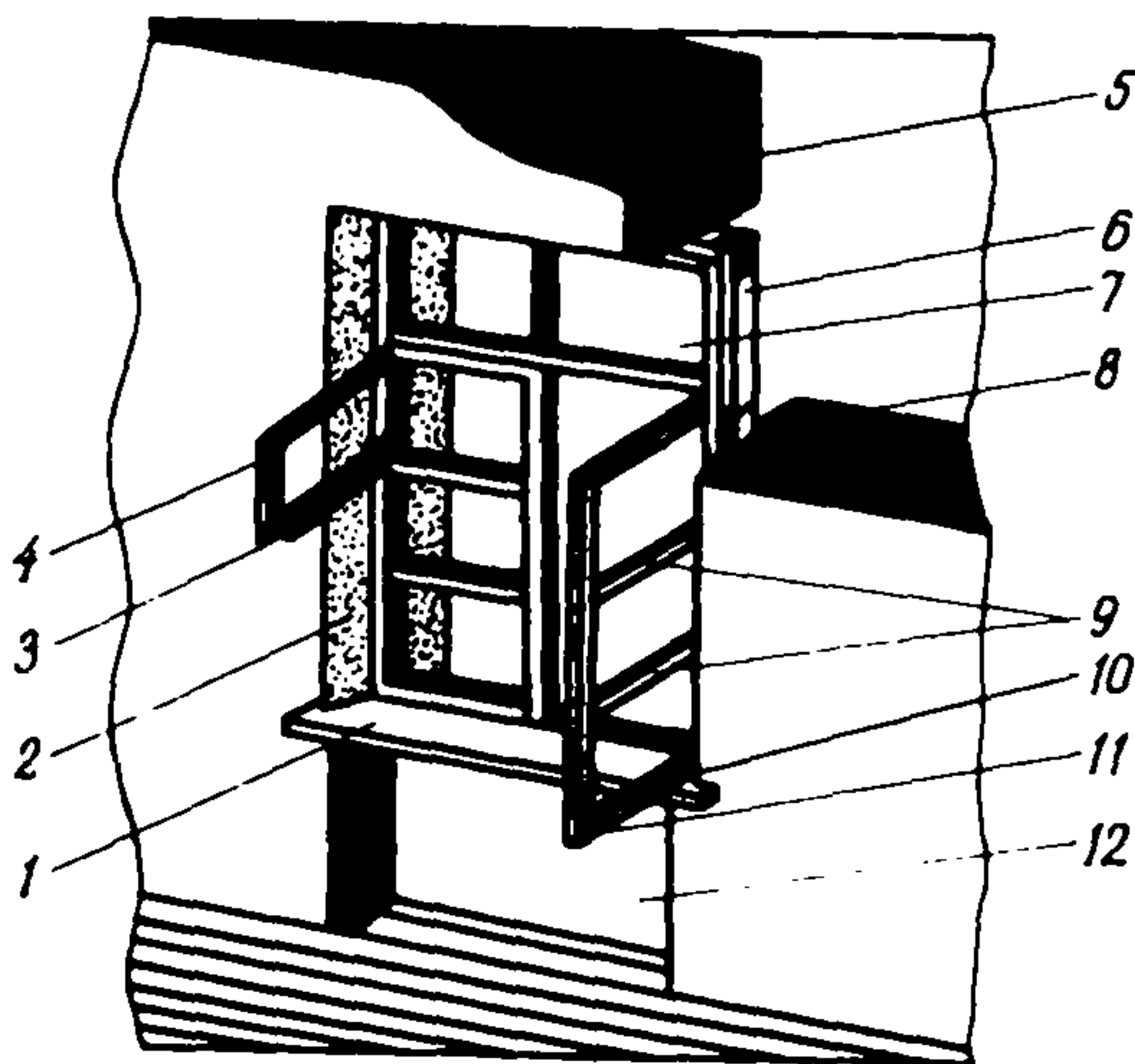
Рис. 14. Окно в оконном проеме:
