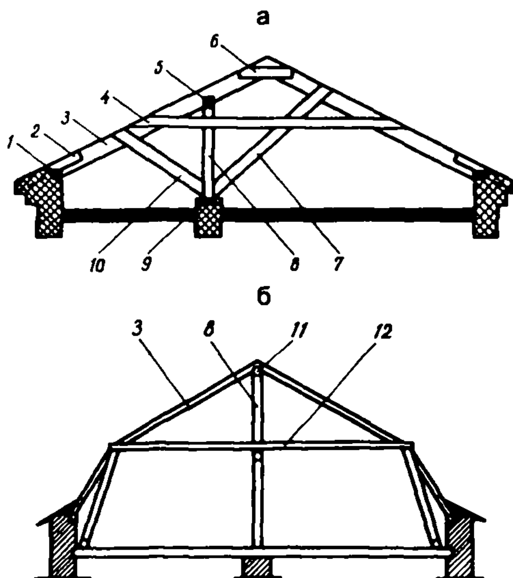
Рис. 11. Схемы и детали наслонных стропил двускатной крыши со смещенной внутренней опорой (а) и стропил мансардной крыши (б): 1 - подстропильный брус (мауэрлат); 2 - кобылка; 3 - стропильная нога (балка); 4 - ригель; 5 - горизонтальный брус (верхний прогон); 6 - накладка; 7, 10 - подкосы; 8 - стойка; 9 - подкладка; 11 - коньковый прогон; 12 - затяжка
