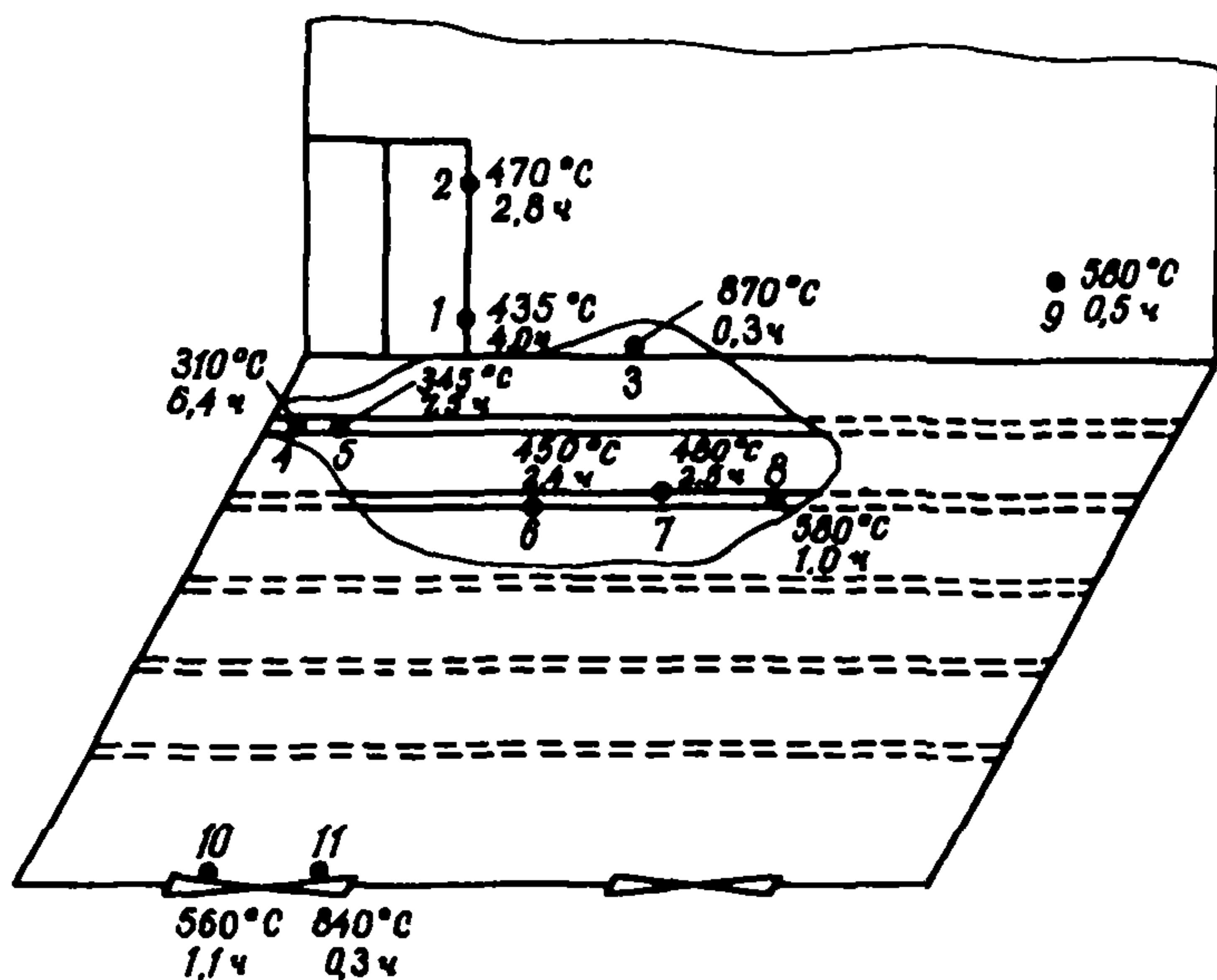
Рис. 3. Схема места пожара, точки отбора проб
