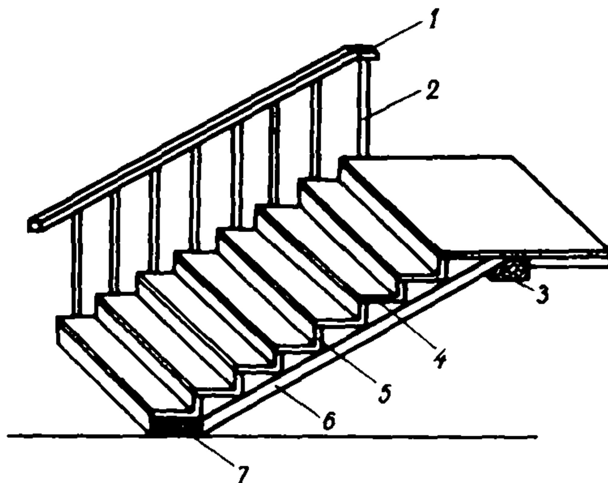
Рис. 13. Внутренняя деревянная лестница:
