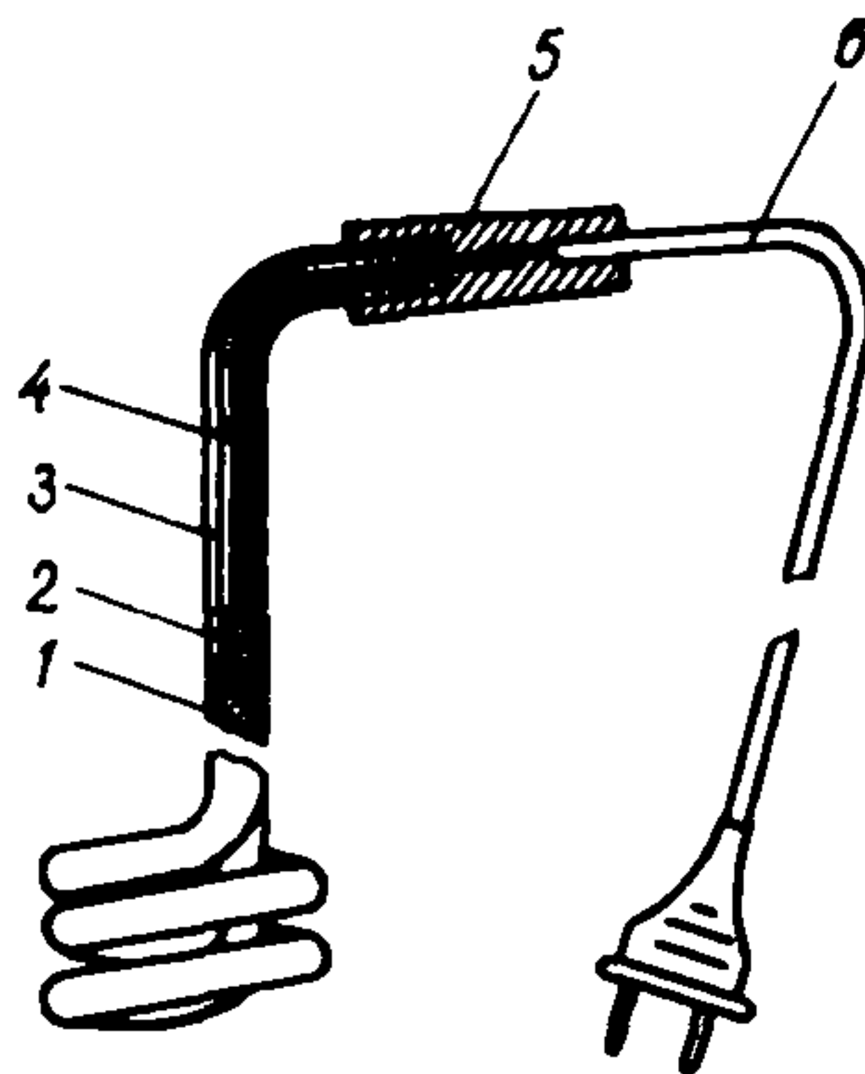
Рис. 35. Электрокипятильник:
