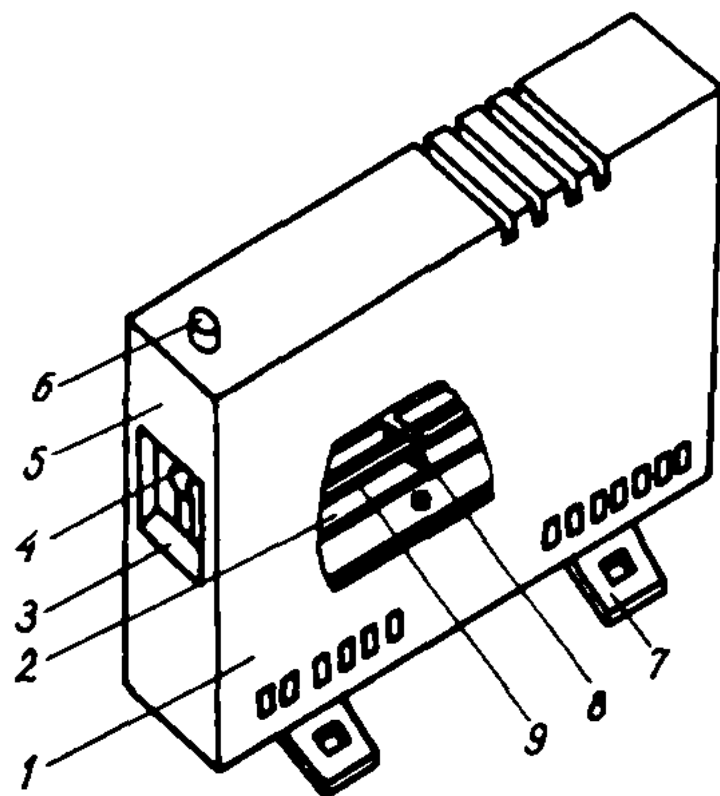
Рис. 37. Электроконвектор ЭВПС 1,0/220:
