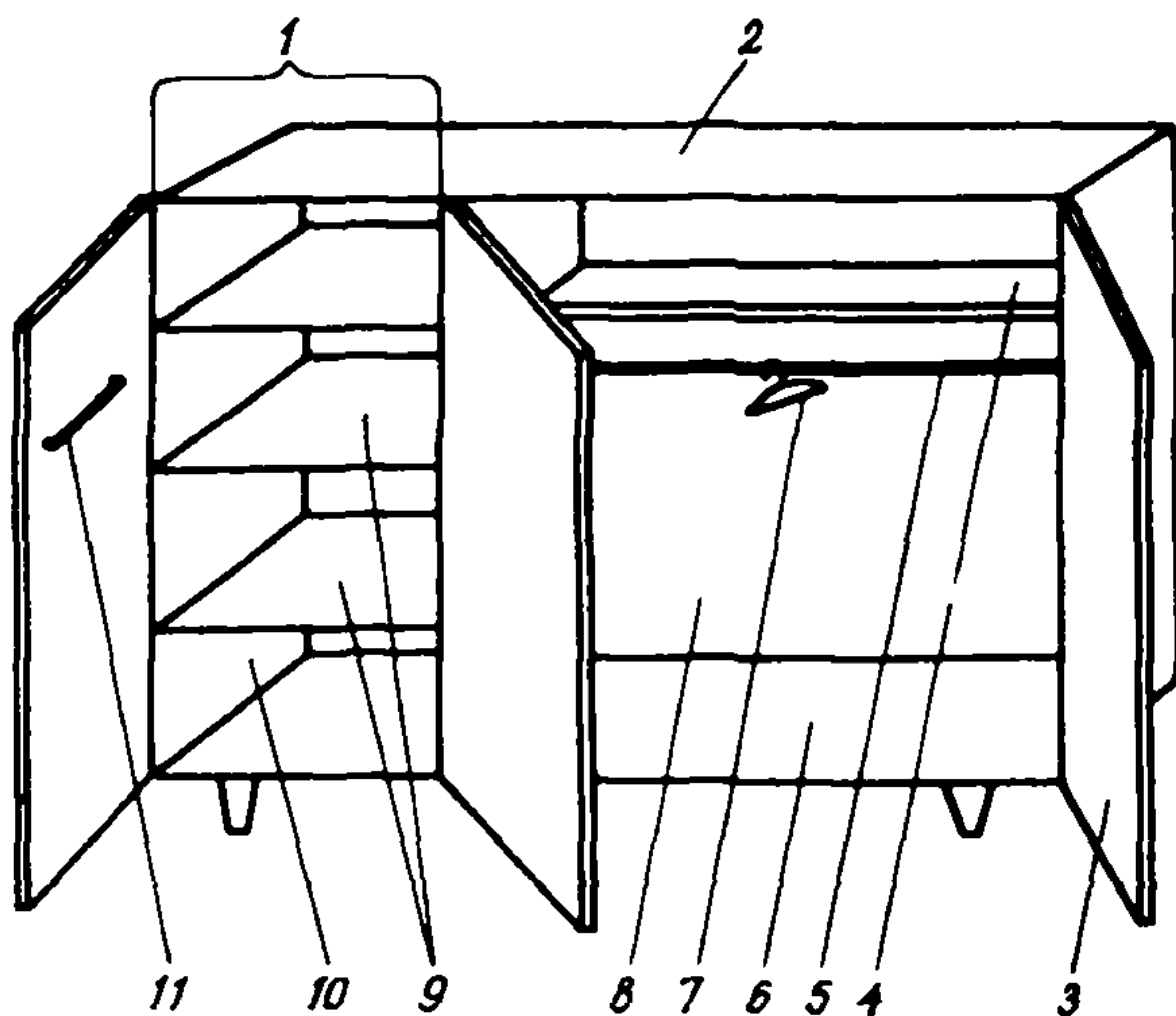
Рис. 26. Шкаф-шифоньер трехстворчатый:
