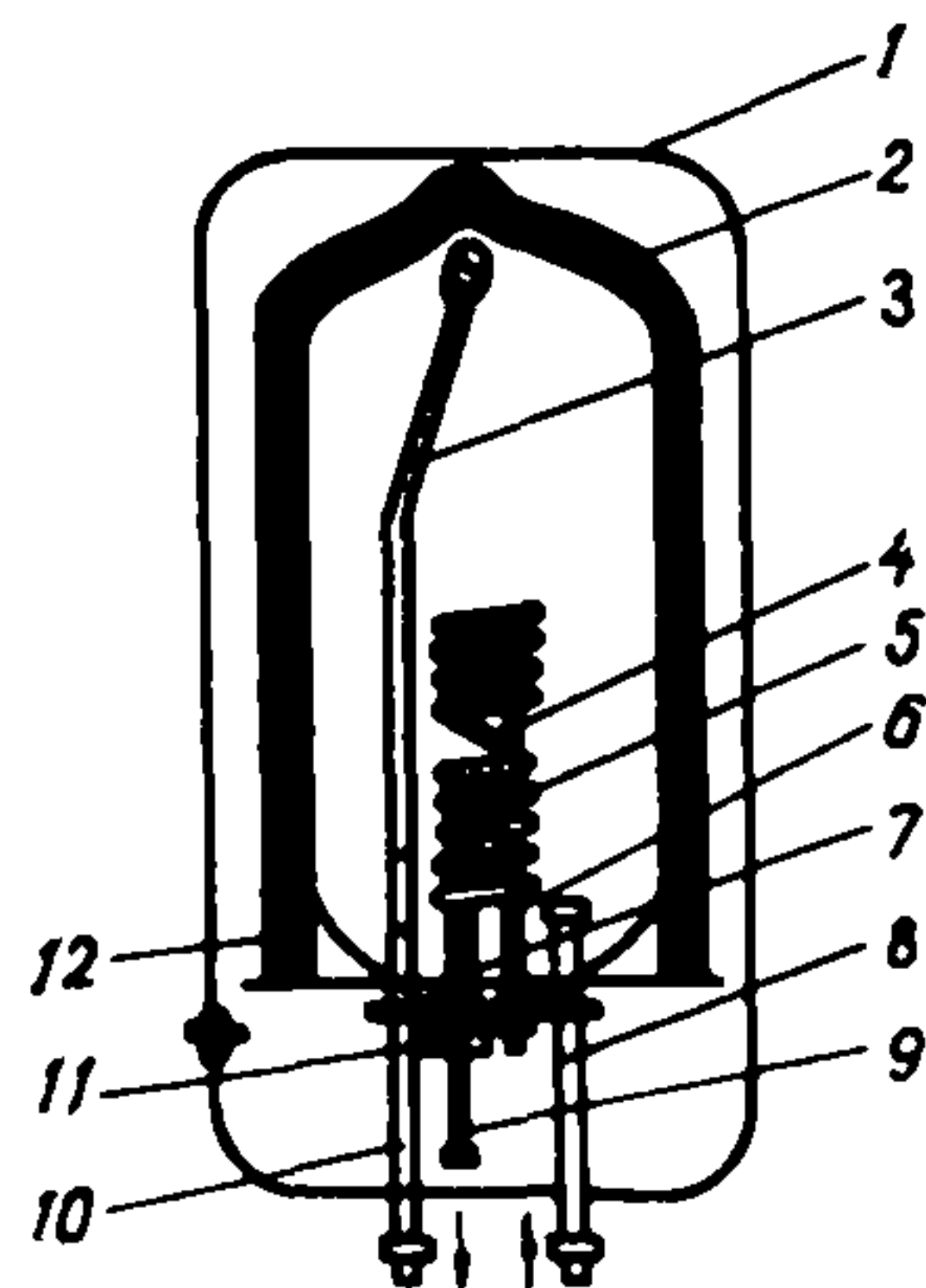
Рис. 34. Проточный электро-нагреватель (титан):
