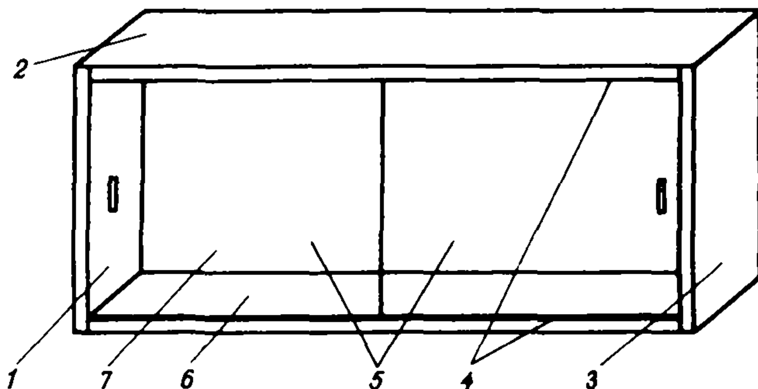
Рис. 20. Полка книжная:
