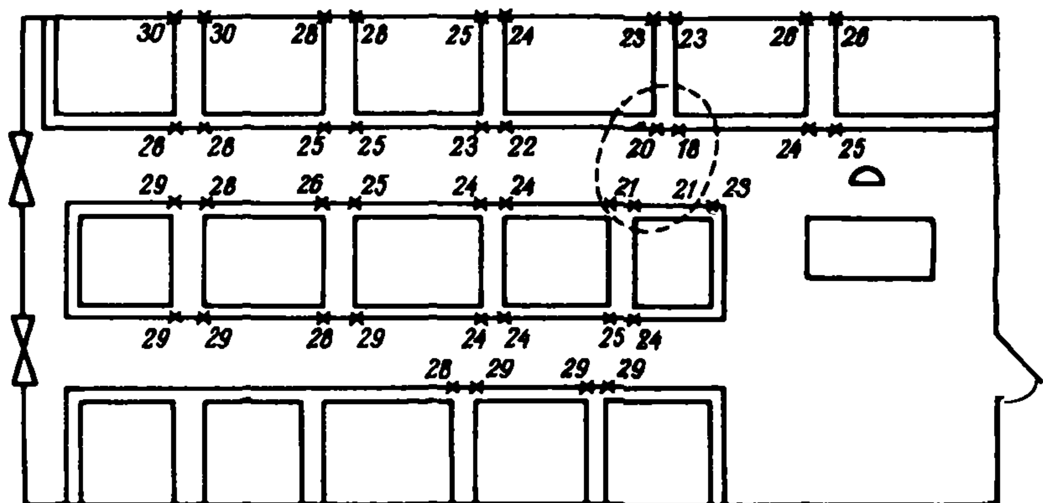
Рис. 4. План помещения и результаты измерения тока размагничивания
