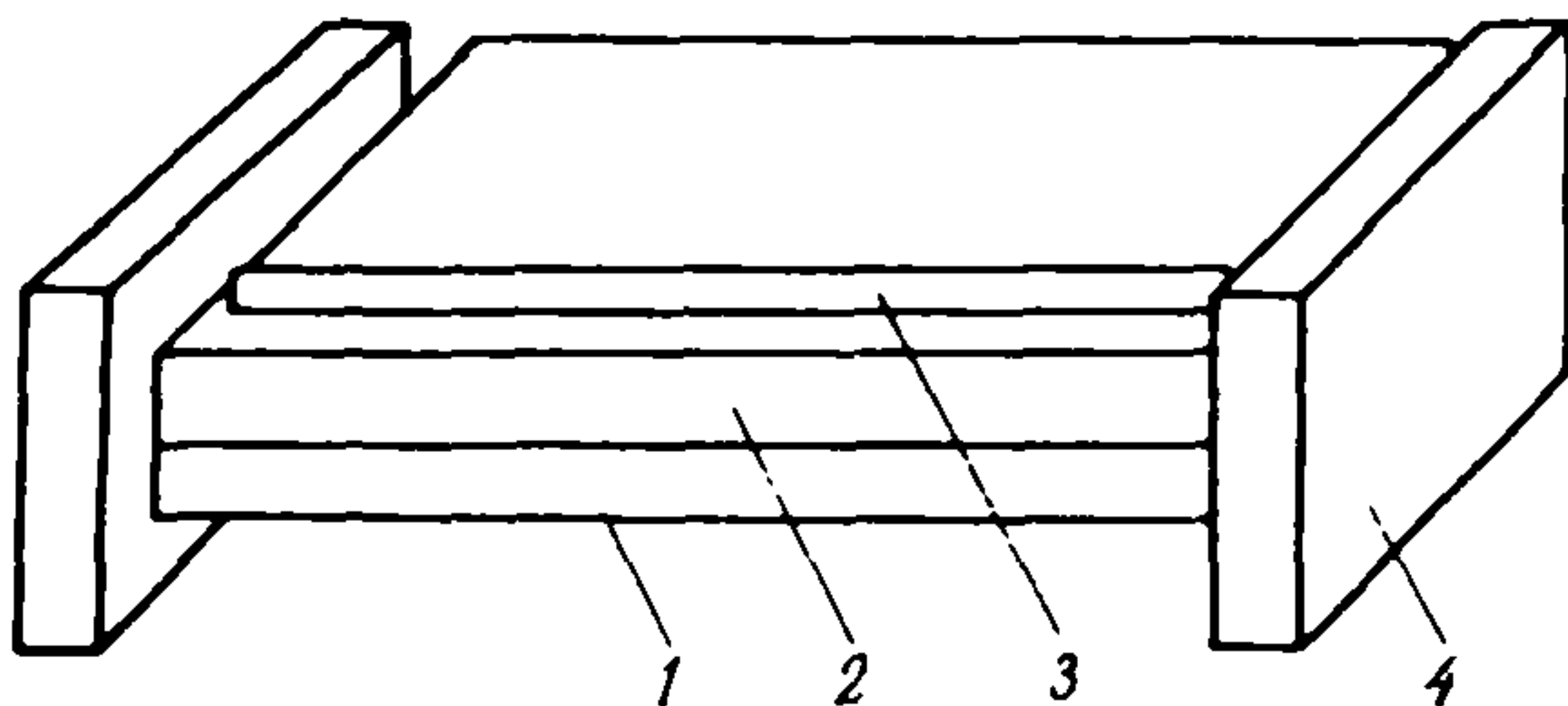
Рис. 19. Кровать: 1 - внешняя доска рамы кровати; 2 - матрас; 3 - наматрасник ватный; 4 - спинка
