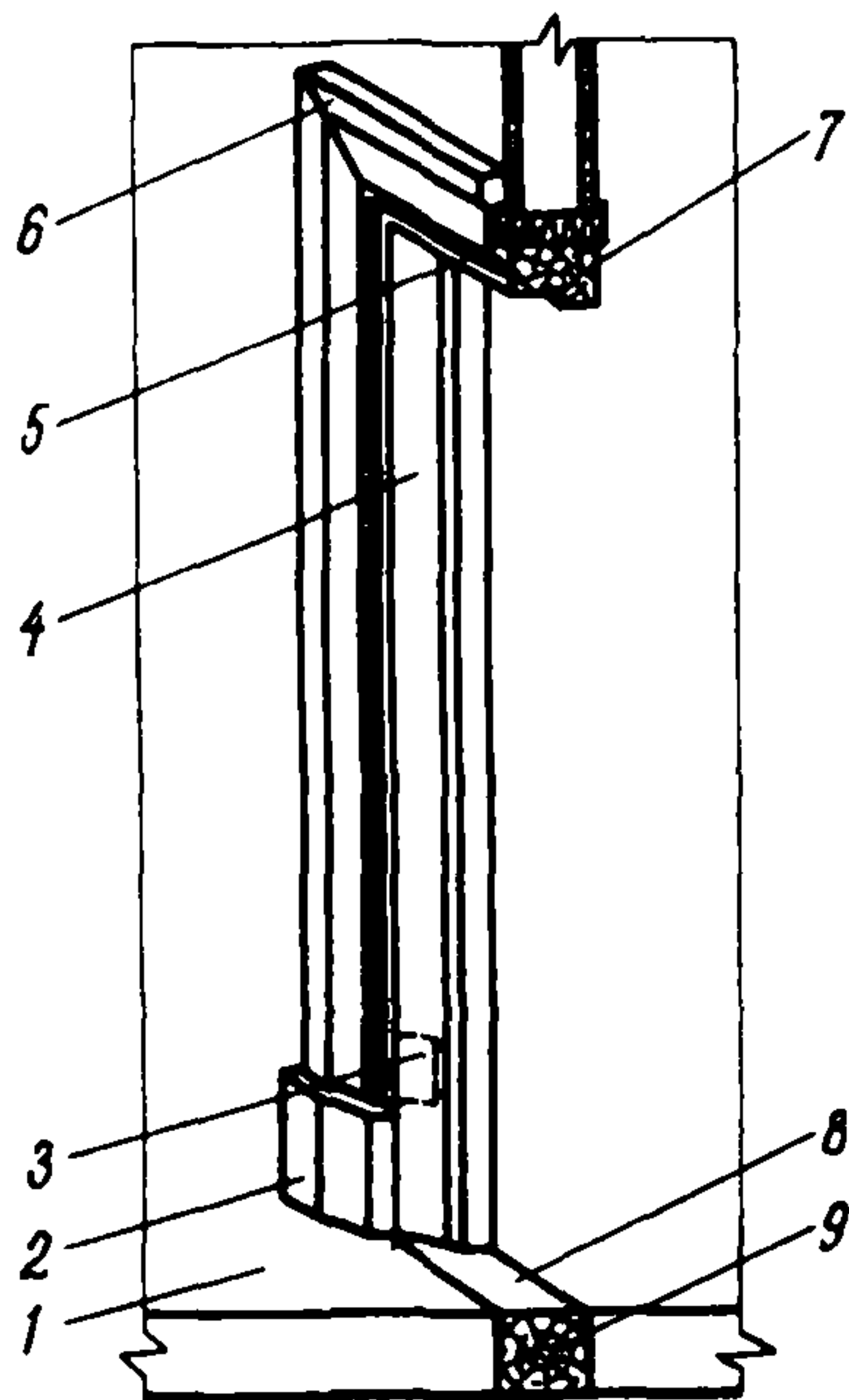
Рис. 15. Дверная коробка с установочными элементами:
