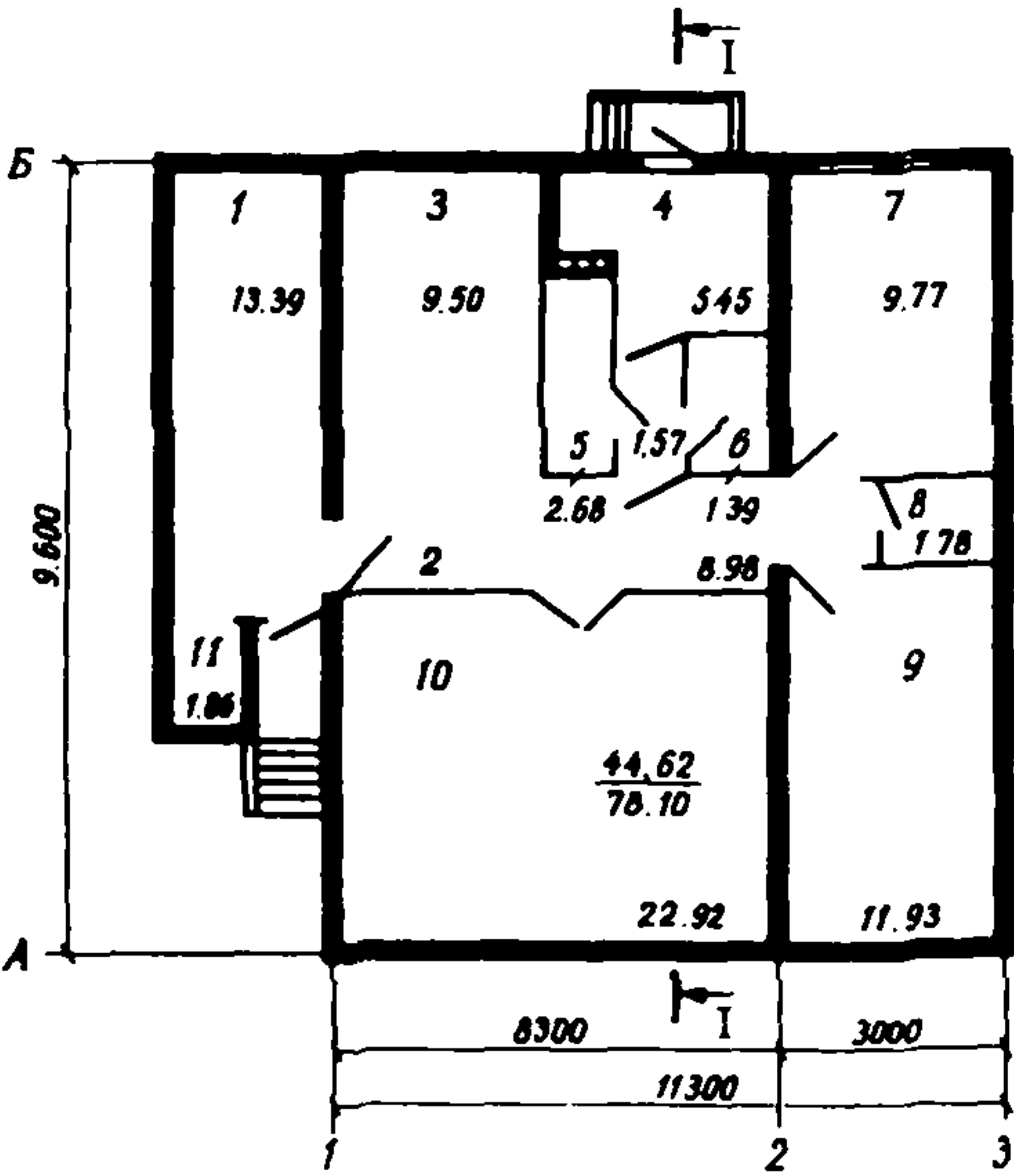
Рис. 2. План одноэтажного жилого дома: 1 - веранда; 2 - передняя; 3 - кухня; 4 - хозяйственная комната; 5 - ванная; 6 - туалет; 7, 9 - спальни; 8 - встроенный шкаф; 10 - общая комната; 11 - кладовая
