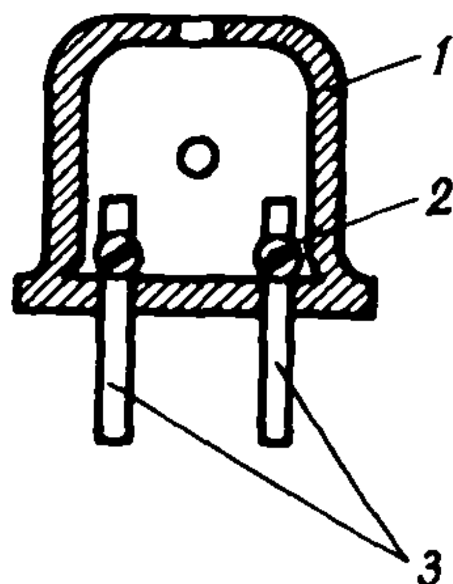
Рис. 28. Штепсельная вилка: 1 - корпус; 2 - контактные зажимы; 3 - контактные штифты
