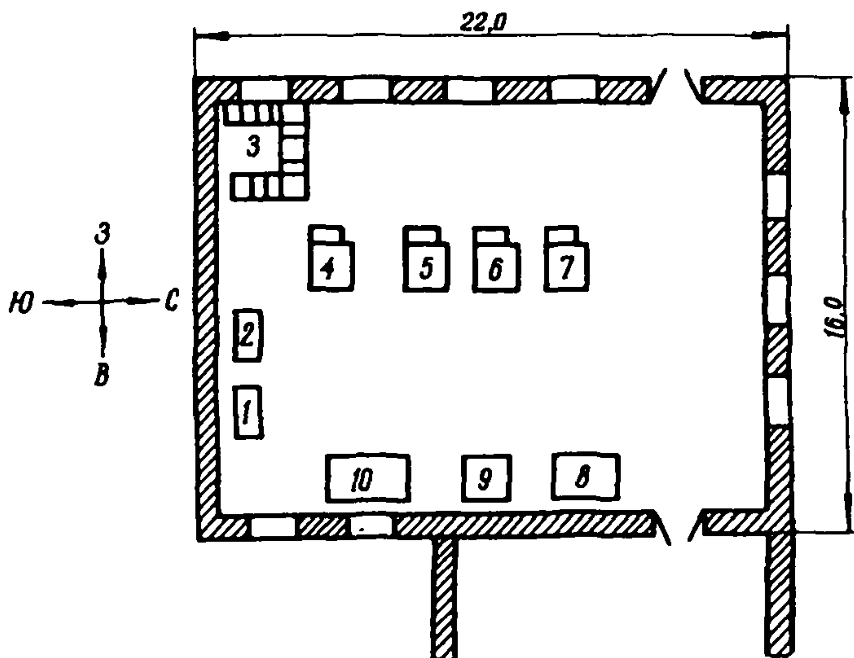
Рис. 5. План места пожара (цех переработки вспененного полиэтилена): 1, 2 - столы рабочие; 3 - металлические шкафчики для спецдежды; 4-7 - прессы гидравлические ДБ-2434; 8 - станок для вертикальной резки полиэтиленовой плиты; 9 - механический пресс; 10 - двохвальная машина
