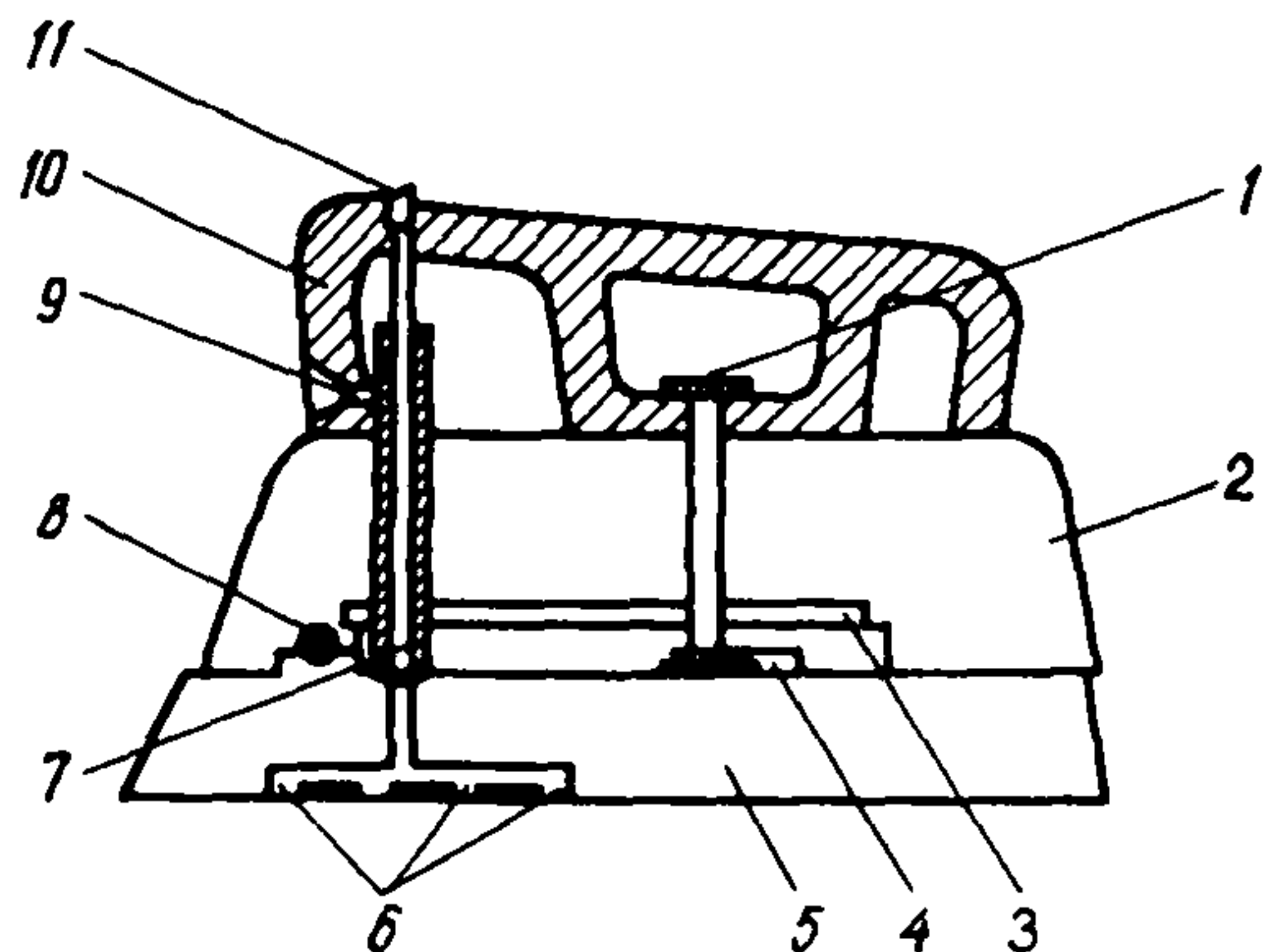
Рис. 40. Электроутюг: 1 - лимб терморегулятора; 2 - корпус; 3 - бачок; 4 - биметаллический терморегулятор; 5 - по- дошва; 6 - лабиринтные каналы в подошве; 7 - клапан; 8 - ТЭН; 9 - отверстие для заливки воды; 10 - ручки; 11 - кнопка отпаривателя
