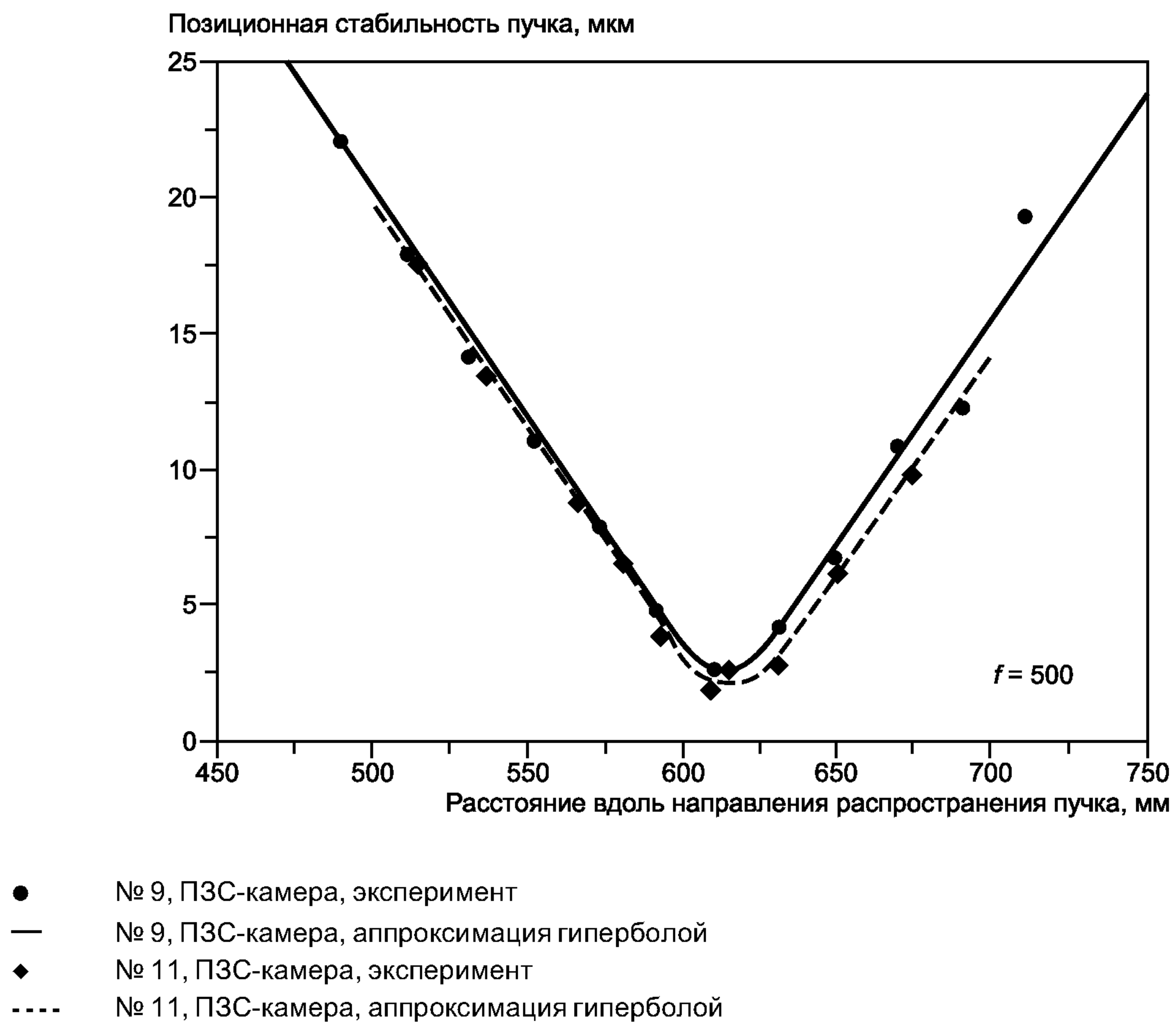
Рисунок А.1 — Позиционная стабильность Nd:YAG лазера с модулированной добротностью, измеренная двумя ПЗС-камерами
