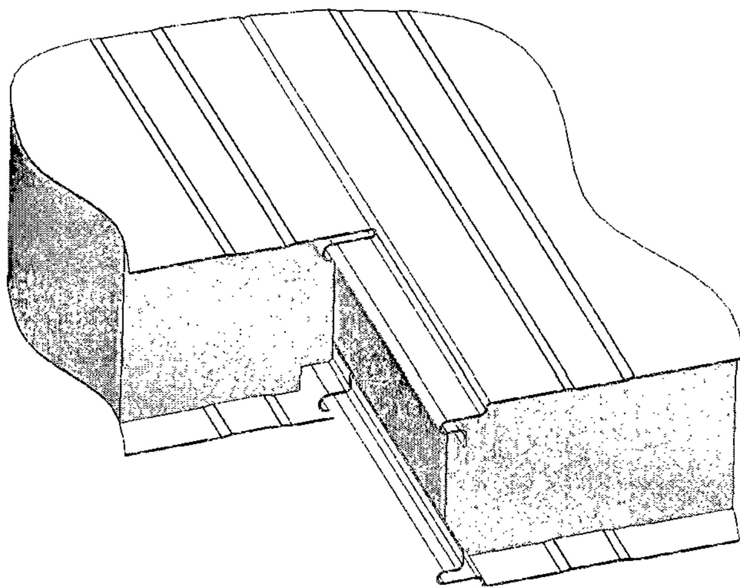
Стыковое соединение панелей ПСТМ
