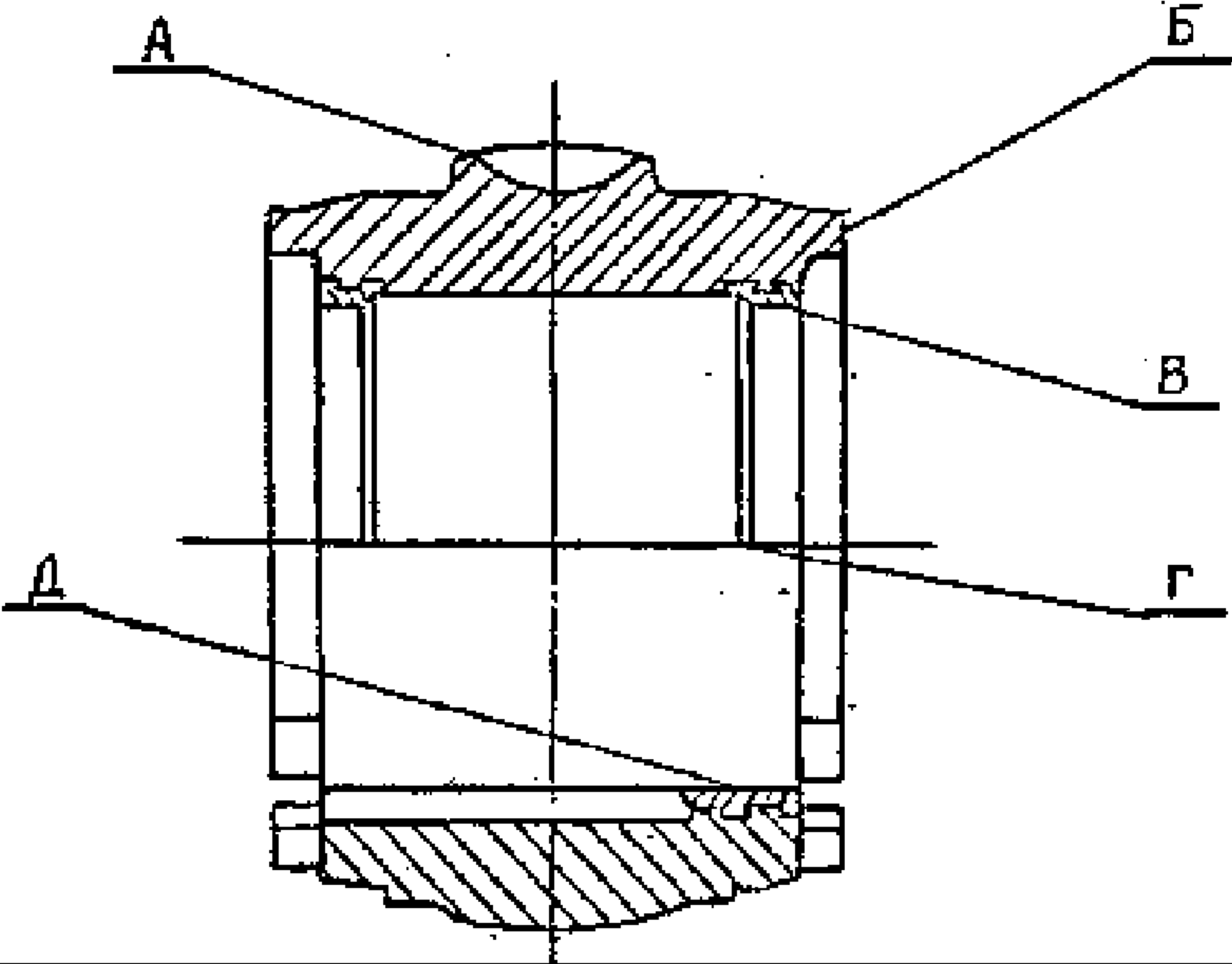
Карта дефектации и ремонта 10 Вкладыш подшипника поз. 2 рисунок 7-4 Количество на изделие, шт. – 1
