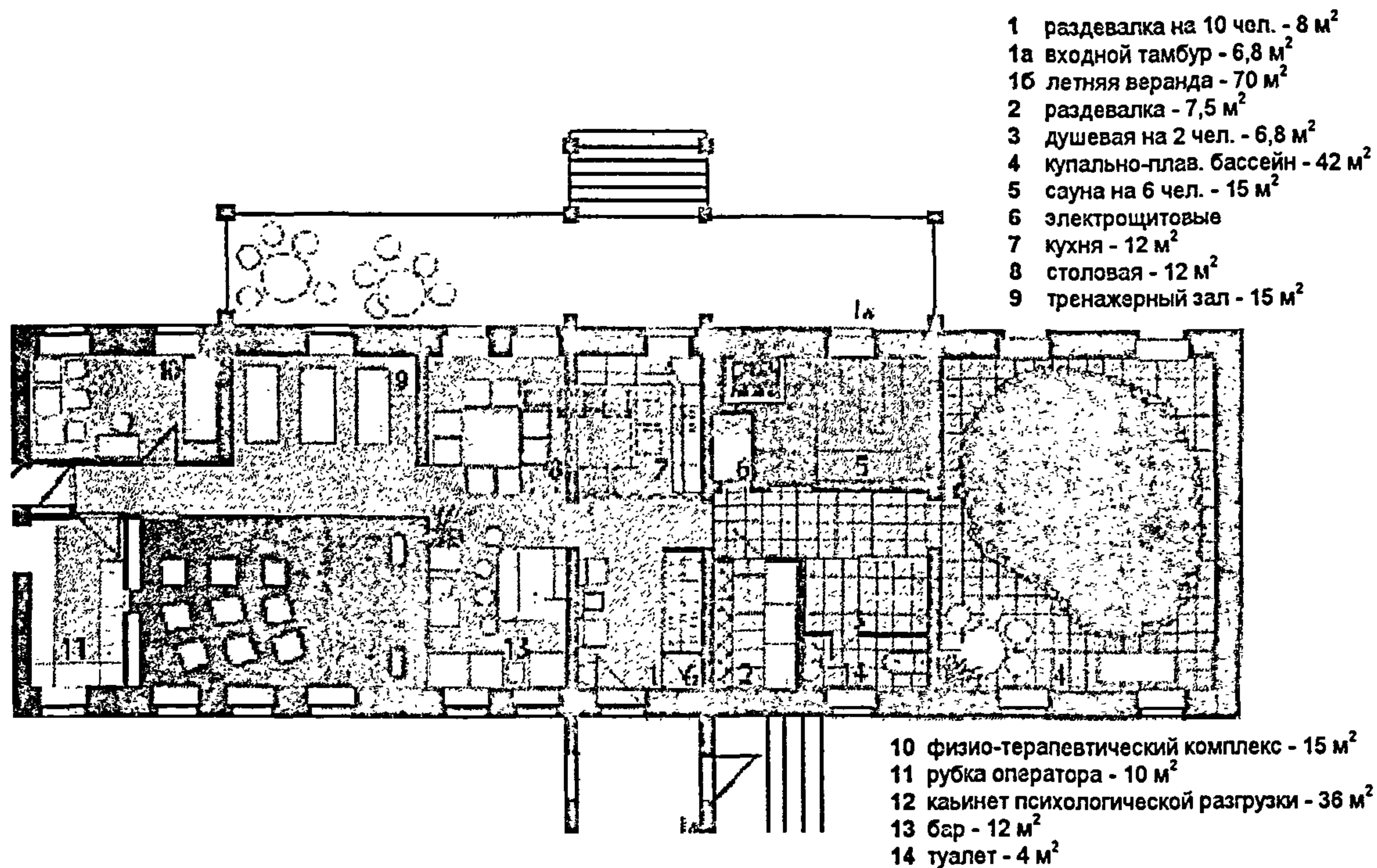
Рис. 3. Планировочное решение стационарного медико-психологического восстановительного комплекса
