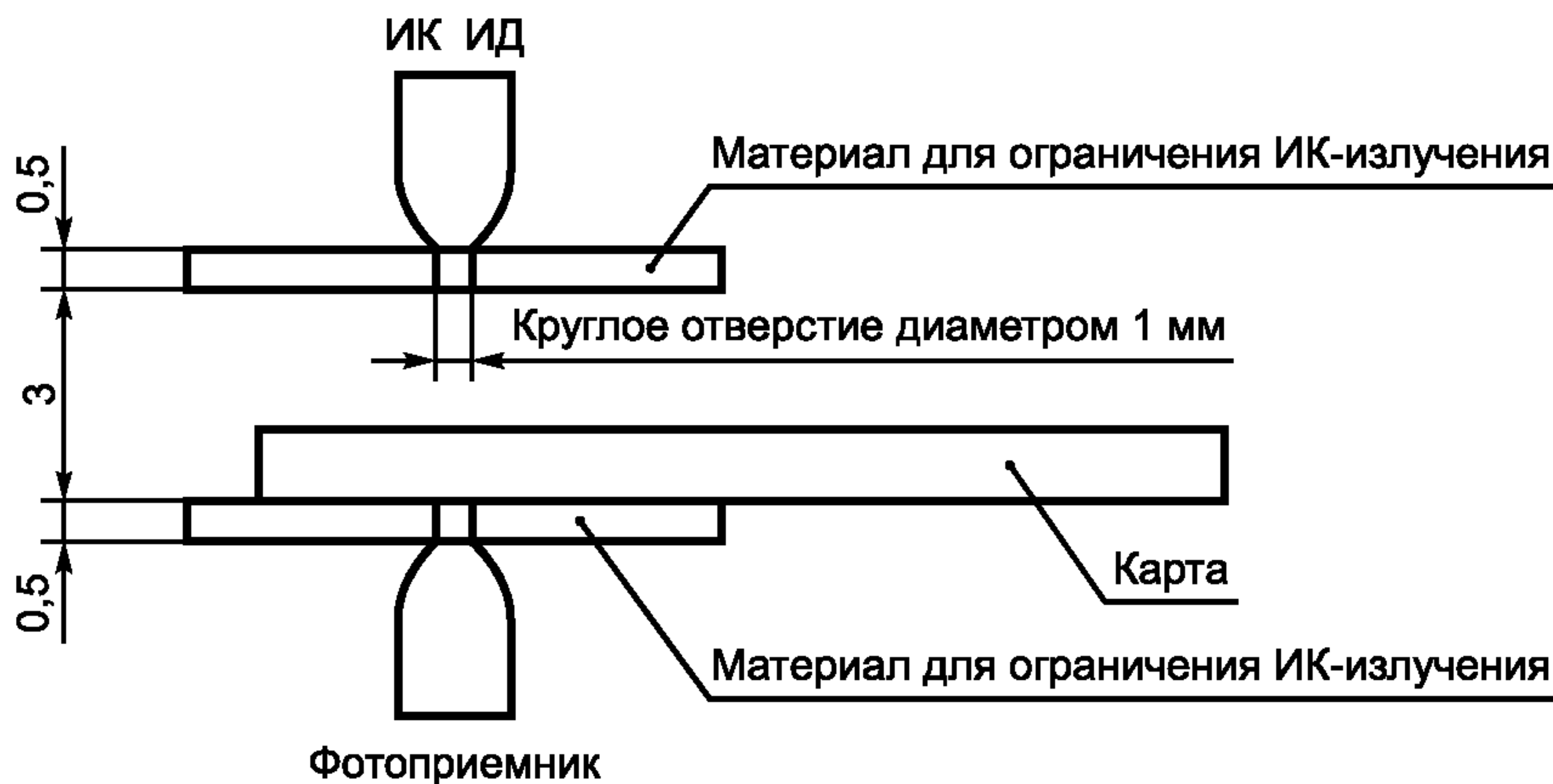
Рисунок 14 — Правильное расположение ИК ИД и фотоприемника
