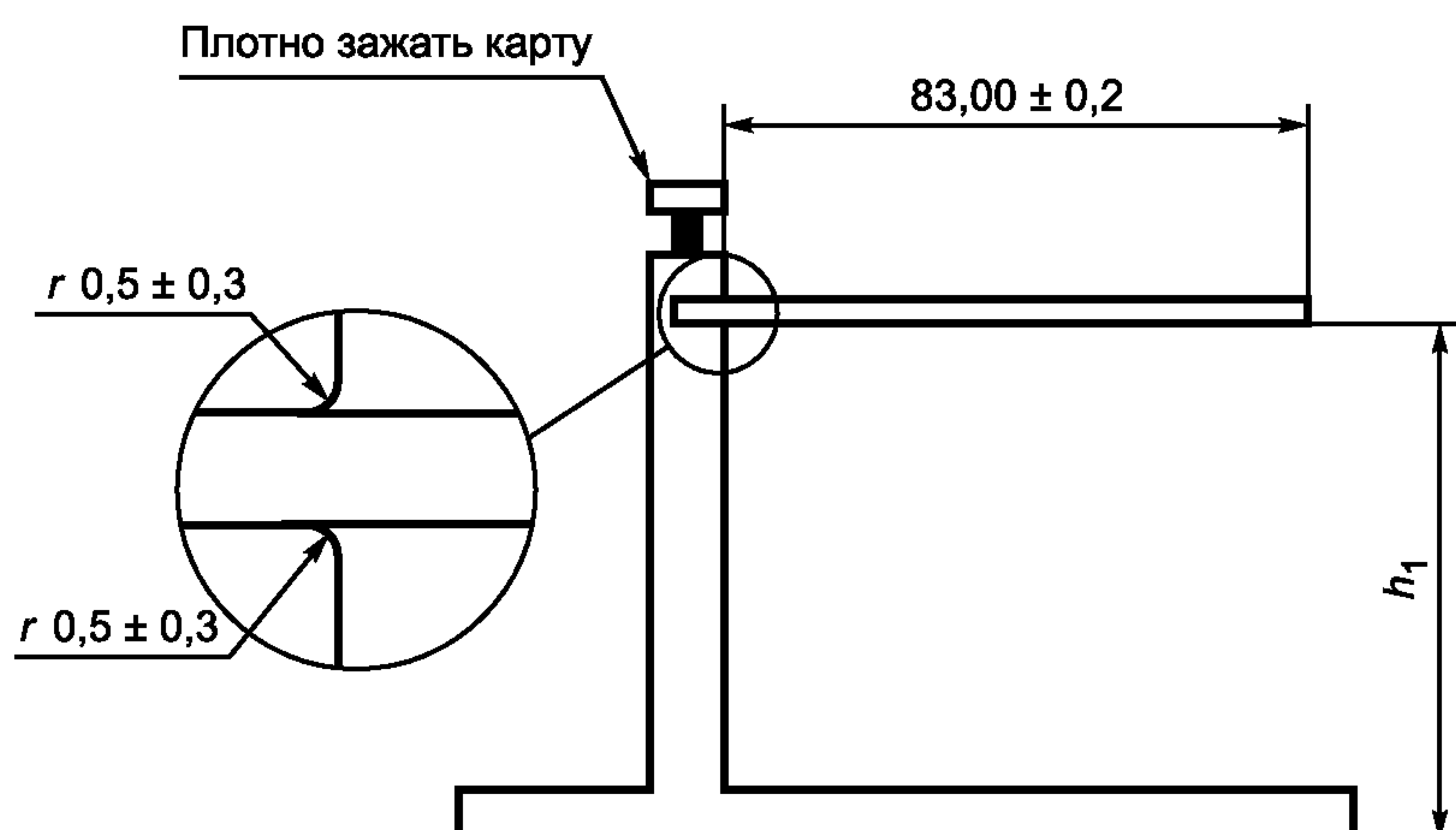
Рисунок 7 — Карта в зажимном устройстве до приложения нагрузки
