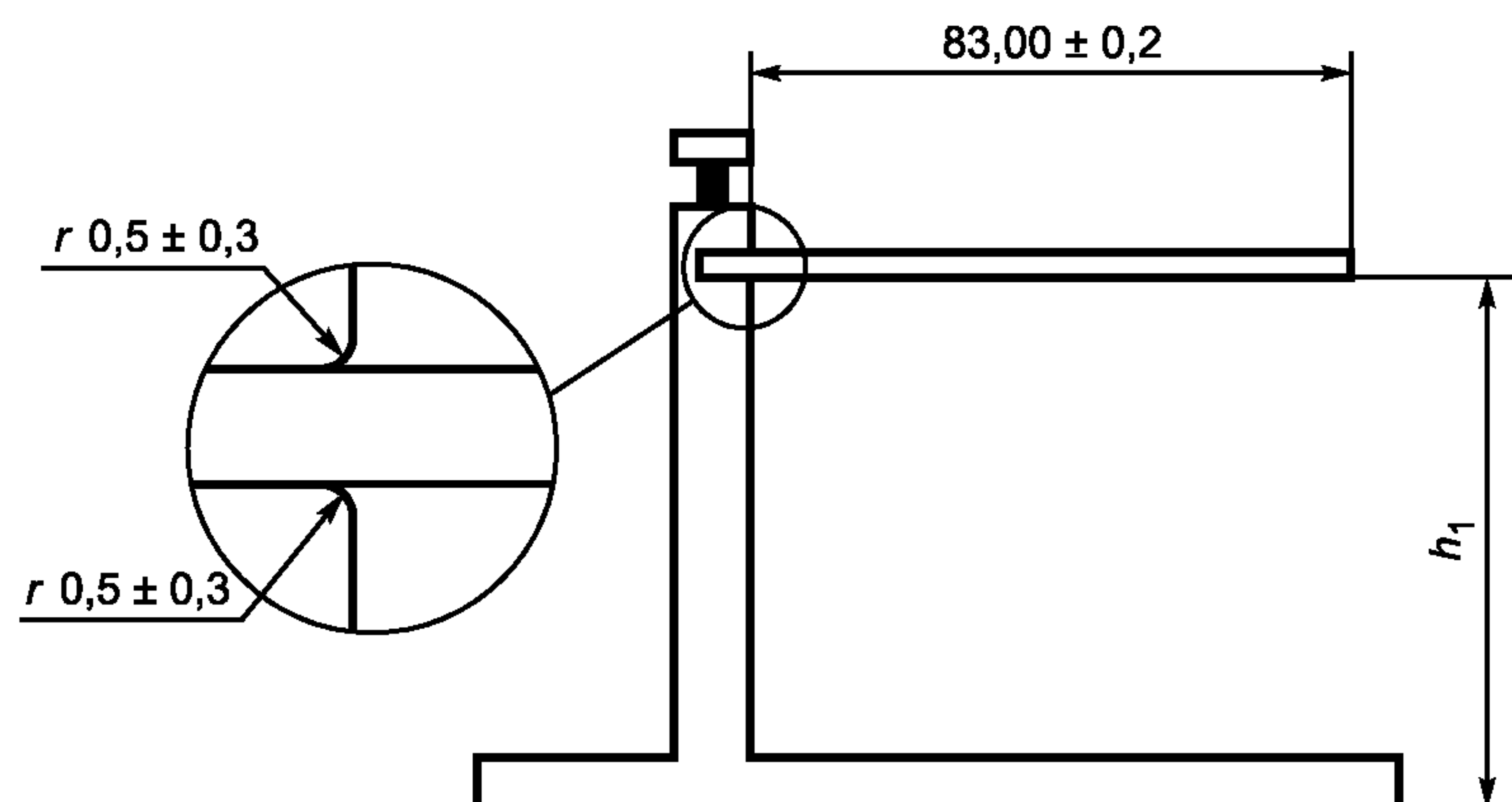
Рисунок 16 — Карта в зажимном устройстве до воздействия температуры
