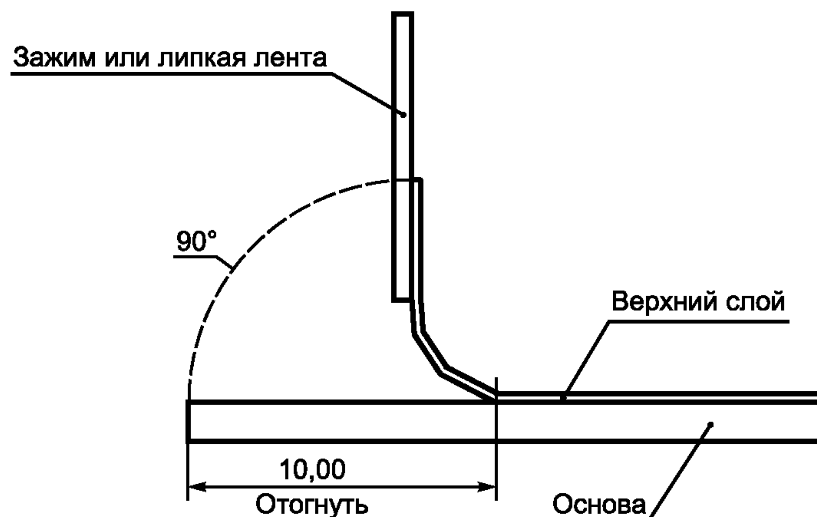
Рисунок 4 — Подготовка образца к испытанию
