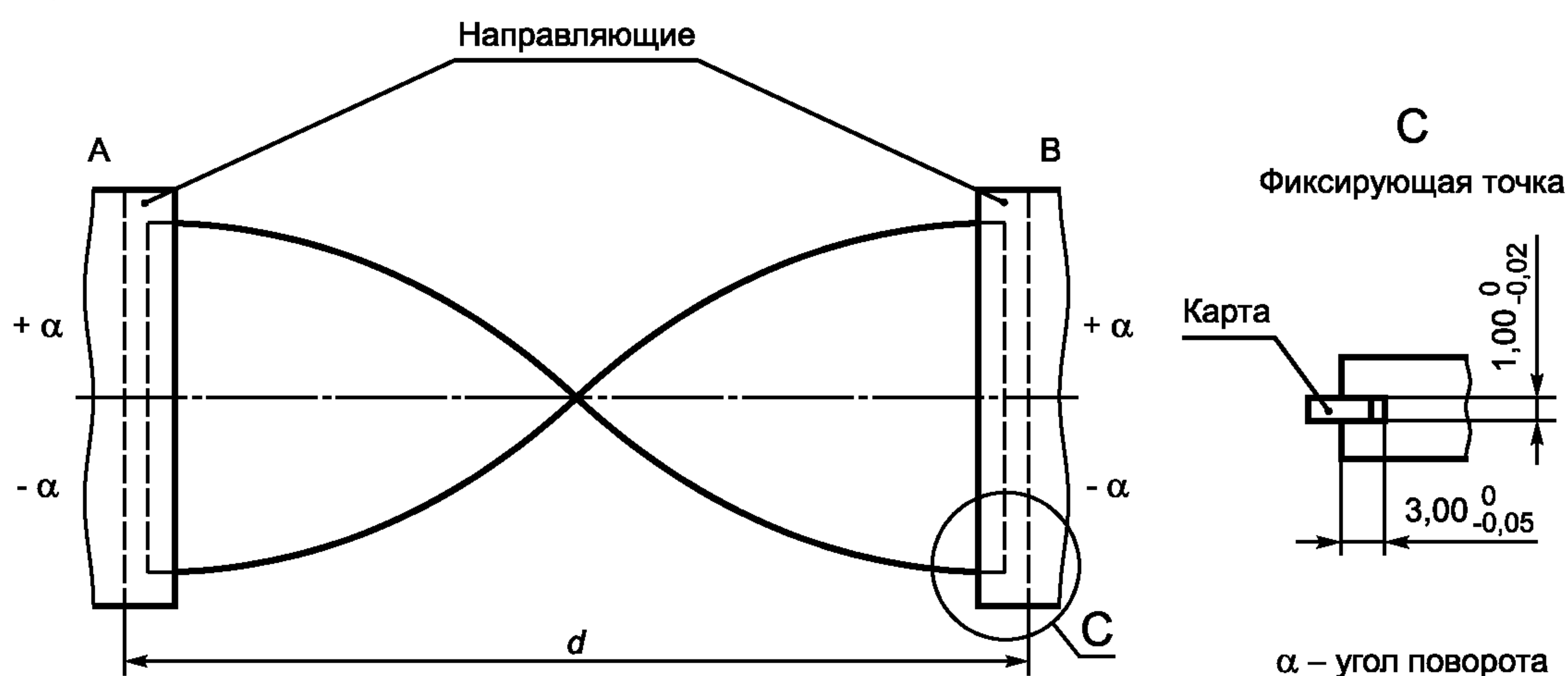
Рисунок 12 — Машина для испытания на скручивание
