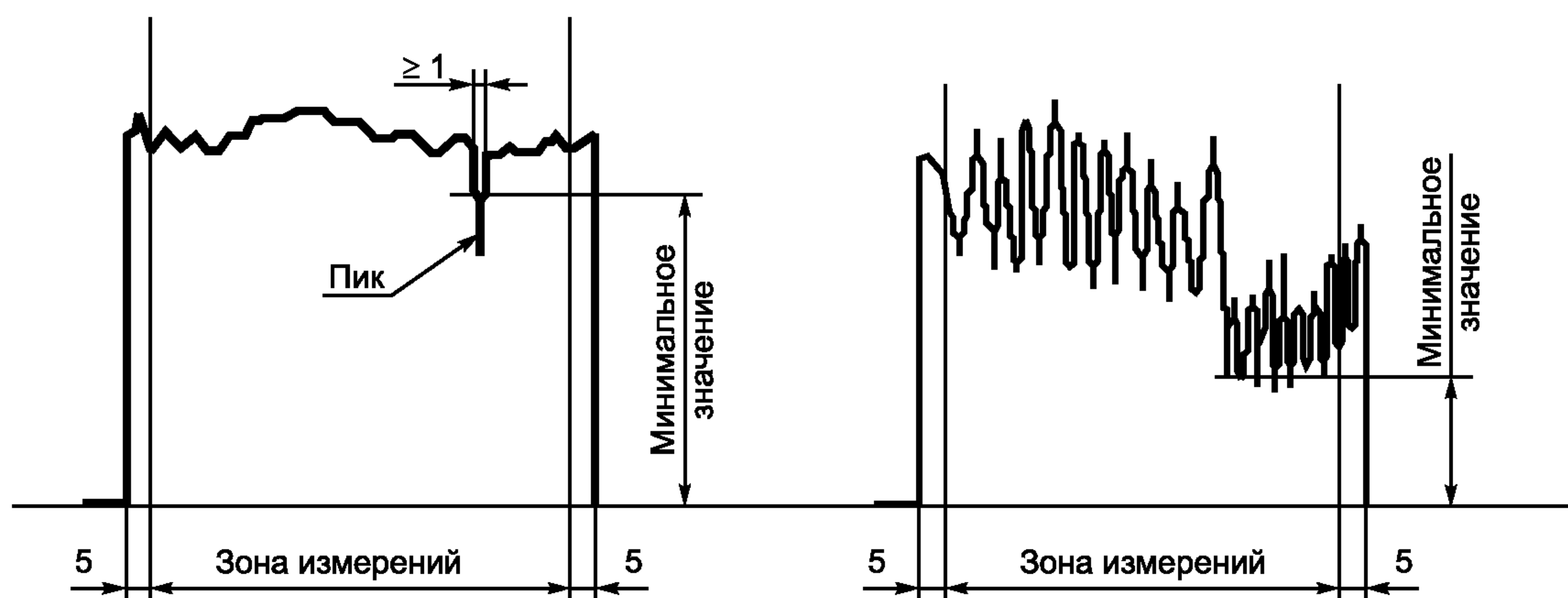
Рисунок 6 — Примеры диаграмм прочности сцепления
