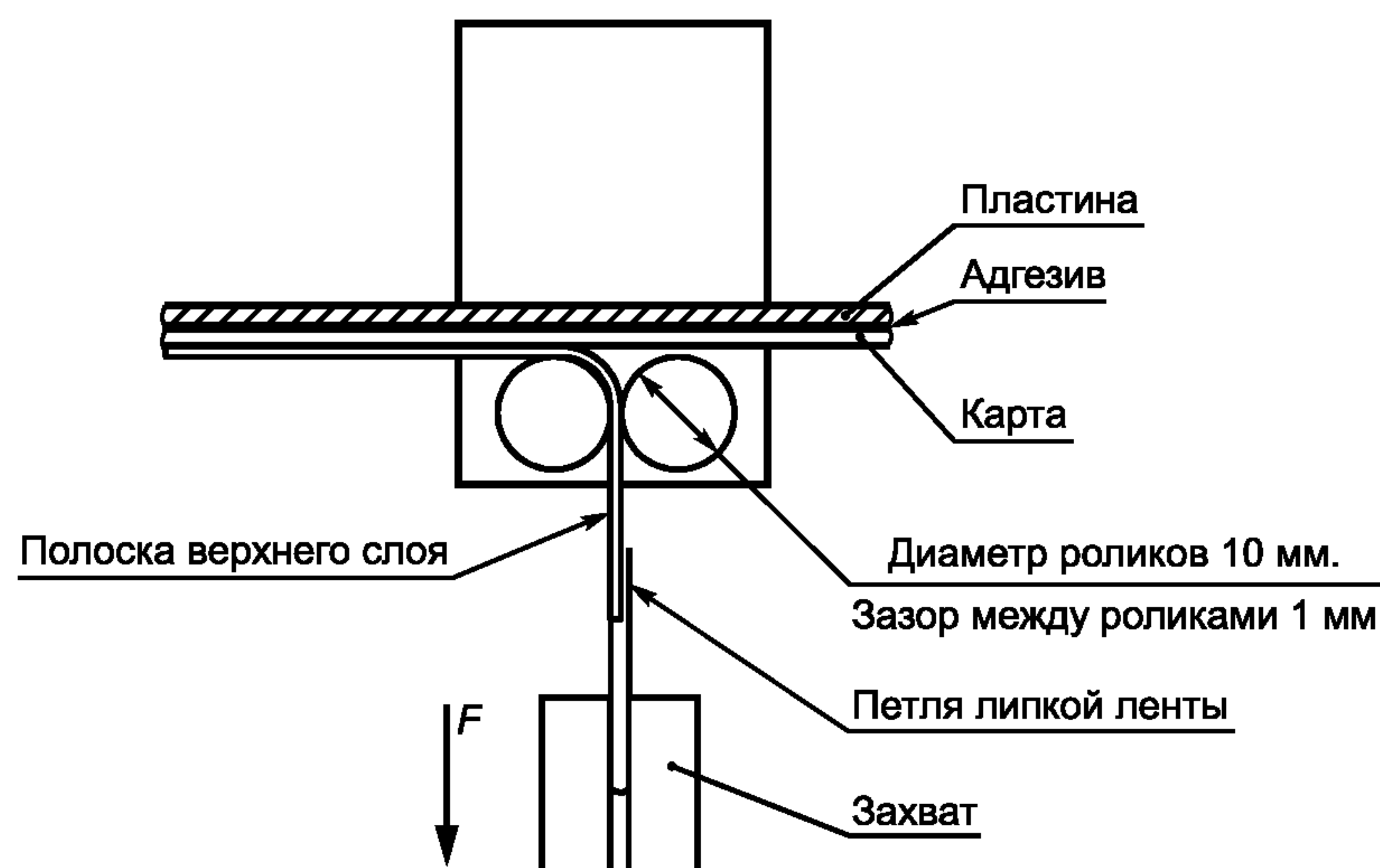
Рисунок 5 — Схема установки карты в разрывной машине
