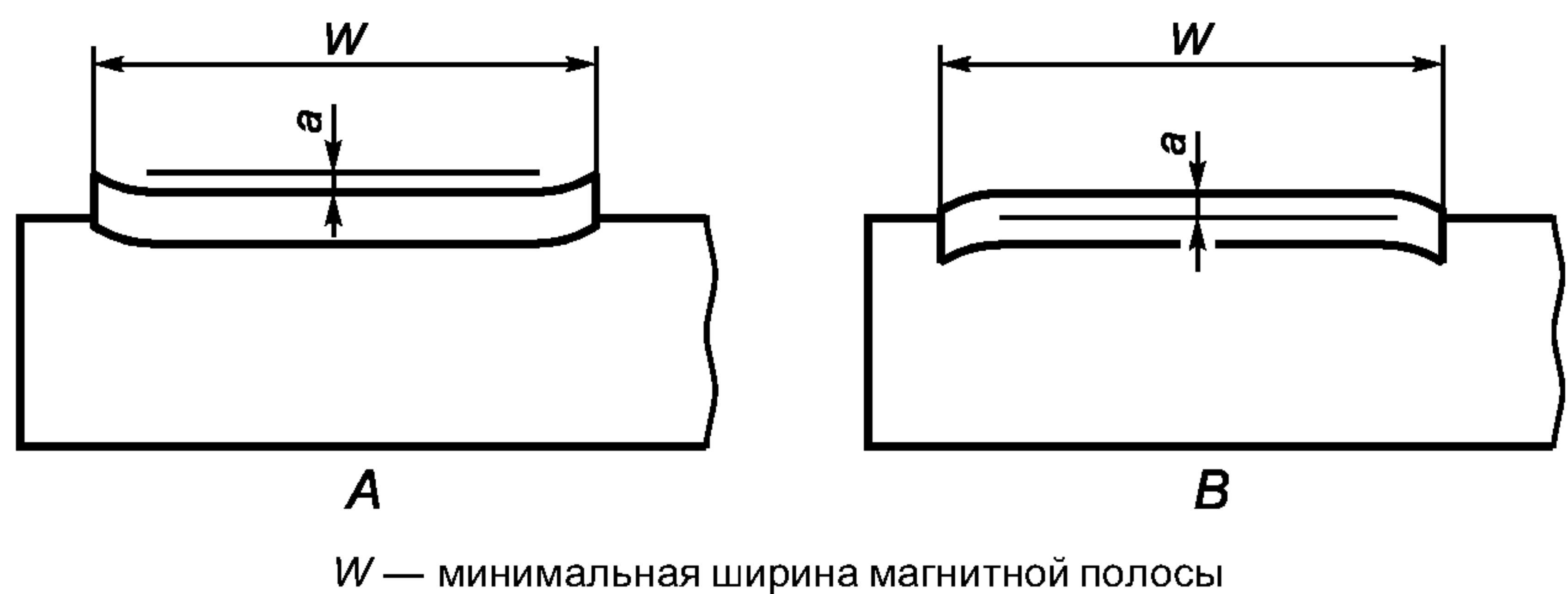
Рисунок 3 — Профиль поверхности
