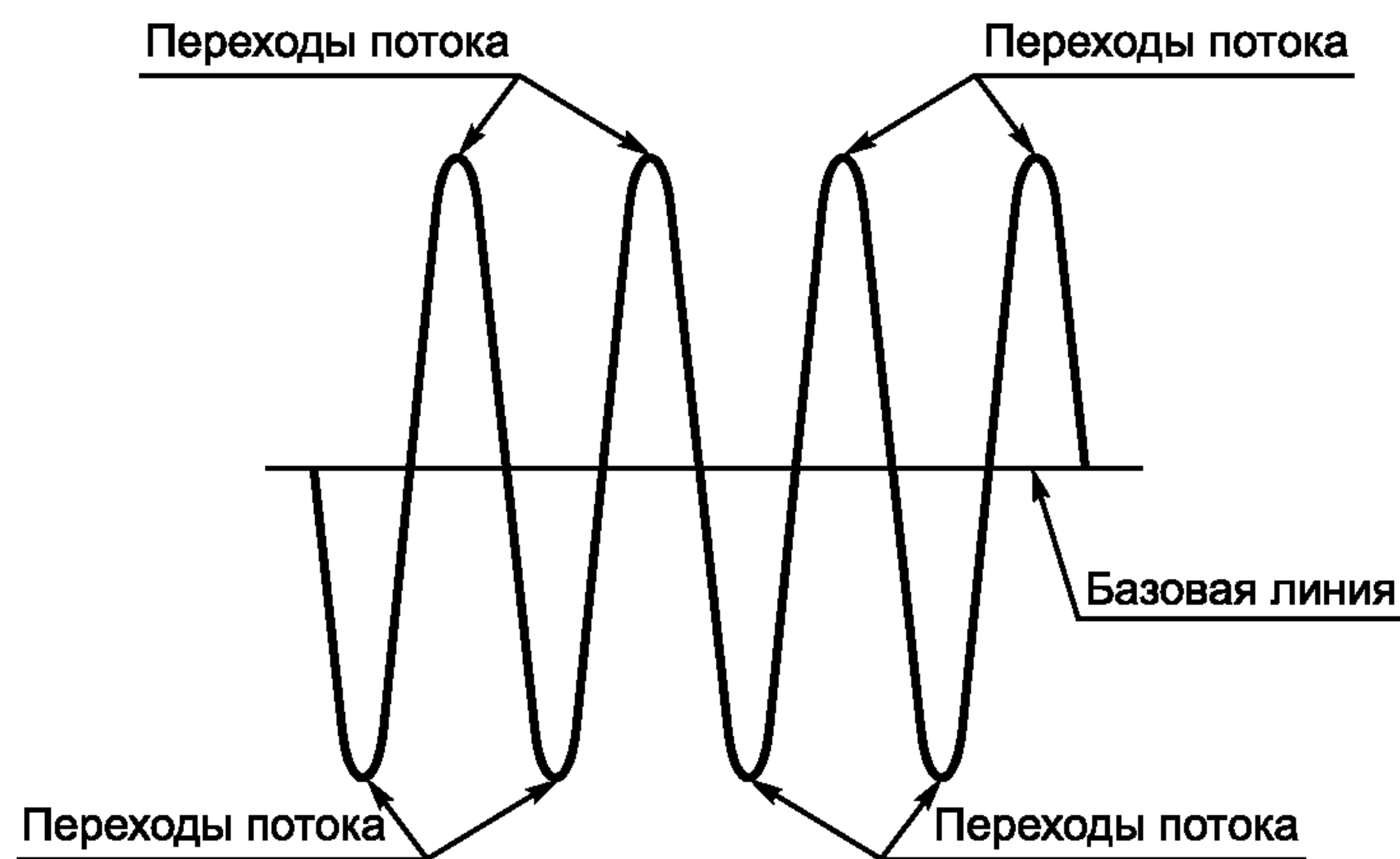
Рисунок 7 — Пример формы сигнала
