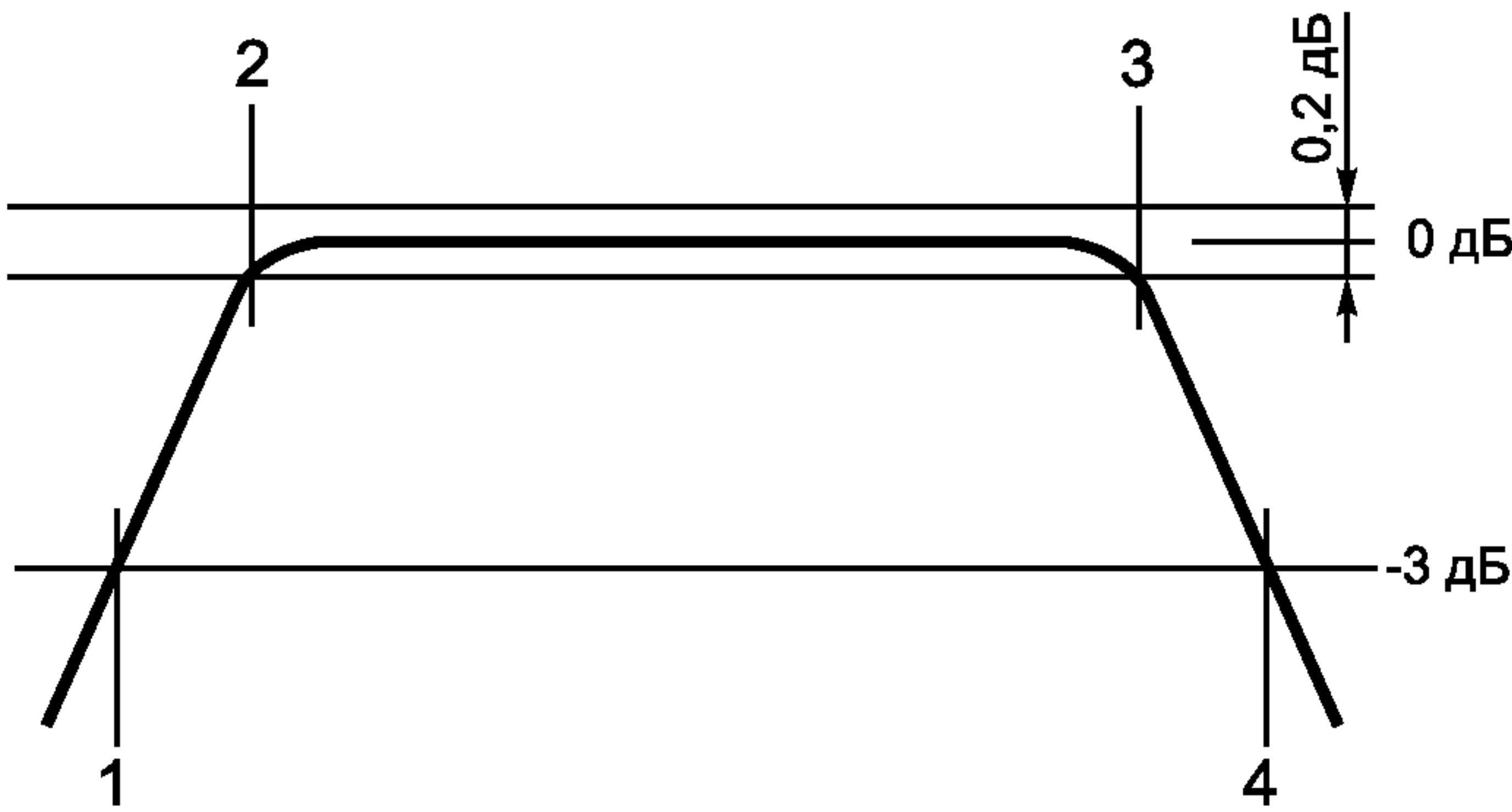
Рисунок В.1 — Характеристики полосового фильтра
