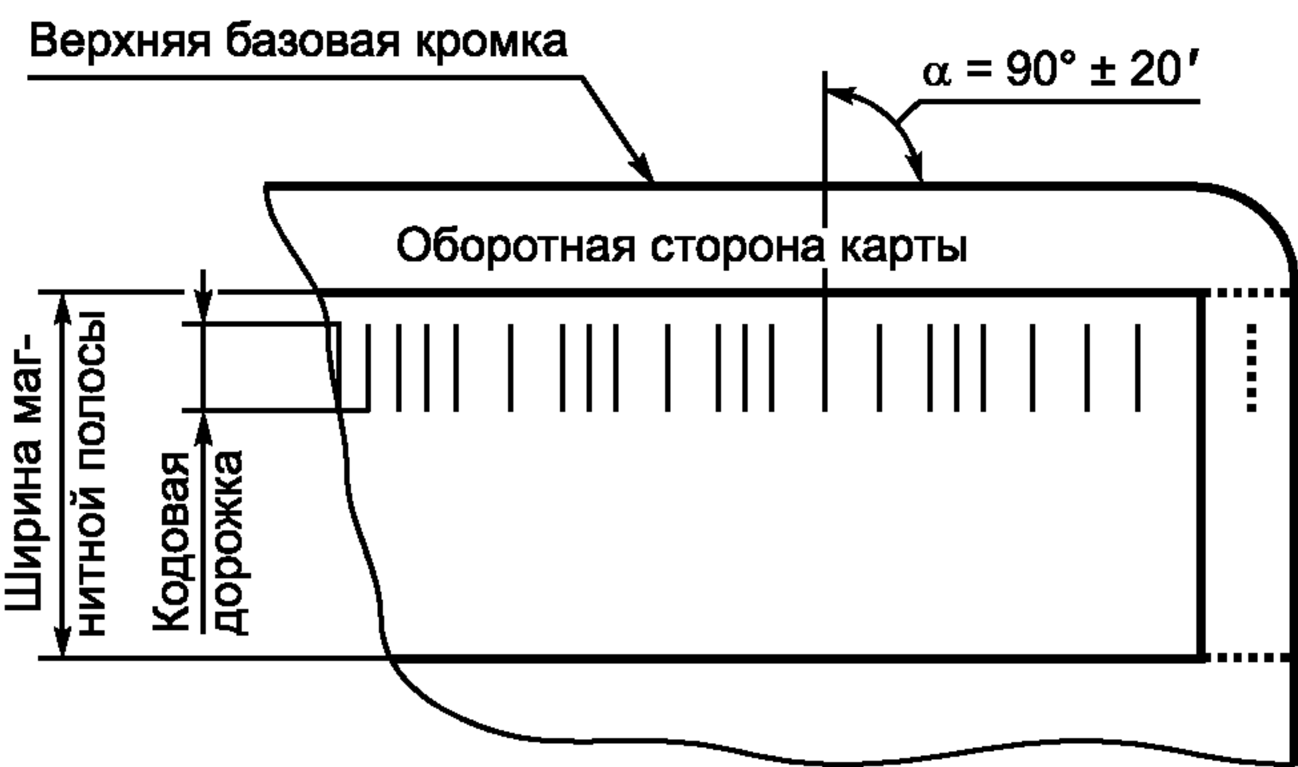
Рисунок 9 — Угол записи
