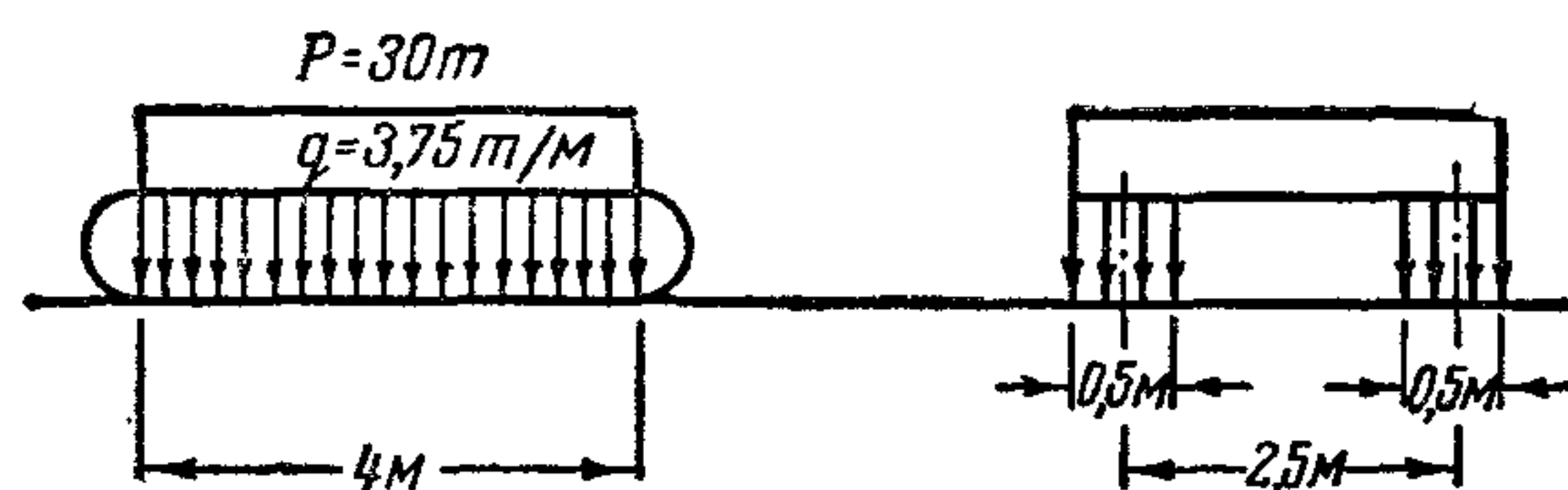
Рис. 5. Нормативная гусеничная нагрузка по схеме НГ-30
