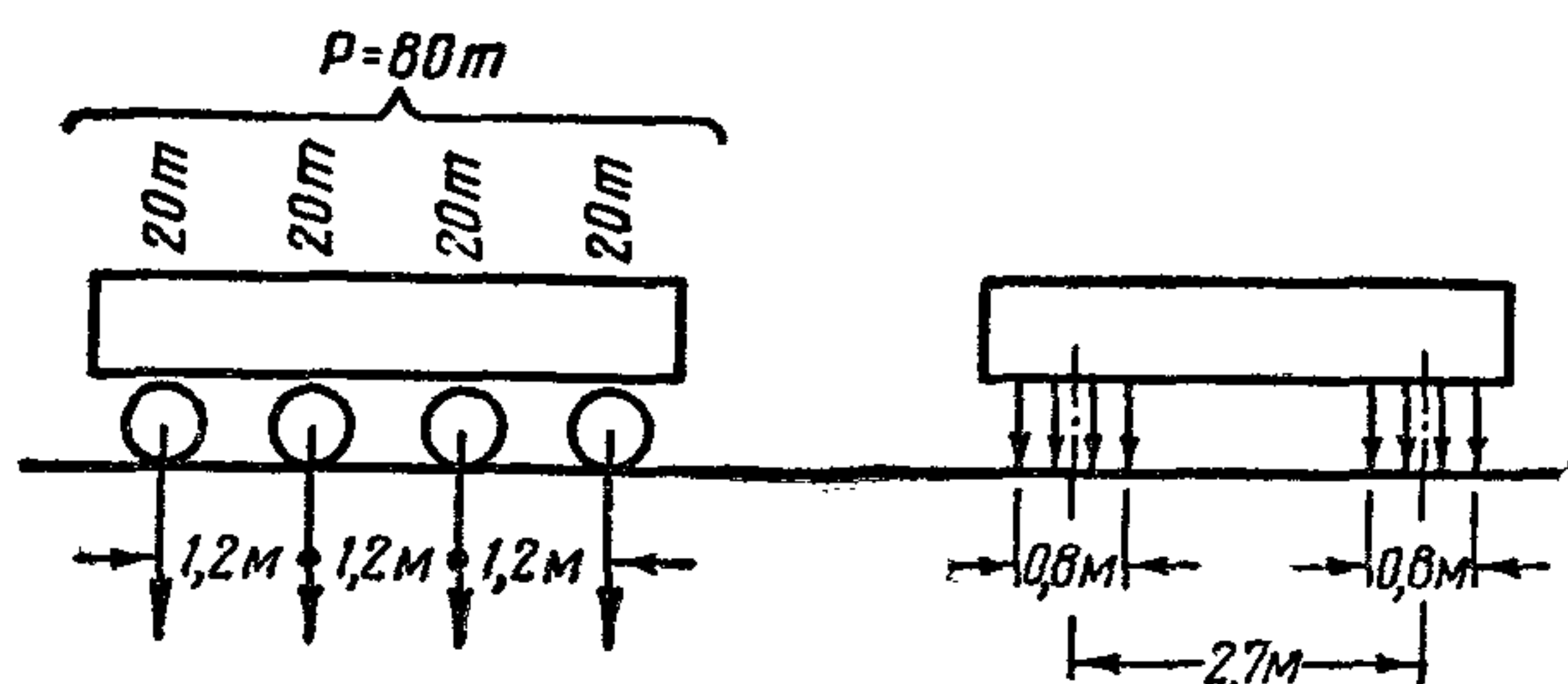
Рис. 3. Нормативная колесная нагрузка по схеме НК-80
