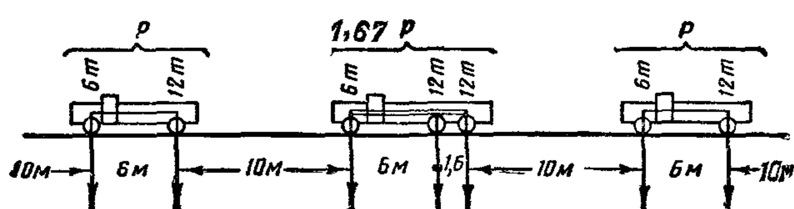
Рис. 1. Нормативная автомобильная нагрузка по схеме Н-18
