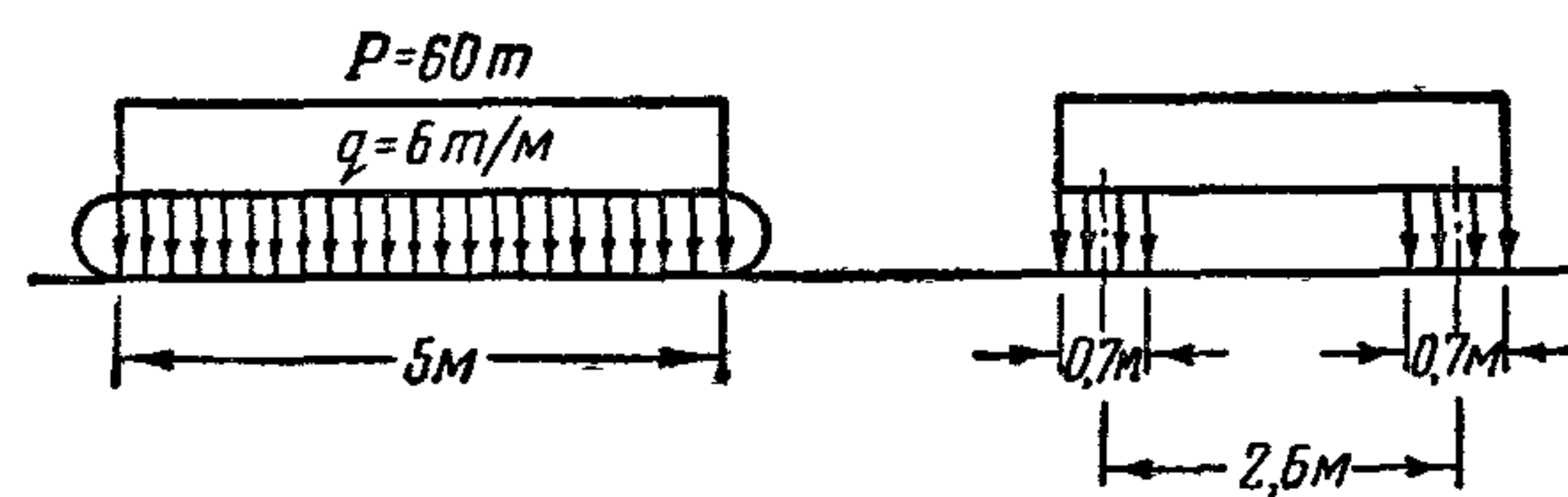
Рис. 4. Нормативная гусеничная нагрузка по схеме НГ-60
