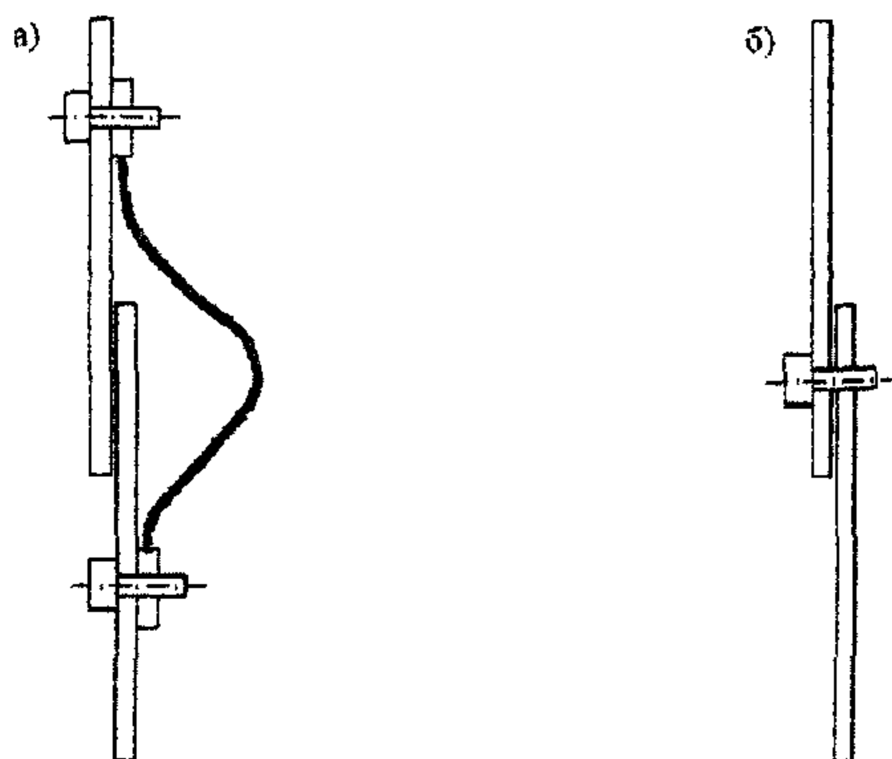
Рисунок Г.29 - Устройство соединения между металлическими сегментами фасада
