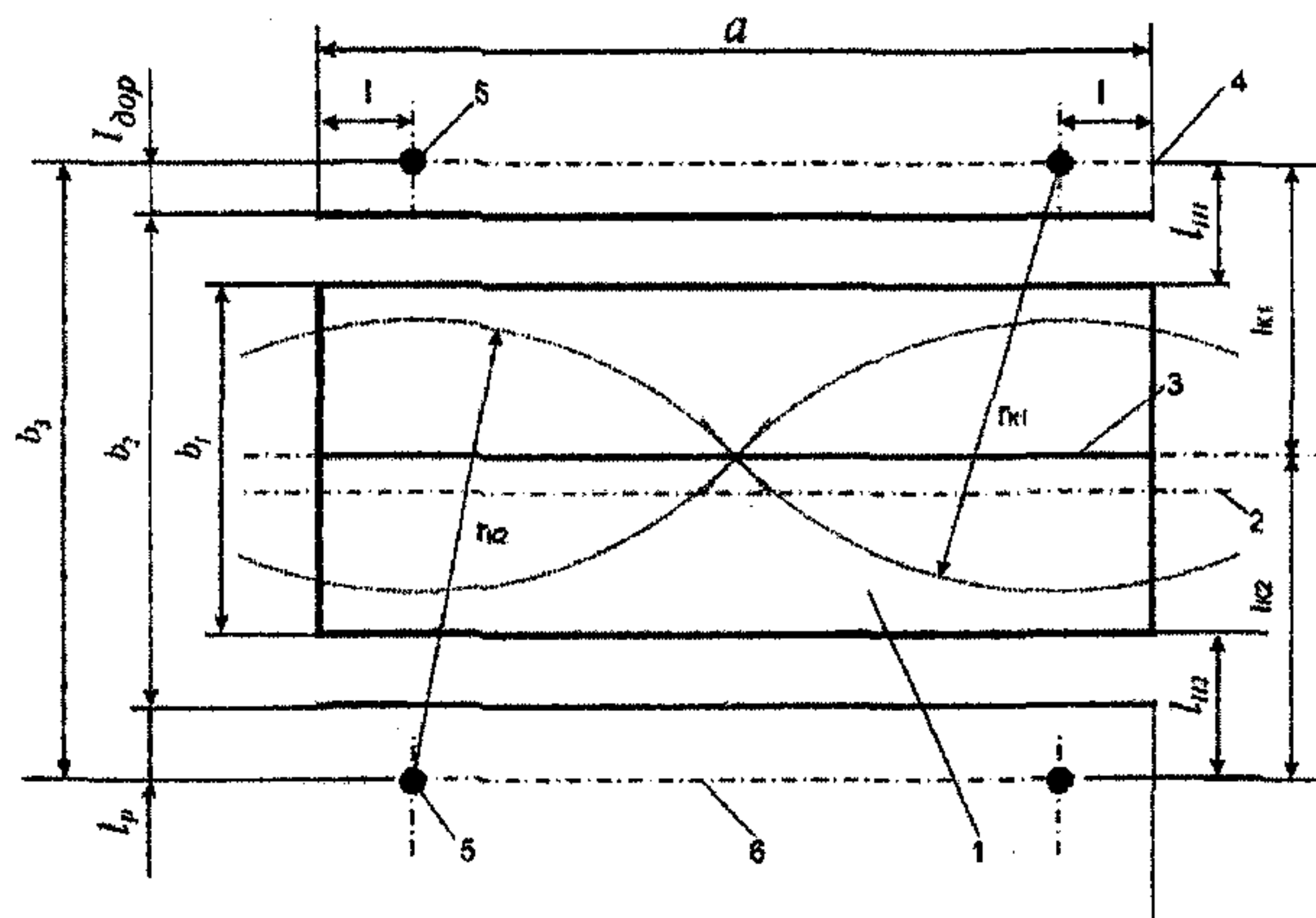
Рисунок Е.2 - Защита объекта четырьмя отдельно стоящими стержневыми молниеотводами
