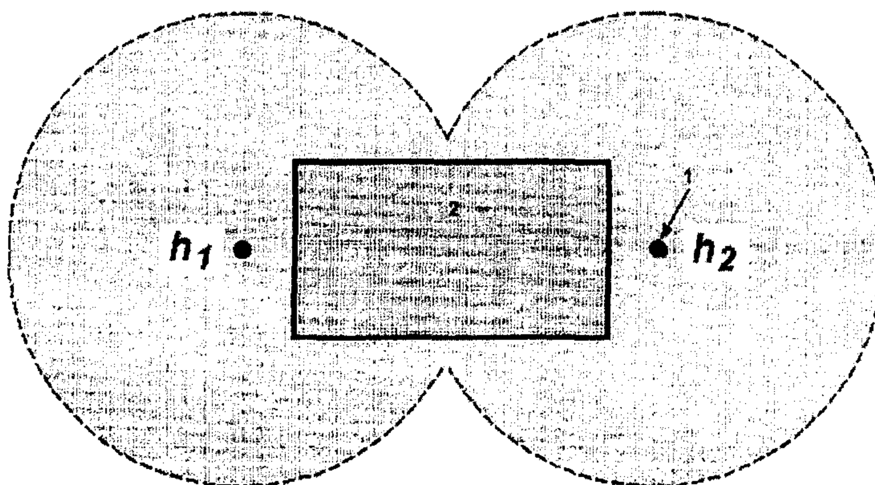
1 – молниеприемник; 2 – объект
