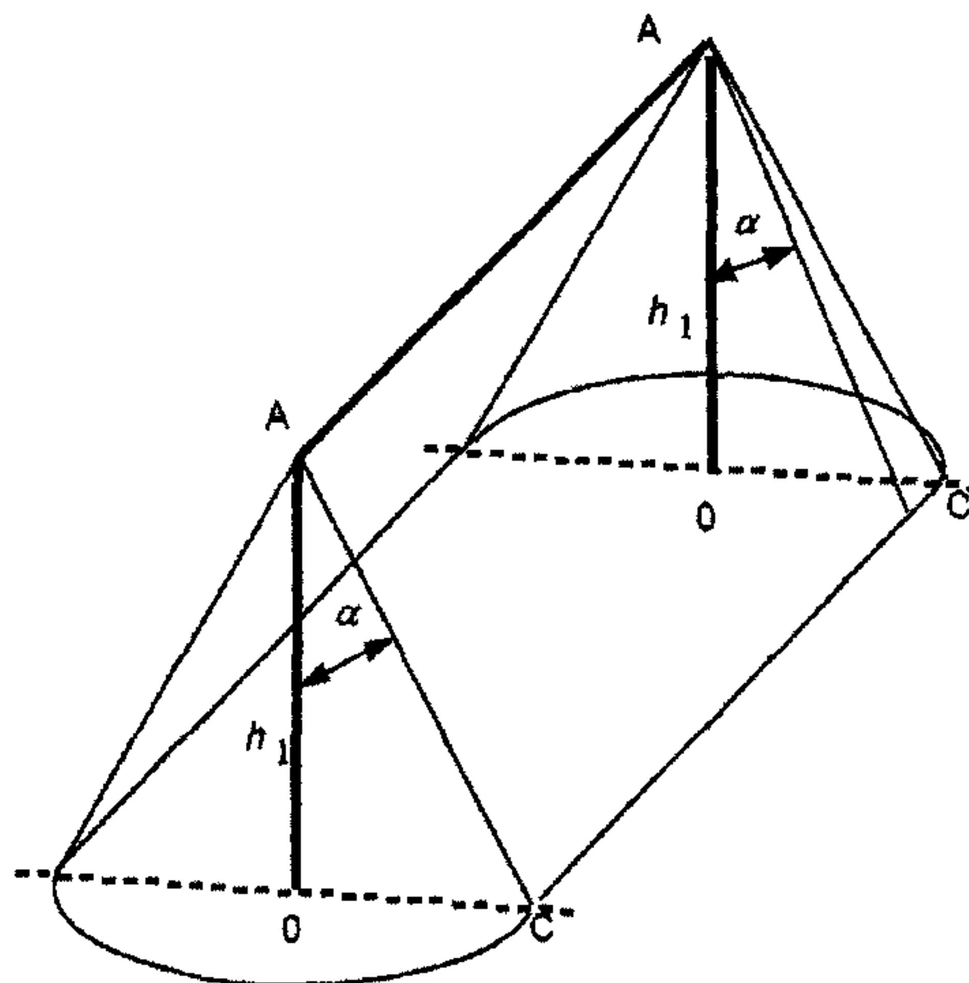
Рисунок Г.14 - Зона защиты одиночного тросового молниеотвода
