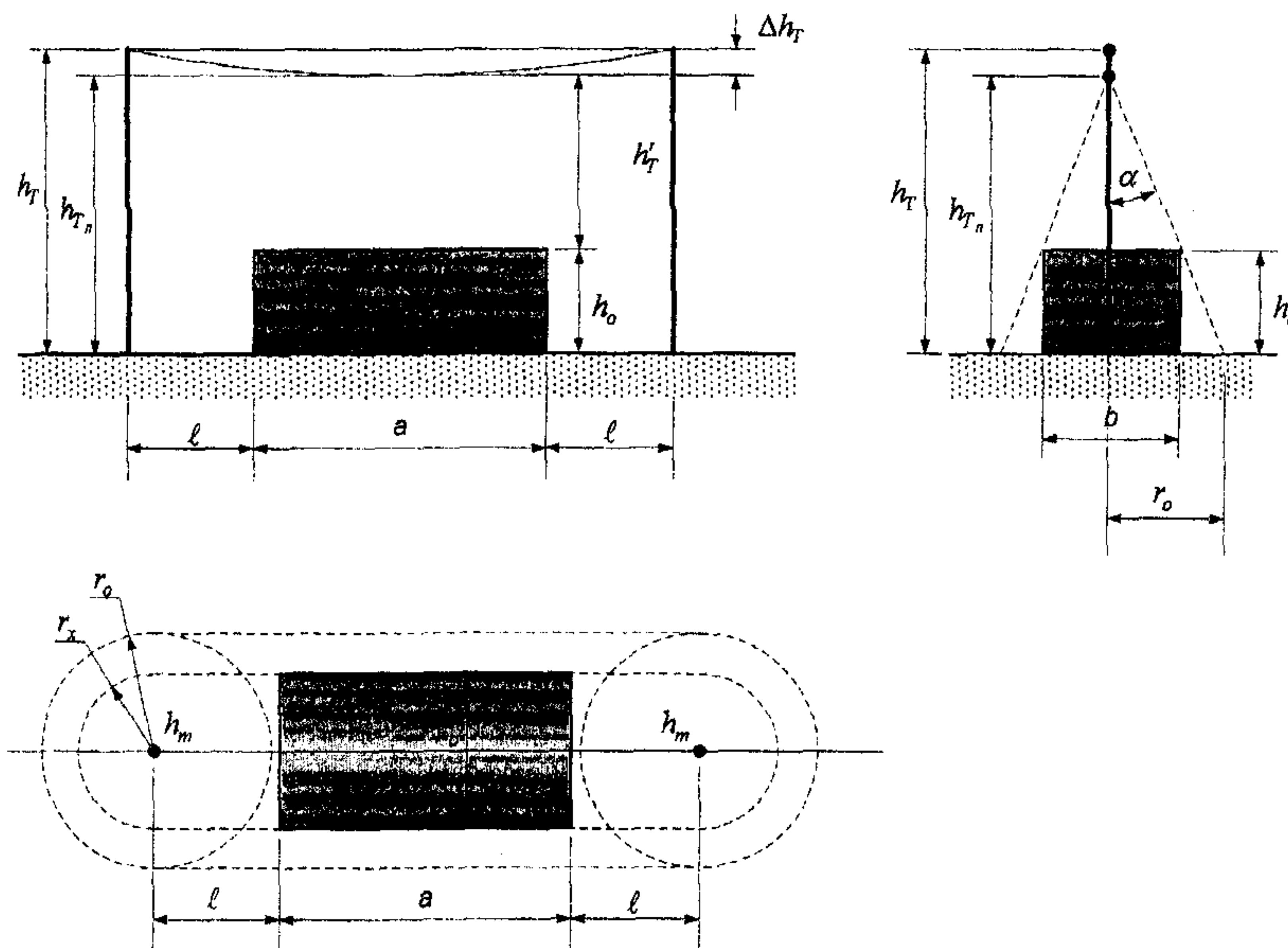
Рисунок 2.4 – Схема для расчета высоты подвеса троса
