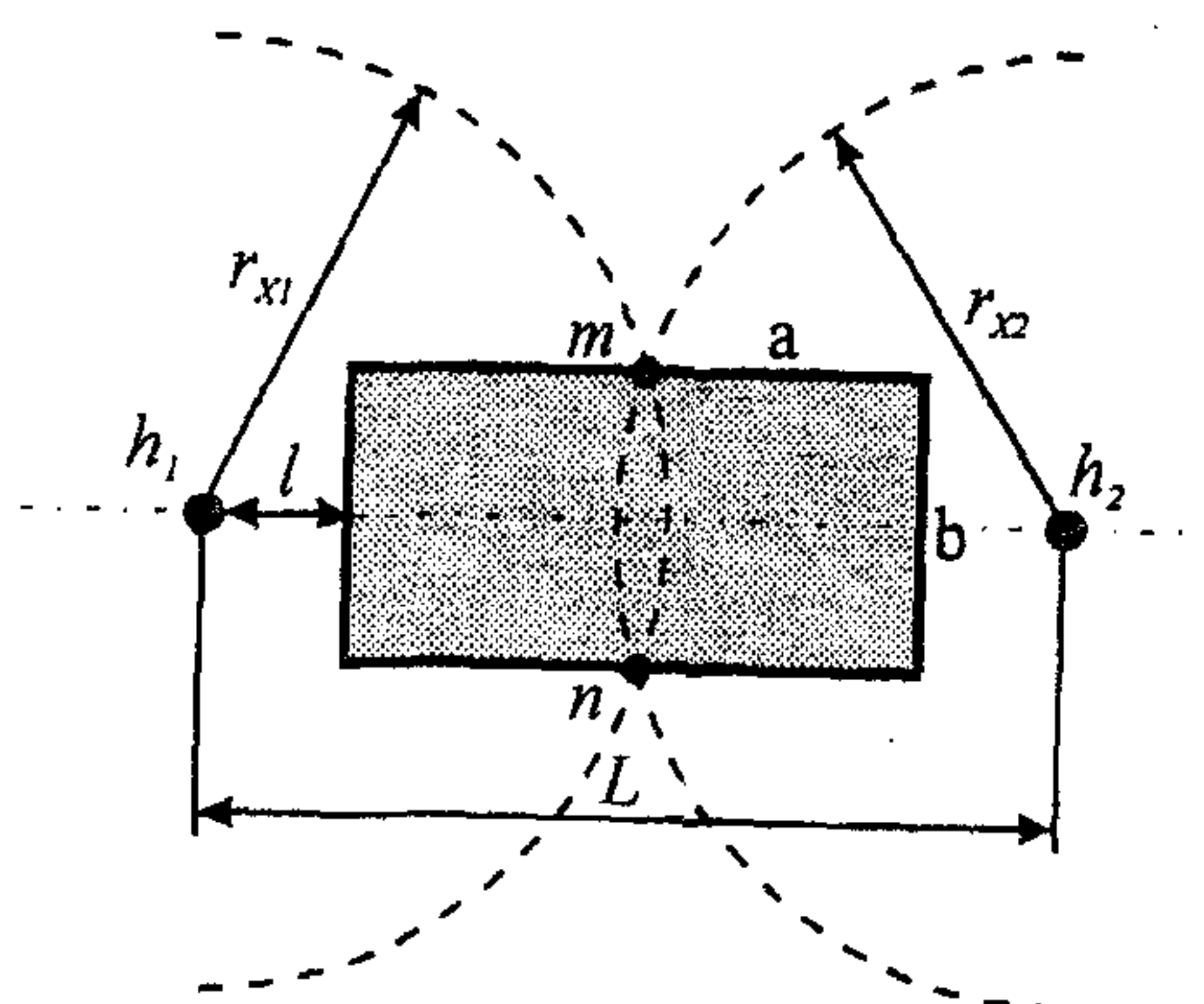
а) традиционное решение двухстержневой молниезащиты
