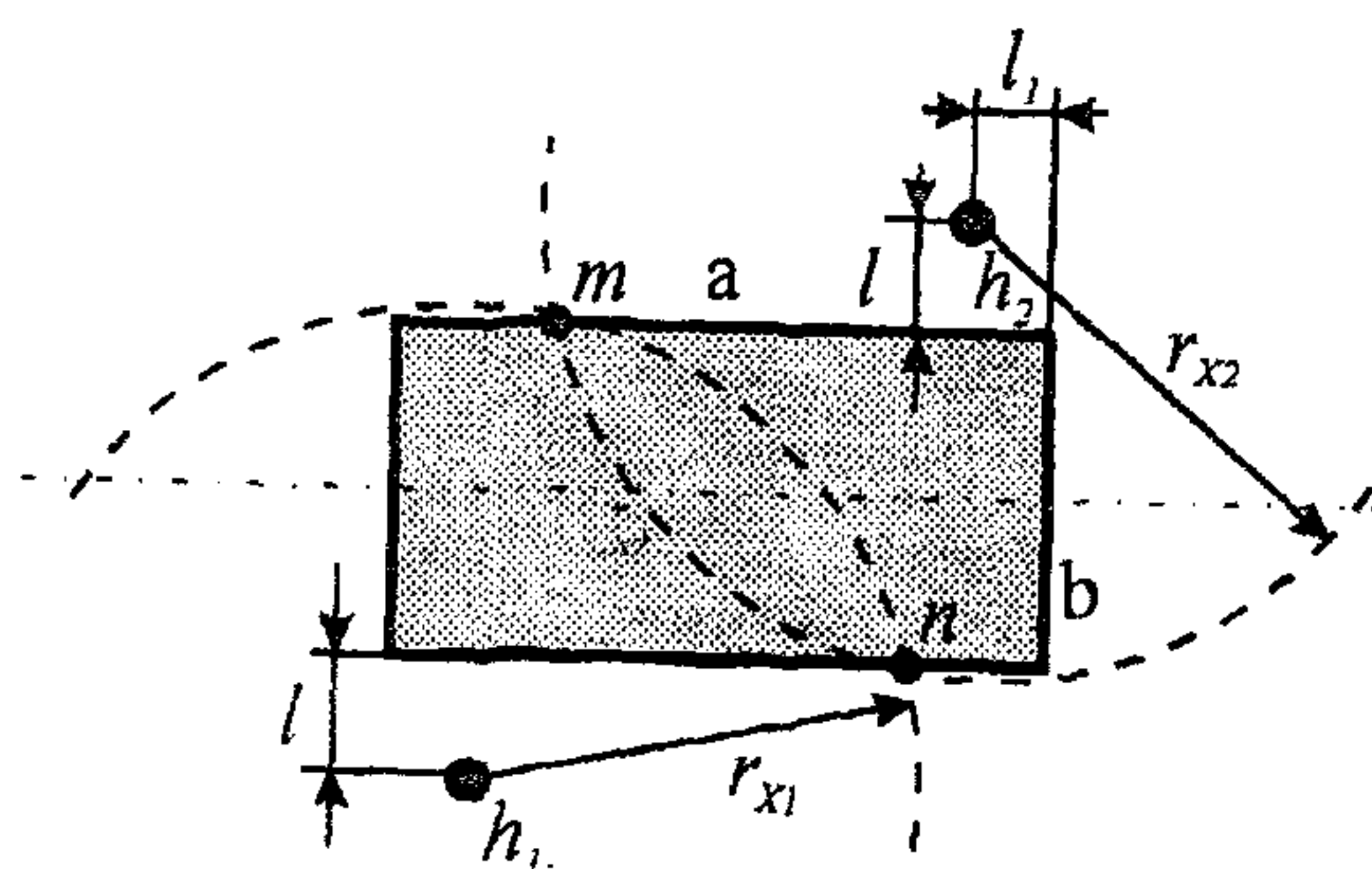
в) размещение молниеприемников по диагонали
