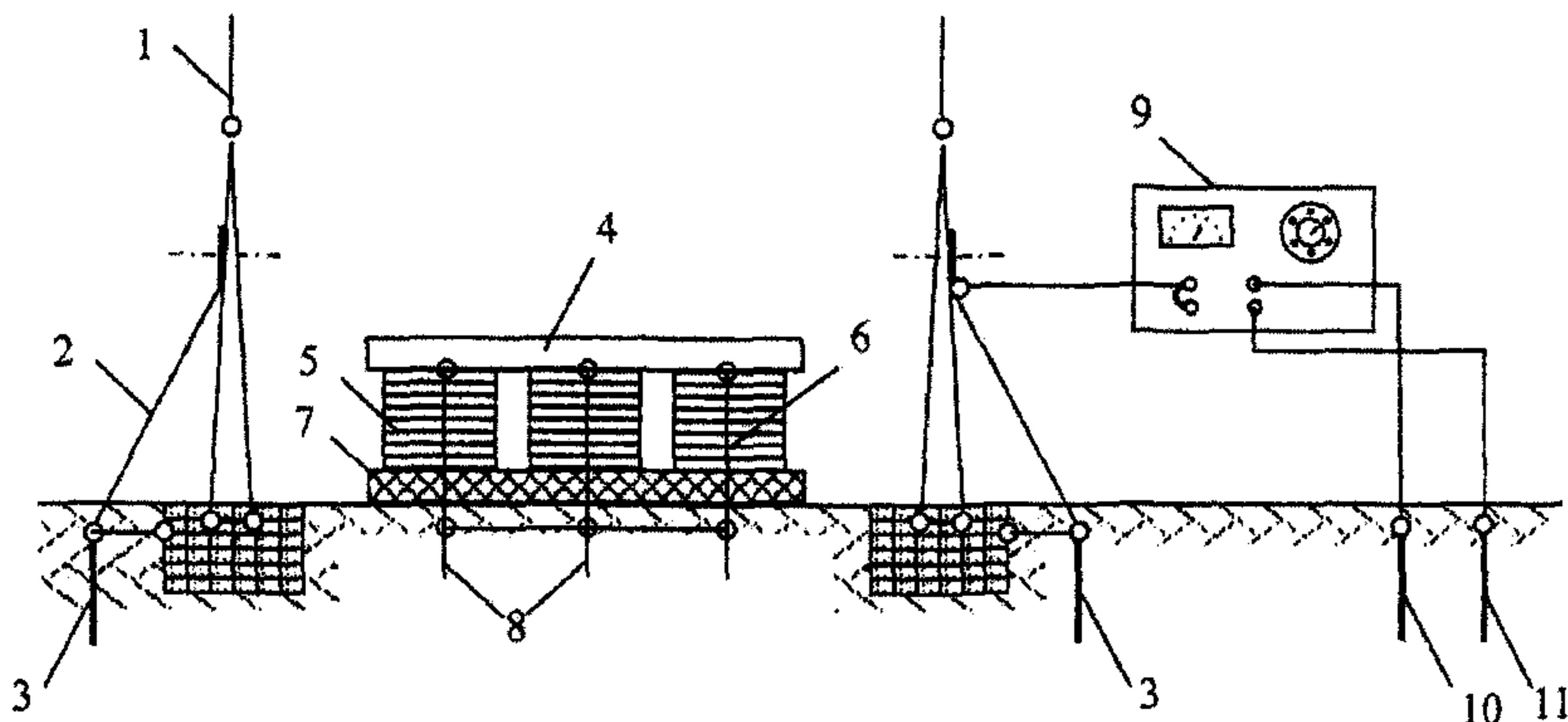
1-молниеприемник; 2-токоспуск; 3-искусственный заземлитель молниеотвода; 4-металлическая крыша хранилища; 5-штабели с изделиями; 6-заземляющие проводники металлической крыши; 7-диэлектрический фундамент хранилища; 8-электроды заземления объекта; 9-измерительный прибор; 10, 11-потенциальный и токовый электроды измерительного прибора
