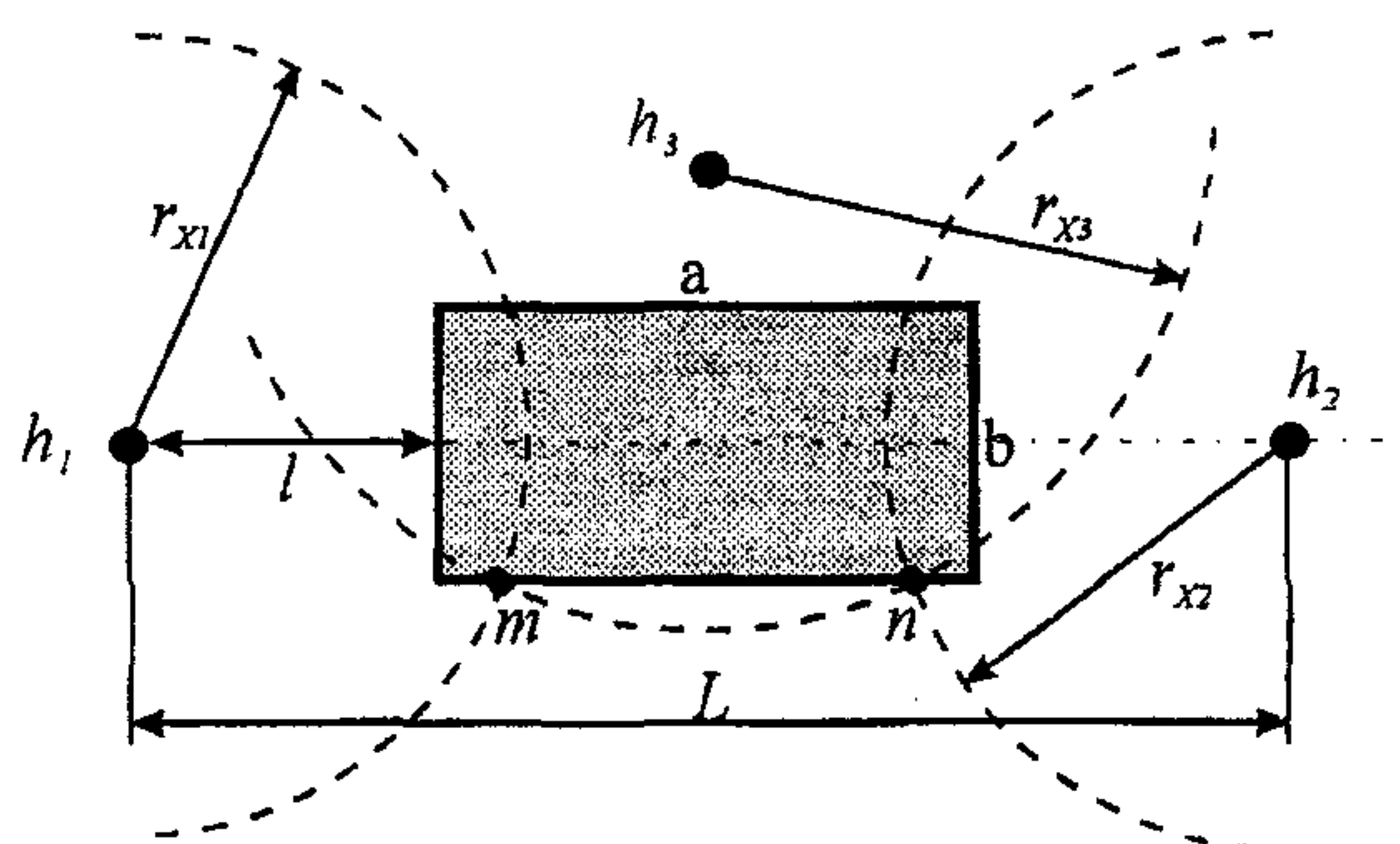
а) трехстержневая молниезащита протяженного объекта
