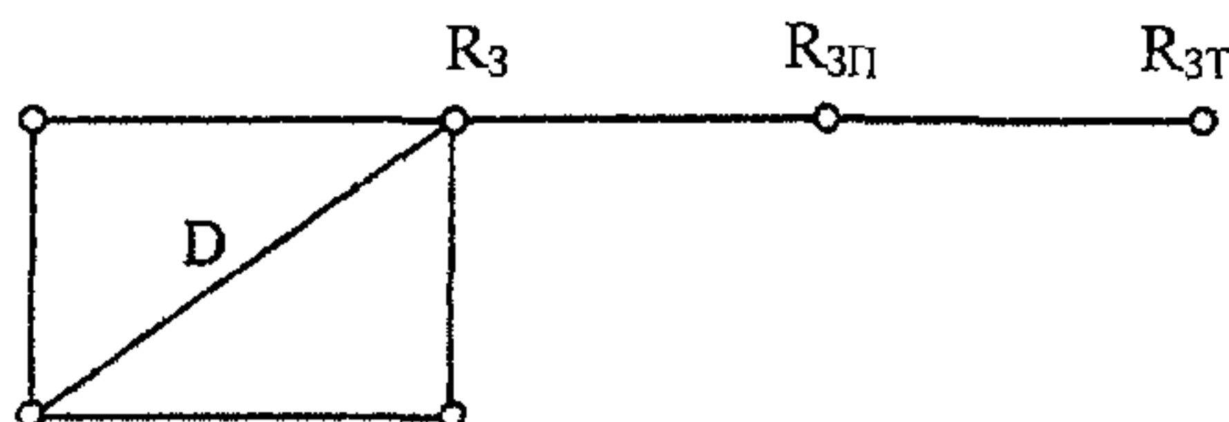
Рисунок Д.2.1 - Однолучевая схема измерений
