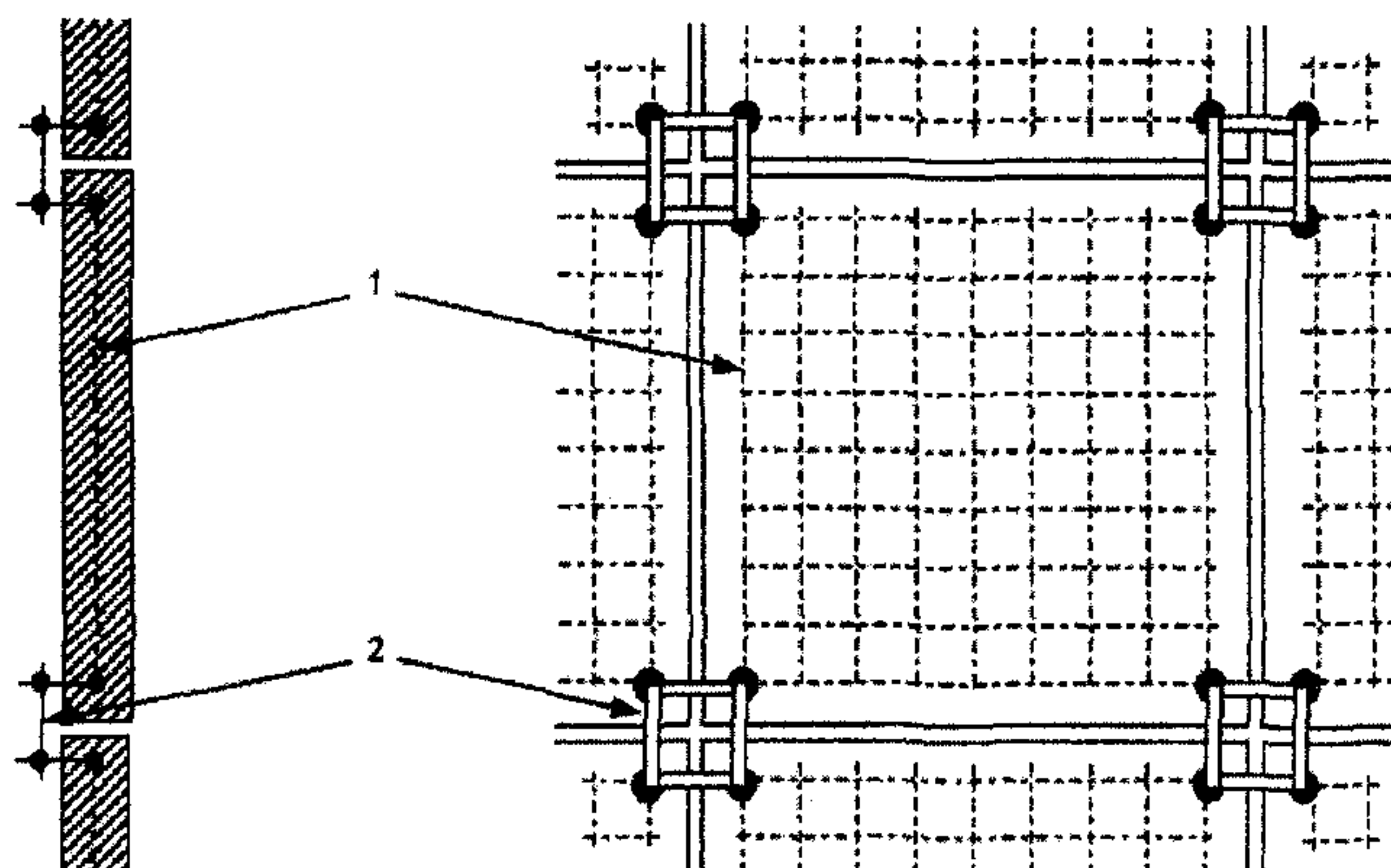
1 – железобетонный блок; 2 – соединительный проводник
