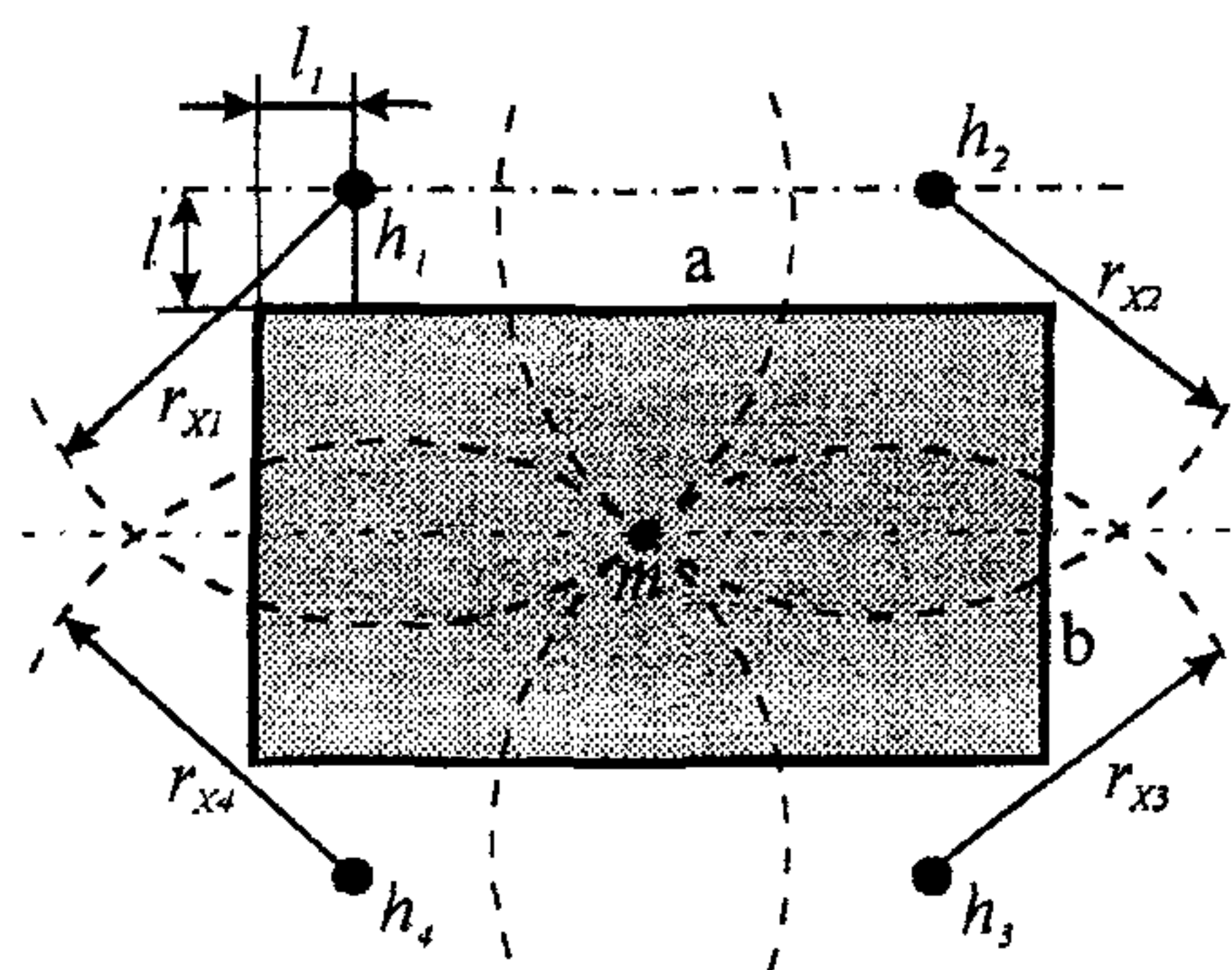
в) четырехстержневая молниезащита прямоугольного объекта
