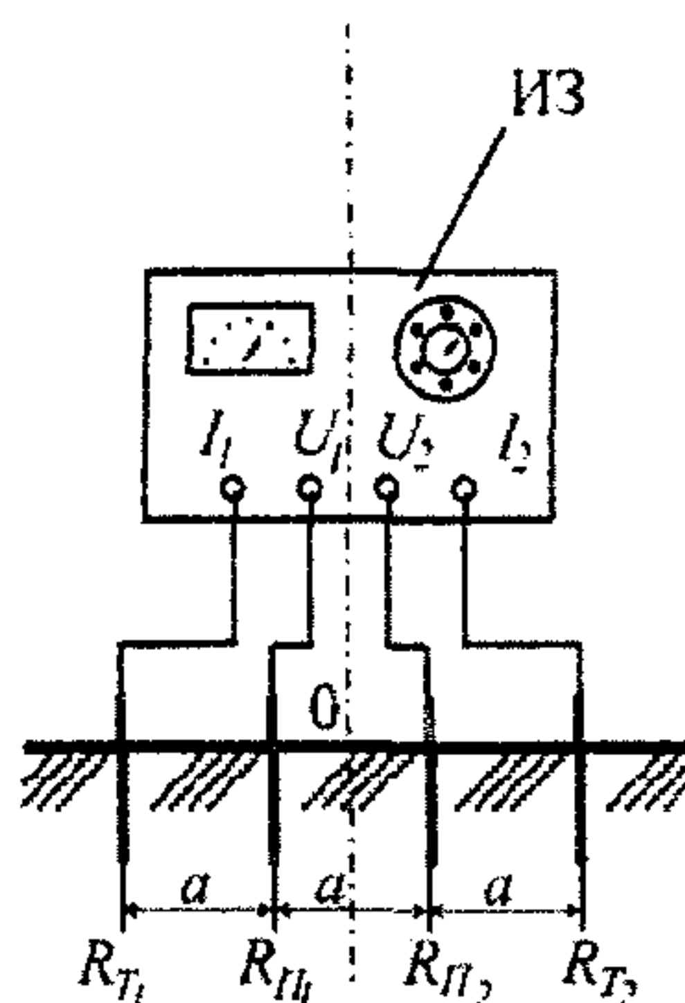
Рисунок Д.2.5 - Метод измерения прибором М416
