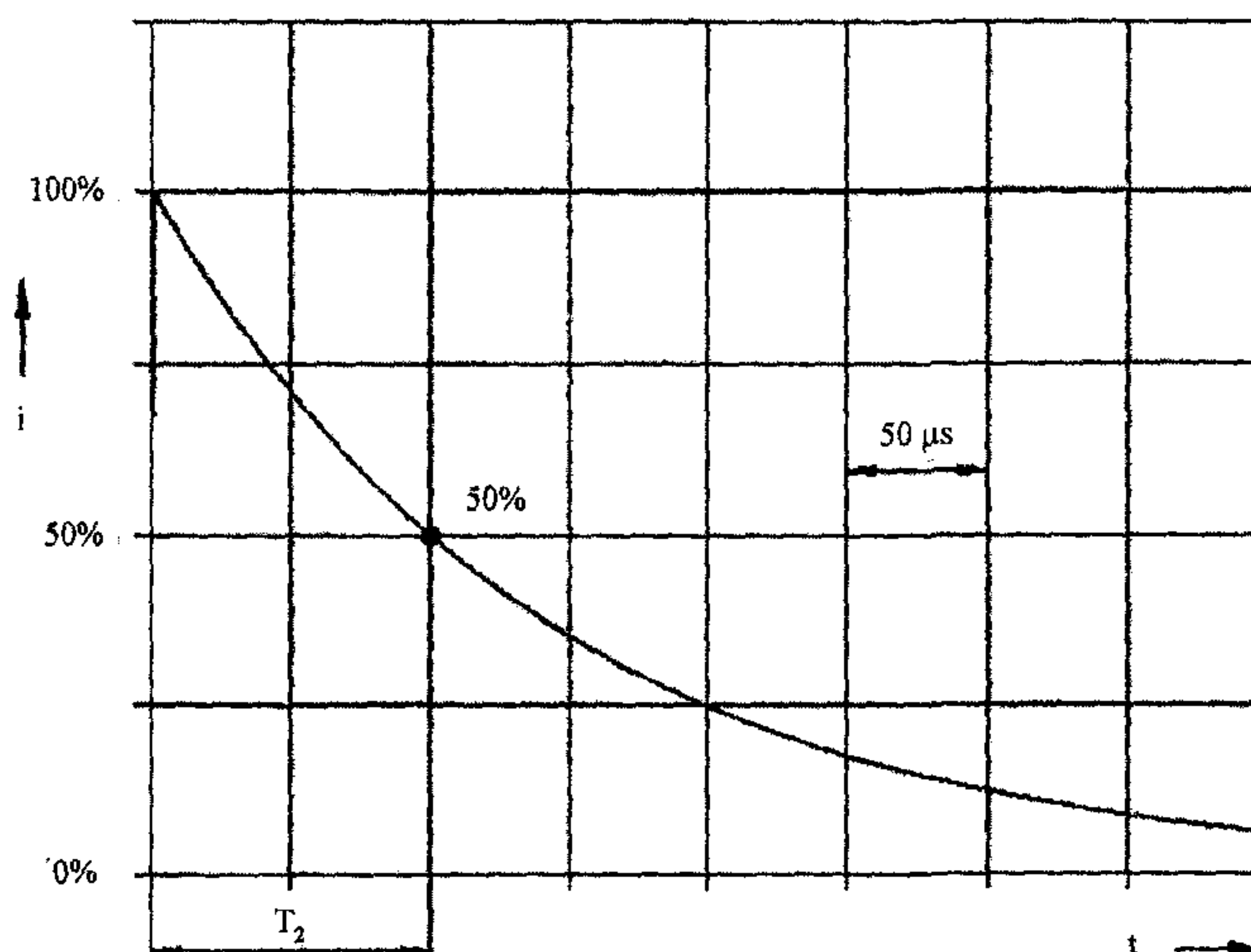
Рисунок Б.4 - Форма импульса тока на спаде для последующих коротких ударов
