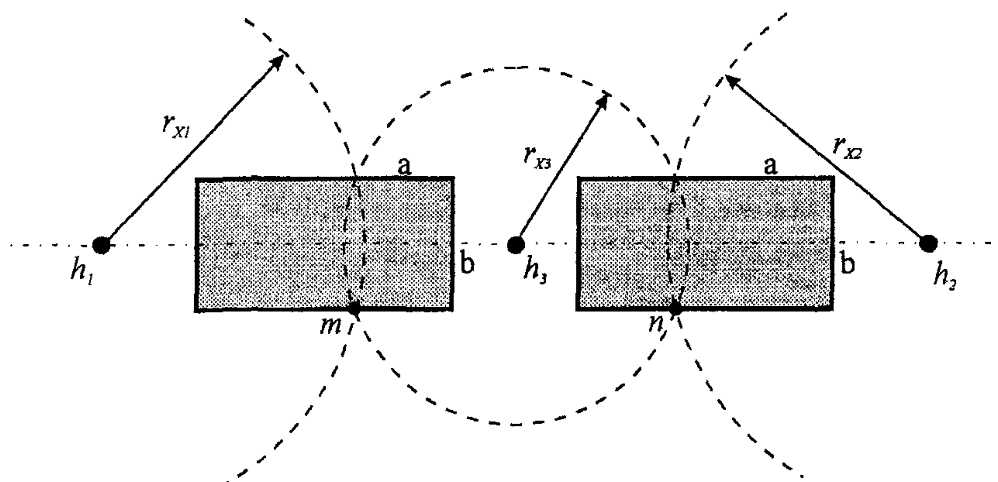
б) трехстержневая молниезащита двух рядом стоящих объектов
