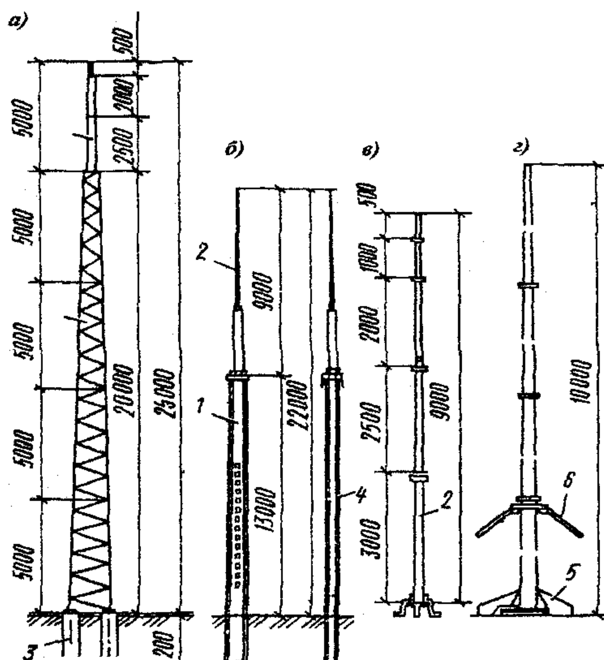
а – опора металлическая решетчатая; б – опора железобетонная; в – молниеприемник для железобетонной опоры; г – молниеприемник из газовых труб 1 опора (стойка); 2 – молниеприемник; 3 – фундамент опоры; 4 – токоотвод (спуск); 5 – фланец, 6 – оттяжка
