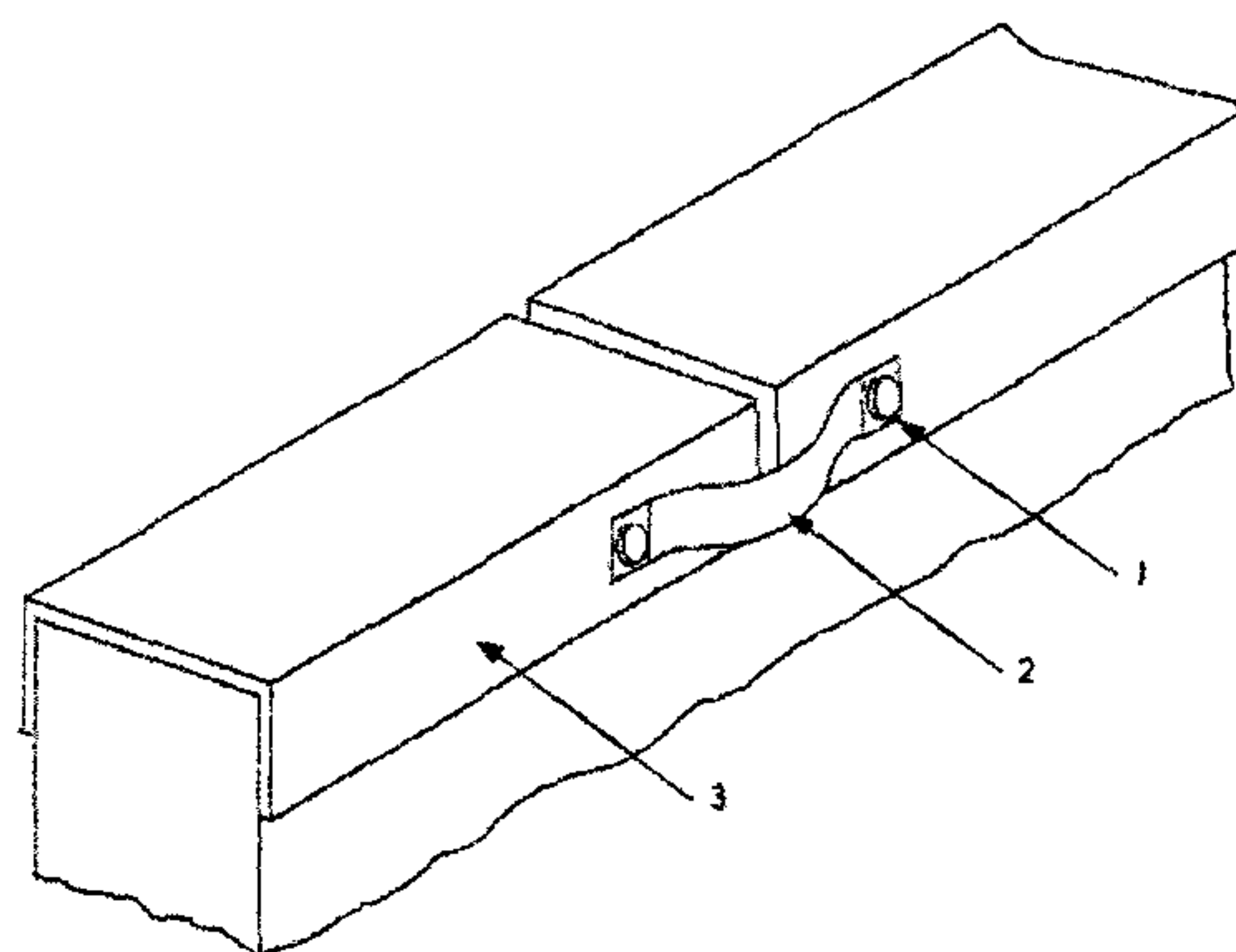
Рисунок Г.30 - Пример устройства металлического покрытия на парапете крыши
