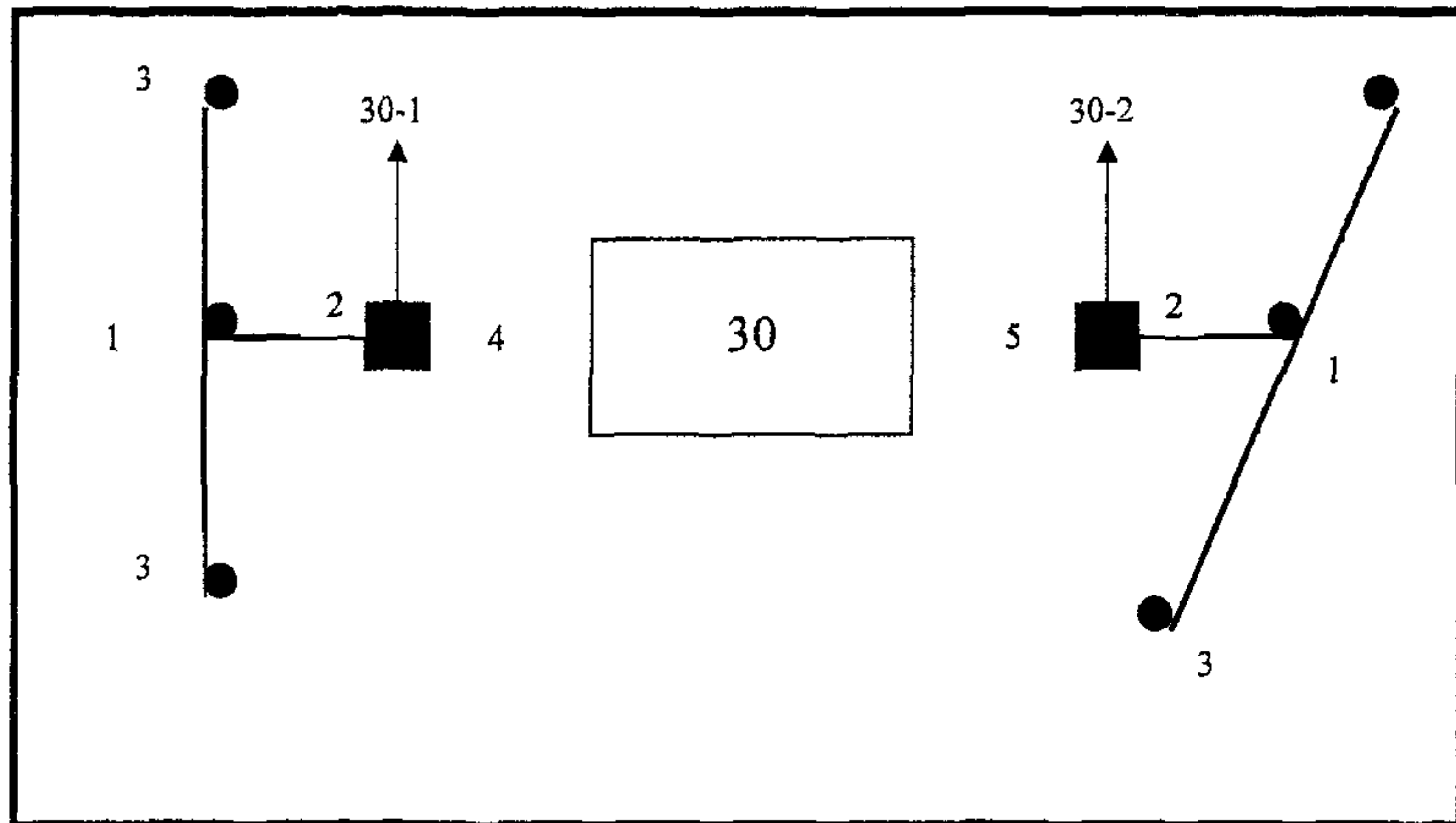
Размер 280х210мм; фон белый; надпись черным цветом; кайма 10мм черным цветом; толщина линий 1,5мм; высота знаков 10мм На схеме показаны: 30 – форма периметра защищаемого здания, сооружения, открытой площадки с номером его по генплану; 30-1, 30-2 – молниеотводы с указанием их порядковых номеров; 1, 3 – заземлители с указанием их лучей; 2 - токопуски; 4,5 – расстояния (м) от защищаемого здания, сооружения, открытой площадки до молниеотводов
