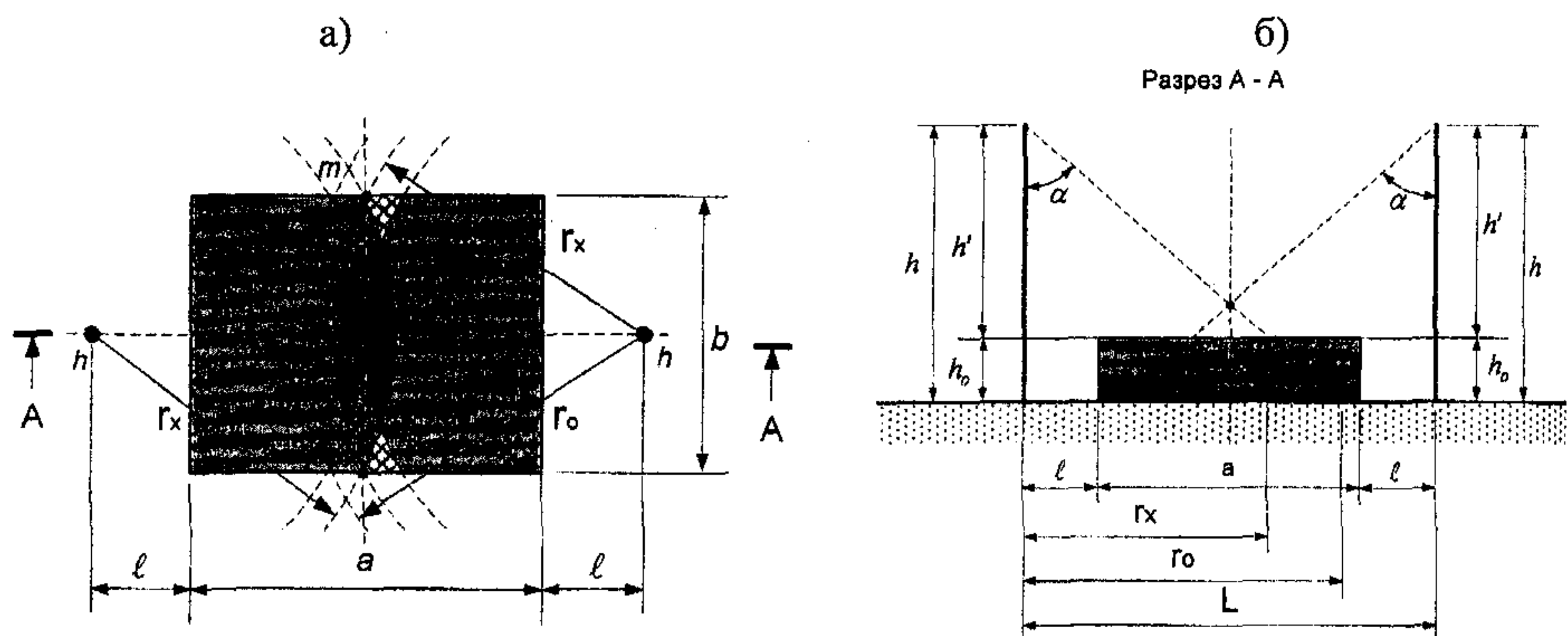
Рисунок 2.3 – Схема для расчета высоты двухстержневых молниеотводов
