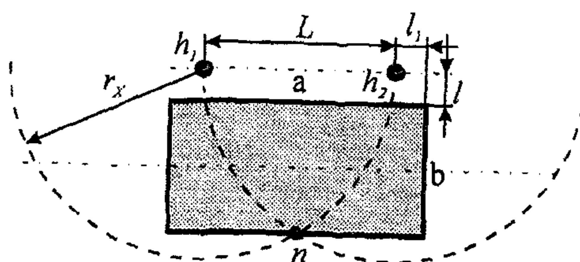
б) одностороннее размещение двухстержневой молниезащиты
