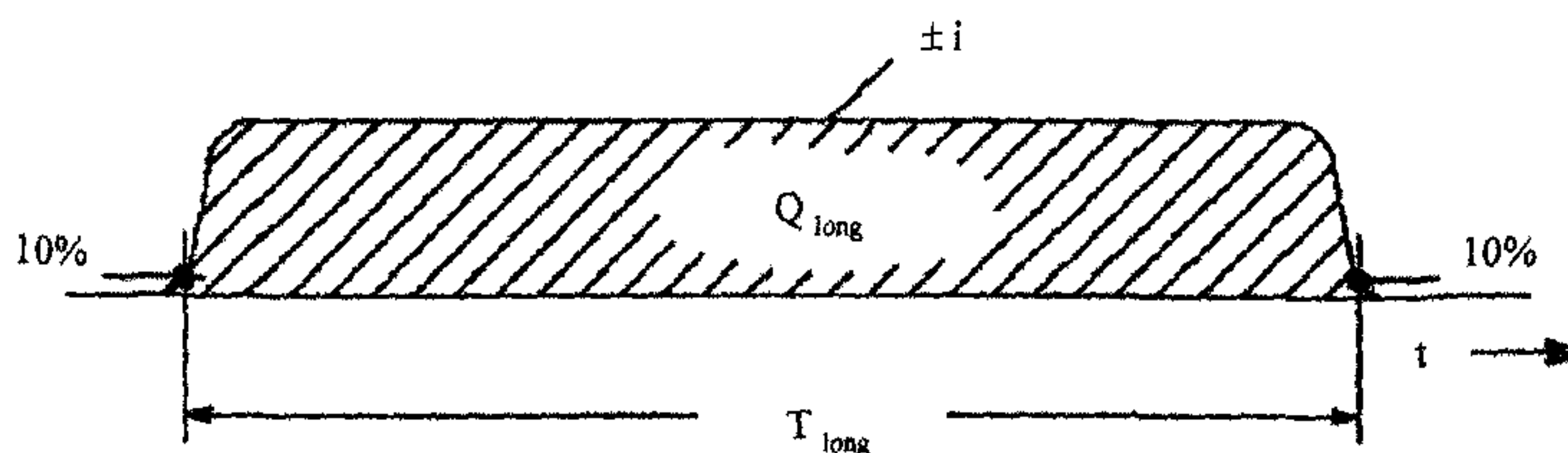
Рисунок Б.2 - Схематичное изображение параметров длинного разряда
