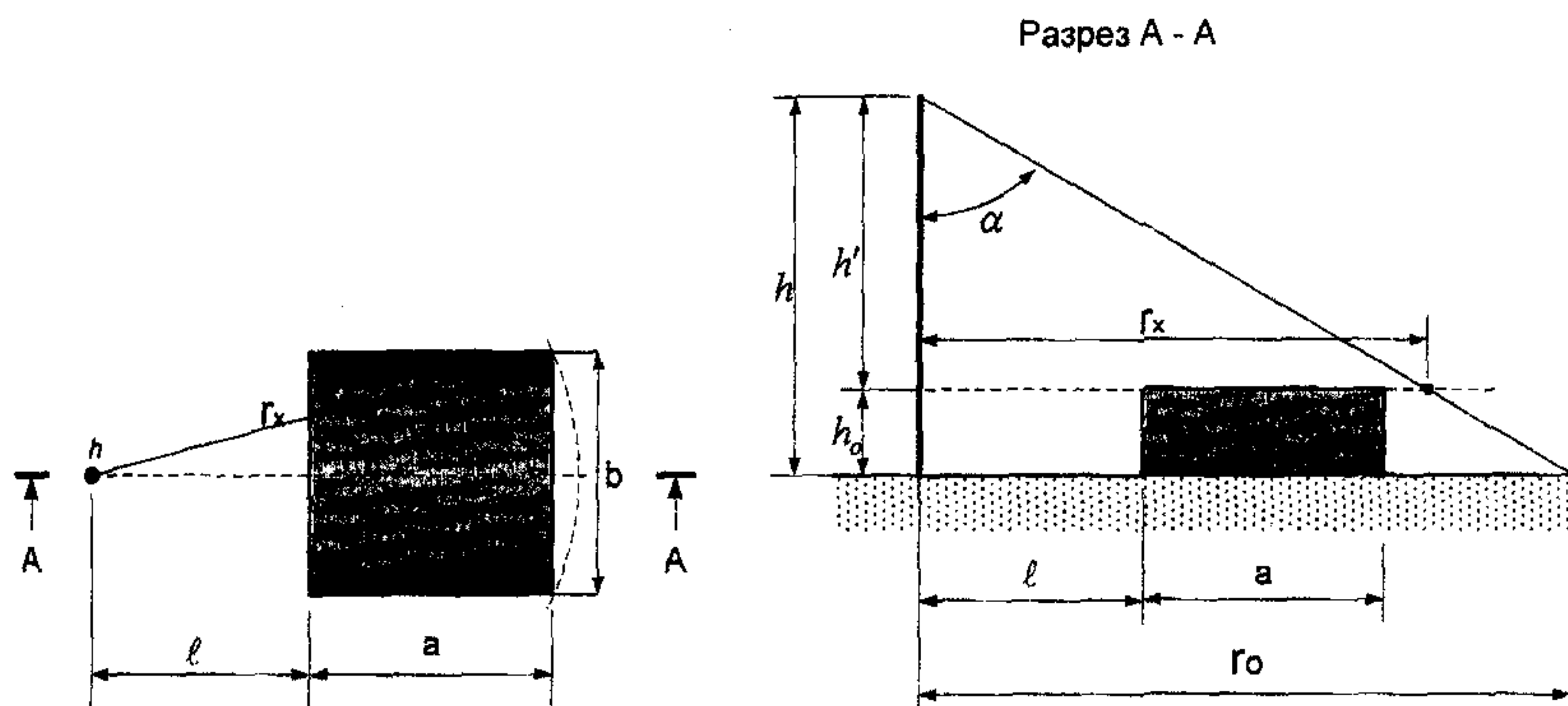
Рисунок 2.2 - Схема для расчета высоты стержневого молниеотвода
