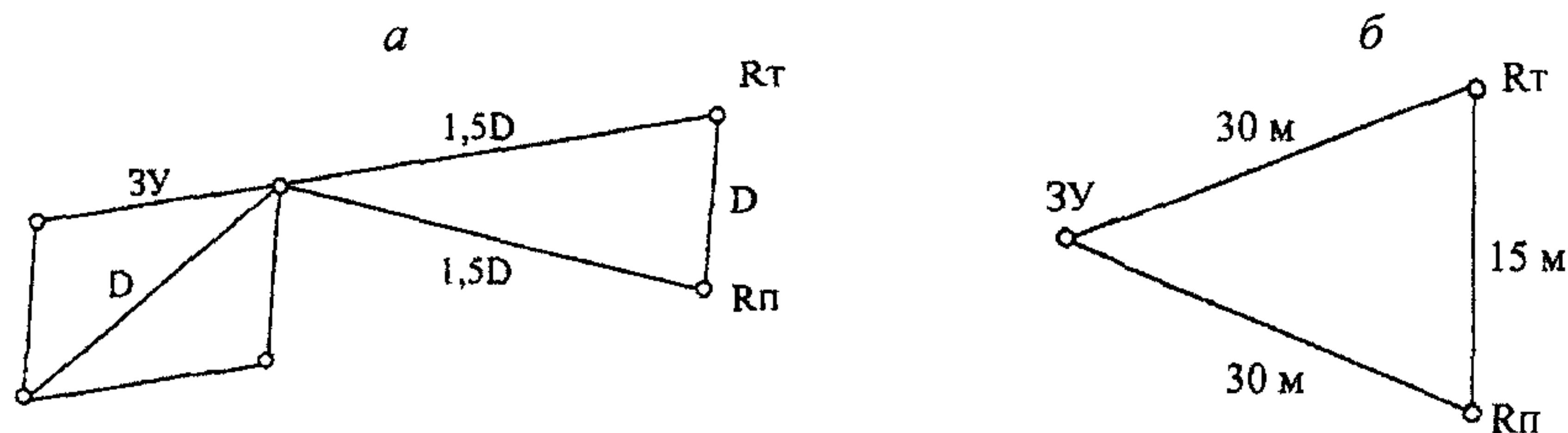
Рисунок Д.2.2 - Двухлучевые схемы измерений
