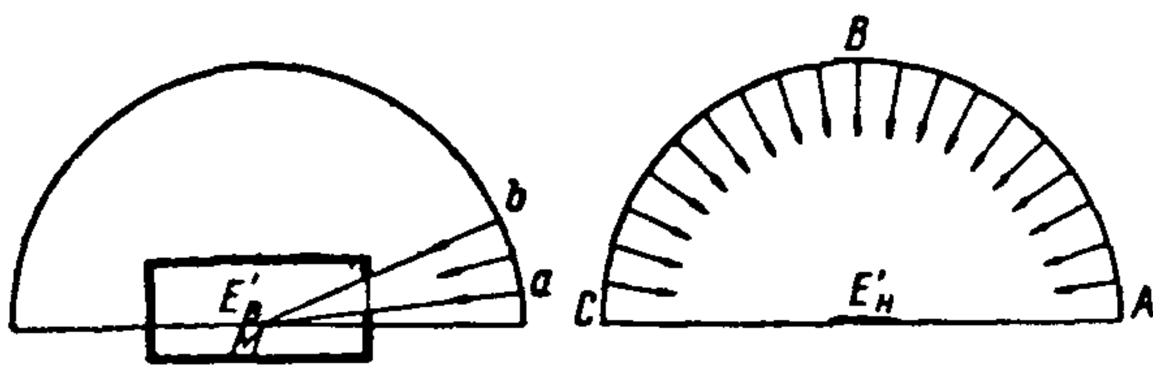
рис. 3. Схема для определения коэффициента небосвода E'_B — освещенность внутри помещения без учета светопотерь и отраженного света; E'_H — наружная горизонтальная освещенность при равномерной яркости неба
