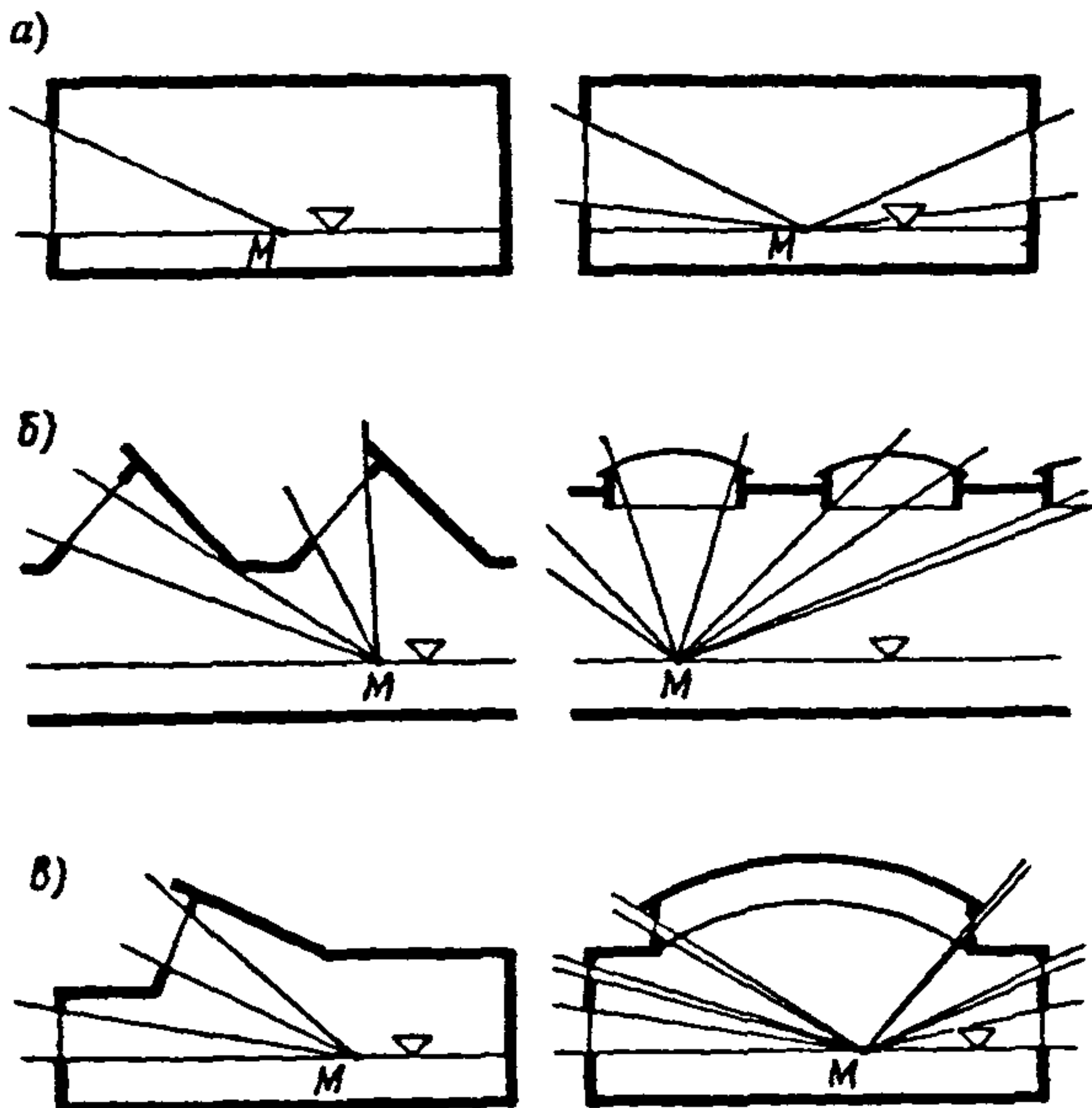
Рис. 1. Схема естественного освещения а — боковое освещение; б — верхнее освещение в — комбинированное освещение, ▽ — уровень рабочей плоскости
