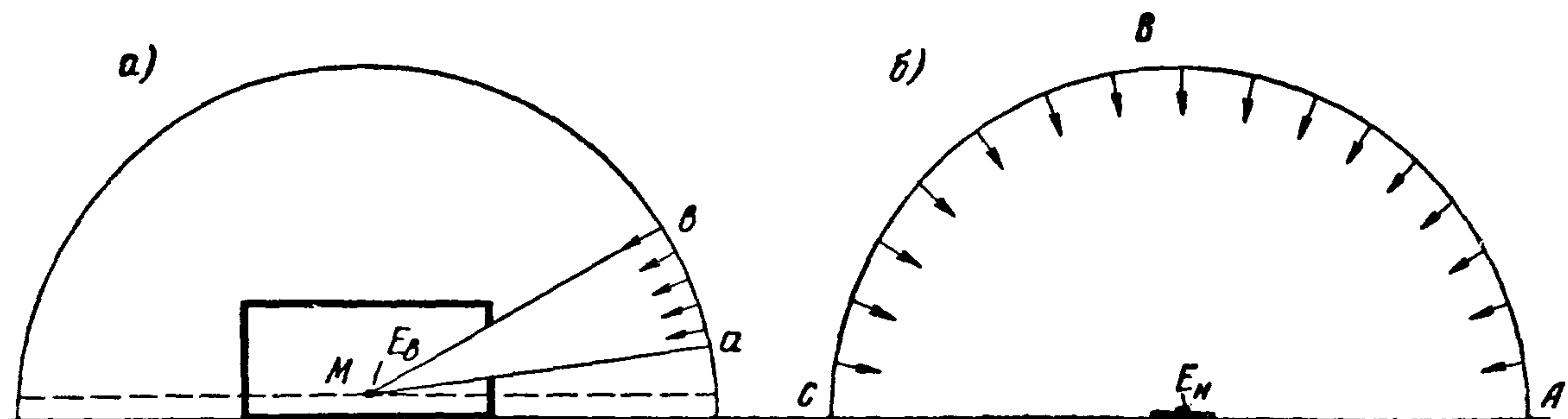
Рис. 1. Схема для определения коэффициента естественной освещенности E_b — освещенность внутри помещения; E_n — наружная горизонтальная освещенность
