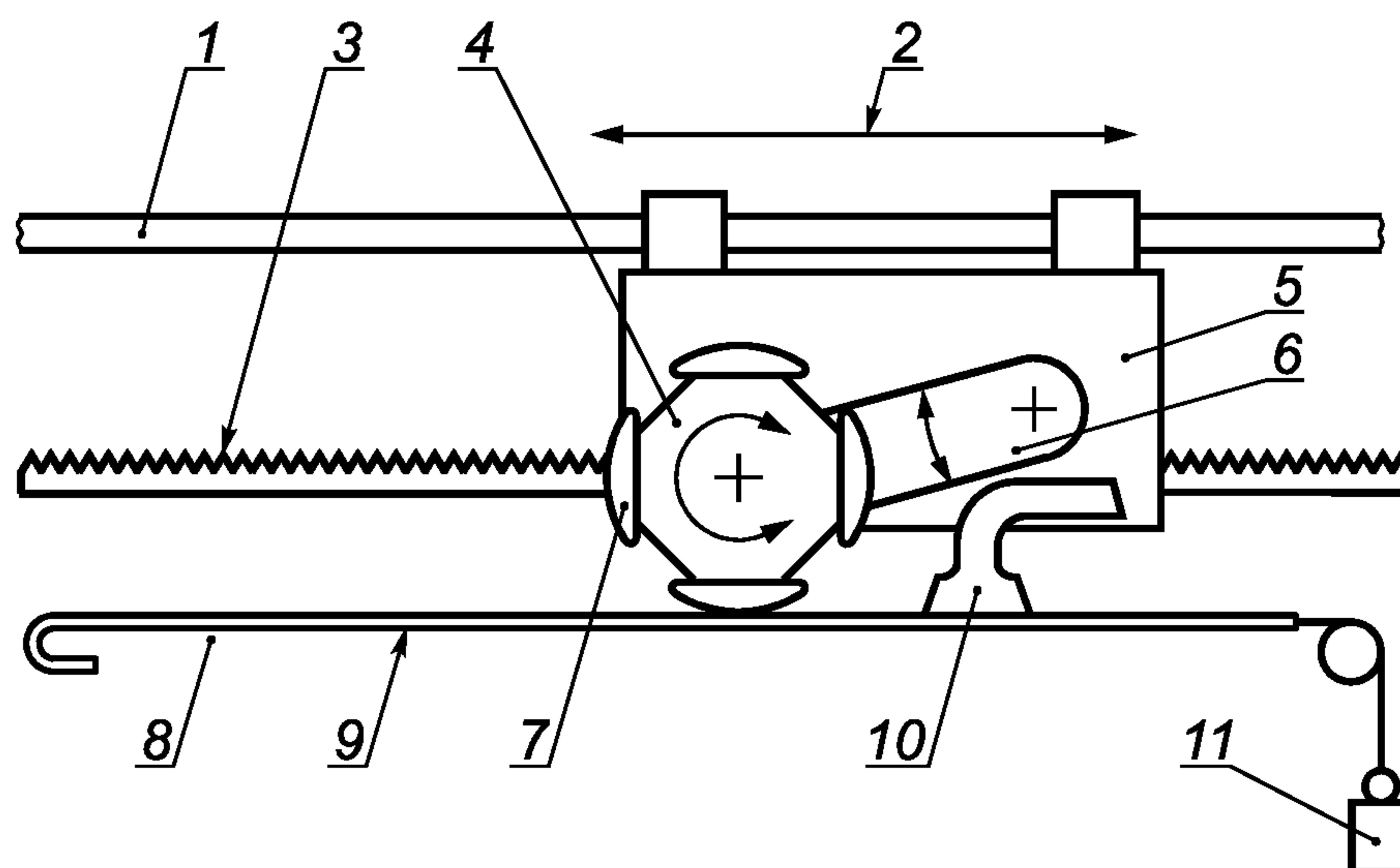
1 — направляющая планка; 2 — направление движения; 3 — зубчатая рейка; 4 — третрад; 5 — рама; 6 — кулиса; 7 — стопа; 8 — плоский столик для укладки проб; 9 — проба; 10 — пылесос; 11 — предварительная нагрузка
