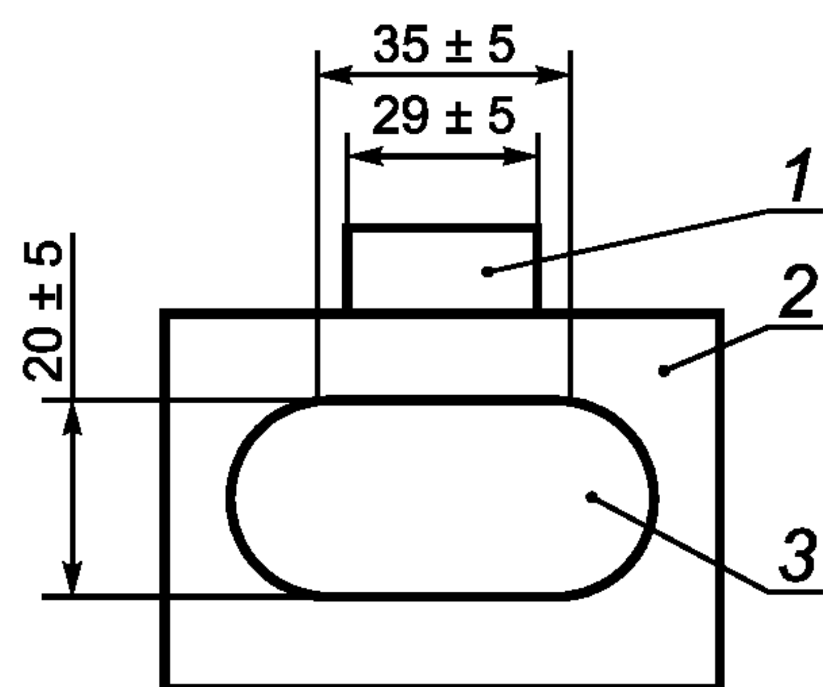
1 — соединение с пылесосом; 2 — отверстие сопла; 3 — насадка
