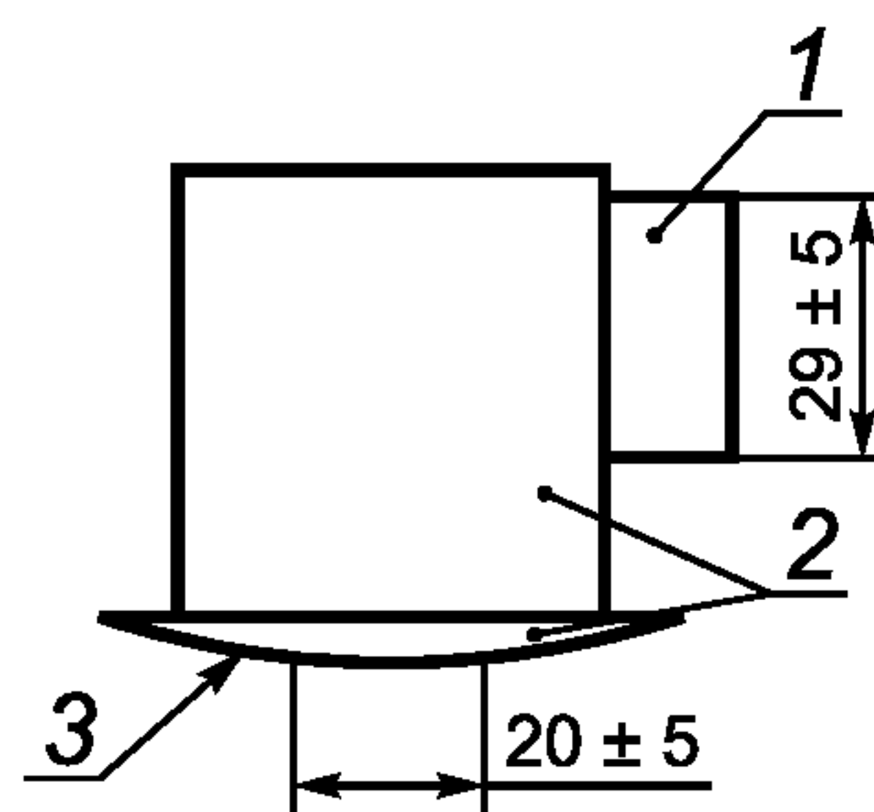
1 — соединение с пылесосом; 2 — отверстие сопла; 3 — насадка
