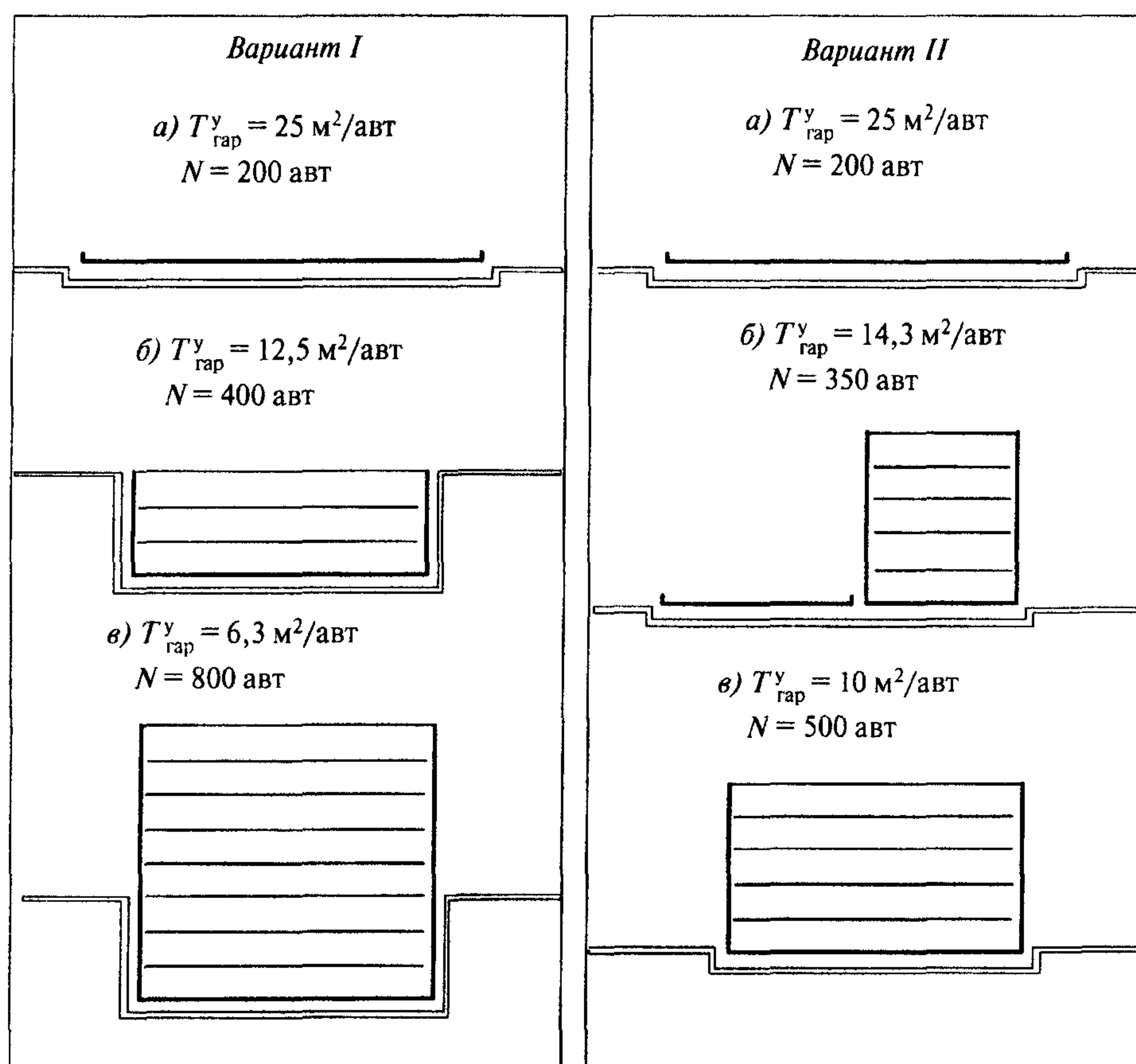
Рисунок 1 — Варианты стадийного увеличения вместимости зоны хранения автомобилей
