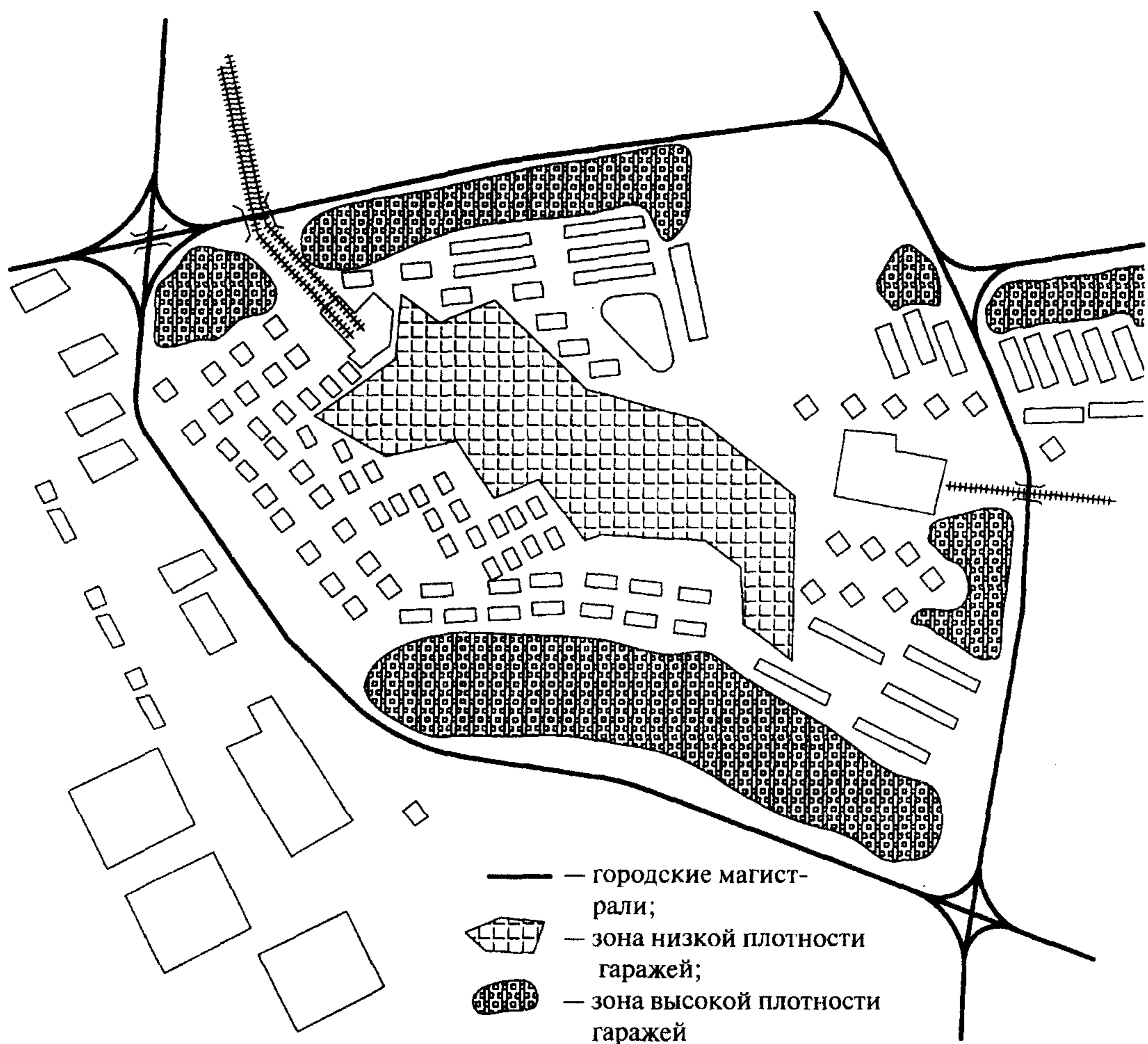
Рисунок 2 — Принципиальная схема размещения гаражей в жилой зоне
