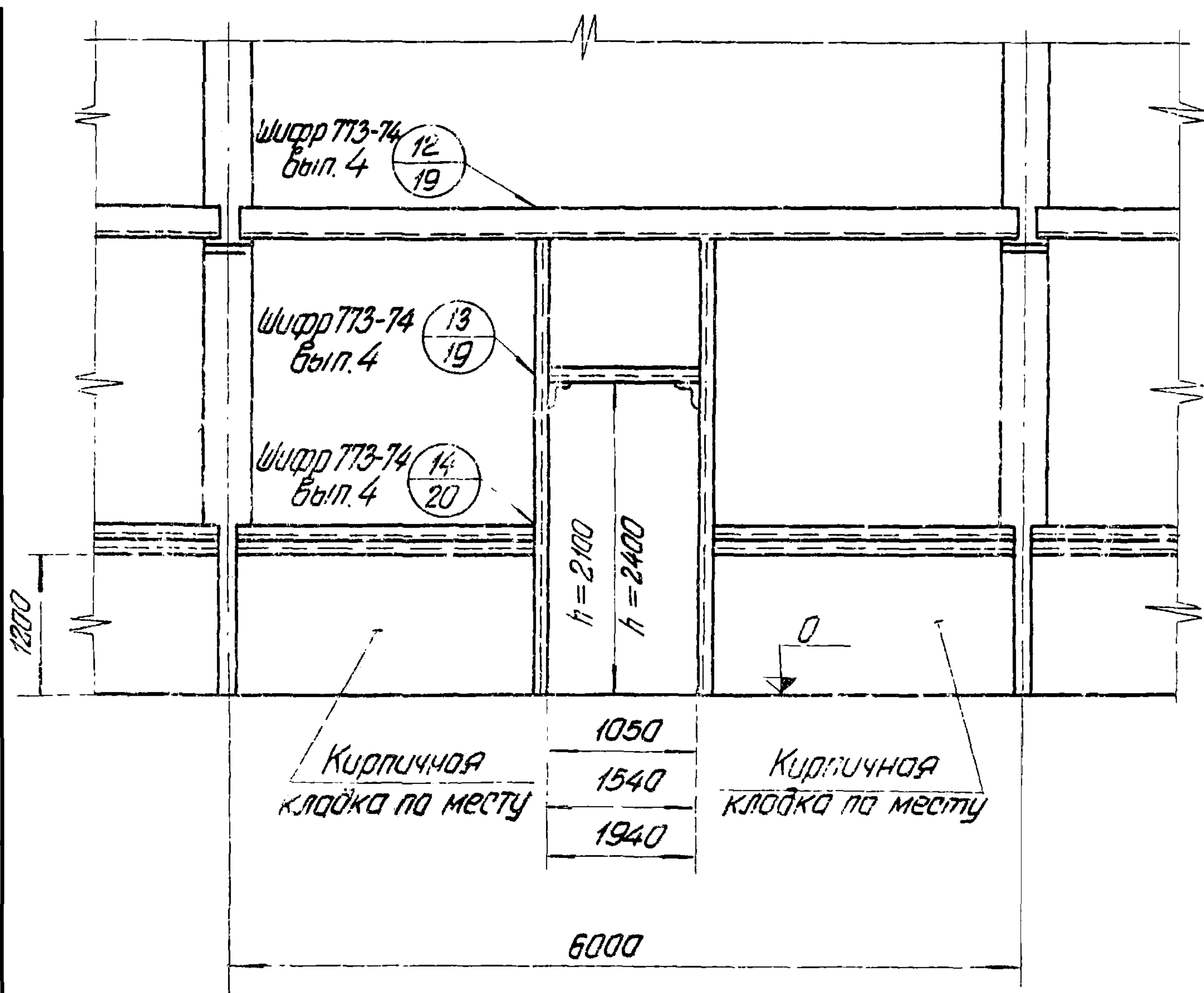
Рис. 3. 1.3 Маркирабочная схема узлов крепления обрамления дверного проема к элементам каркаса здания.
