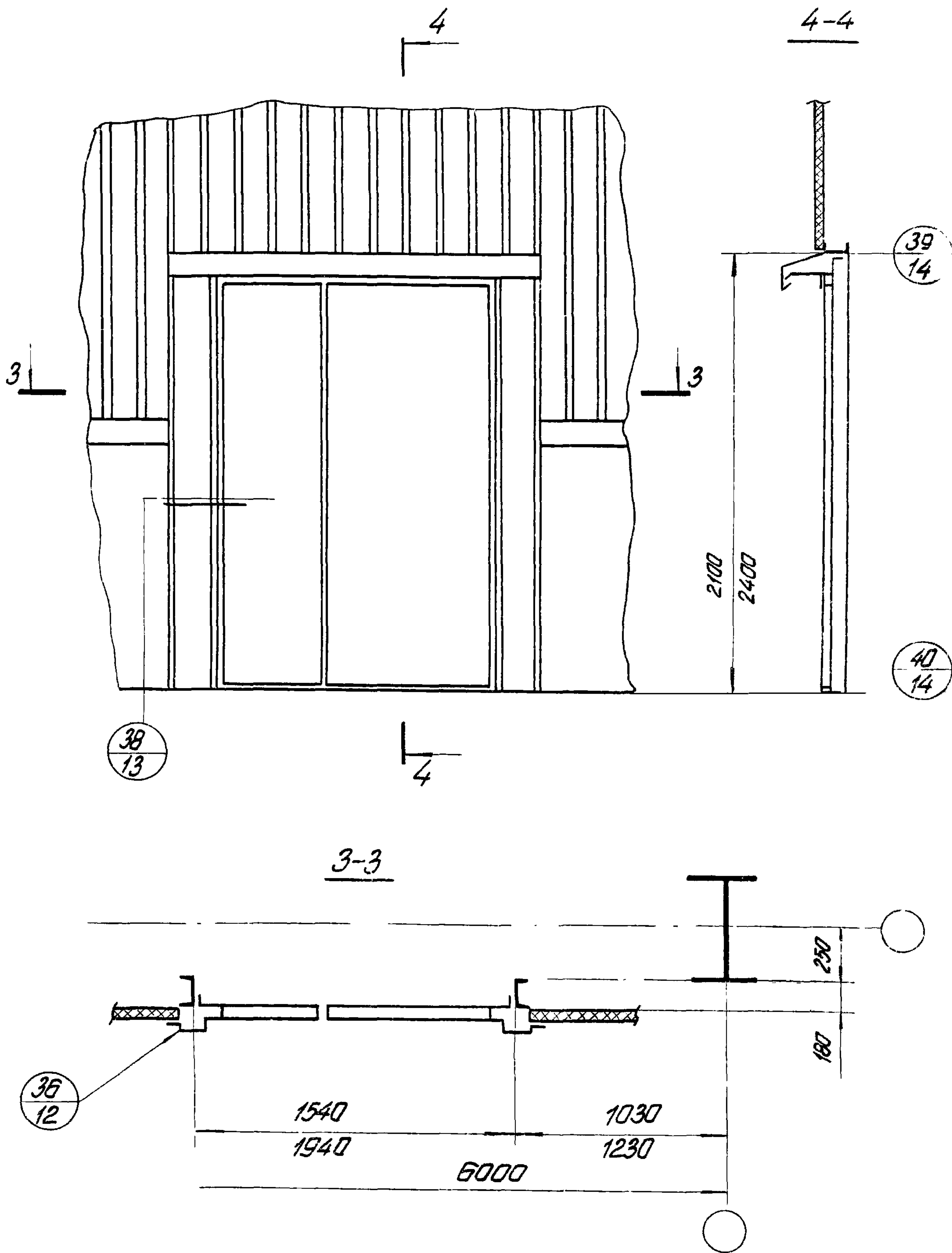
Рис. 3. 1. 2 Маркировочная схема архитектурных узлов
