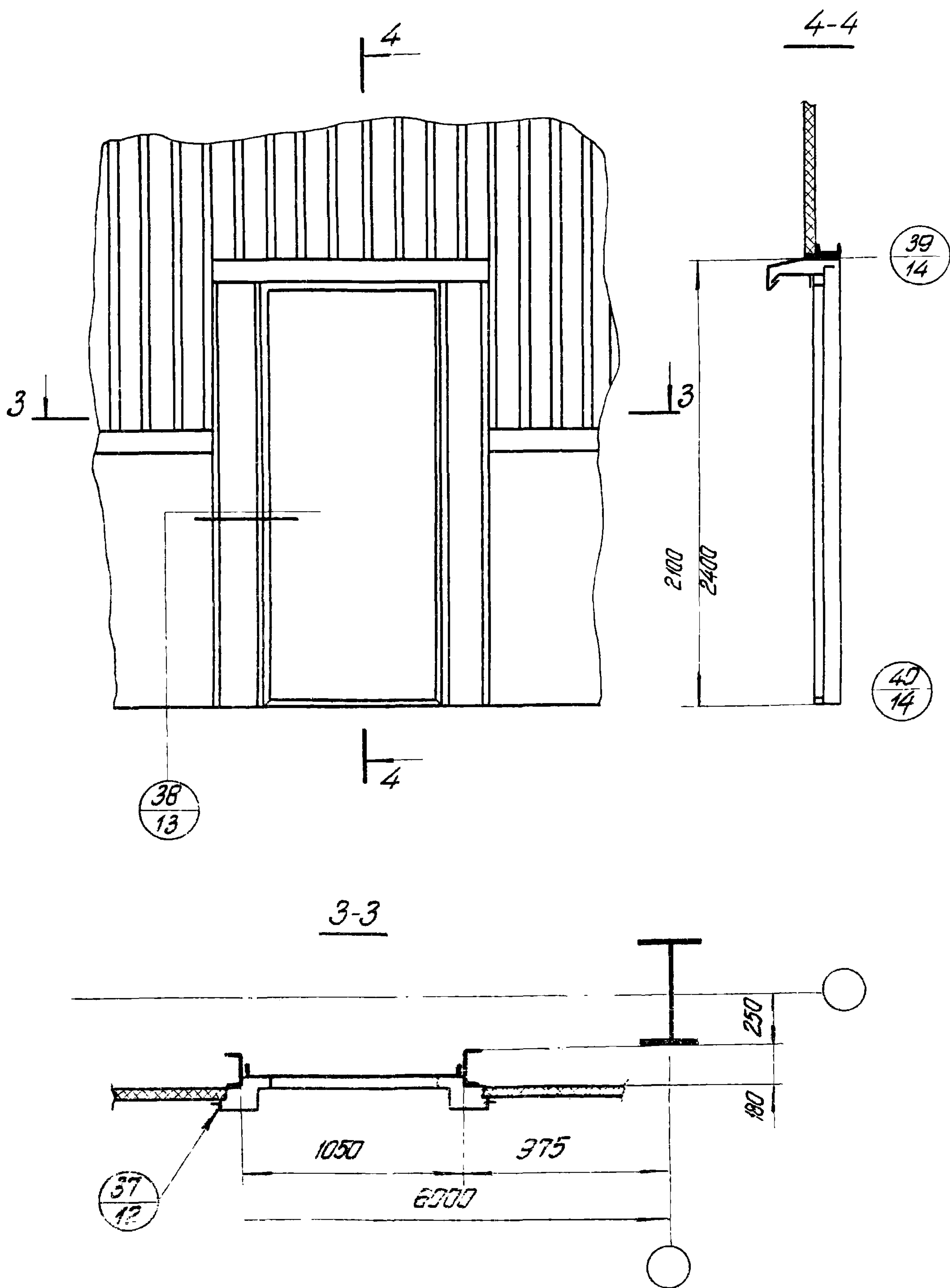
Рис. 3.11 Маркировочная схема архитектурных узлов.
