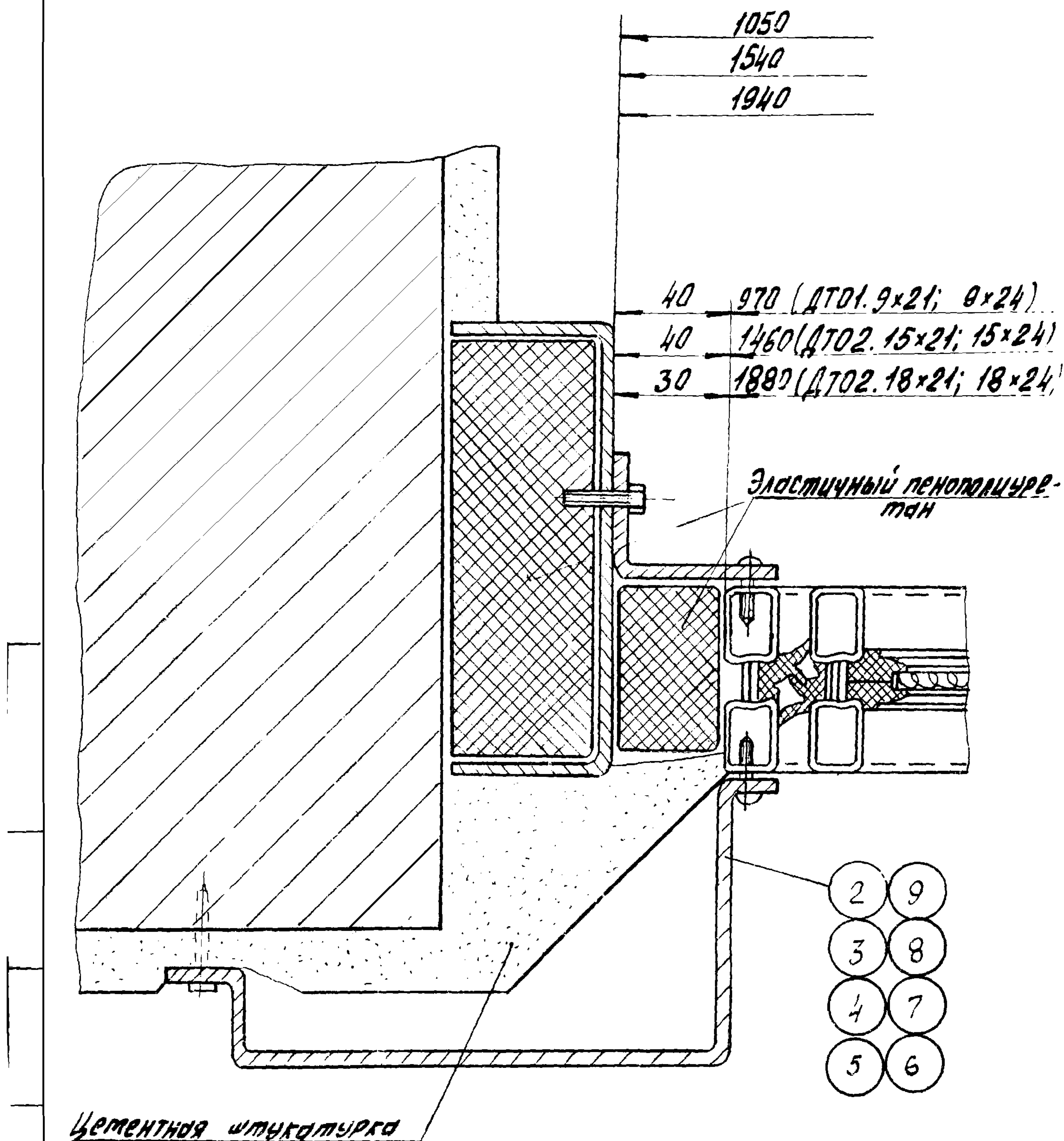
Рис. 3.15. Установка дверного блока типа ДТО и ДТГ в стене. Расонные элементы № 2-9 см. шифр 773-74, выпуск 4, лист 52.
