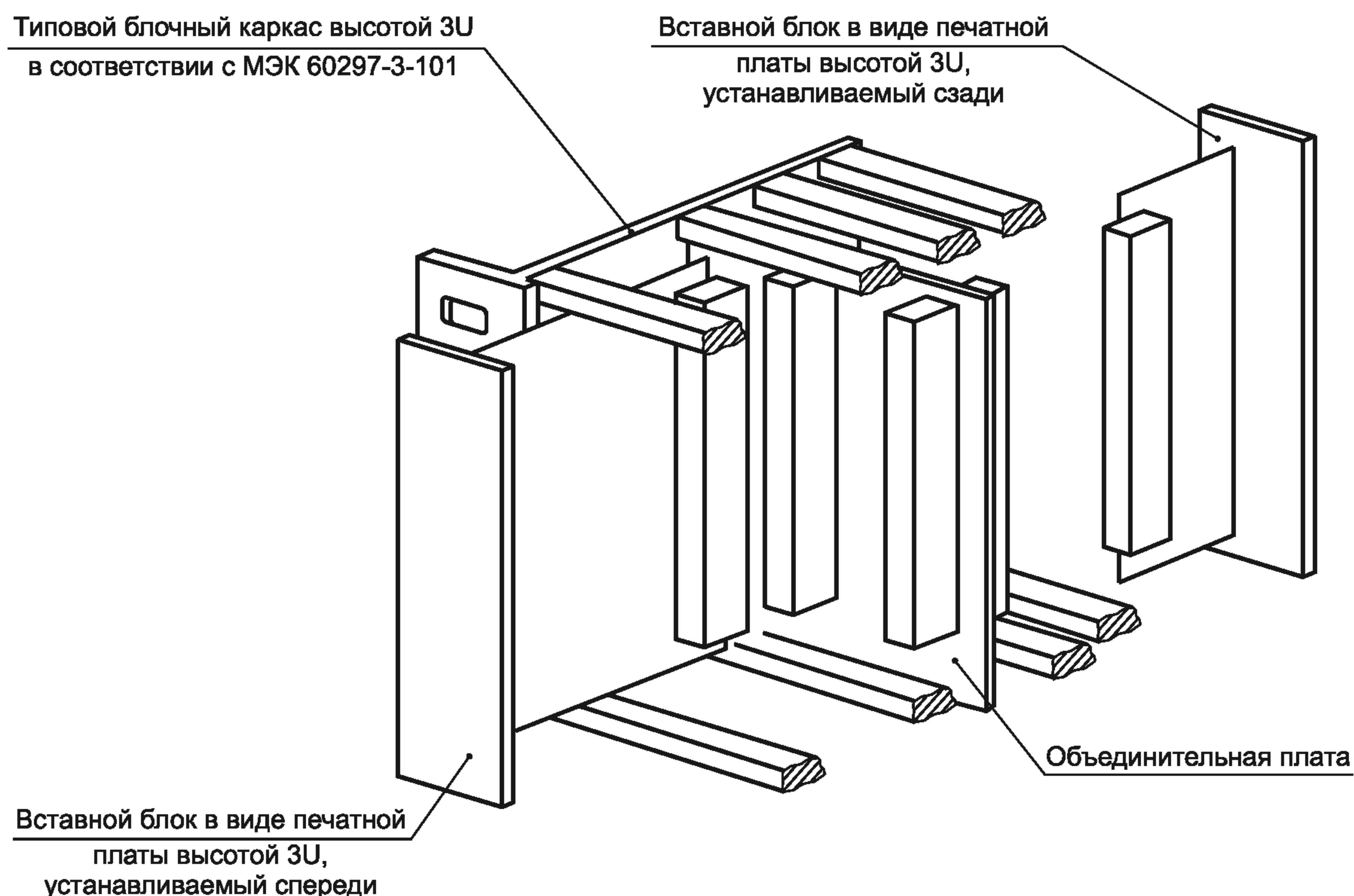
Рисунок 1 — Общая компоновка
