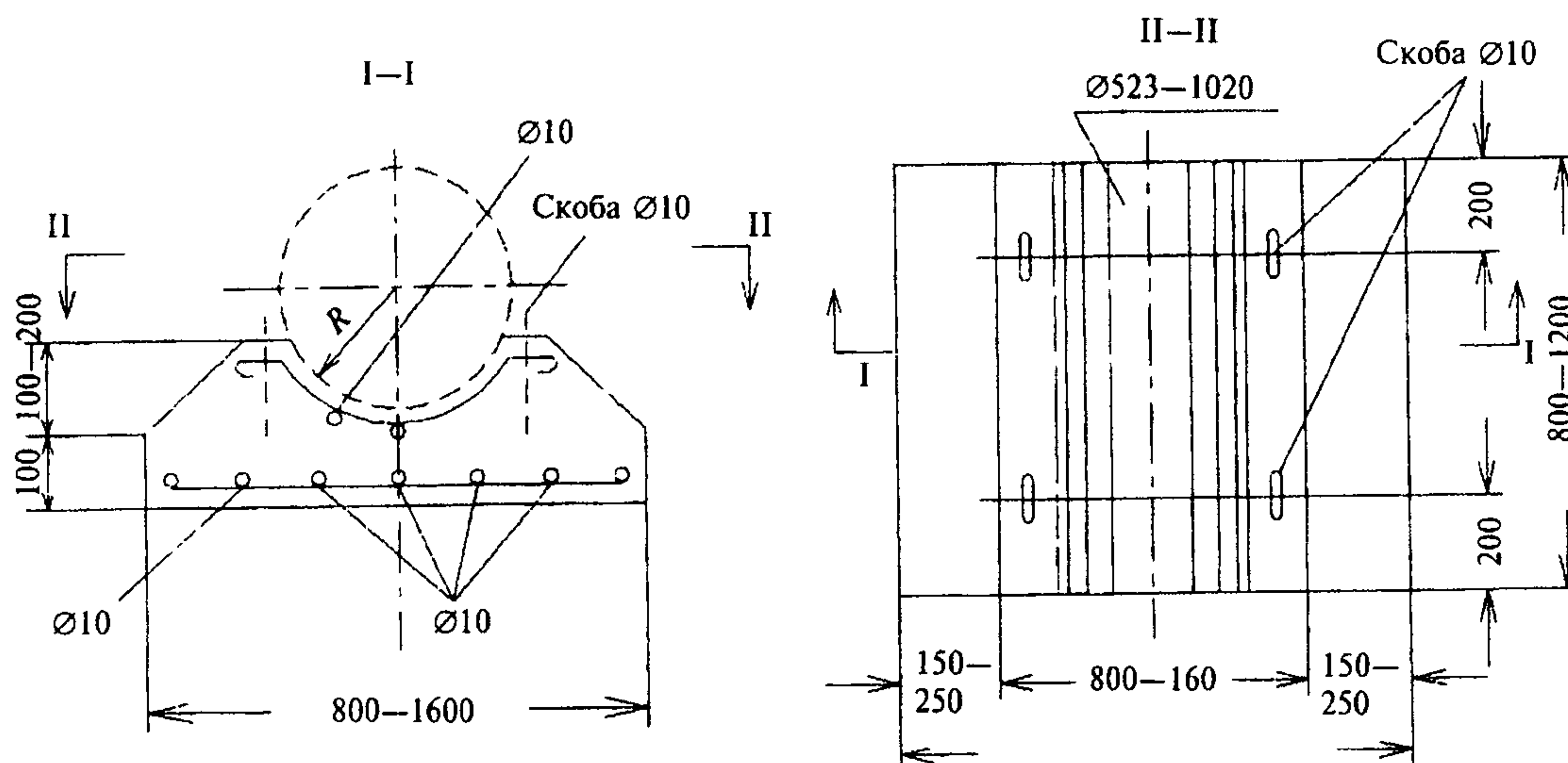
Рисунок 6.4 — Плитная опора с ложем для укладки трубопровода
