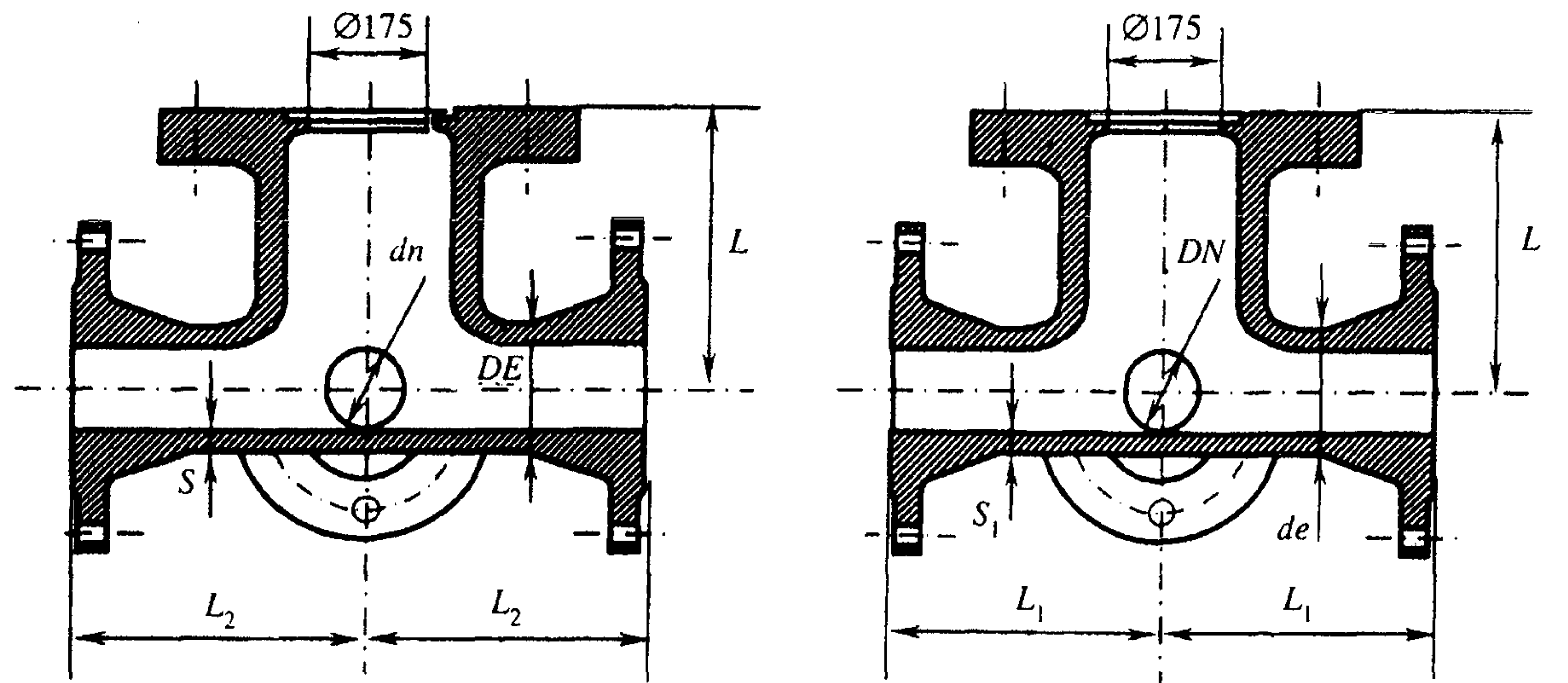
Рисунок Б.31 — Крест фланцевый с пожарной подставкой
