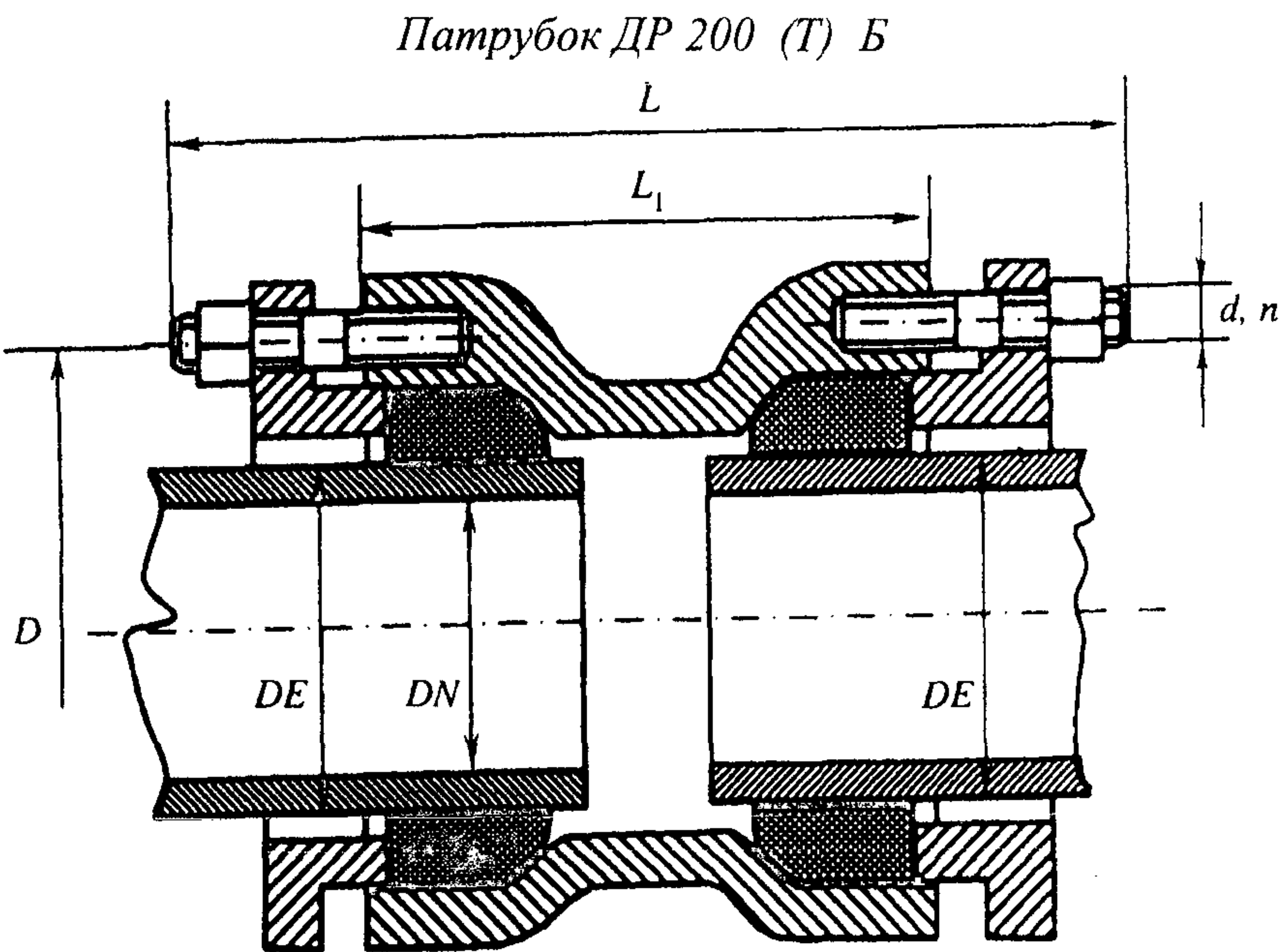
Рисунок Б.21 — Двойной раструб компенсационный
