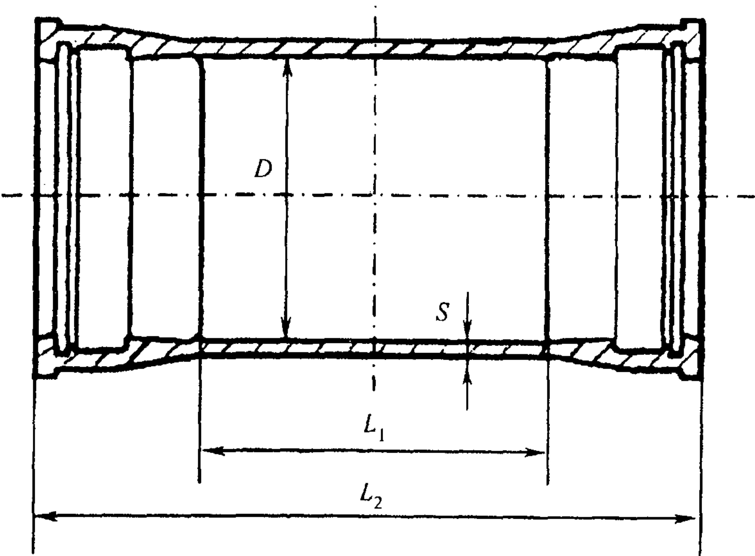
Рисунок Б.33 — Муфта надвижная
