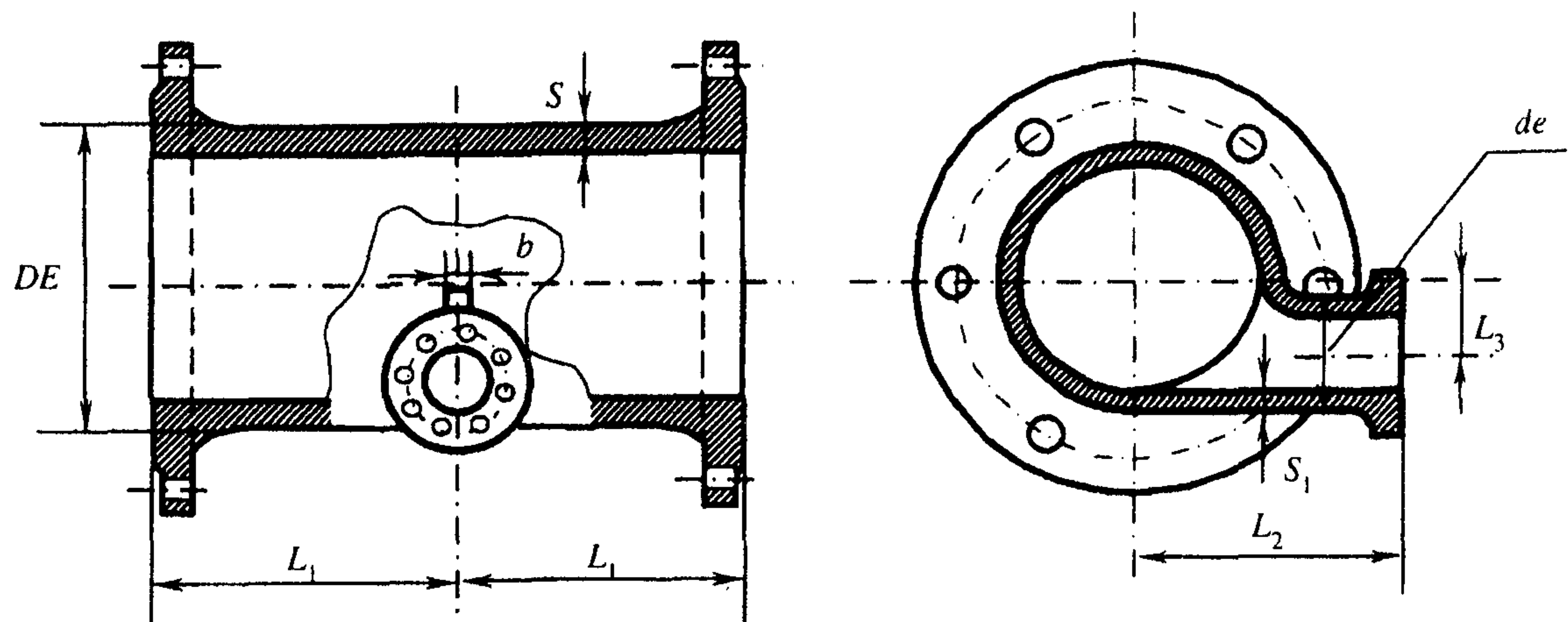
Рисунок Б.23 — Выпуск фланцевый
