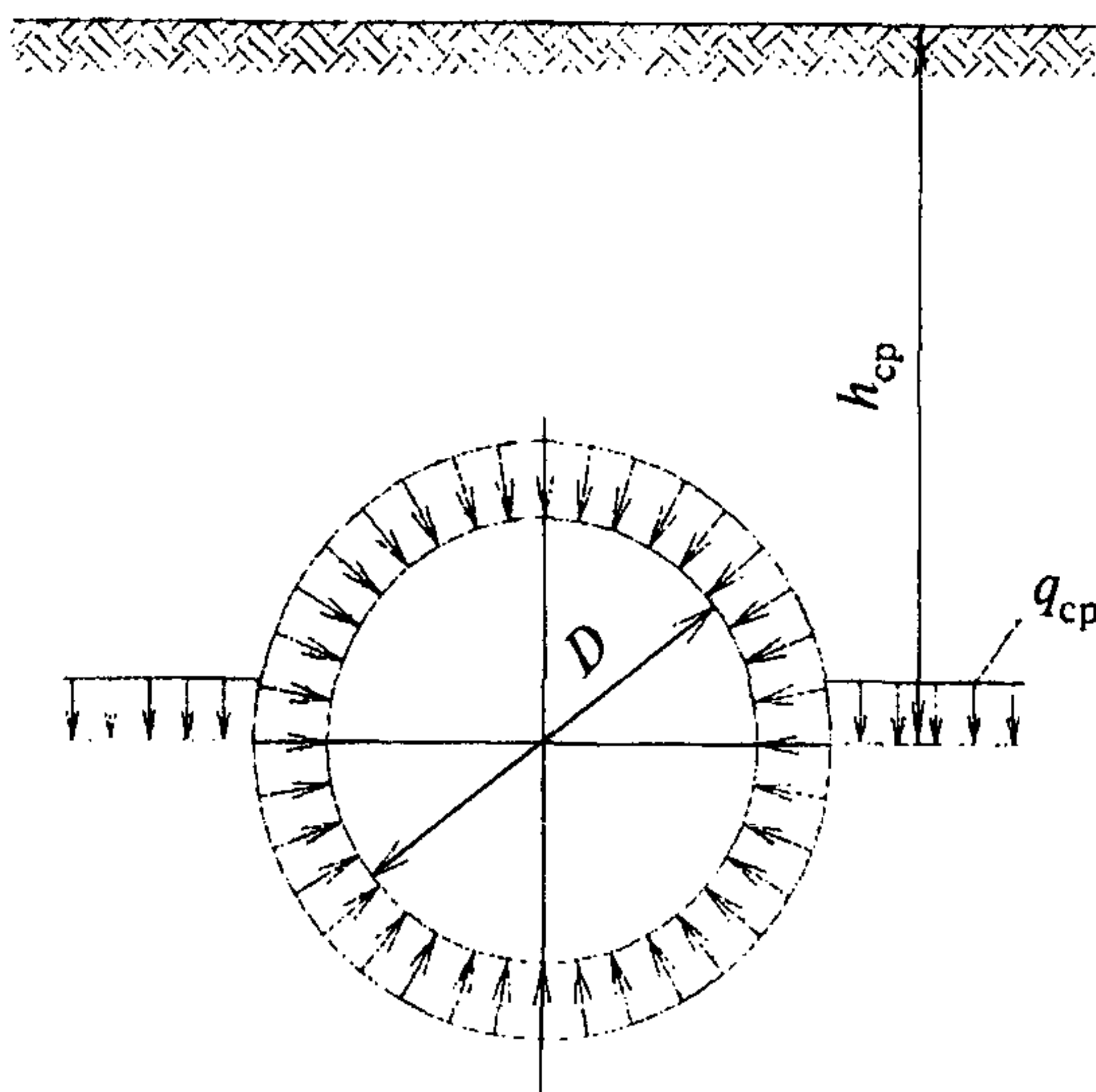
Рисунок 7.1 — Среднее давление грунта на подземный трубопровод
