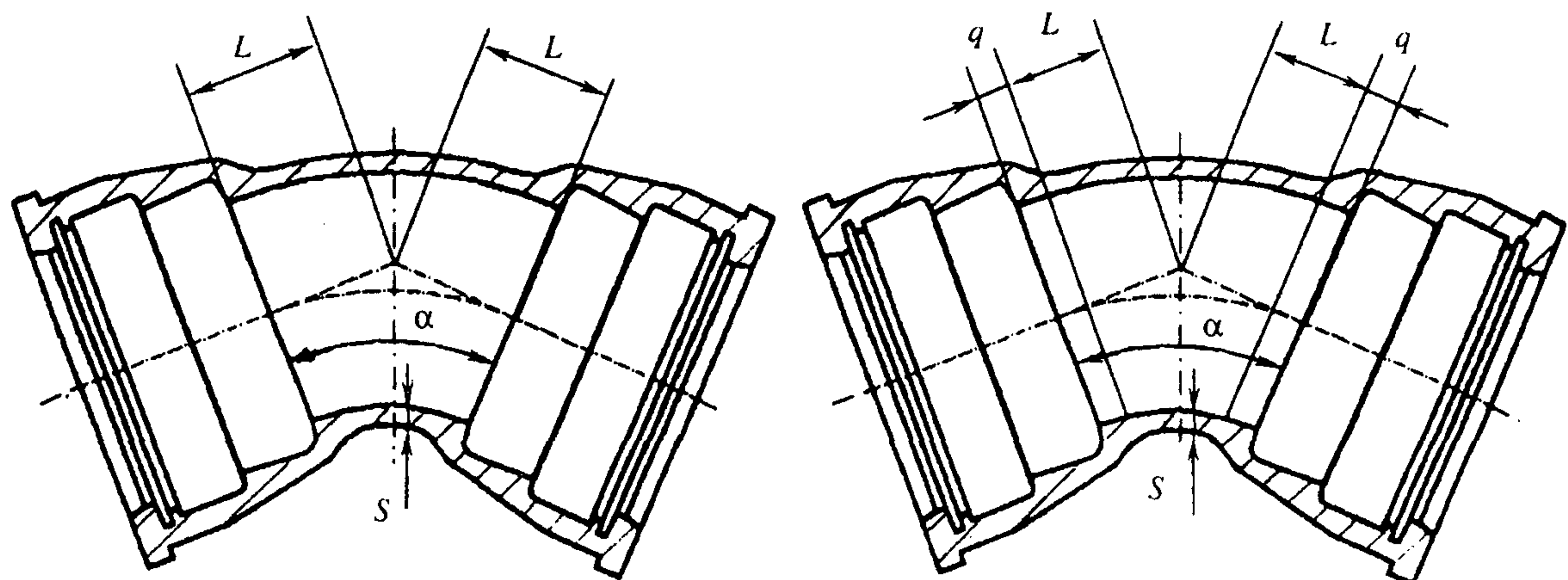
Рисунок Б.11 — Отвод раструбный
