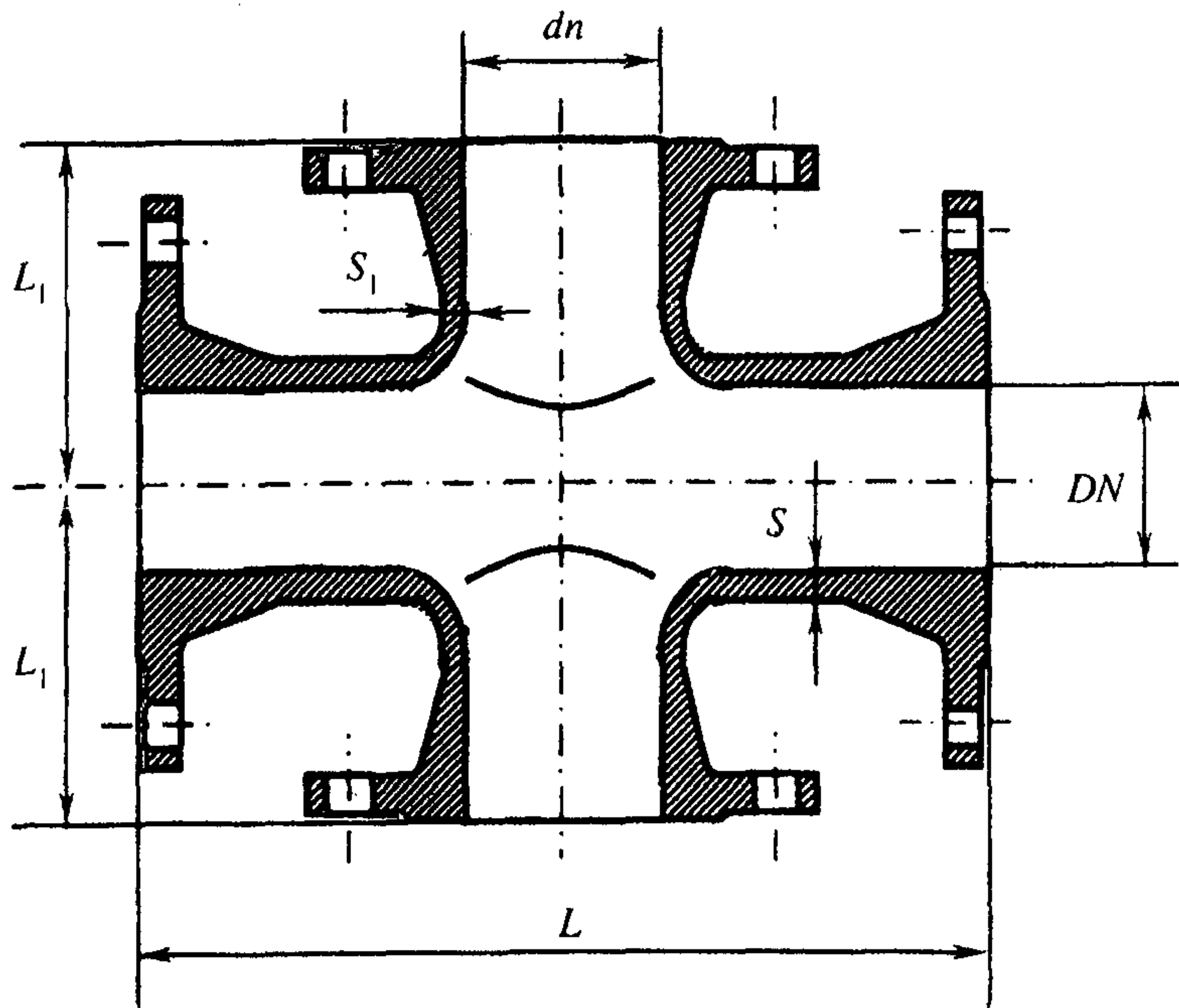
Рисунок Б.29 — Крест фланцевый
