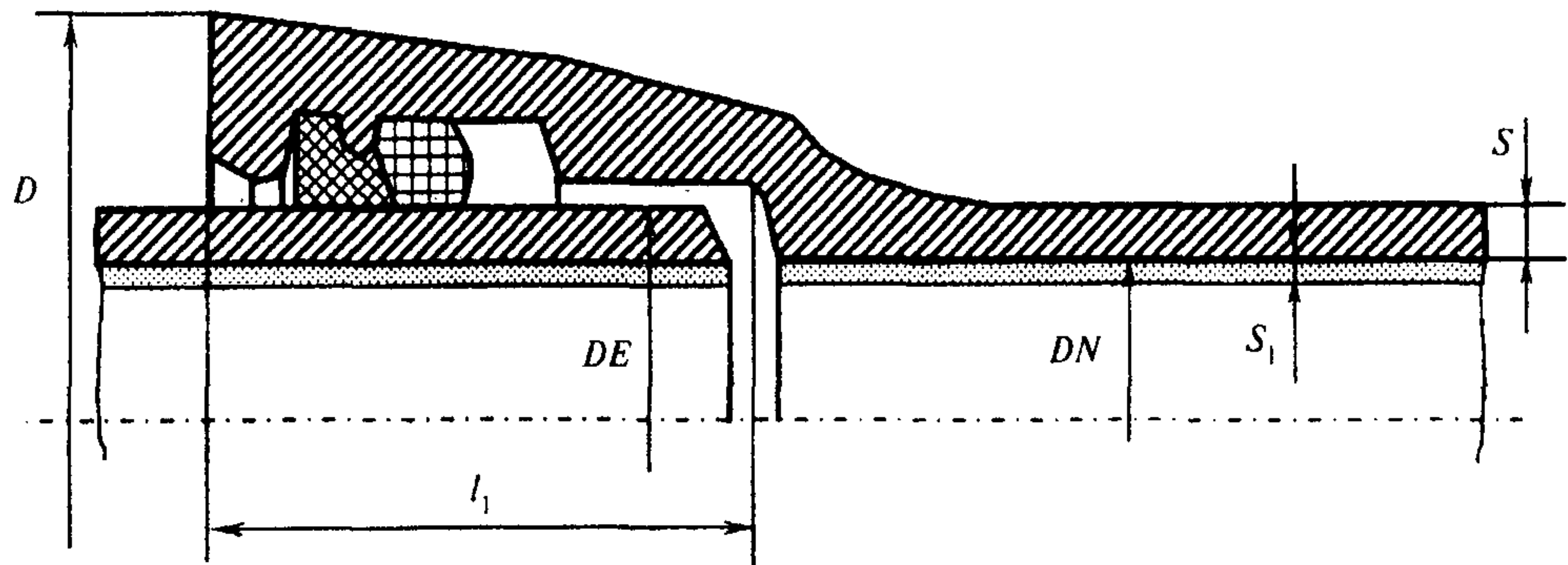
Рисунок Б.2 — Раструбное соединение типа «TYTON»
