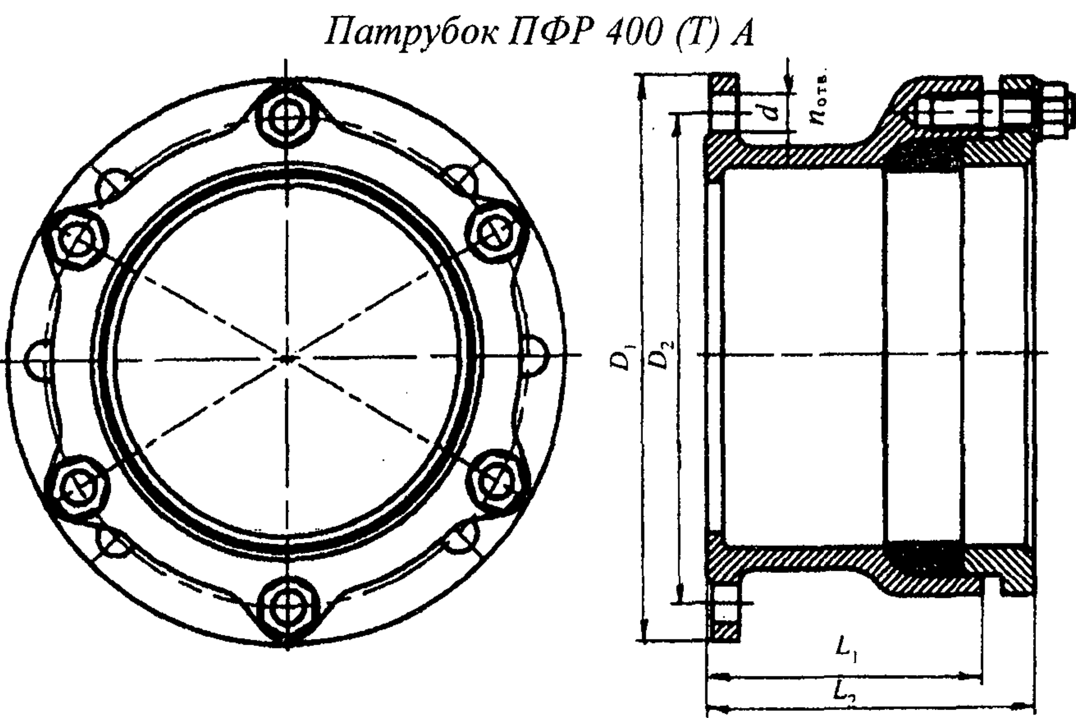
Рисунок Б.18 — Патрубок фланец-раструб компенсационный
