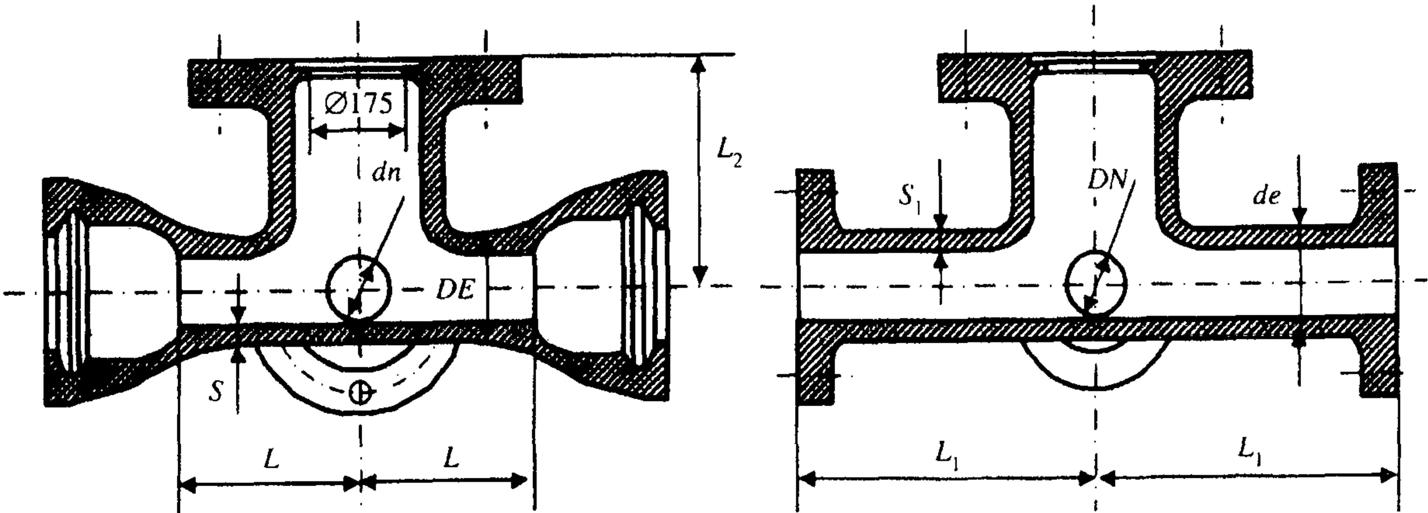
Рисунок Б.30 — Крест раструб-фланец с пожарной подставкой
