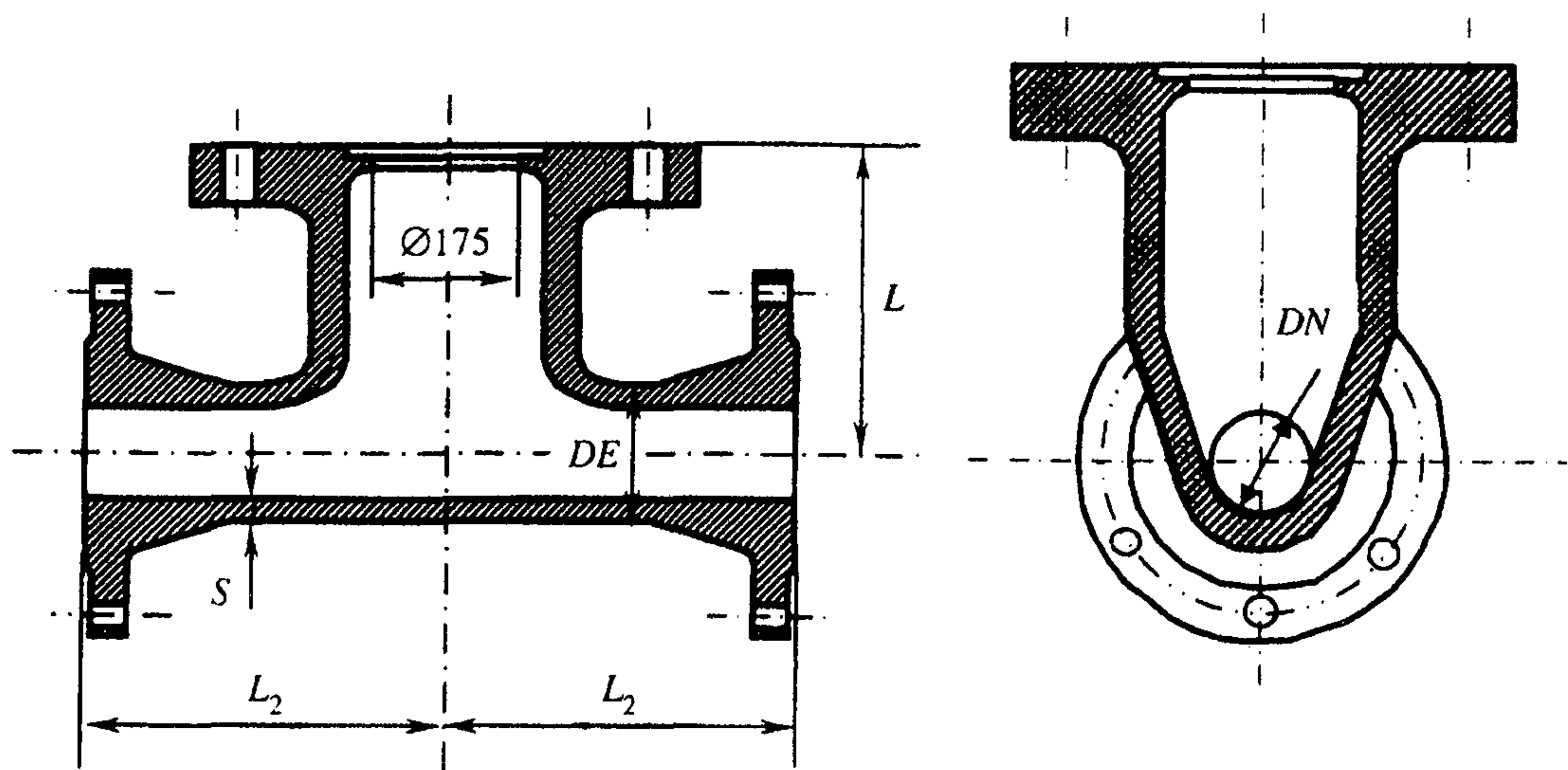
Рисунок Б.35 — Пожарная подставка фланцевая
