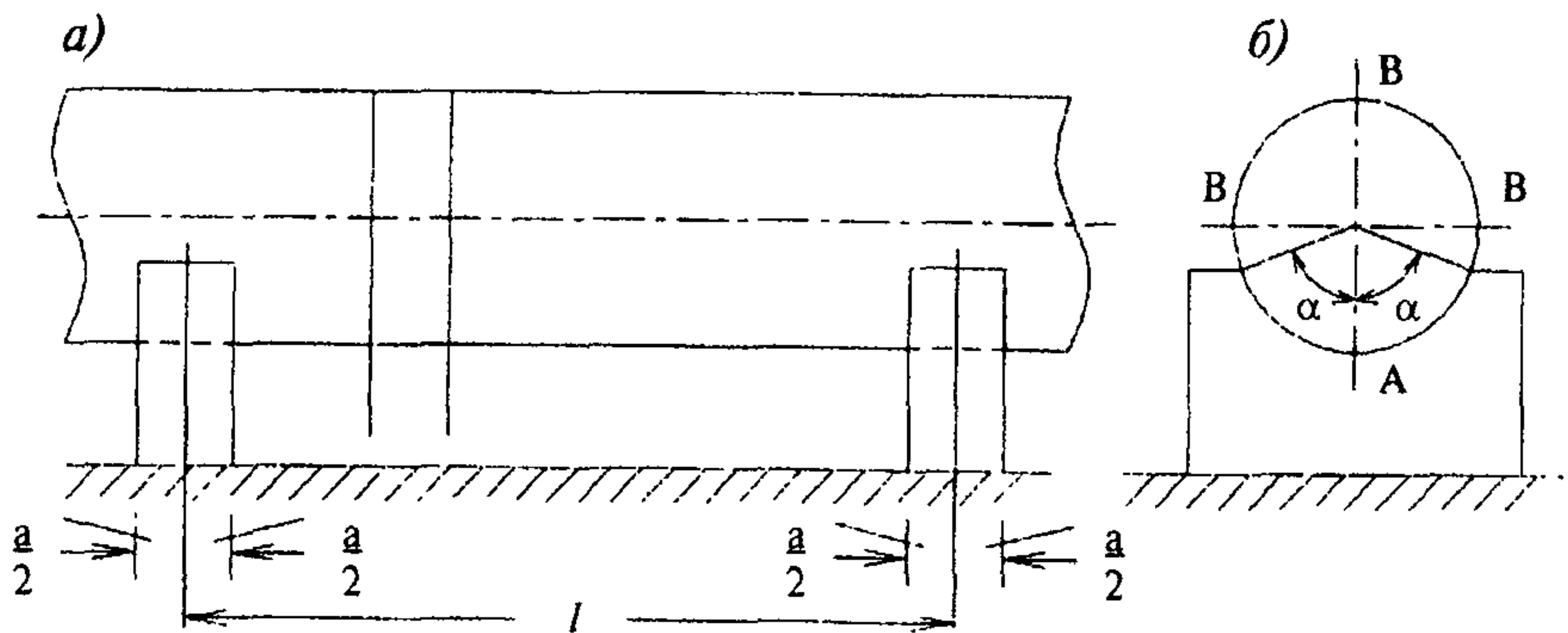
Рисунок 6.2 —Трубопровод на отдельных опорах
