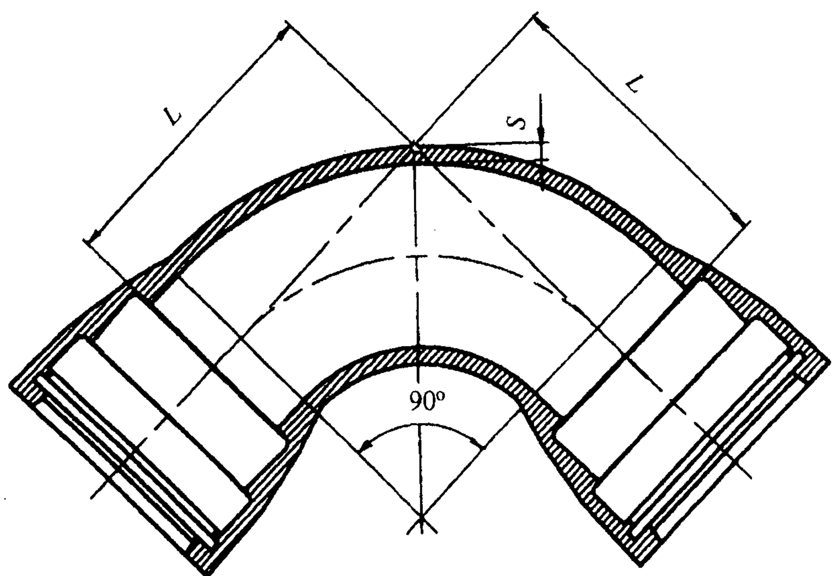
Рисунок Б.9 — Колено раструбное
