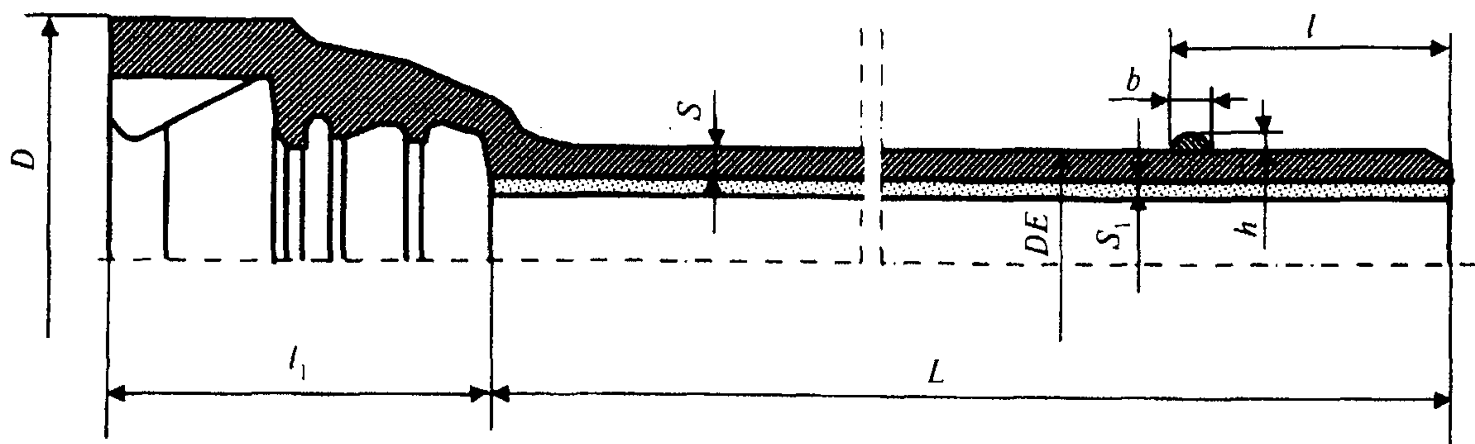
Рисунок А.2 — Труба раструбная под соединение «RJ»
