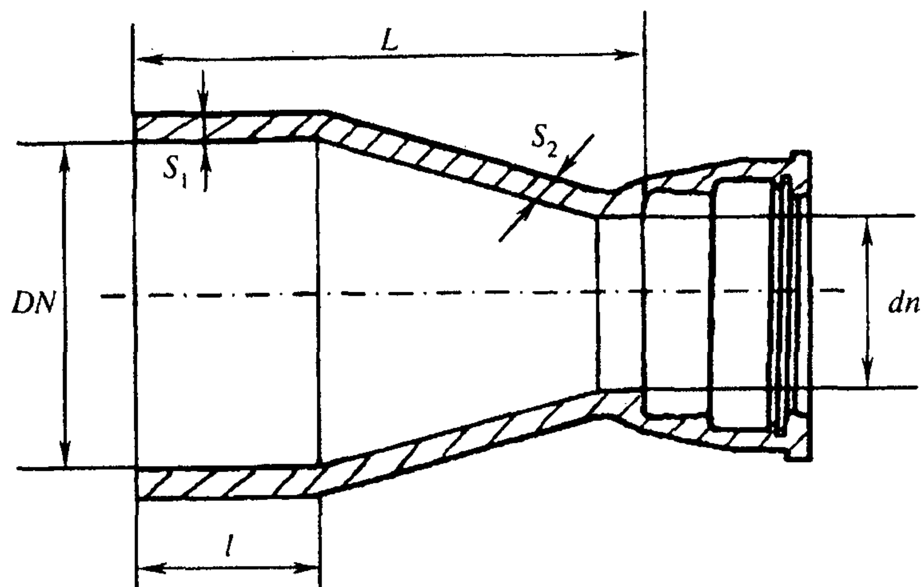
Рисунок Б.13 — Переход раструб — гладкий конец
