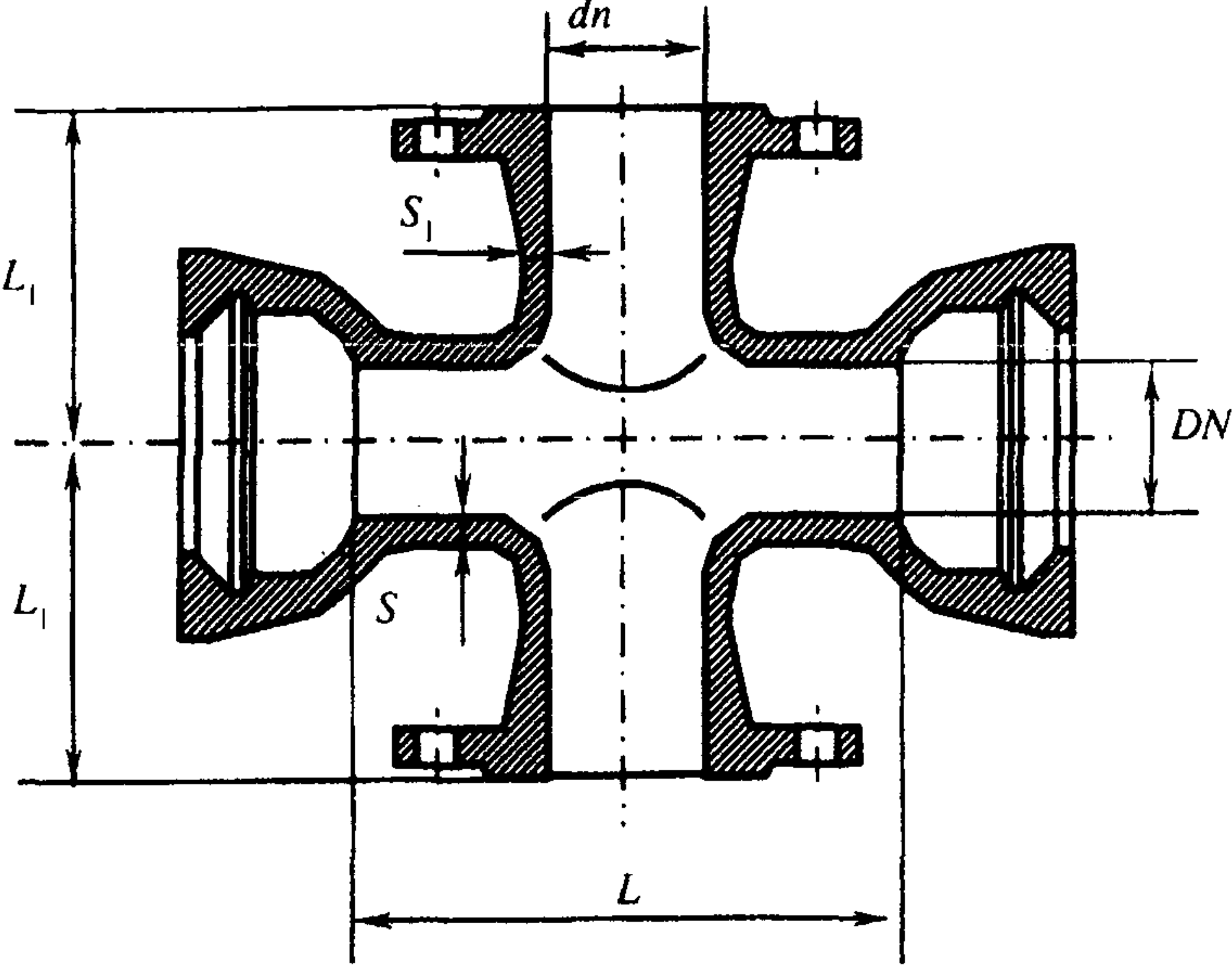
Рисунок Б.27 — Крест раструб-фланец
