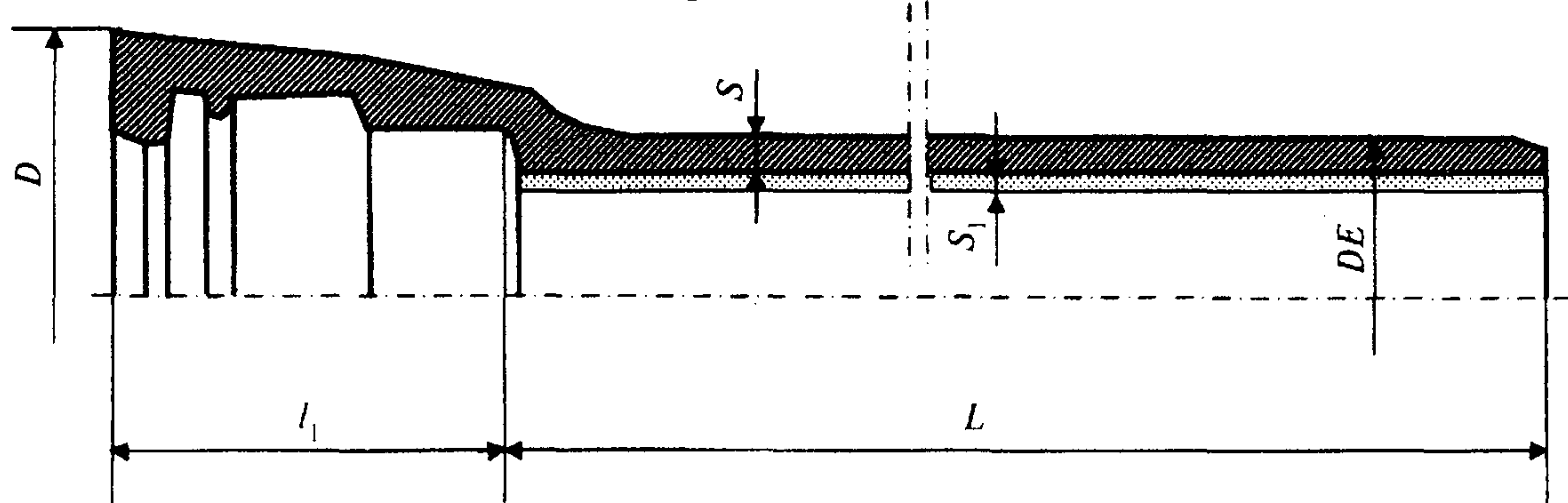
Рисунок А.1 — Труба раструбная под соединение «TYTON»
