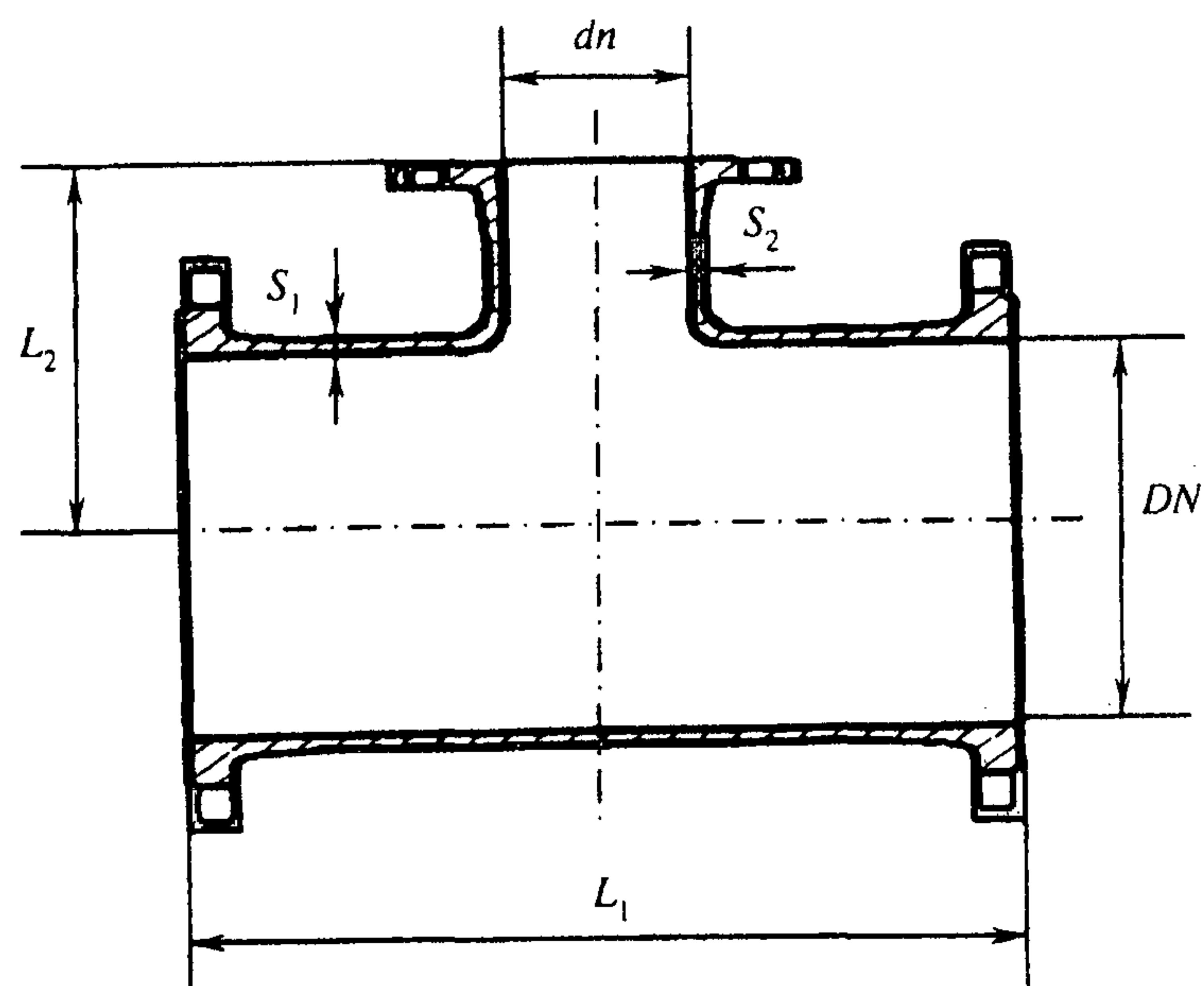
Рисунок Б.6 — Тройник фланцевый
