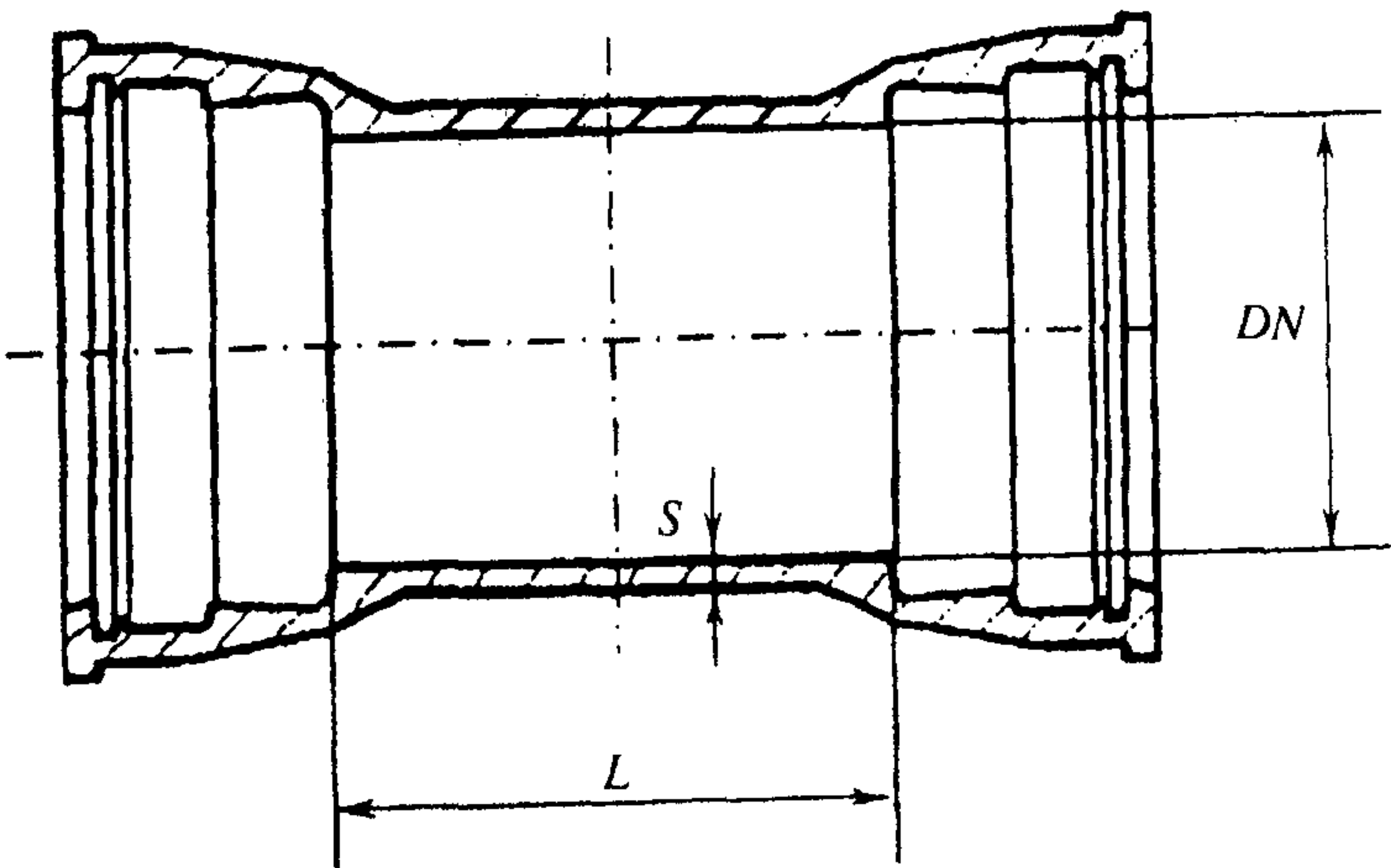
Рисунок Б.20 — Двойной раструб
