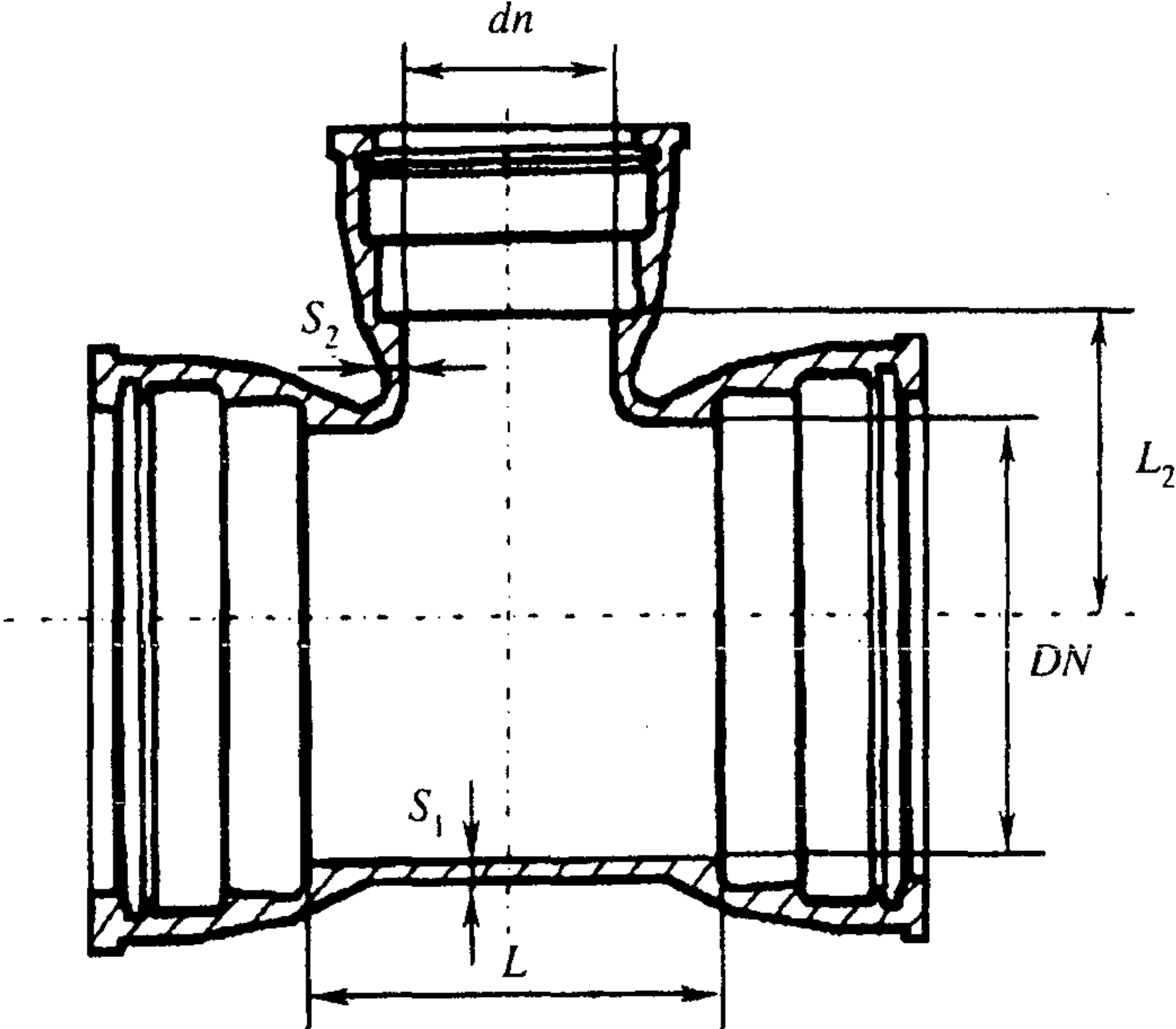
Рисунок Б.5 — Тройник раструбный
