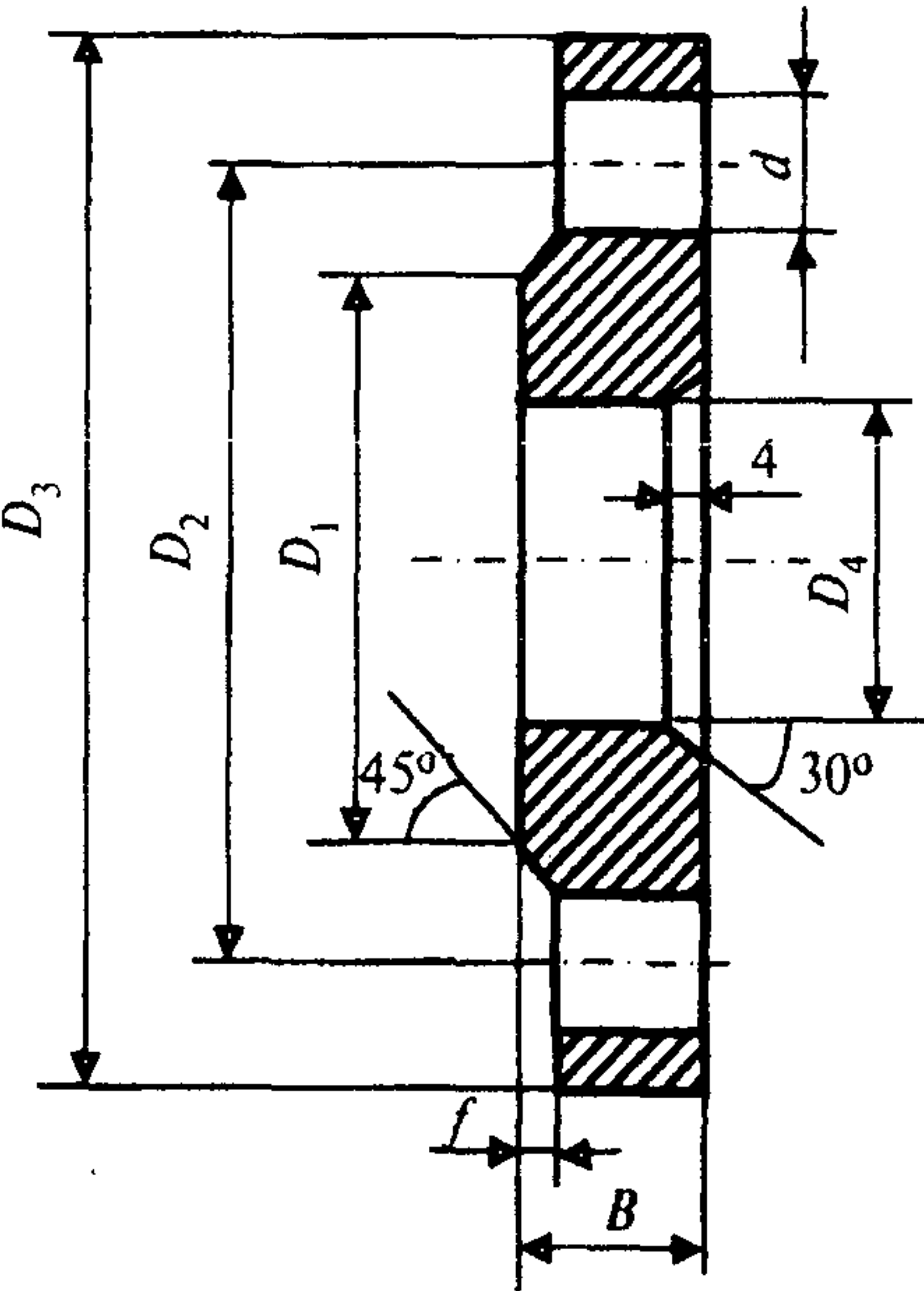
Рисунок А.4 — Фланец из высокопрочного чугуна
