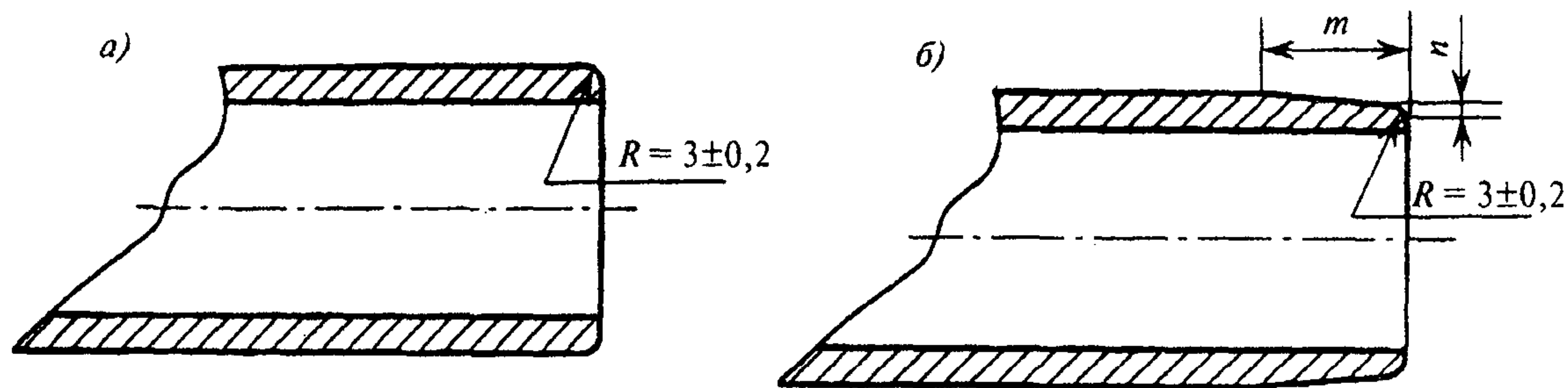
a — радиус; б — фаска с переходом на радиус Рисунок А.5 — Торец гладкого конца трубы
