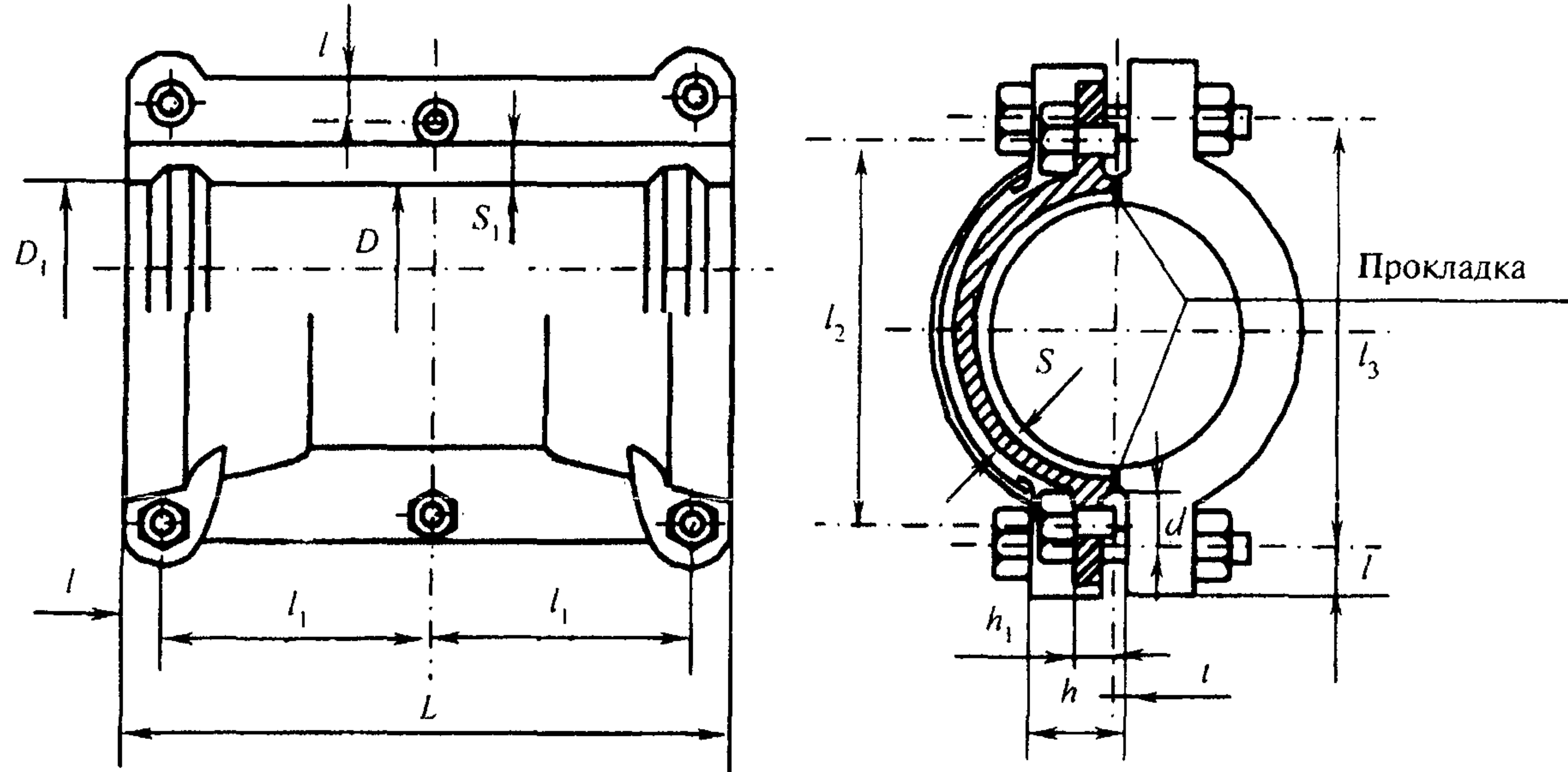
Рисунок Б.32 — Муфта свертная
