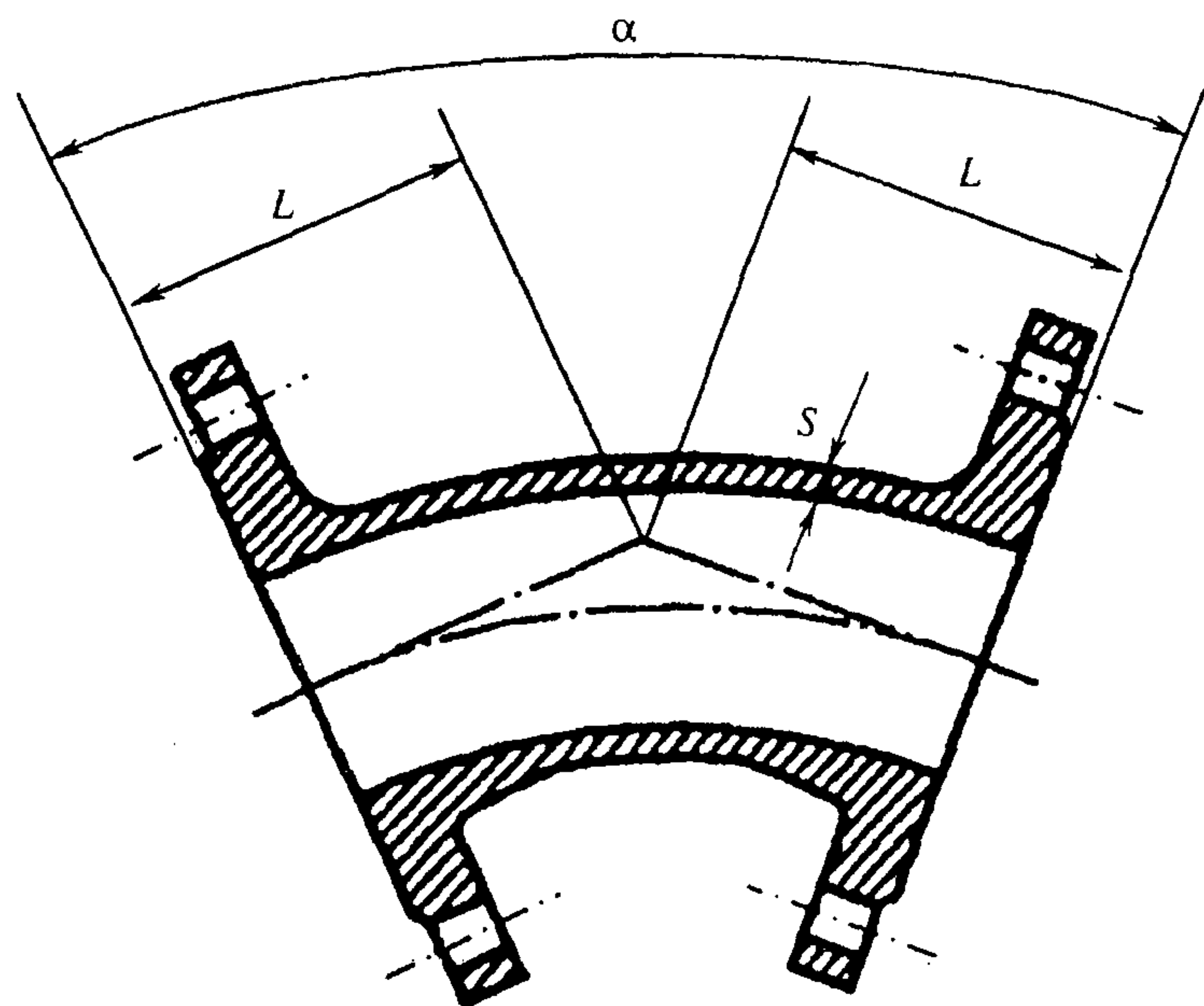
Рисунок Б.12 — Отвод фланцевый
