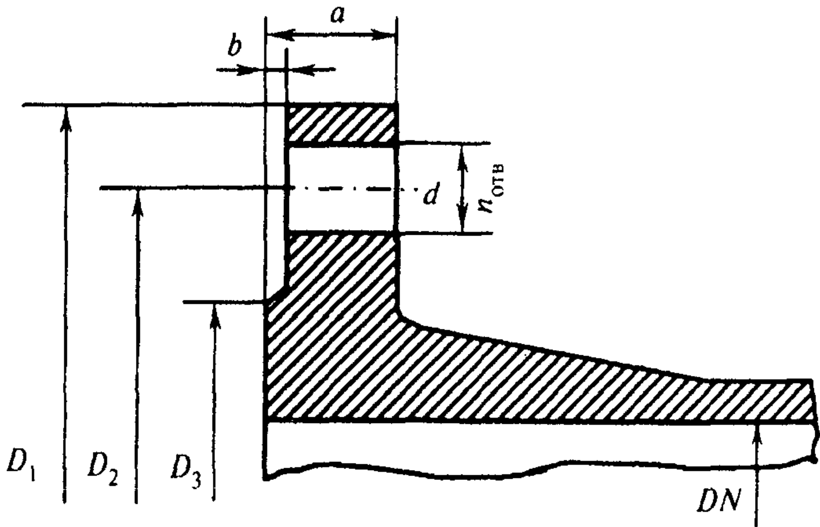
Рисунок Б.3 — Фланец
