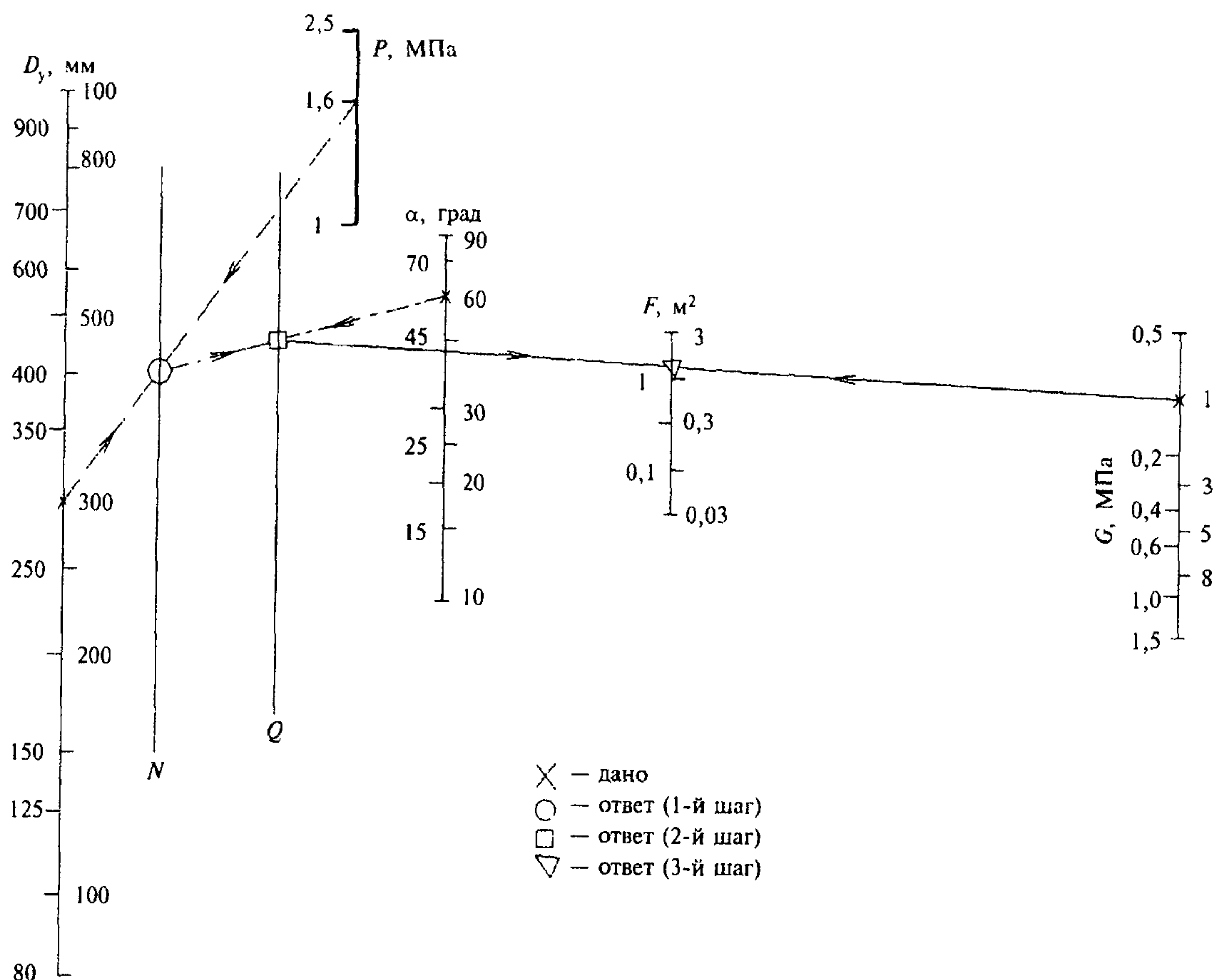
Рисунок 5.10 — Номограмма для выбора опорной площади упоров F на напорном трубопроводе условным диаметром D_y из труб из высокопрочного чугуна с шаровидным графитом с раструбными соединениями, находящегося под внутренним давлением P , при угле поворота трассы \alpha с опорой на грунт прочностью G ( N и Q — промежуточные шкалы)
