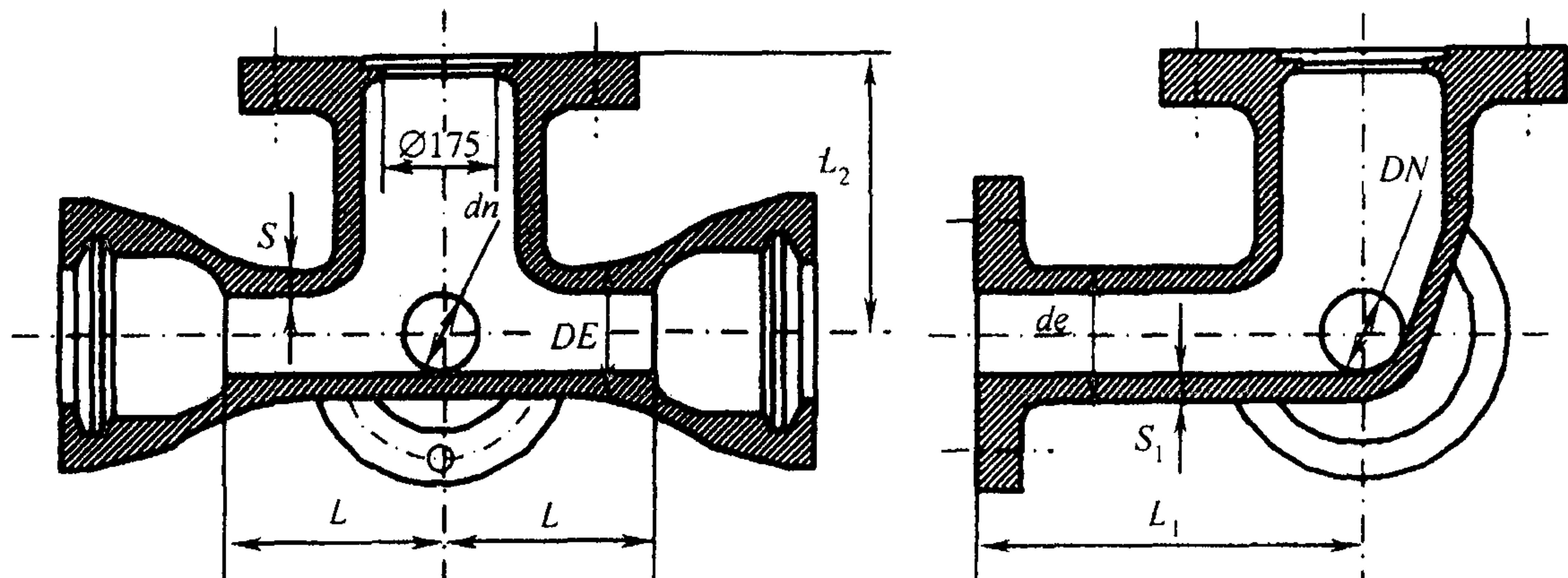
Рисунок Б.25 — Тройник раструб-фланец с пожарной подставкой
