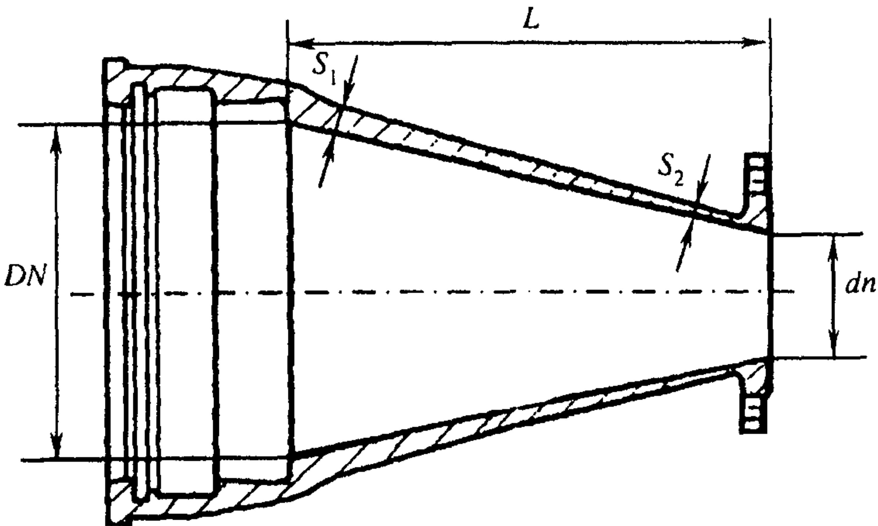
Рисунок Б.14 — Переход раструб-фланец
