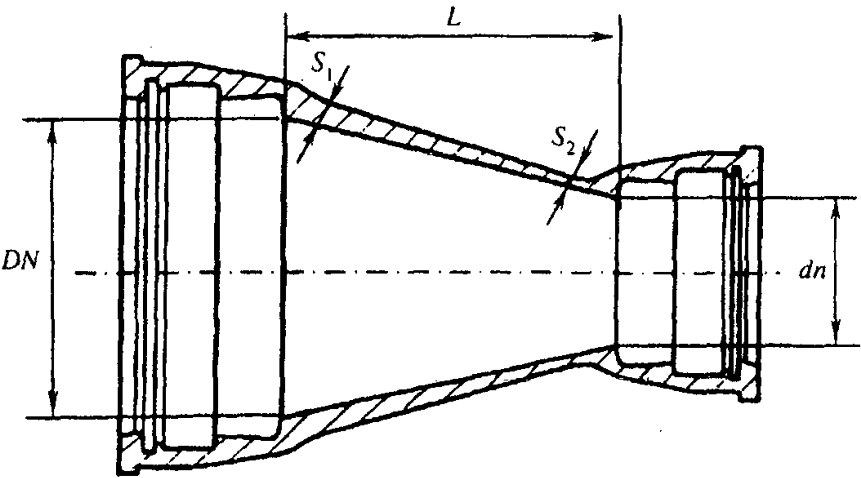
Рисунок Б.16 — Переход раструбный
