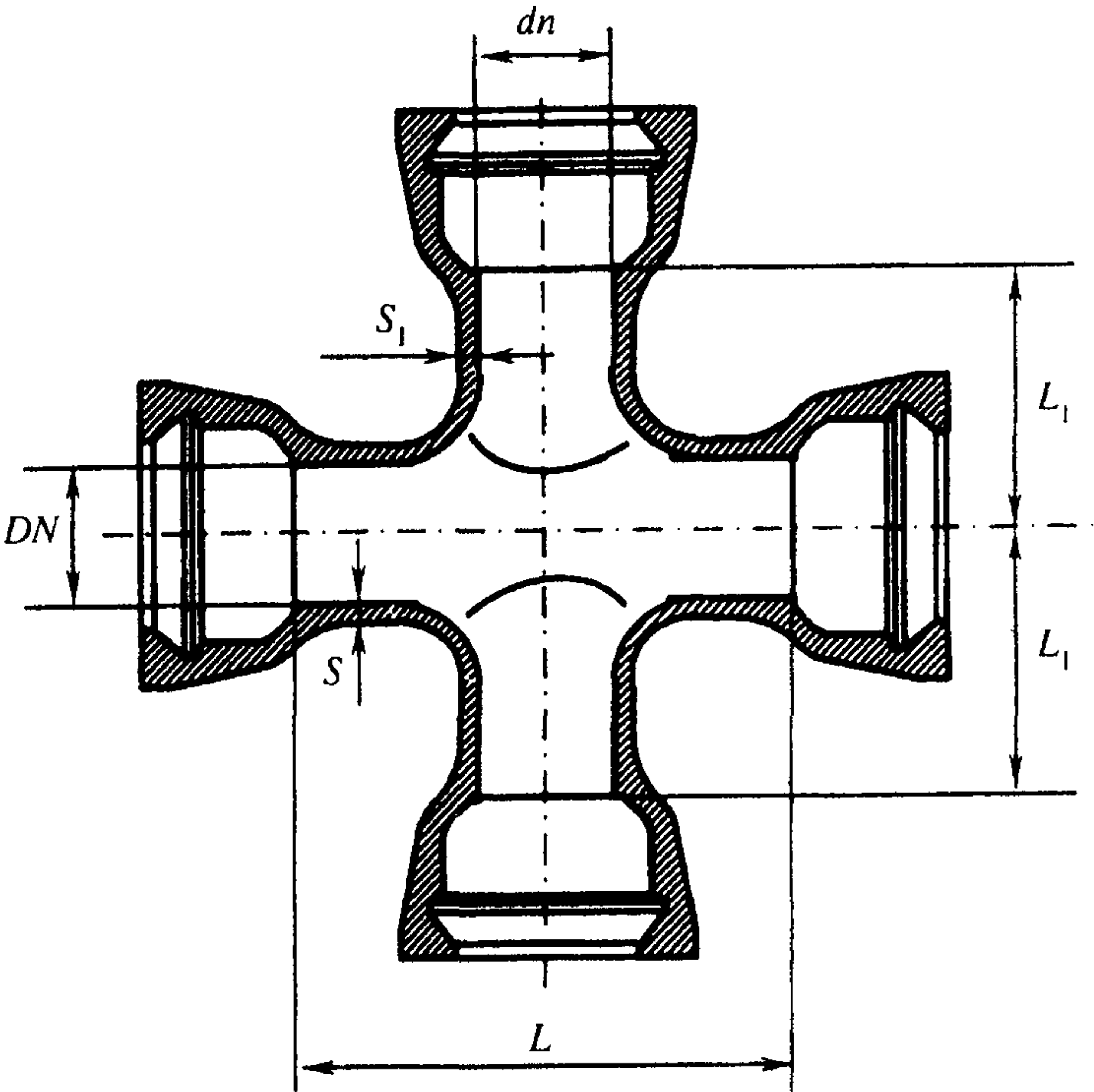
Рисунок Б.28 — Крест раструбный
