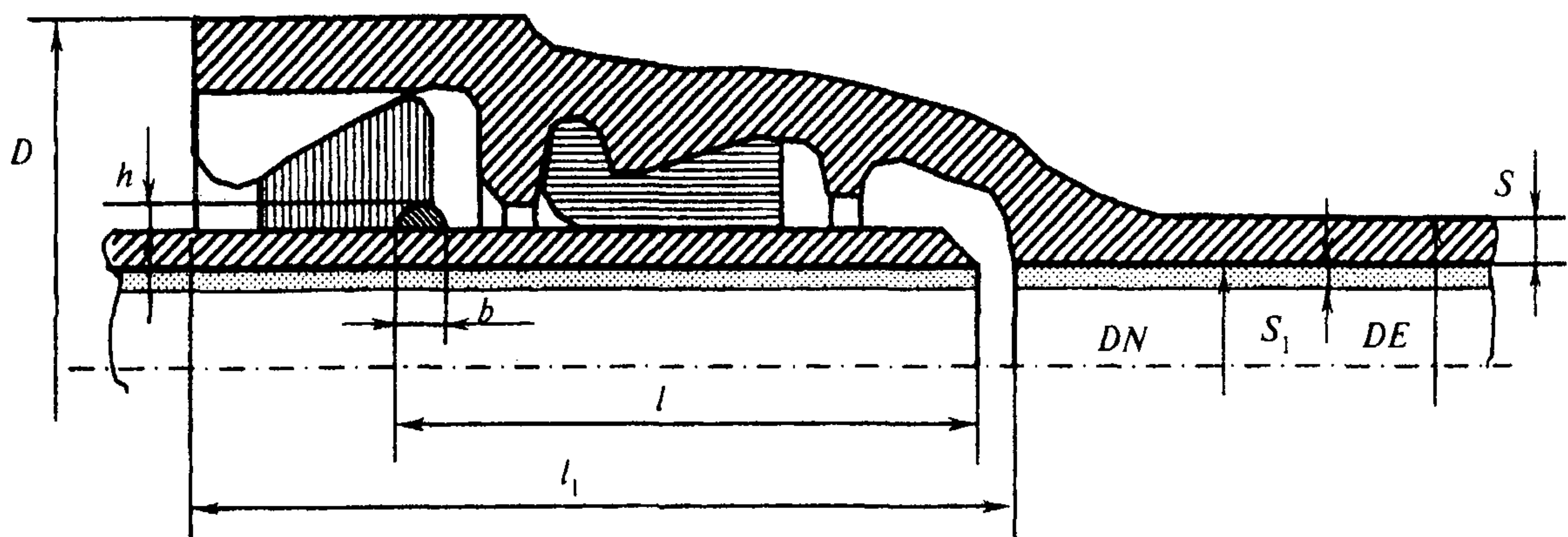
Рисунок Б.1 — Раструбное соединение типа «RJ»
