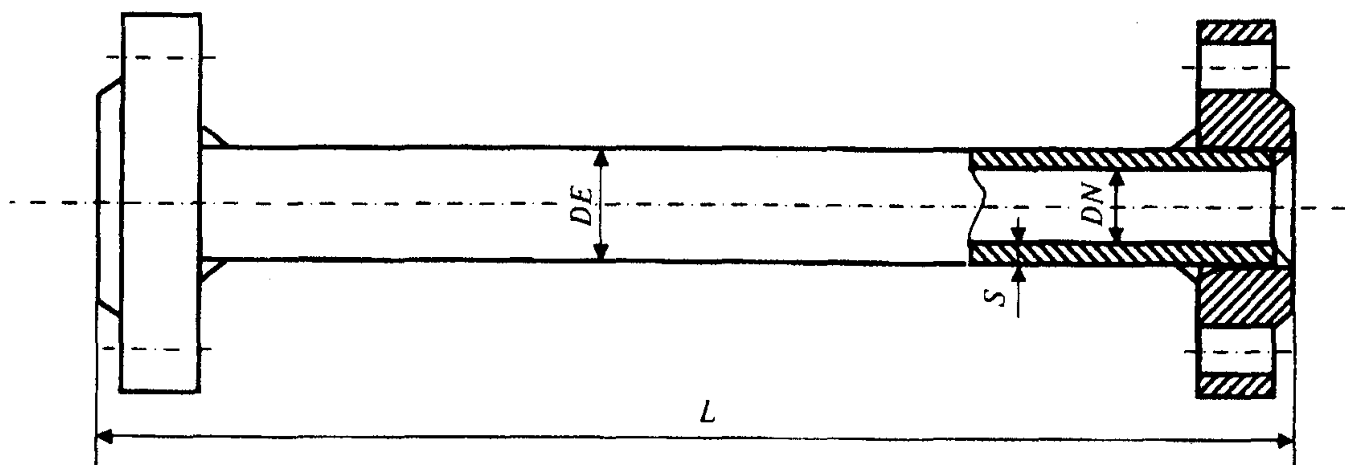
Рисунок А.3 — Труба с приваренными фланцами
