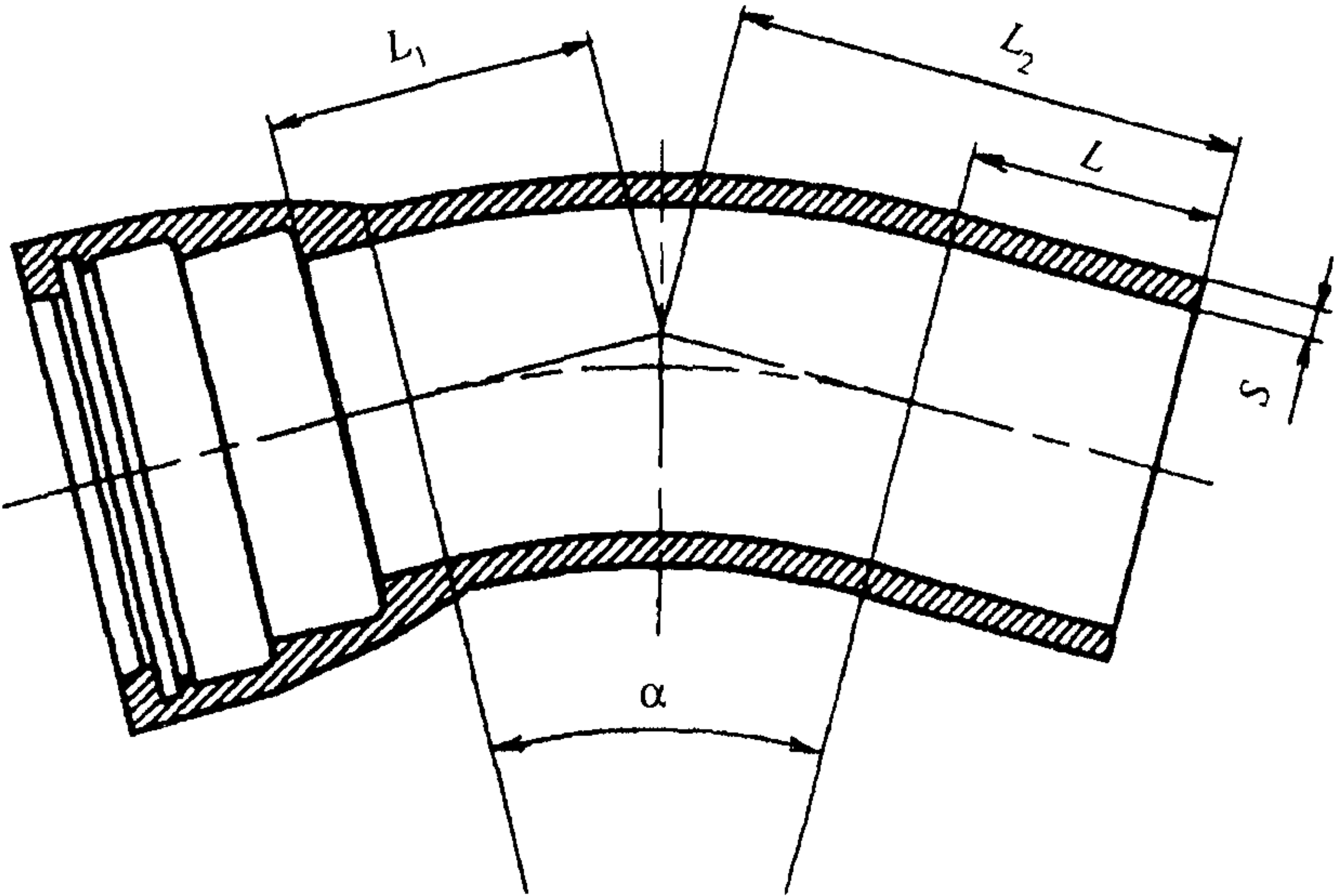
Рисунок Б.10 — Отвод раструб — гладкий конец
