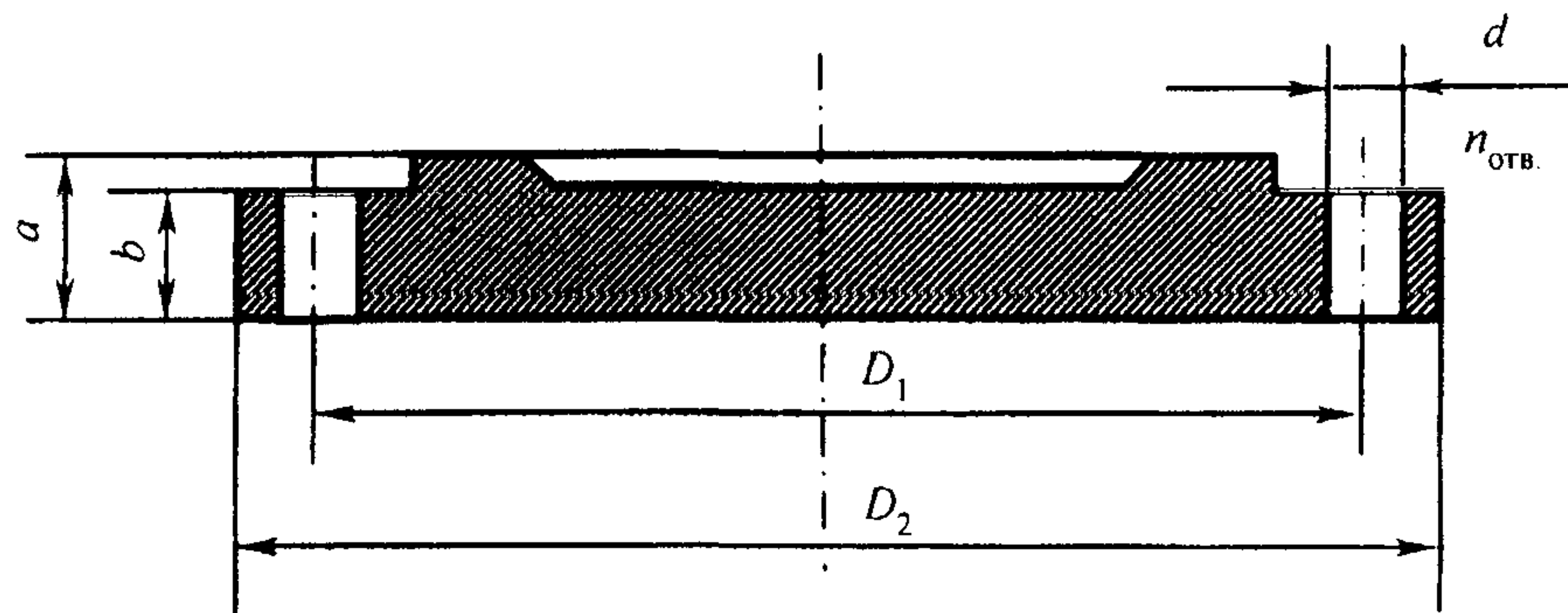
Рисунок Б.34 — Заглушка фланцевая
