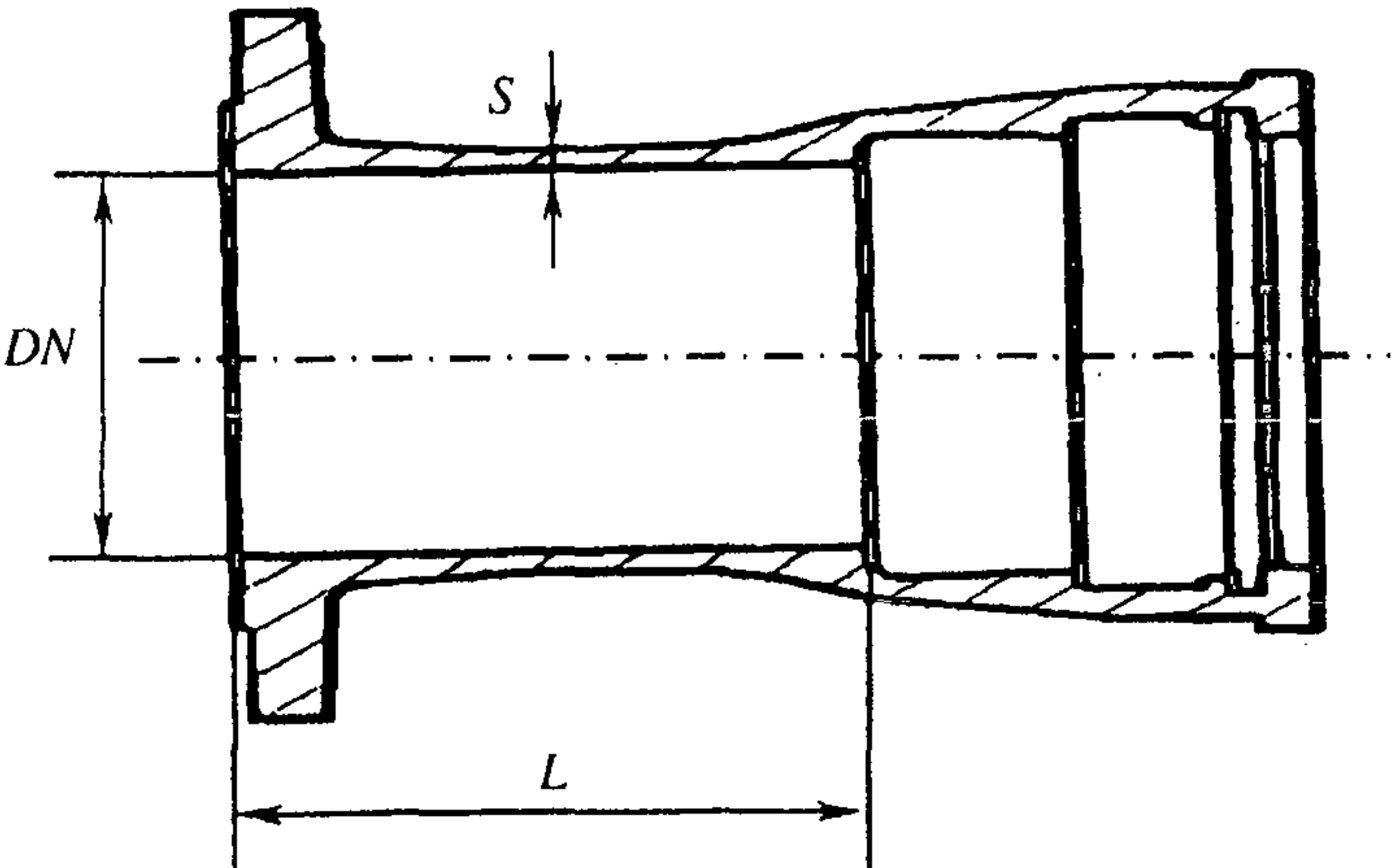
Рисунок Б.17 — Патрубок фланец-раструб
