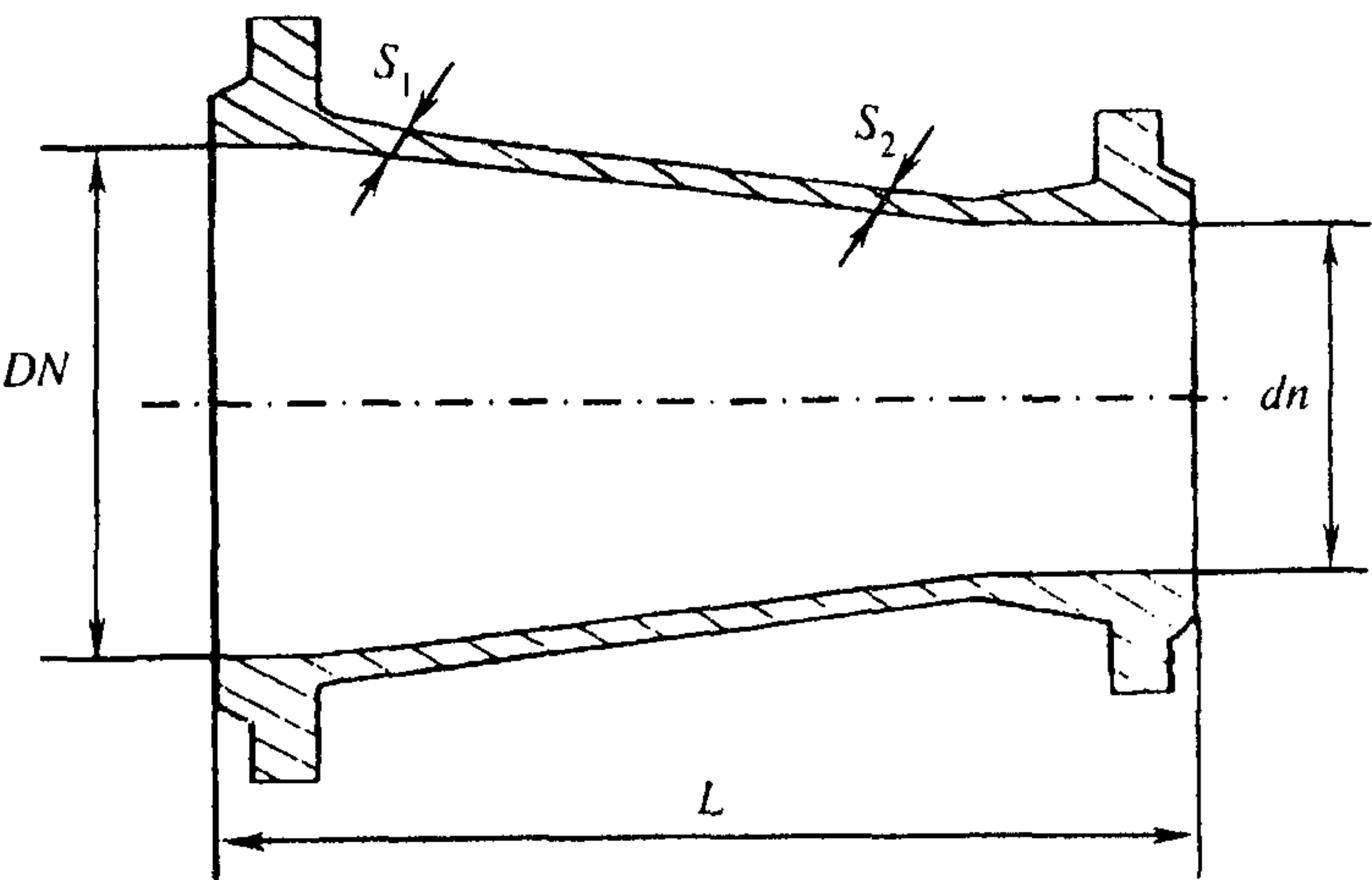
Рисунок Б.15 — Переход фланцевый
