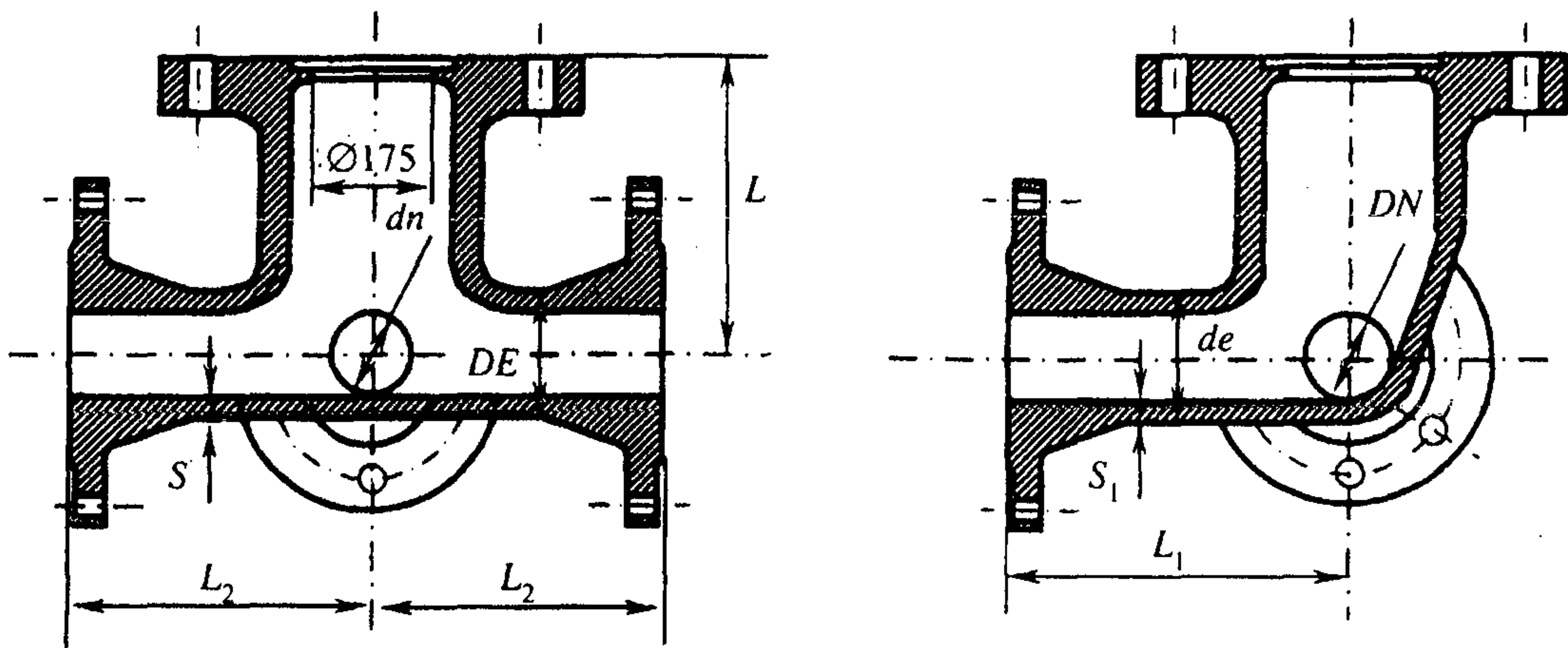
Рисунок Б.26 — Тройник фланцевый с пожарной подставкой
