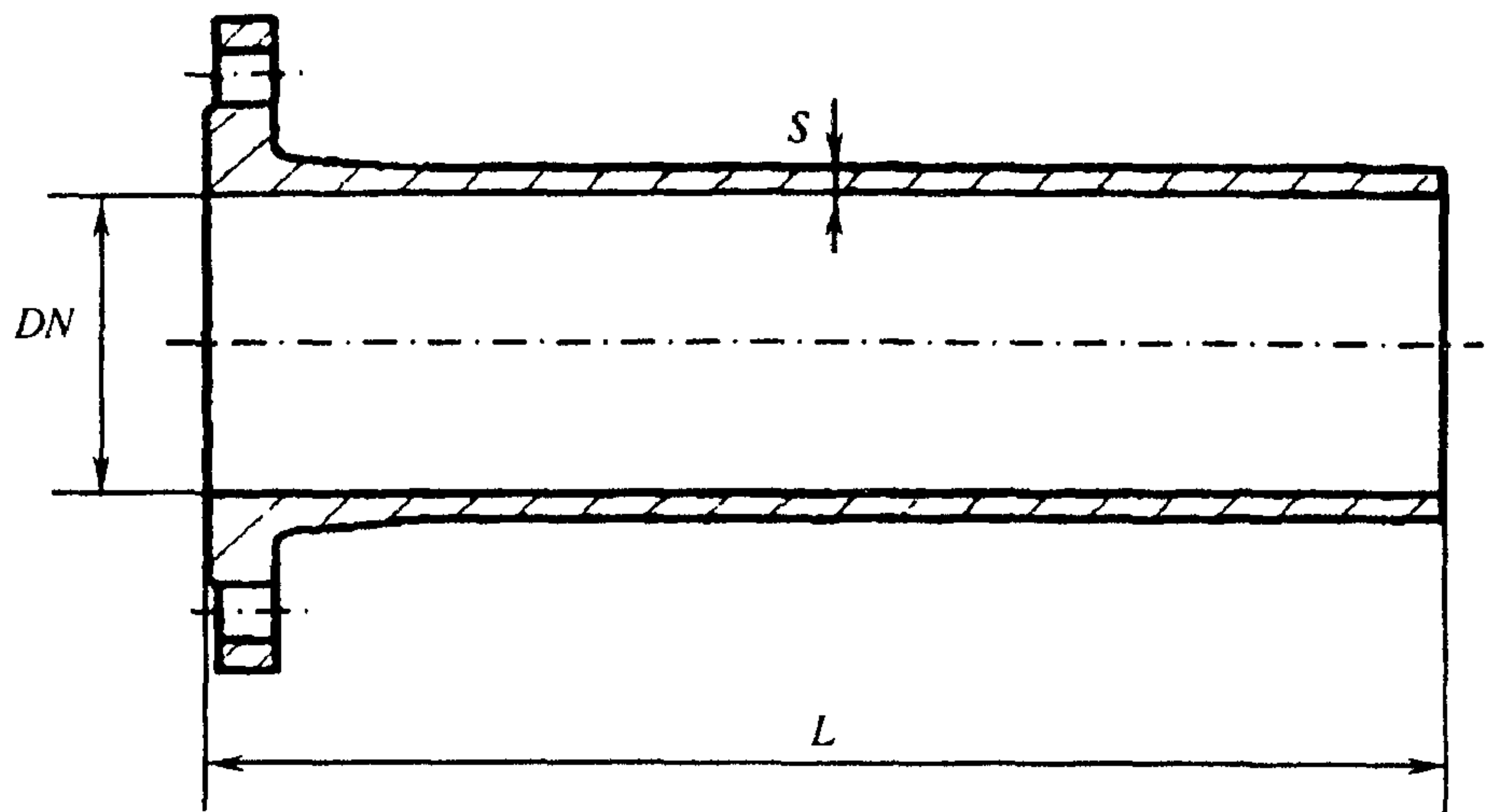
Рисунок Б.19 — Патрубок фланец — гладкий конец
