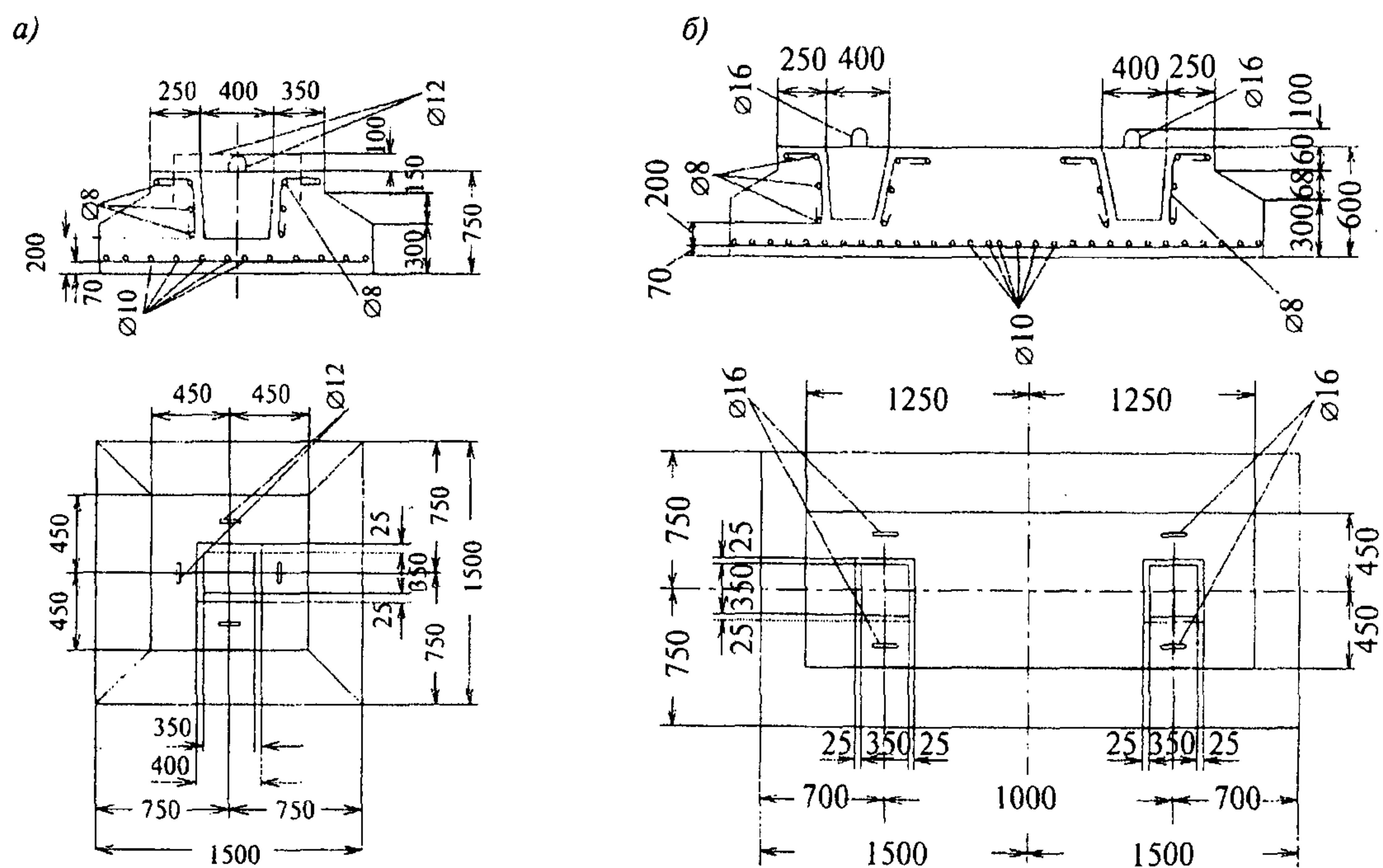
Рисунок 6.5 — Опорные железобетонные башмаки для труб диаметрами 400—500 мм под одну стойку (а), под две стойки (б)
