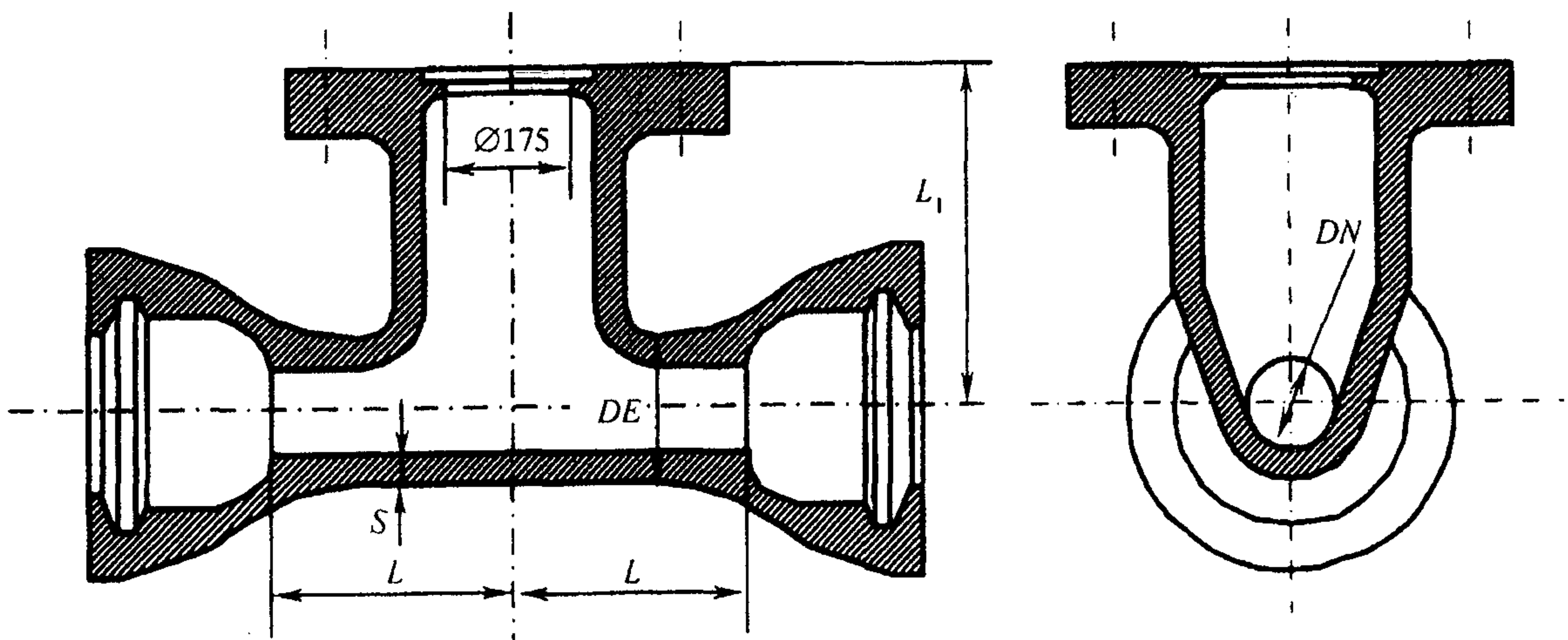
Деталь построения фланца под пожарный кран
