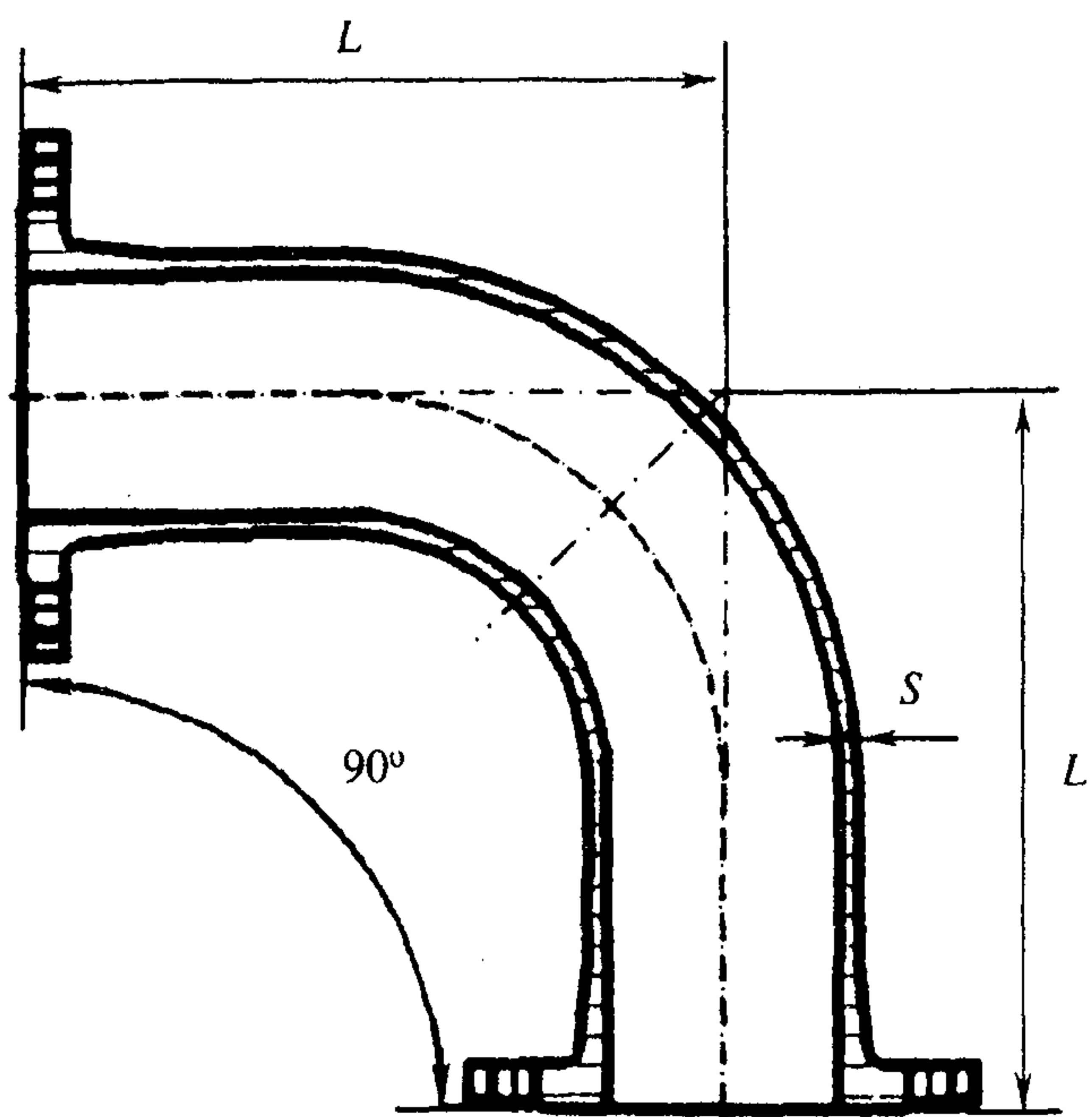
Рисунок Б.8 — Колено фланцевое
