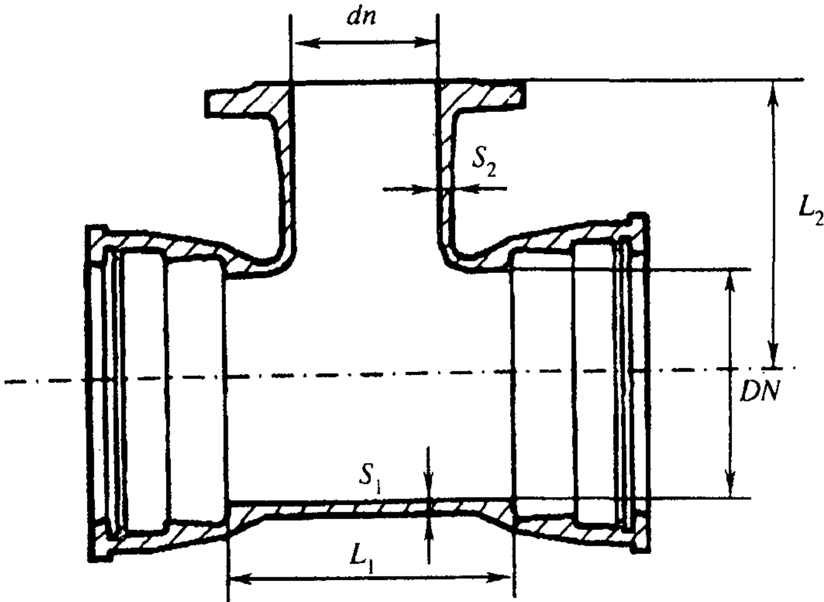
Рисунок Б.4 — Тройник раструб-фланец
