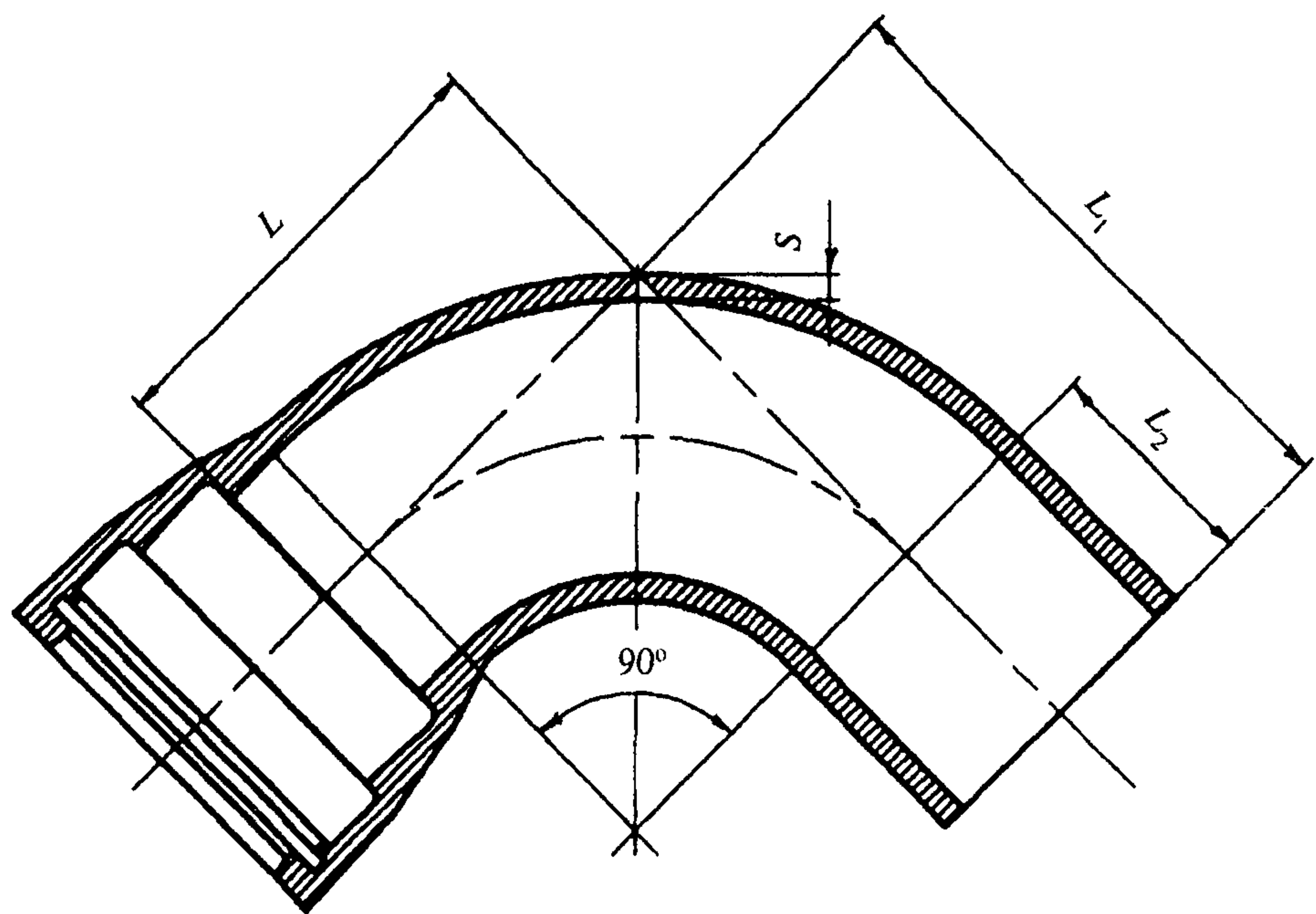
Рисунок Б.7 — Колено раструб — гладкий конец
