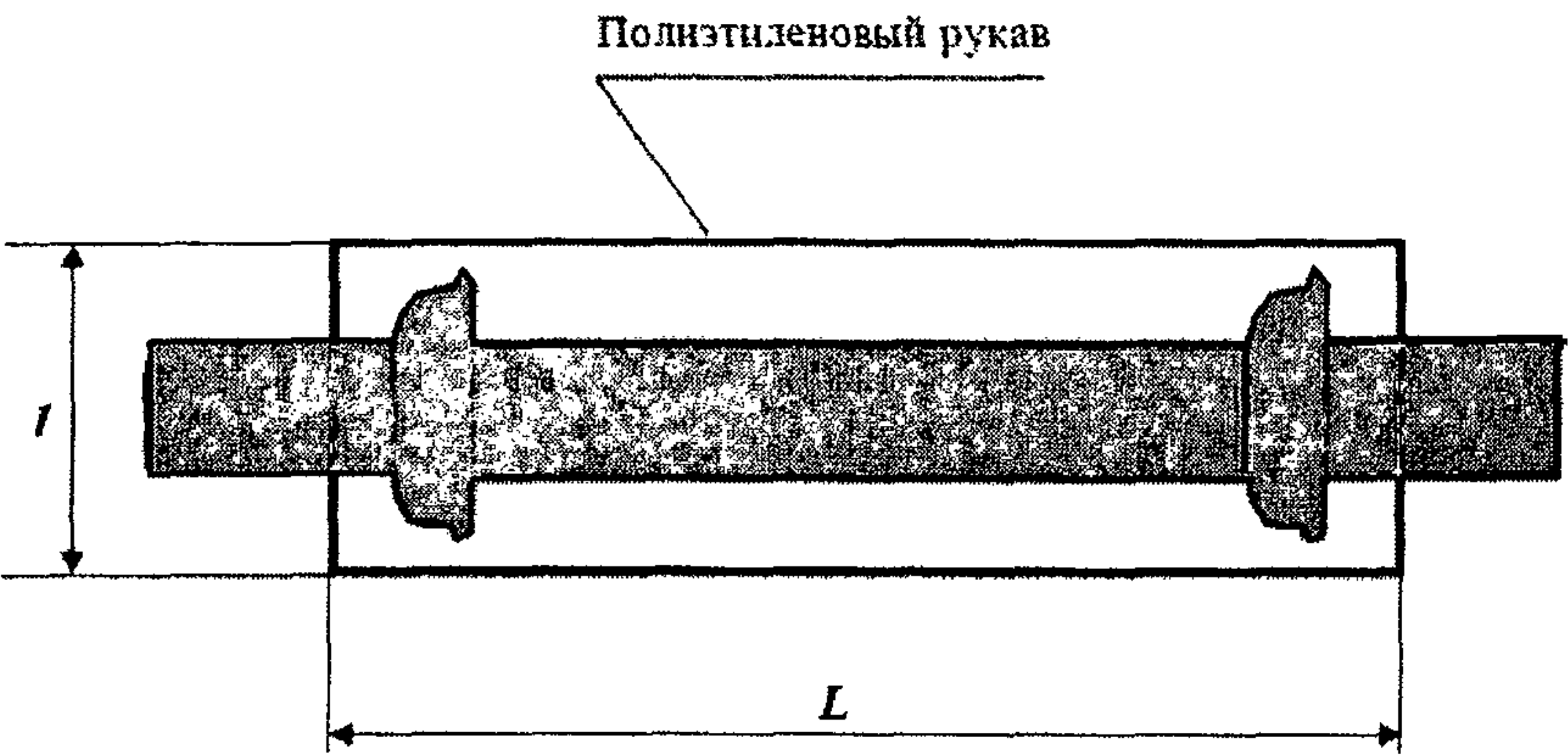
Рисунок 5.7 — Полиэтиленовый рукав для труб
