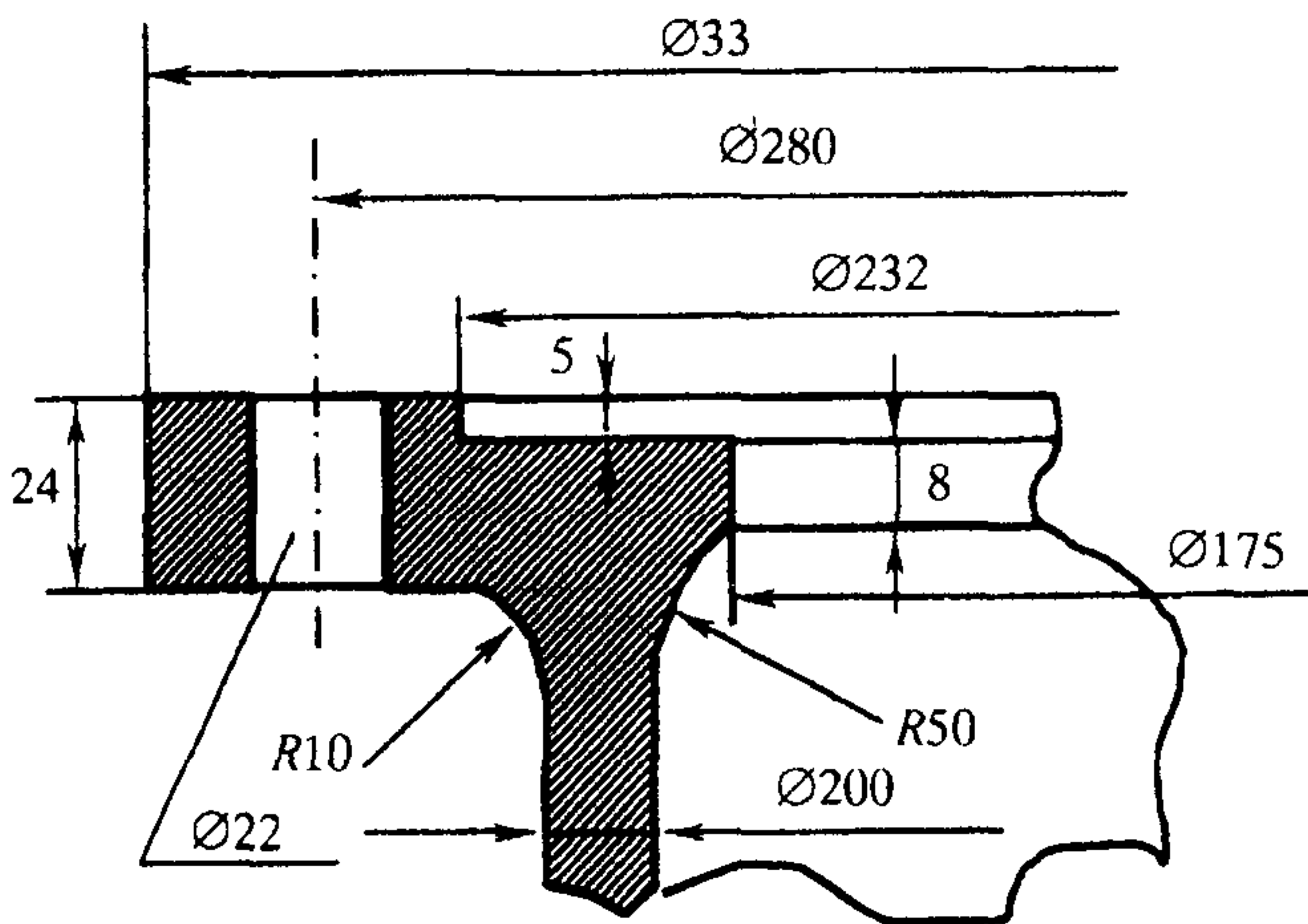
Рисунок Б.24 — Пожарная подставка раструбная
