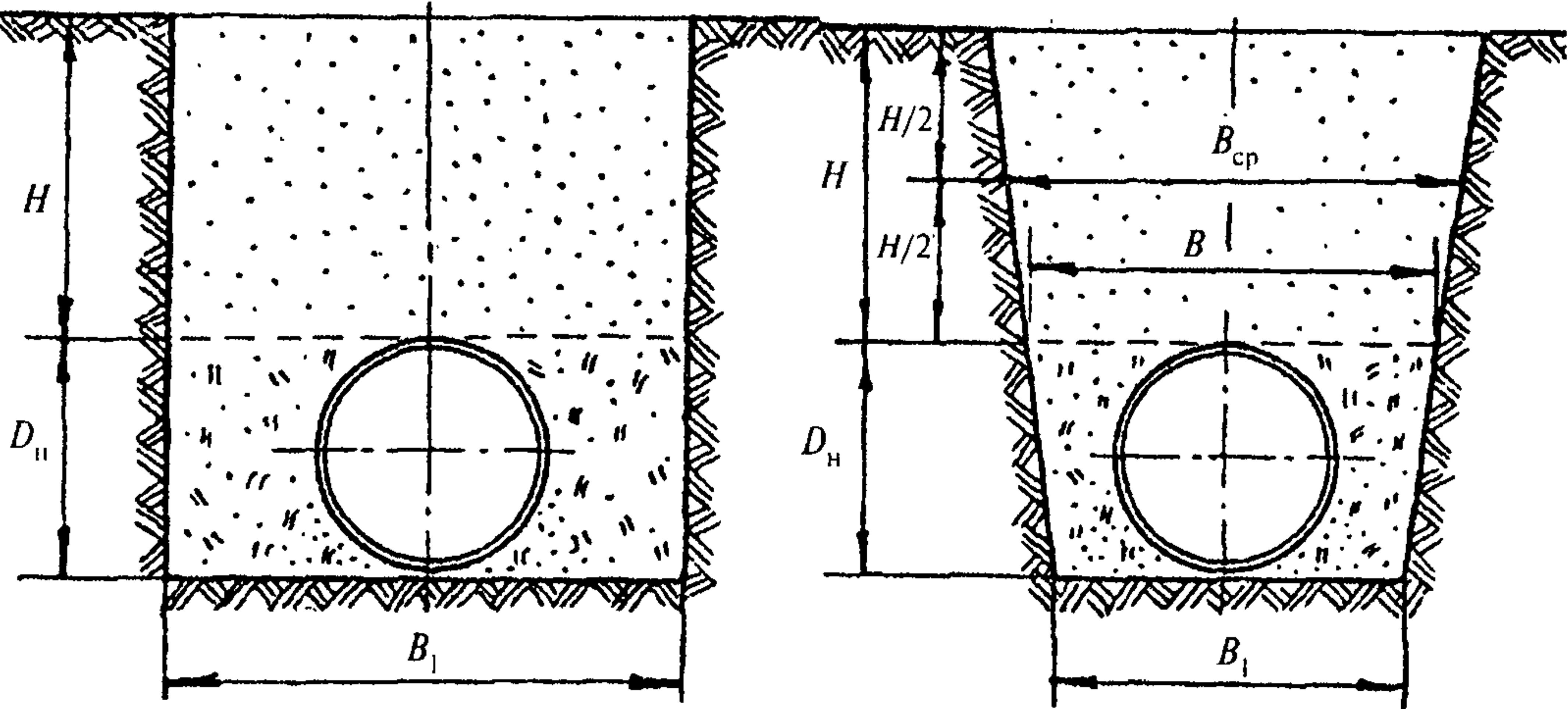
Рисунок 5.5 — Схемы укладки подземного трубопровода
