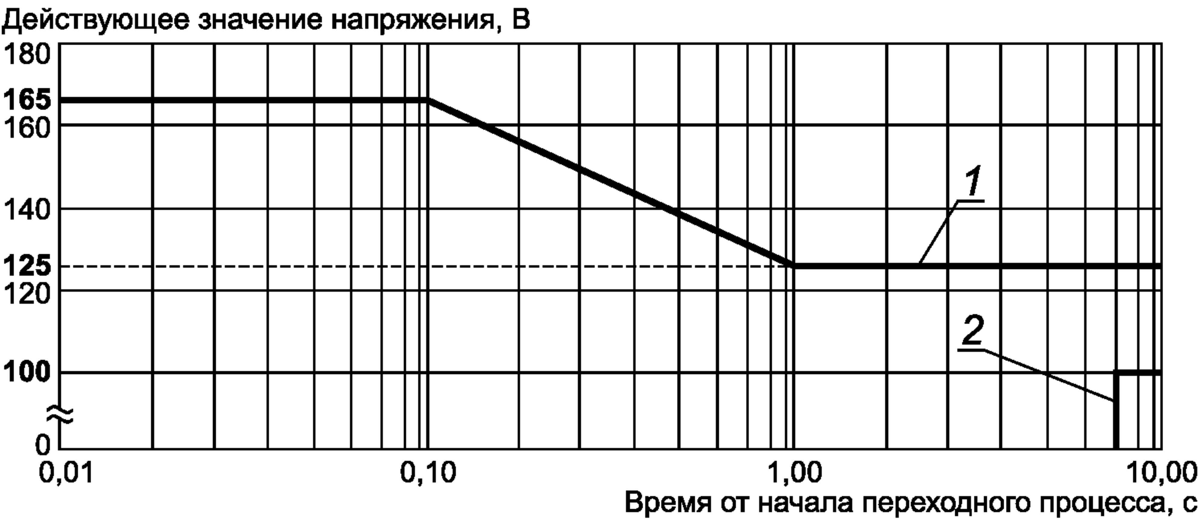
1 — верхний предел действующего значения напряжения; 2 — нижний предел действующего значения напряжения
