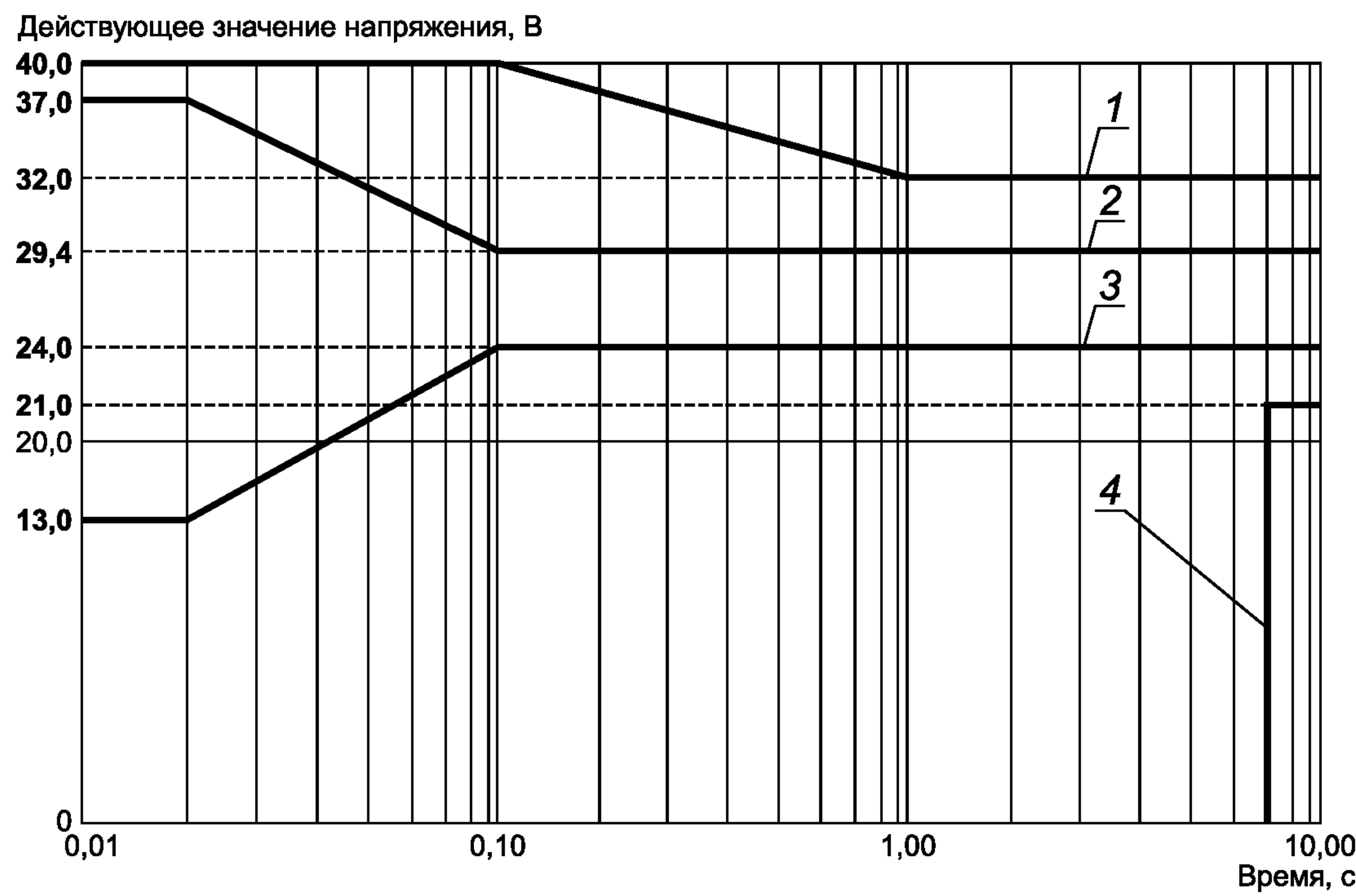
1 и 4 — верхний и нижний пределы при ненормальной работе СЭС; 2 и 3 — верхний и нижний пределы при нормальной или частичной работе СЭС
