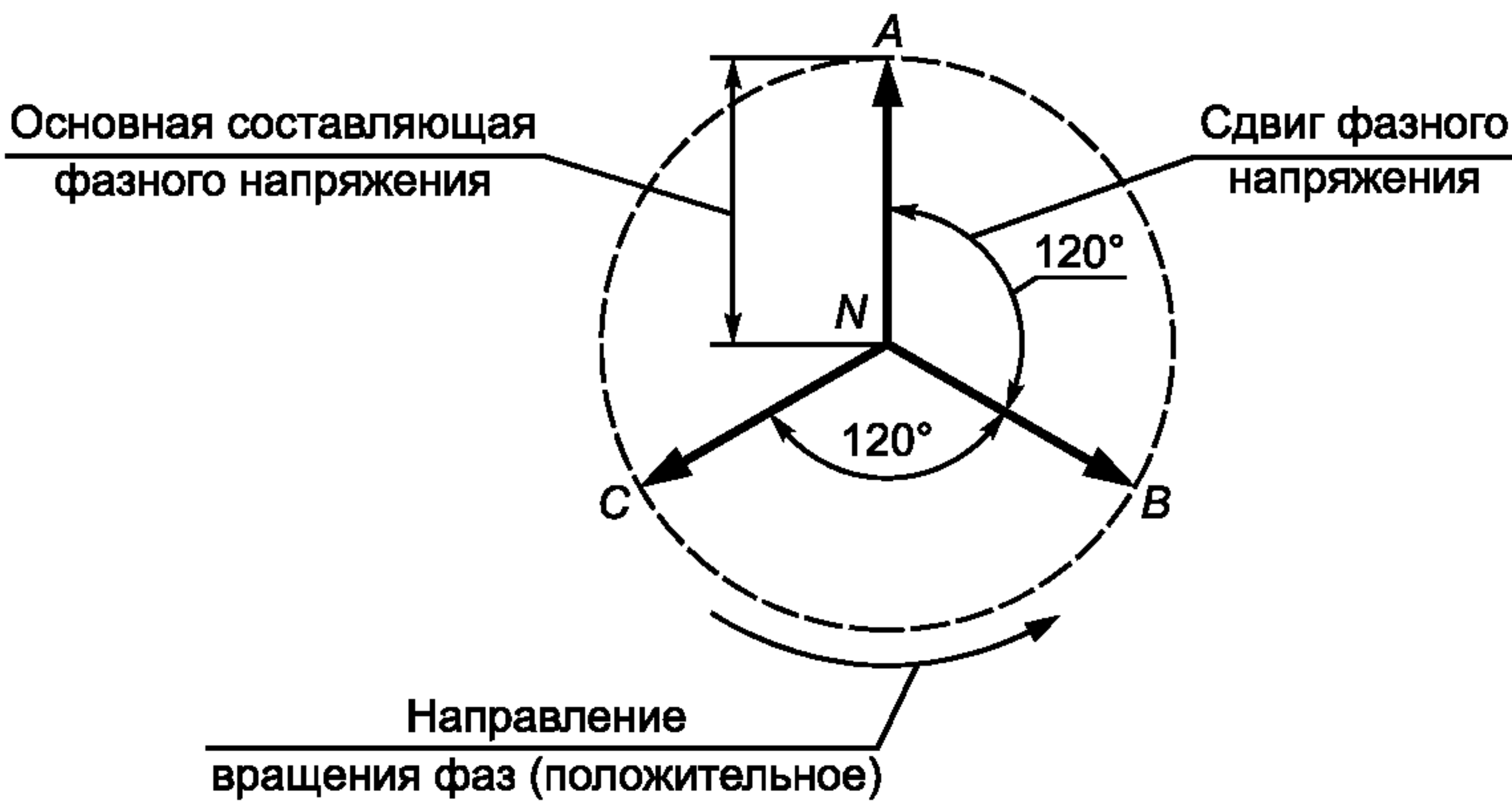
Рисунок 1 — Сдвиг и последовательность фазных напряжений в трехфазной системе электроснабжения
