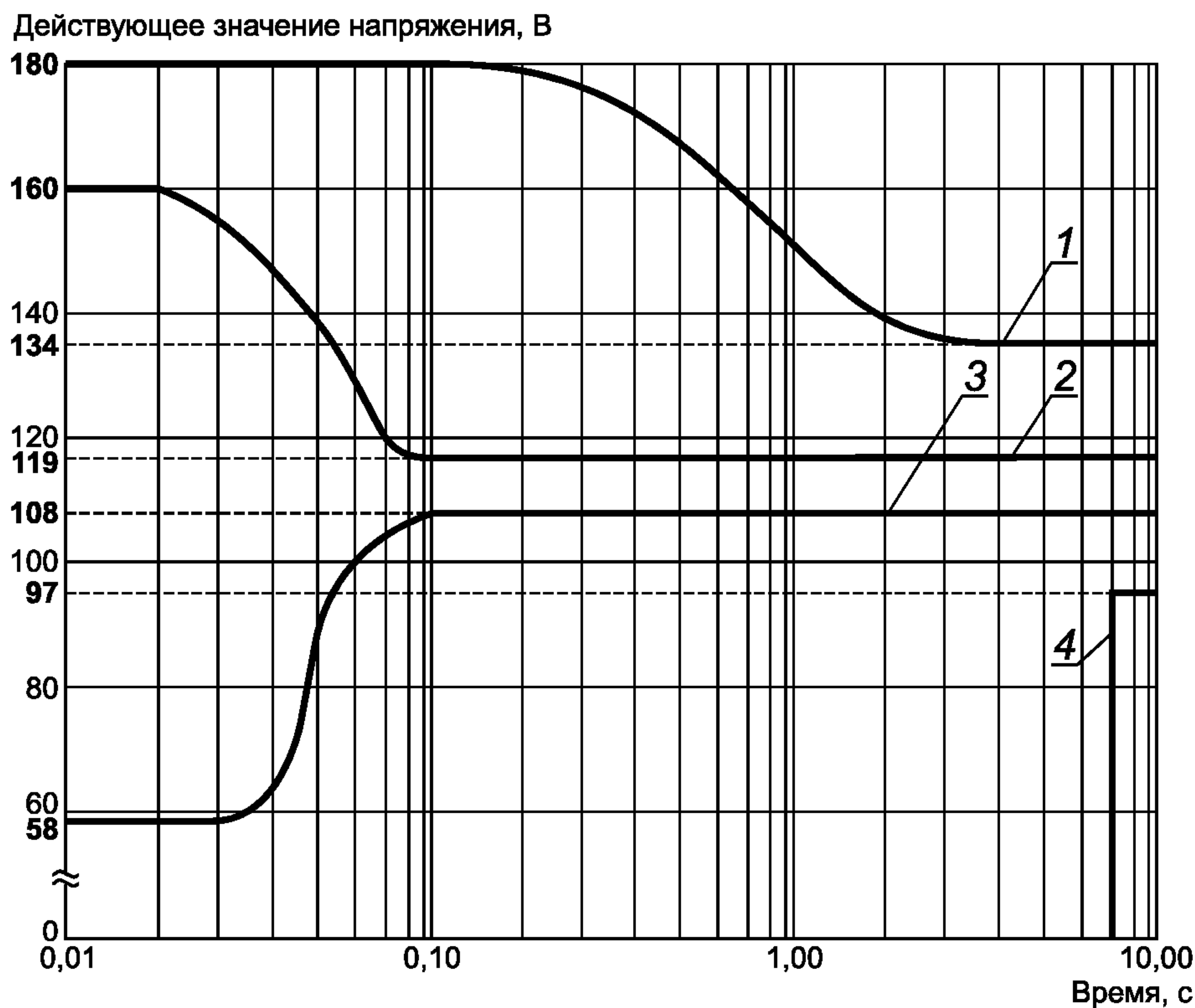
1 и 4 — верхний и нижний пределы при ненормальной работе СЭС; 2 и 3 — верхний и нижний пределы при нормальной или частичной работе СЭС
