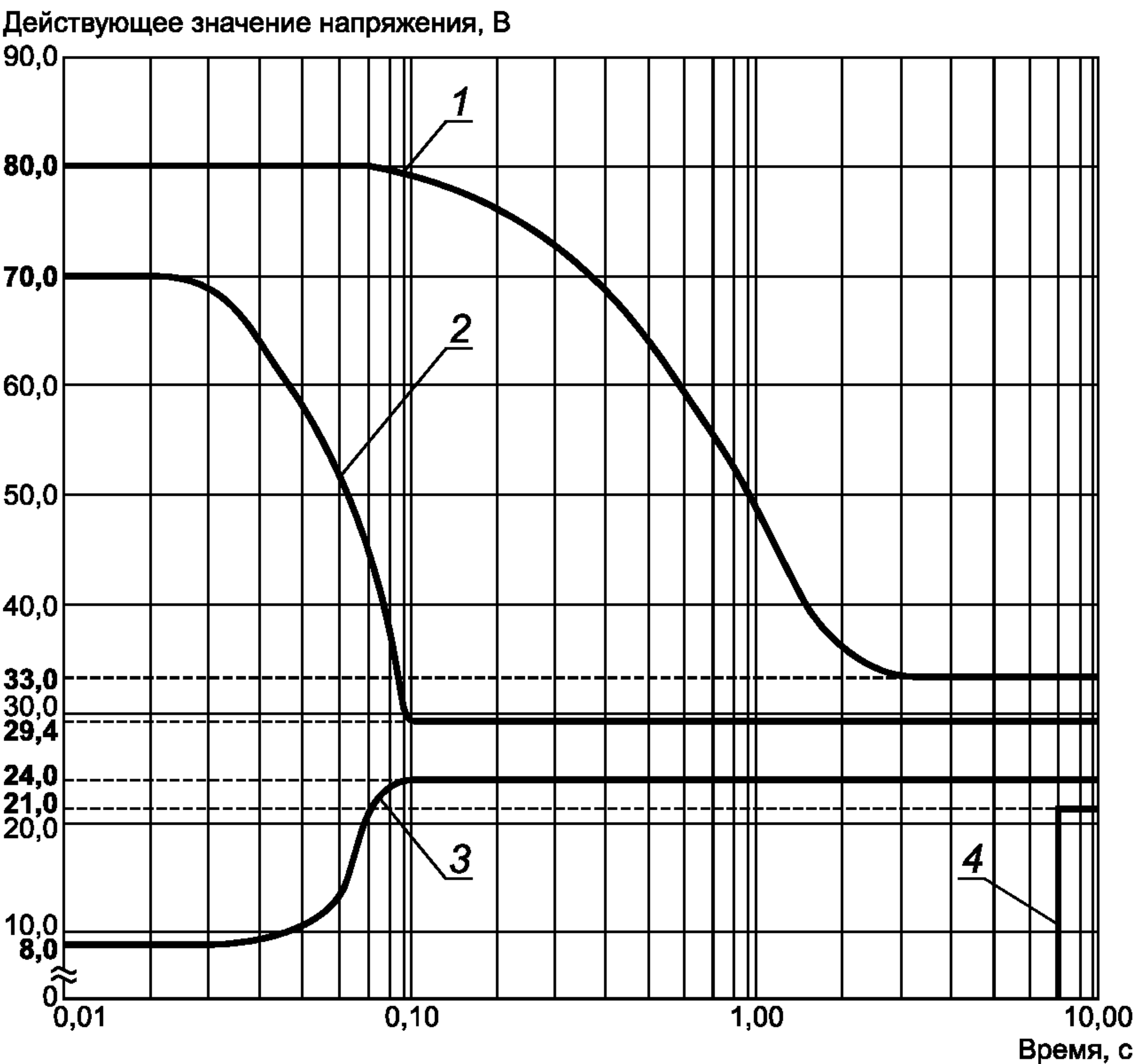
1 и 4 — верхний и нижний пределы при ненормальной работе СЭС; 2 и 3 — верхний и нижний пределы при нормальной или частичной работе СЭС
