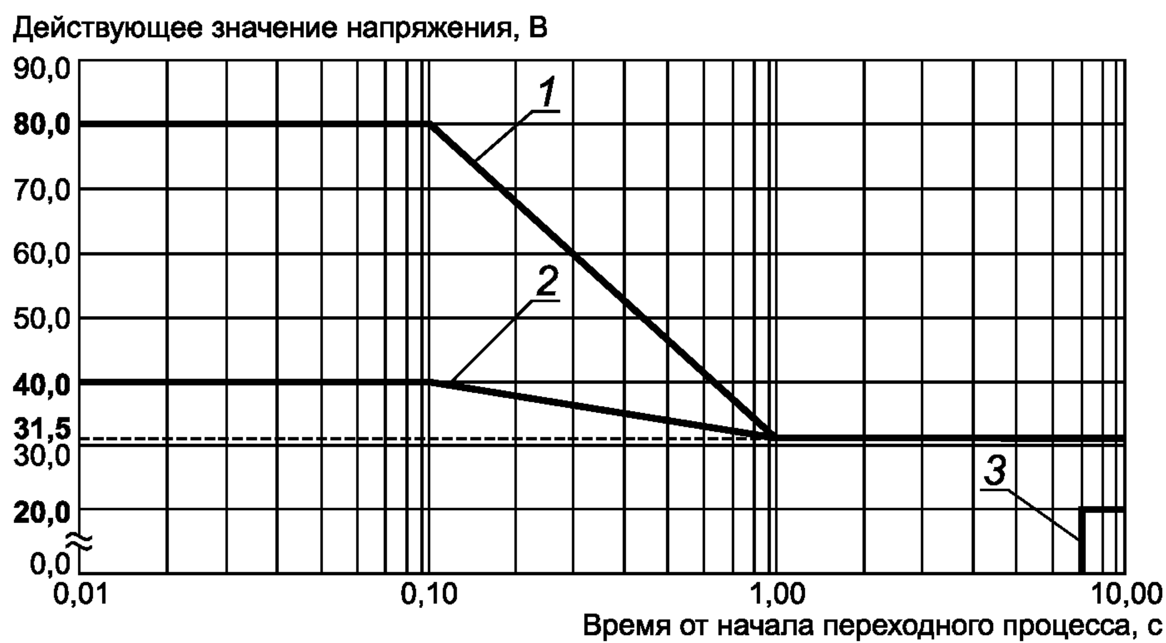
1 — верхний предел при питании от СЭС переменной частоты; 2 — верхний предел при питании от СЭС постоянной частоты; 3 — нижний предел при питании от СЭС переменной и постоянной частоты
