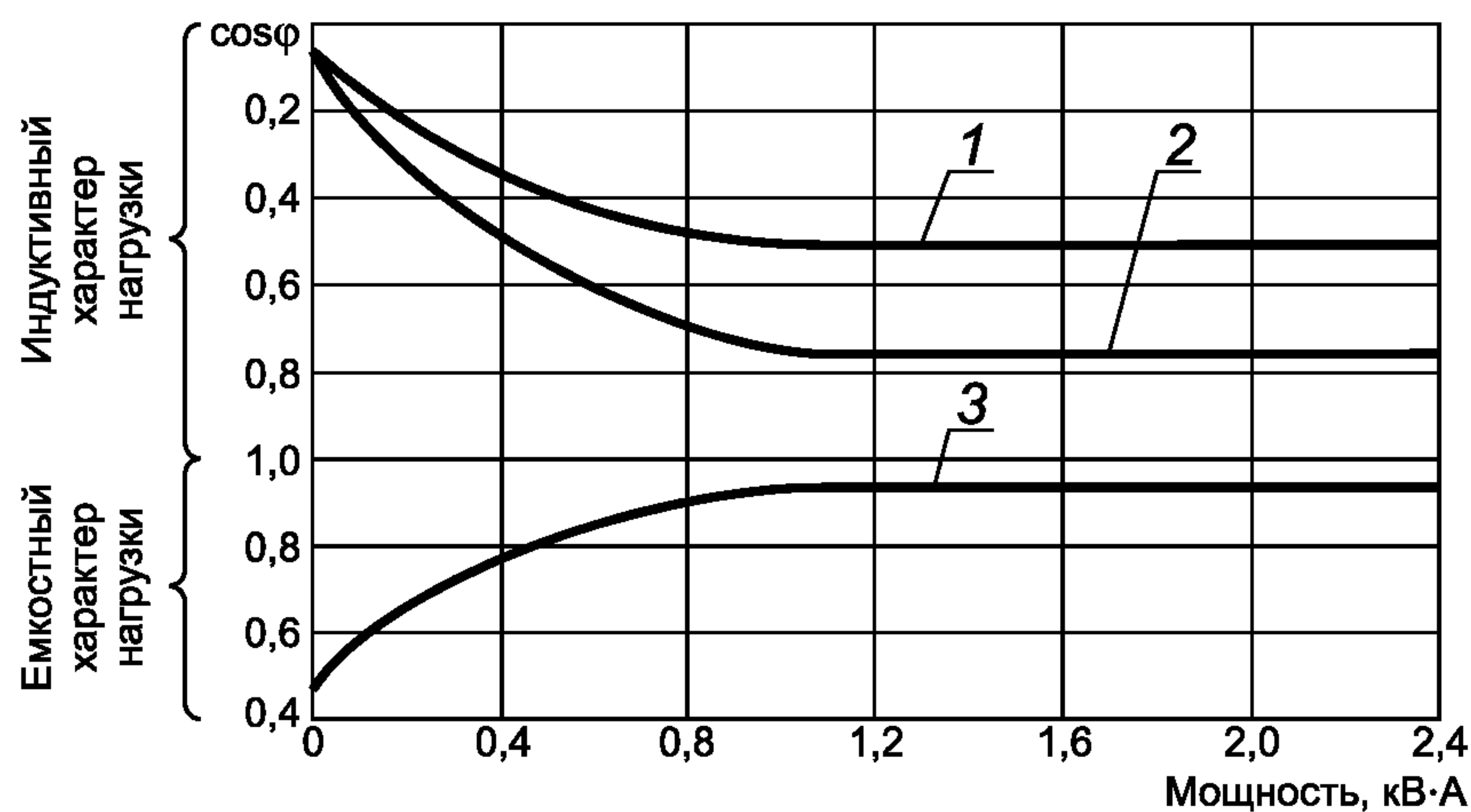
1 — асинхронные электродвигатели; 2 — индуктивная нагрузка; 3 — емкостная нагрузка
