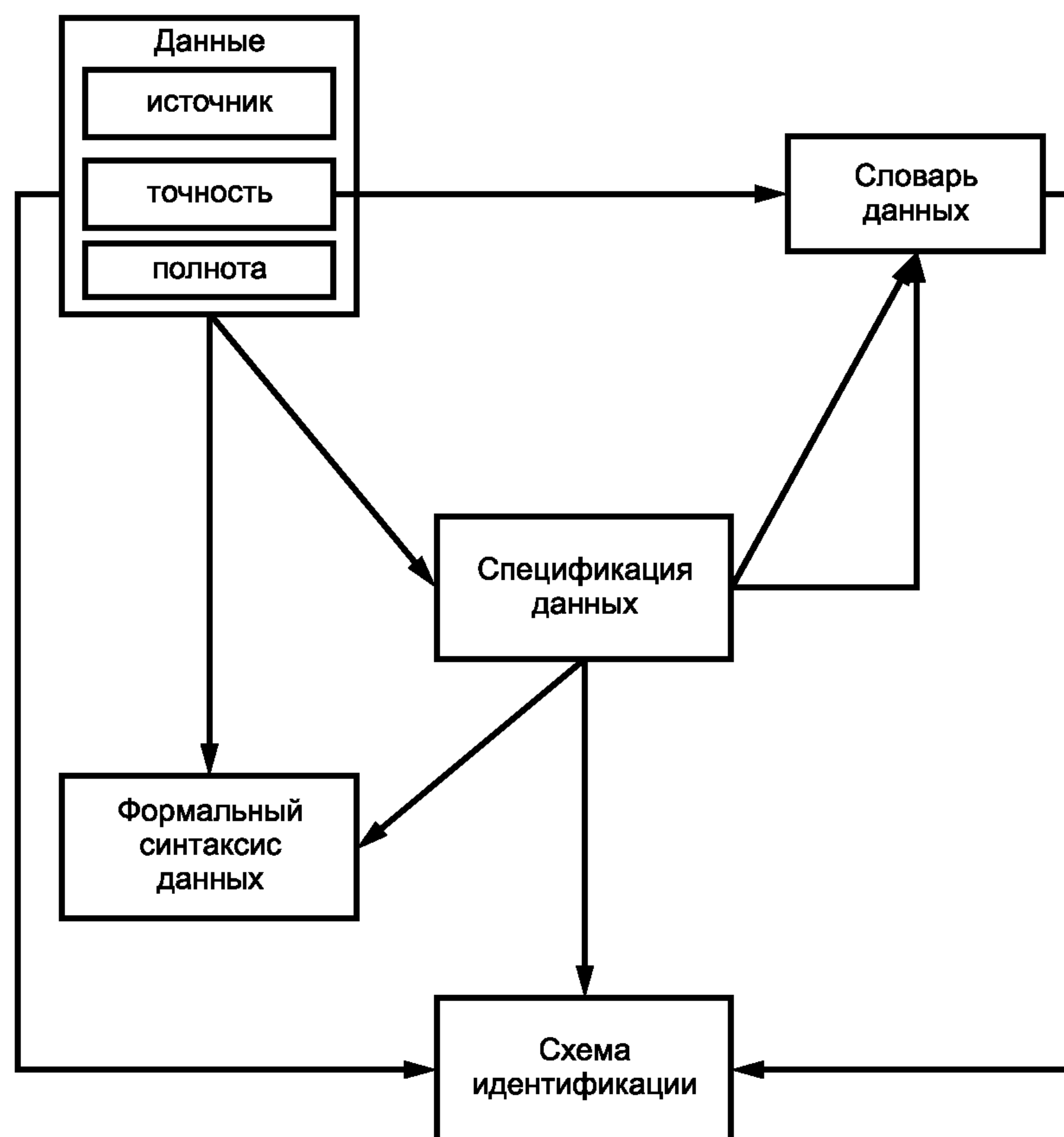
Рисунок 2 — Структура информационных данных
