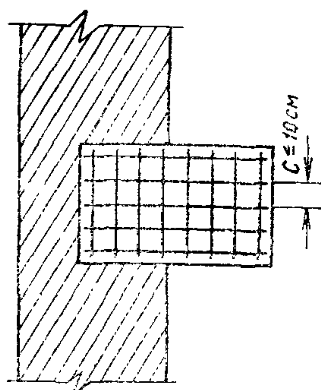
Рис. 5. Железобетонные распределительные плиты
