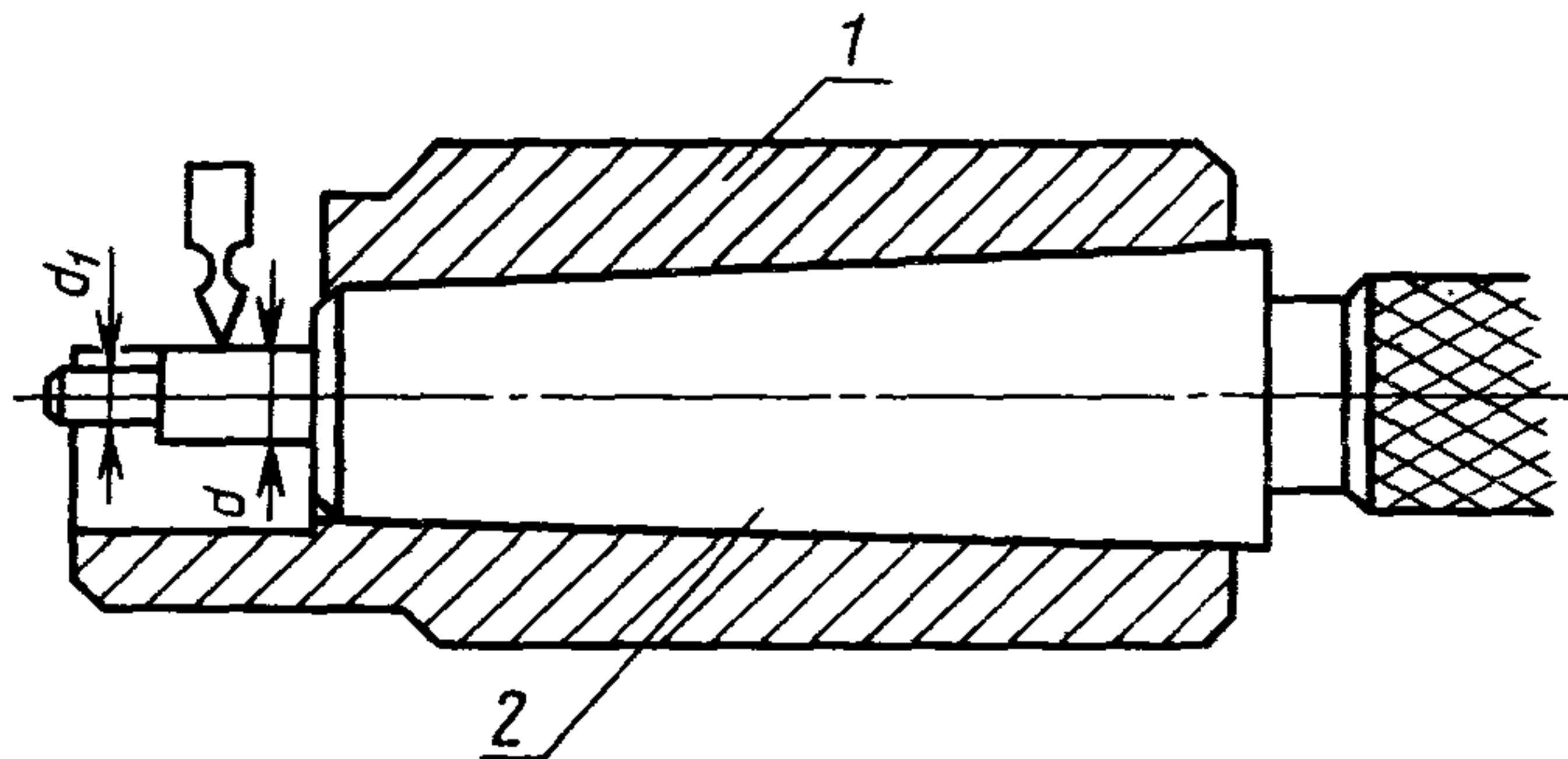
1 — калибр-втулка; 2 — специальная пробка
