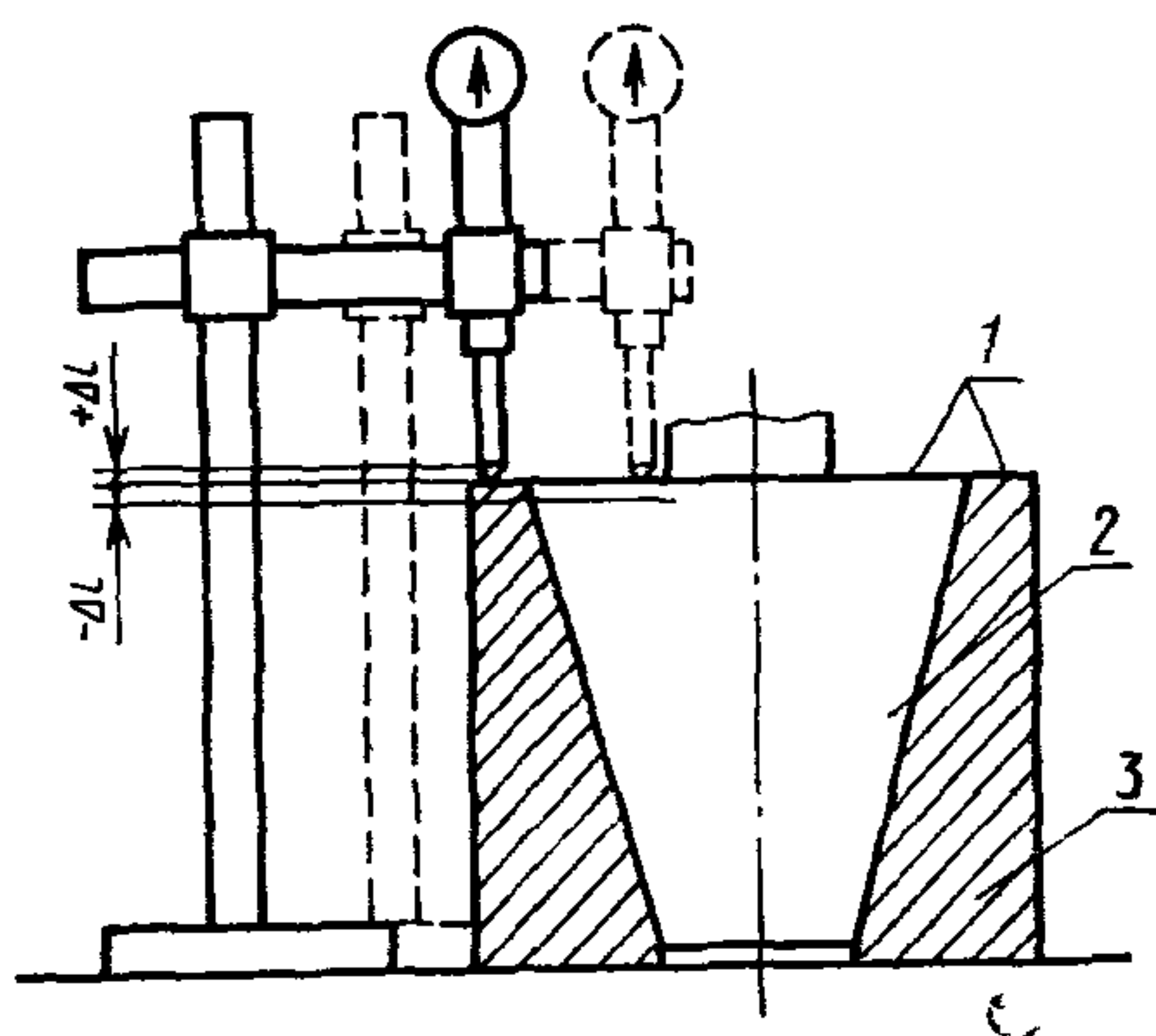
1 — контрольные плоскости; 2 — калибр-пробка контрольный; 3 — калибр-втулка
