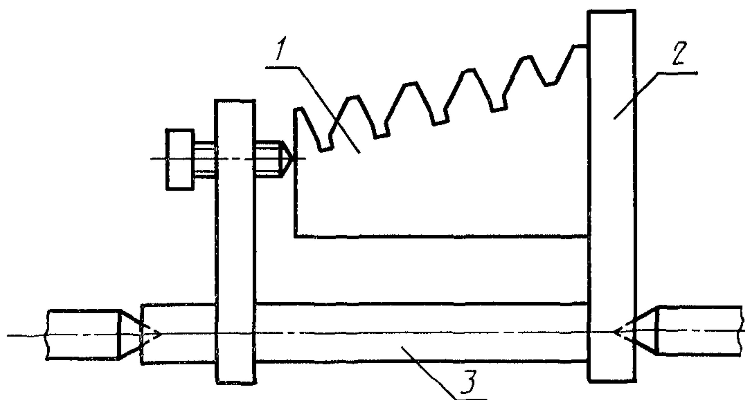
1—отливка; 2—базовая плоскость; 3—валик
