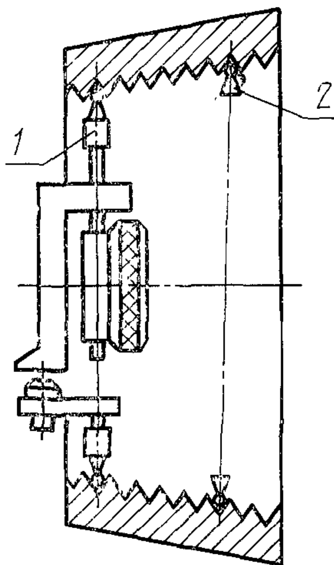
1—положение 1-го прибора; 2—положение 2-го прибора
