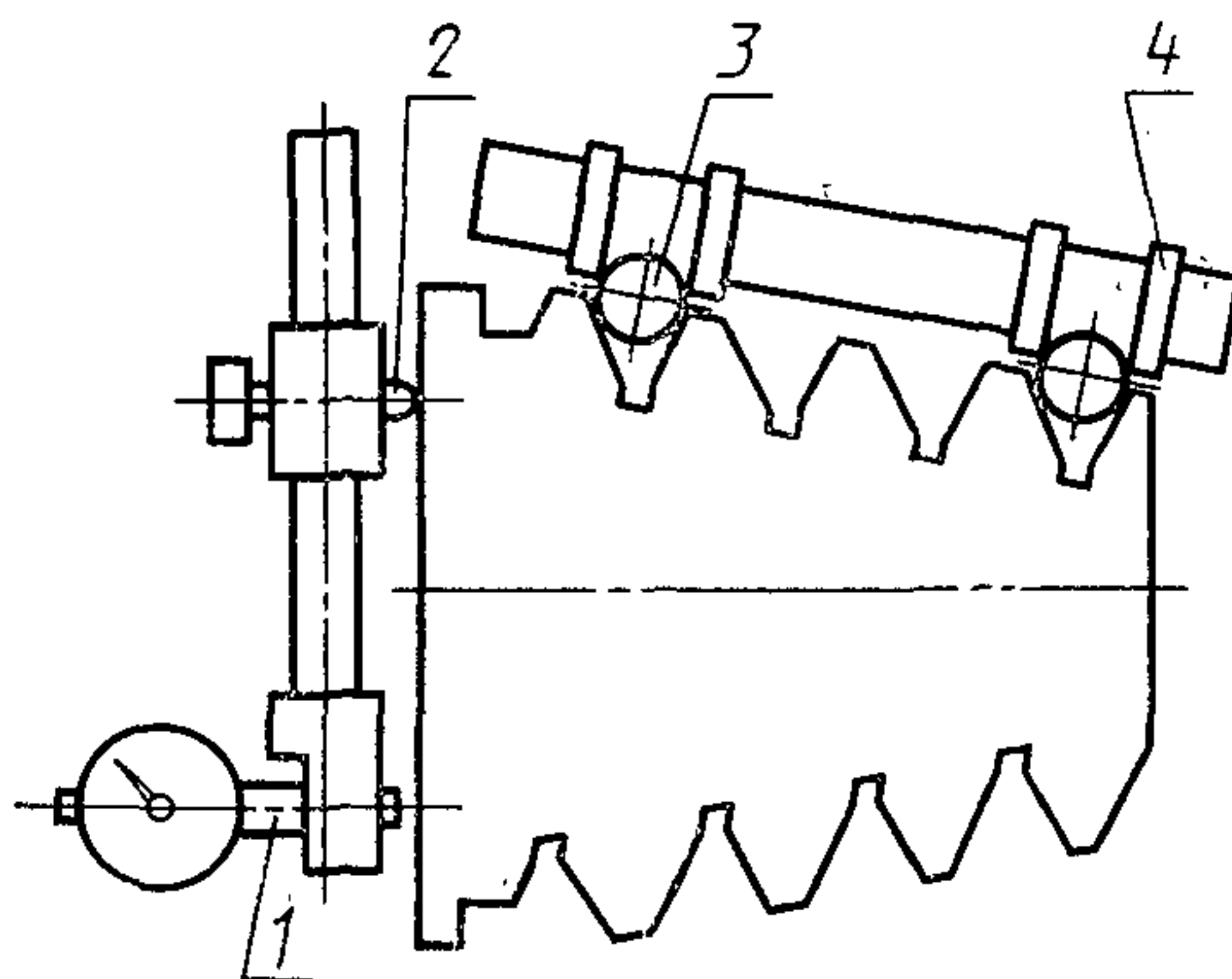
1—измерительная головка, 2—упор; 3—проводочки; 4—резинки
