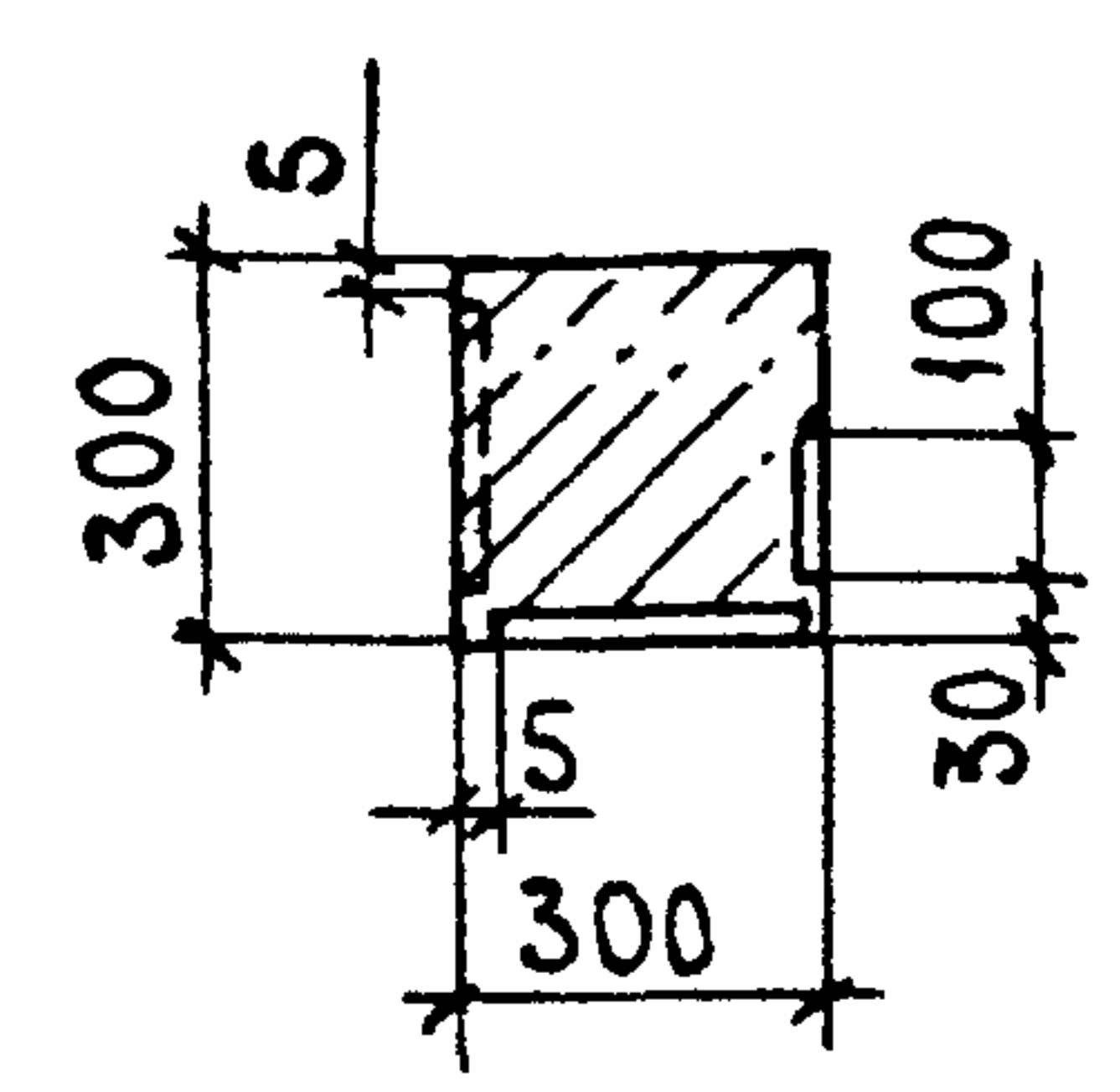
2-2 М 1:20
