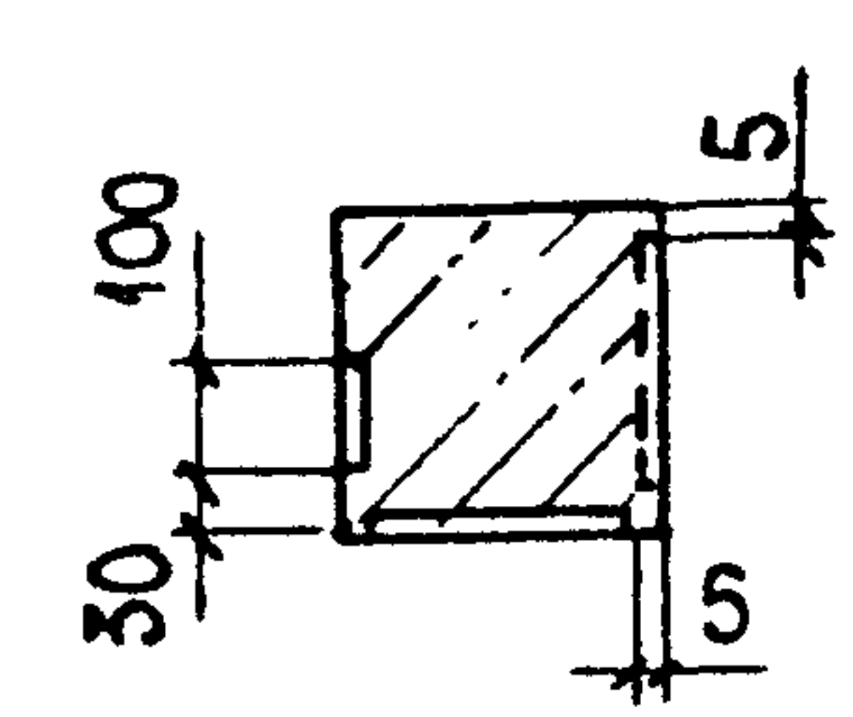
3-3 М 1:20
