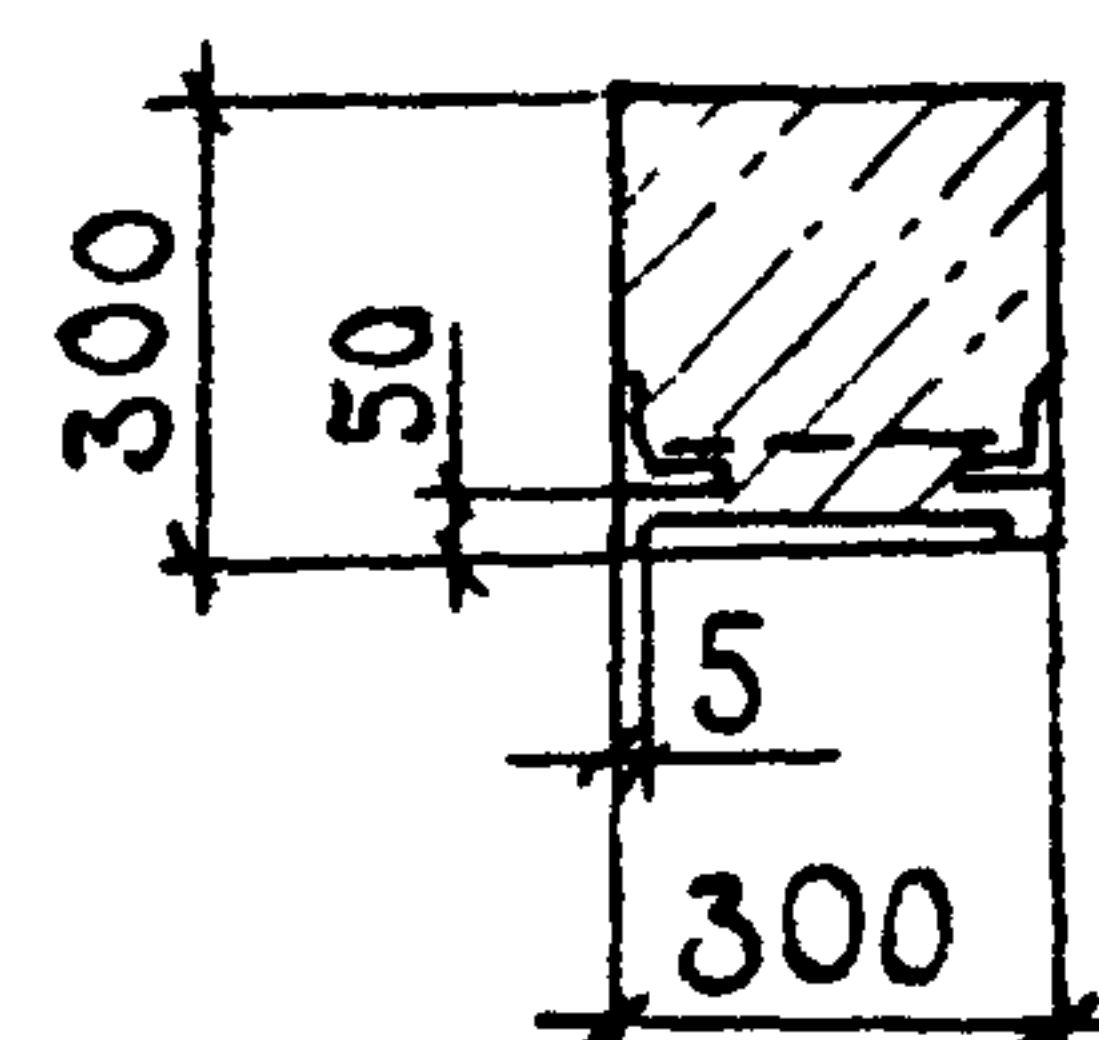
А-А М 1:20
