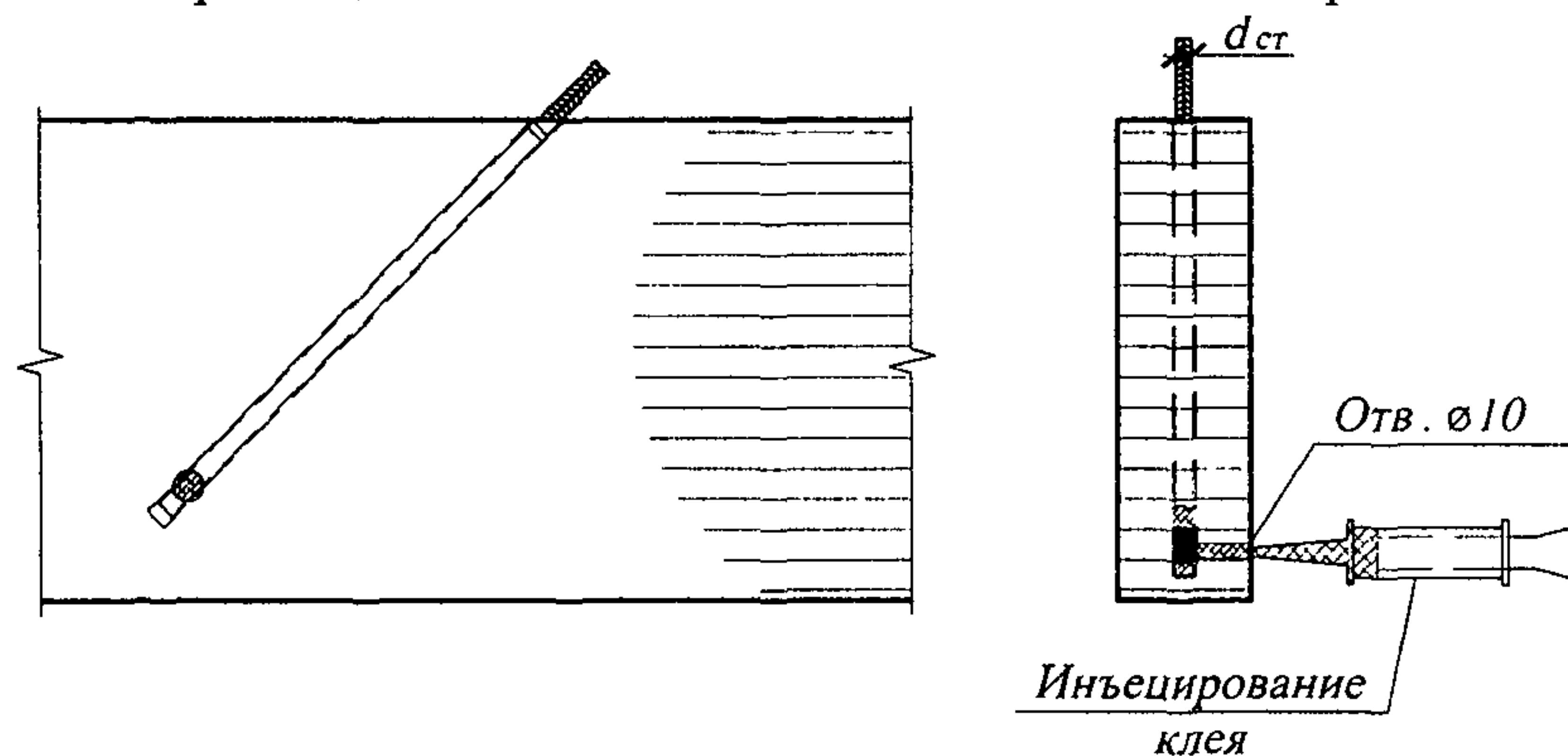
Рисунок И.2 — Схема подачи клея под давлением
