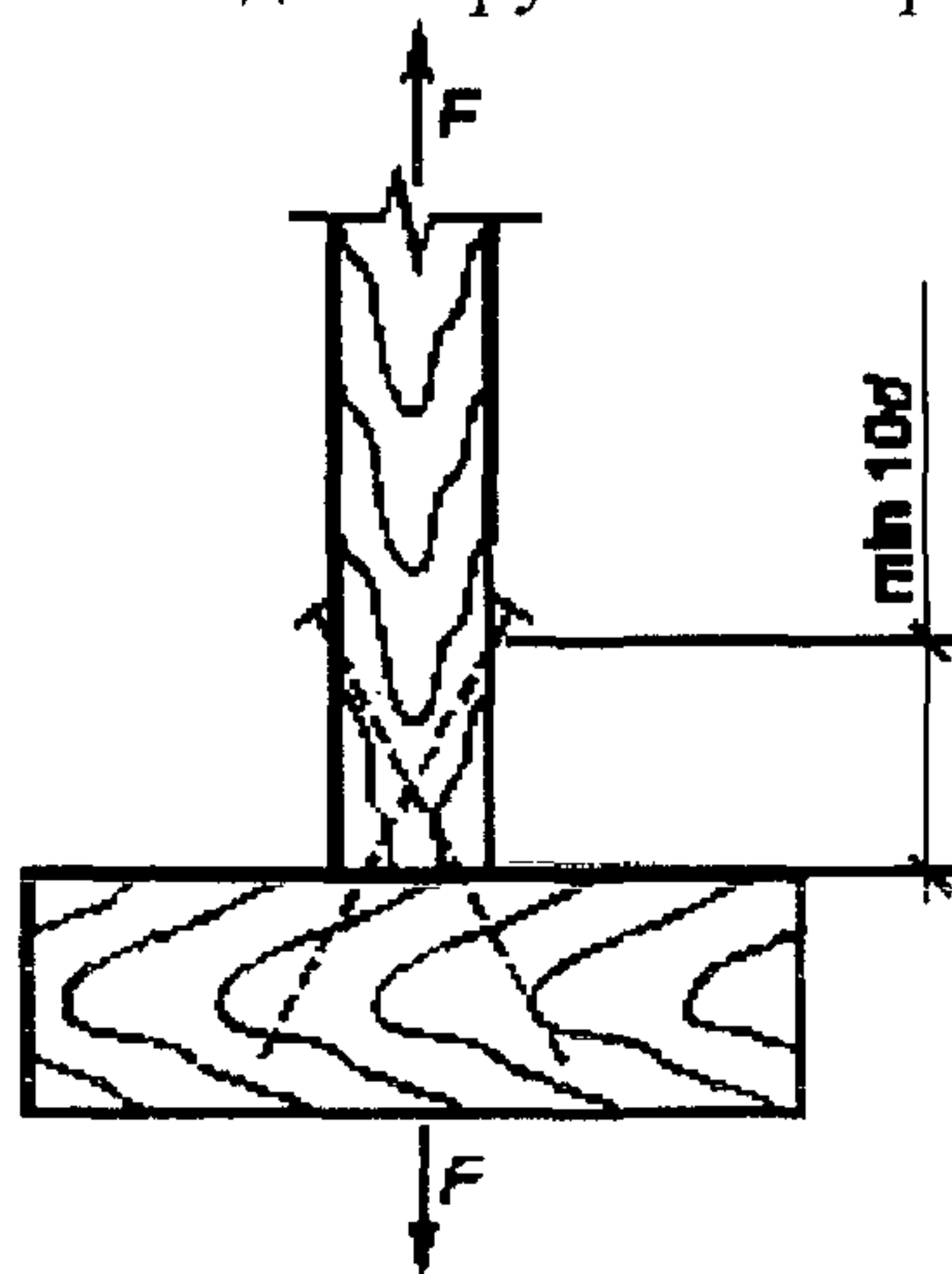
Рисунок 14 — Наклонная забивка гвоздей
