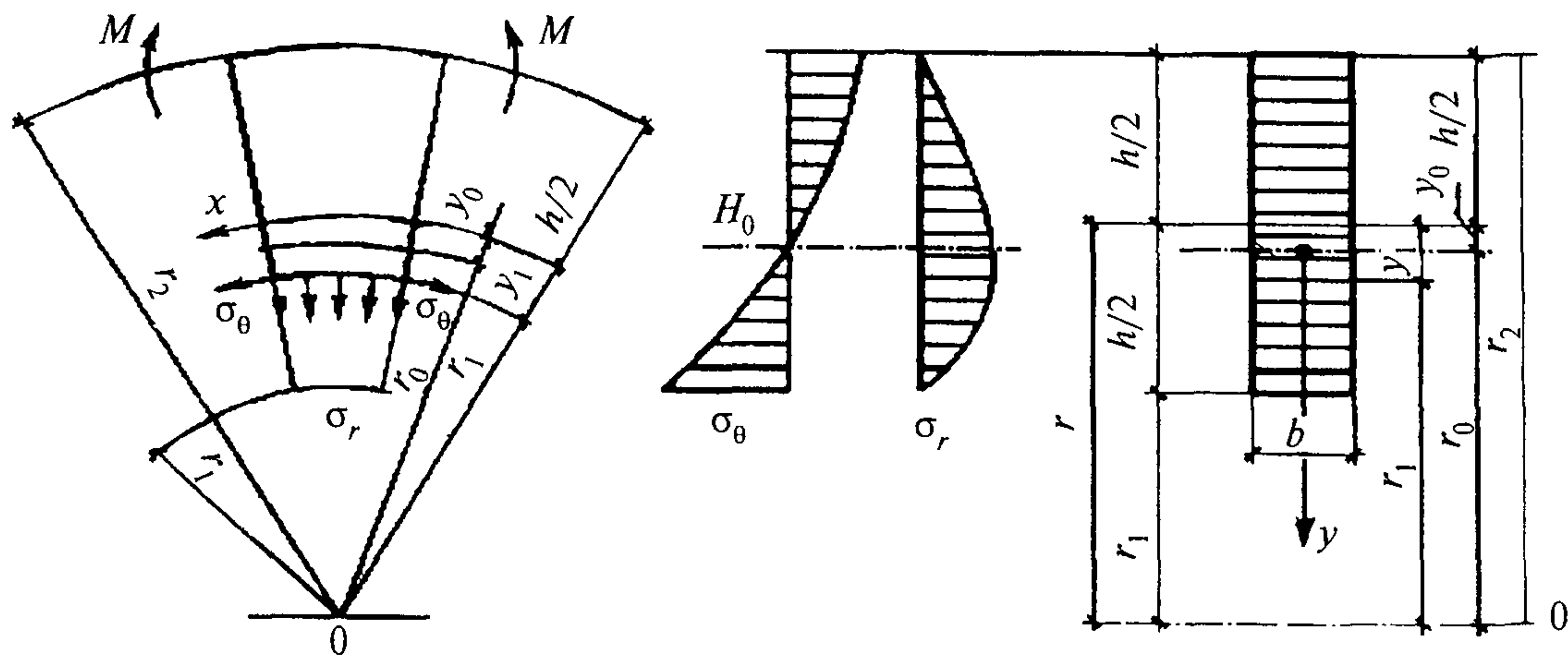
Рисунок 3 — Расчетная схема кривого бруса при чистом изгибе
