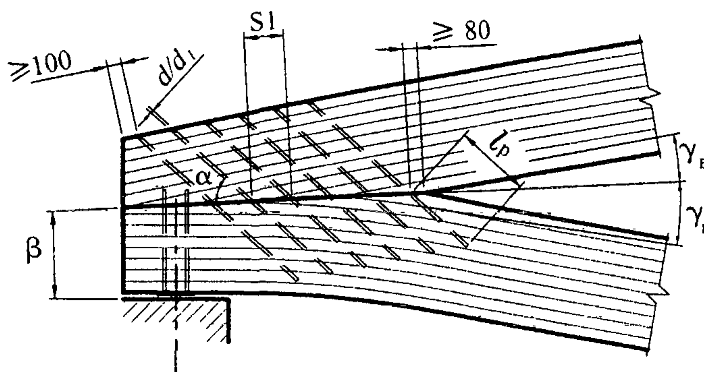
Рисунок 24 — Схема опорного узла линзообразной фермы
