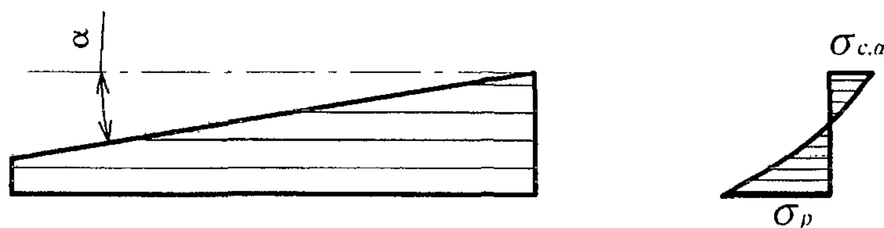
Рисунок 21 — Односкатная балка
