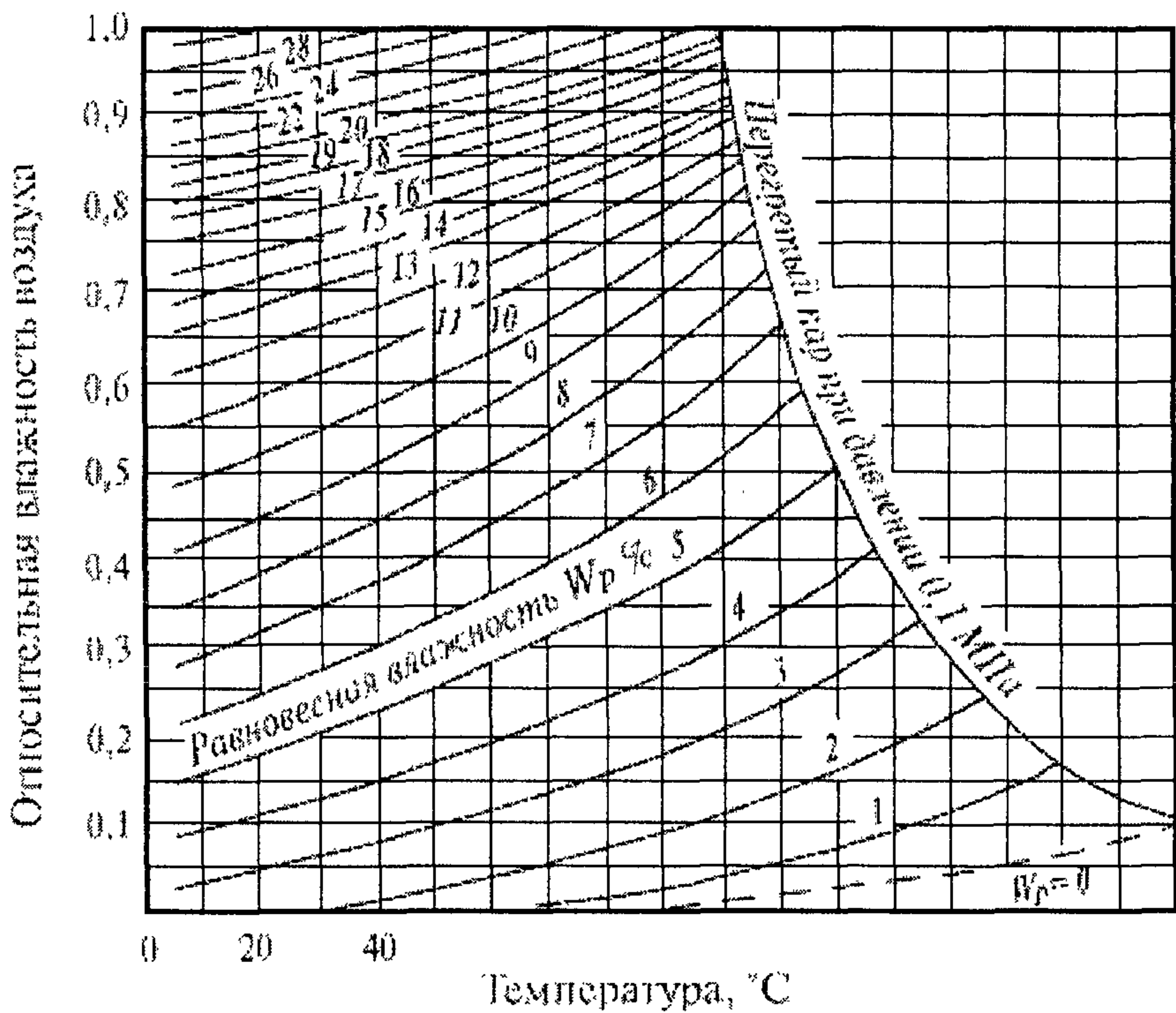
Рисунок Г.1 — Диаграмма равновесной влажности древесины
