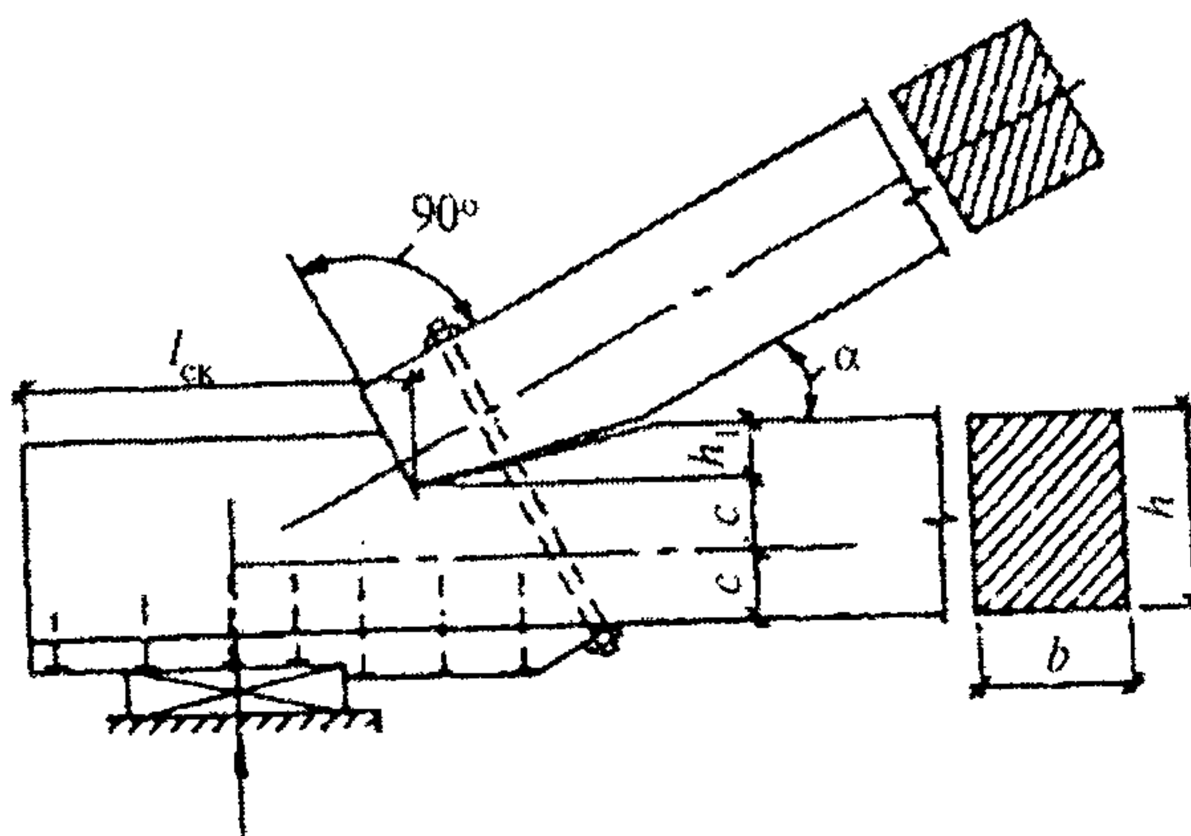
Рисунок 8 — Лобовая врубка с одним зубом
