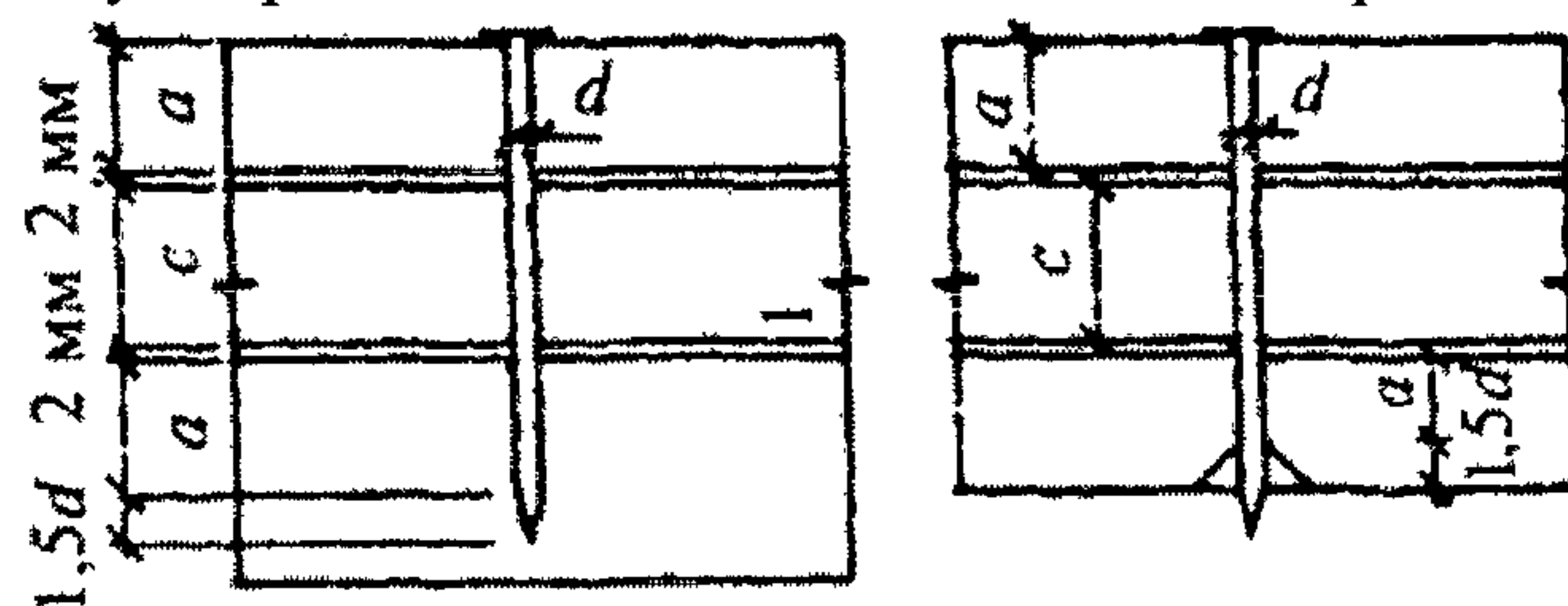
Рисунок 12 — Определение расчетной длины защемления конца гвоздя
