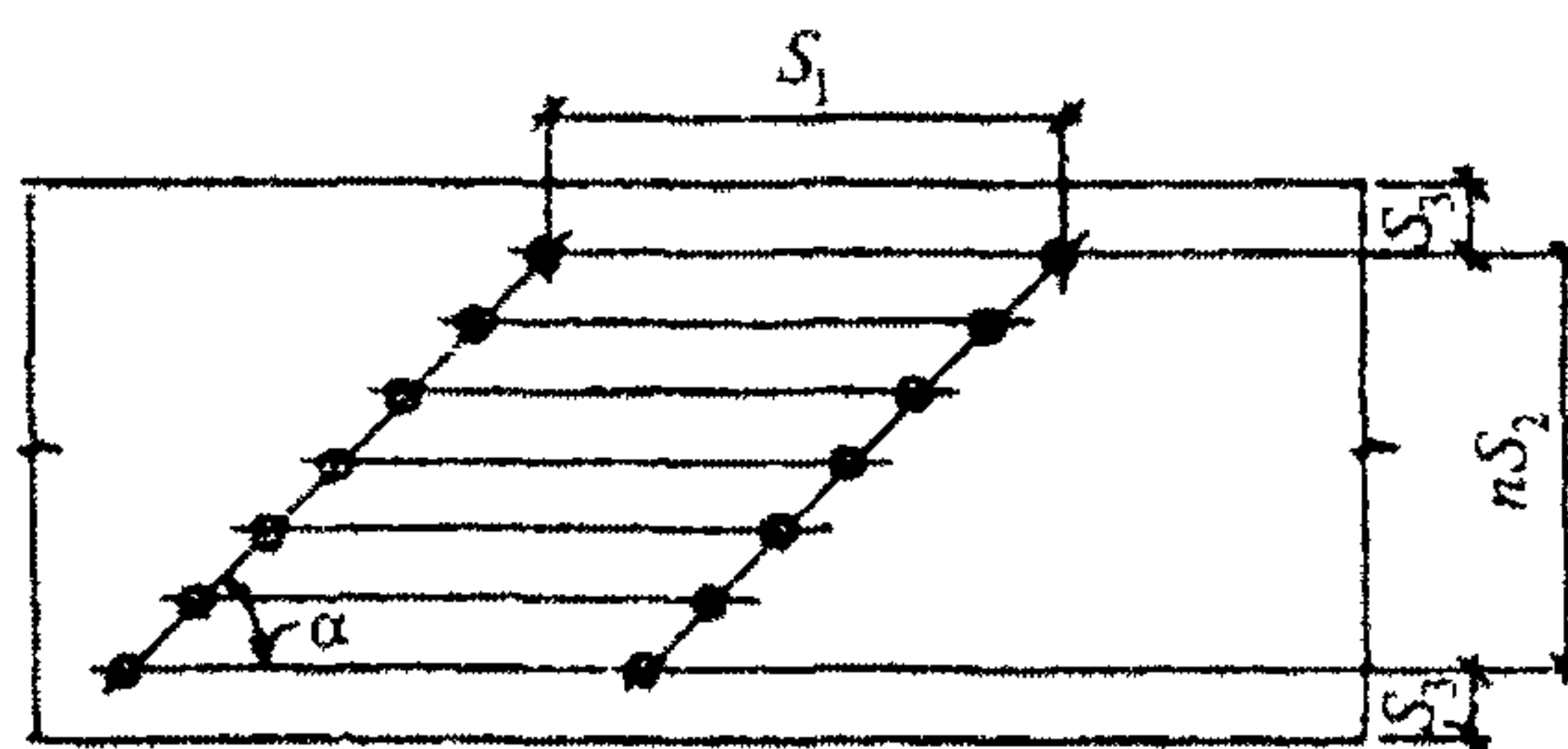
Рисунок 13 — Расстановка гвоздей косыми рядами
