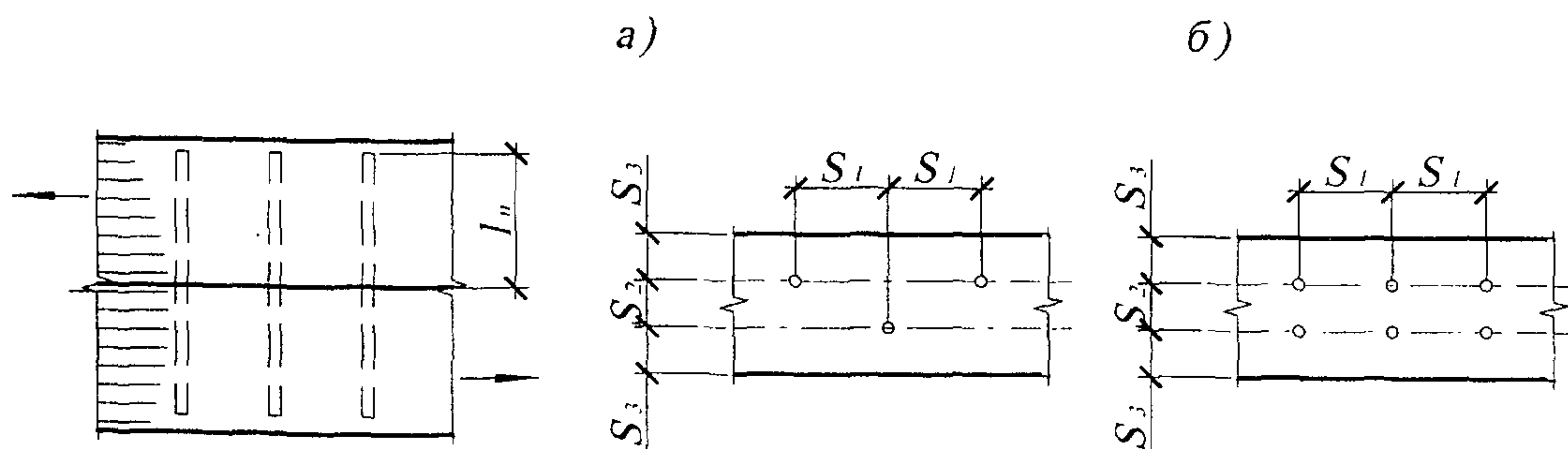
а — шахматная расстановка; б — двухрядная расстановка
