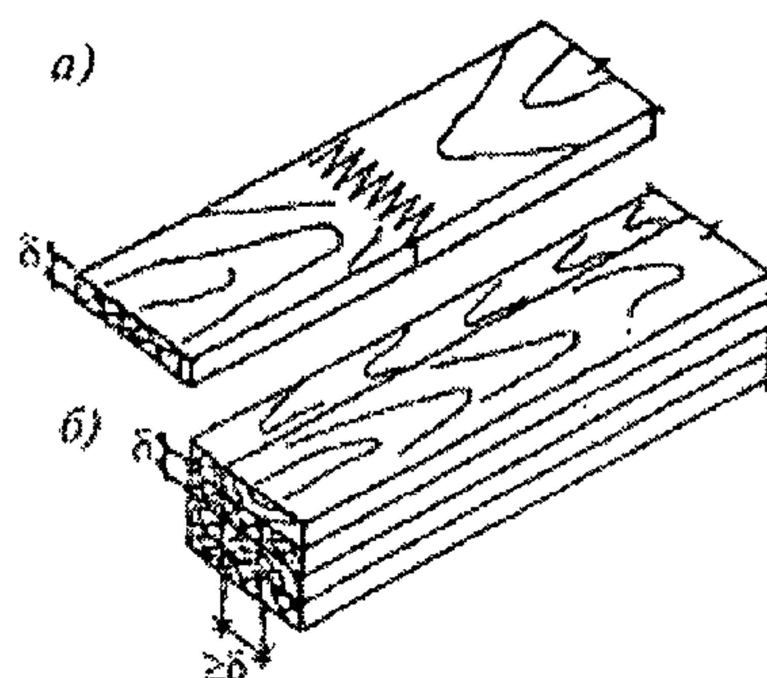
a — при стыковании отдельных слоев по длине зубчатым шипом, выходящим на пласть; б — при образовании пакетов и сплачивании по пласти и кромке
