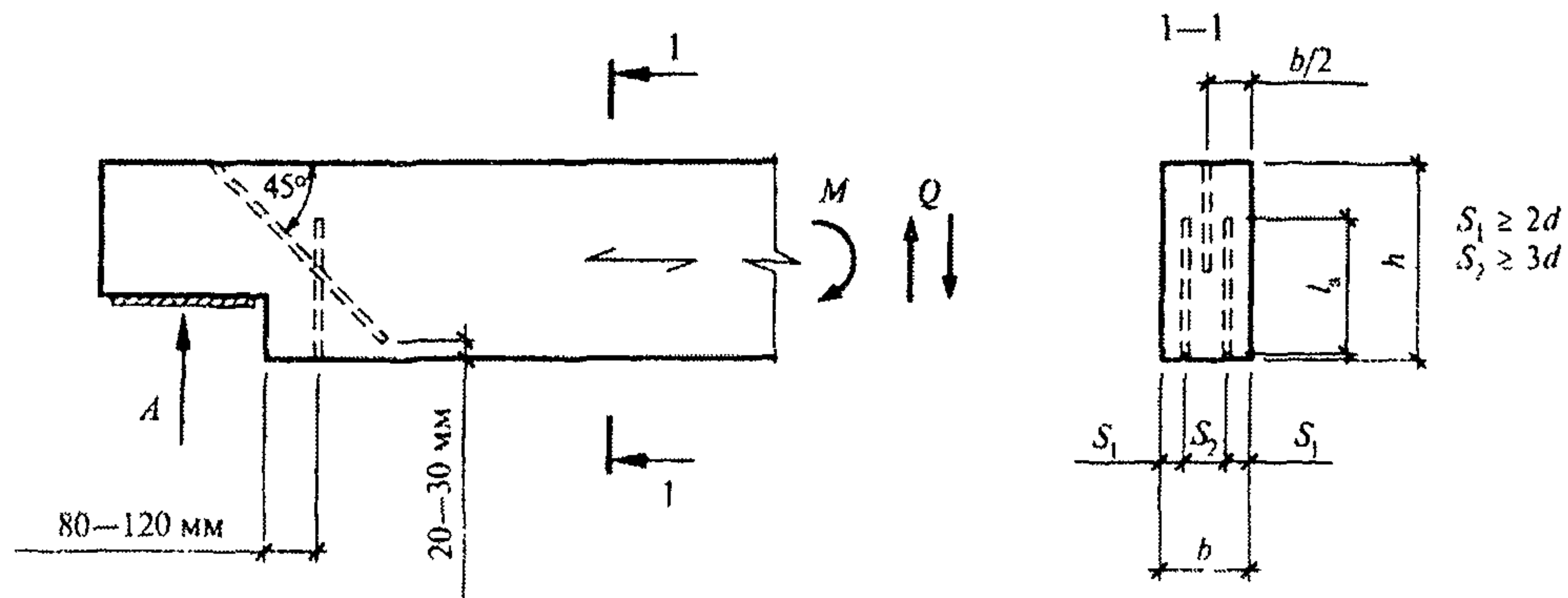
Рисунок 19 — Скошенная подрезка конца балки
