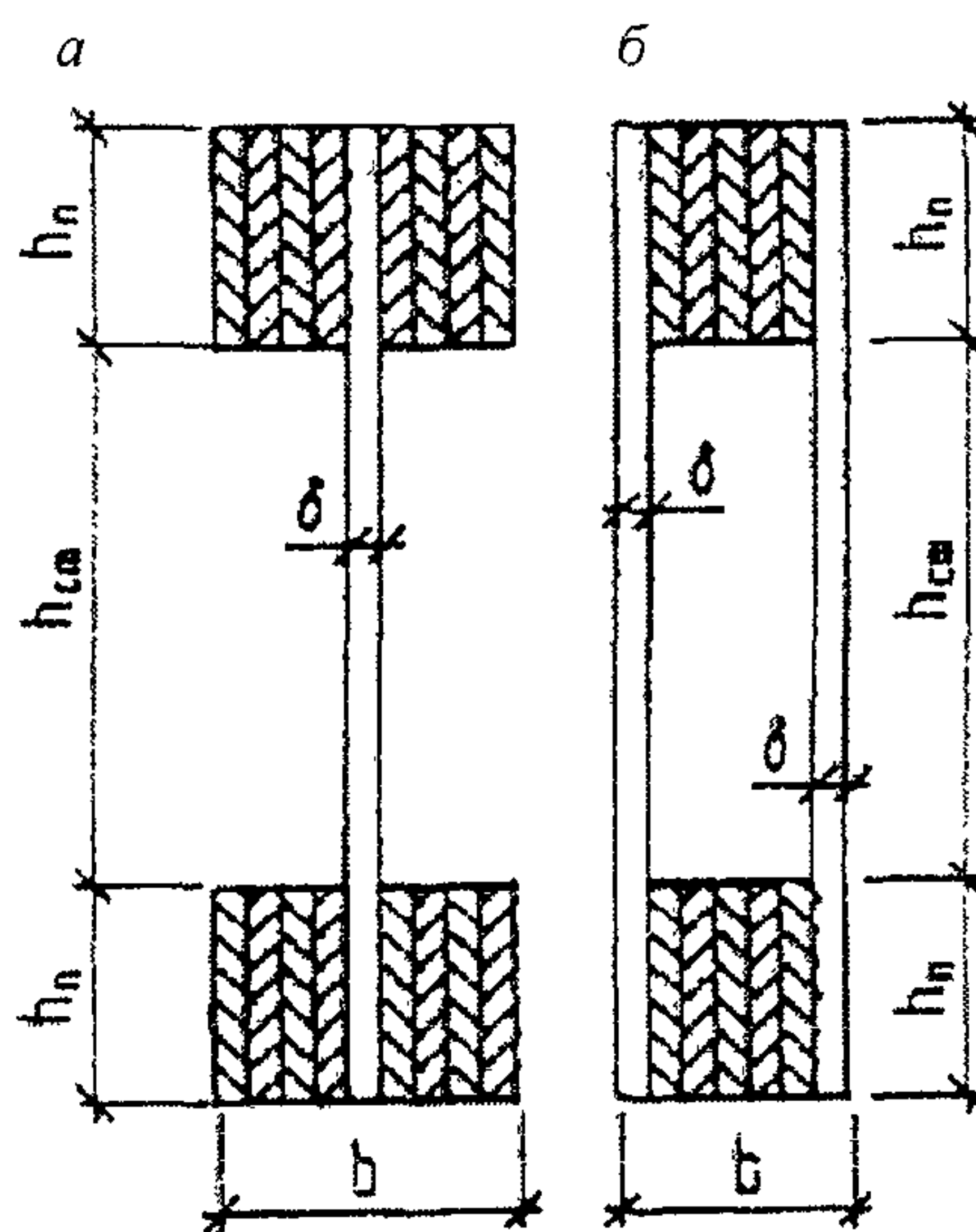
а — двутаврового сечения; б — коробчатого сечения
