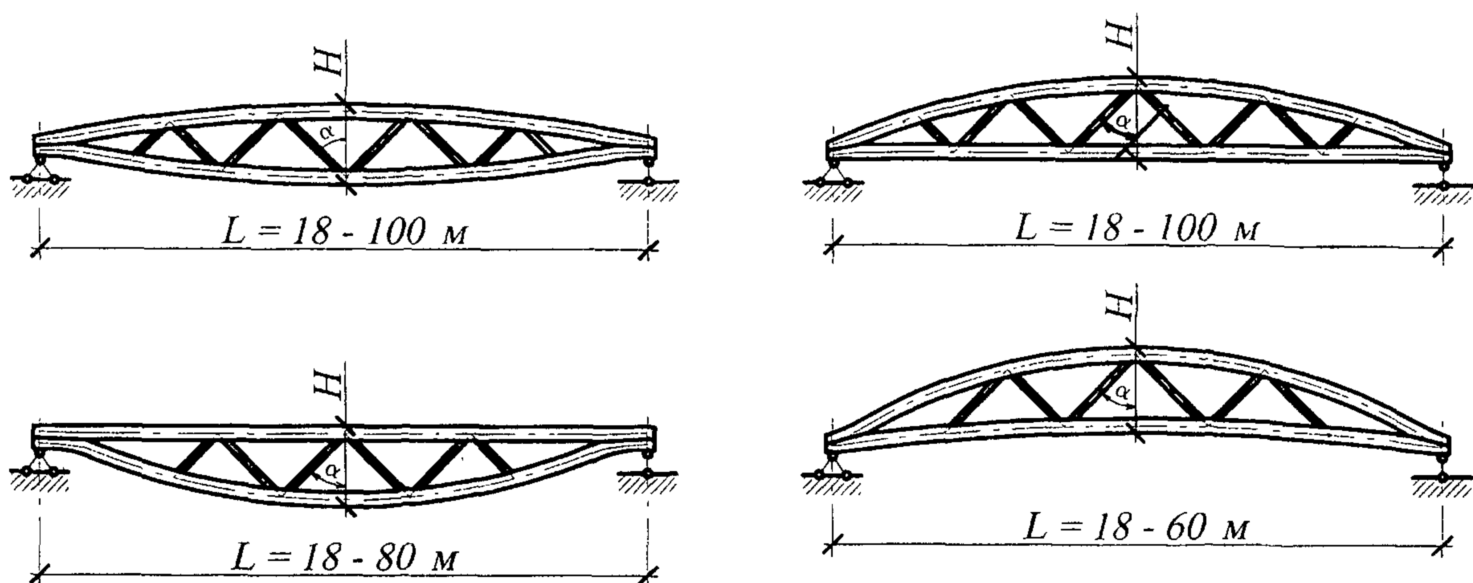
Рисунок 23 — Схемы линзообразных ферм
