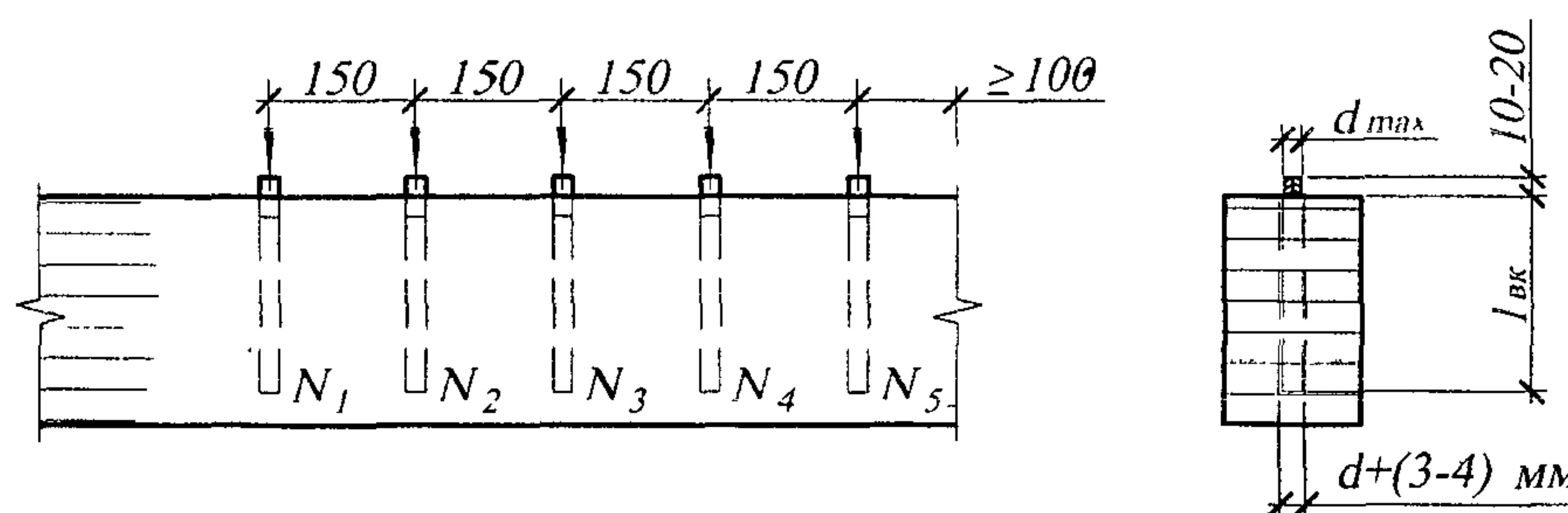
Рисунок И.3 — Схема образцов для испытаний
