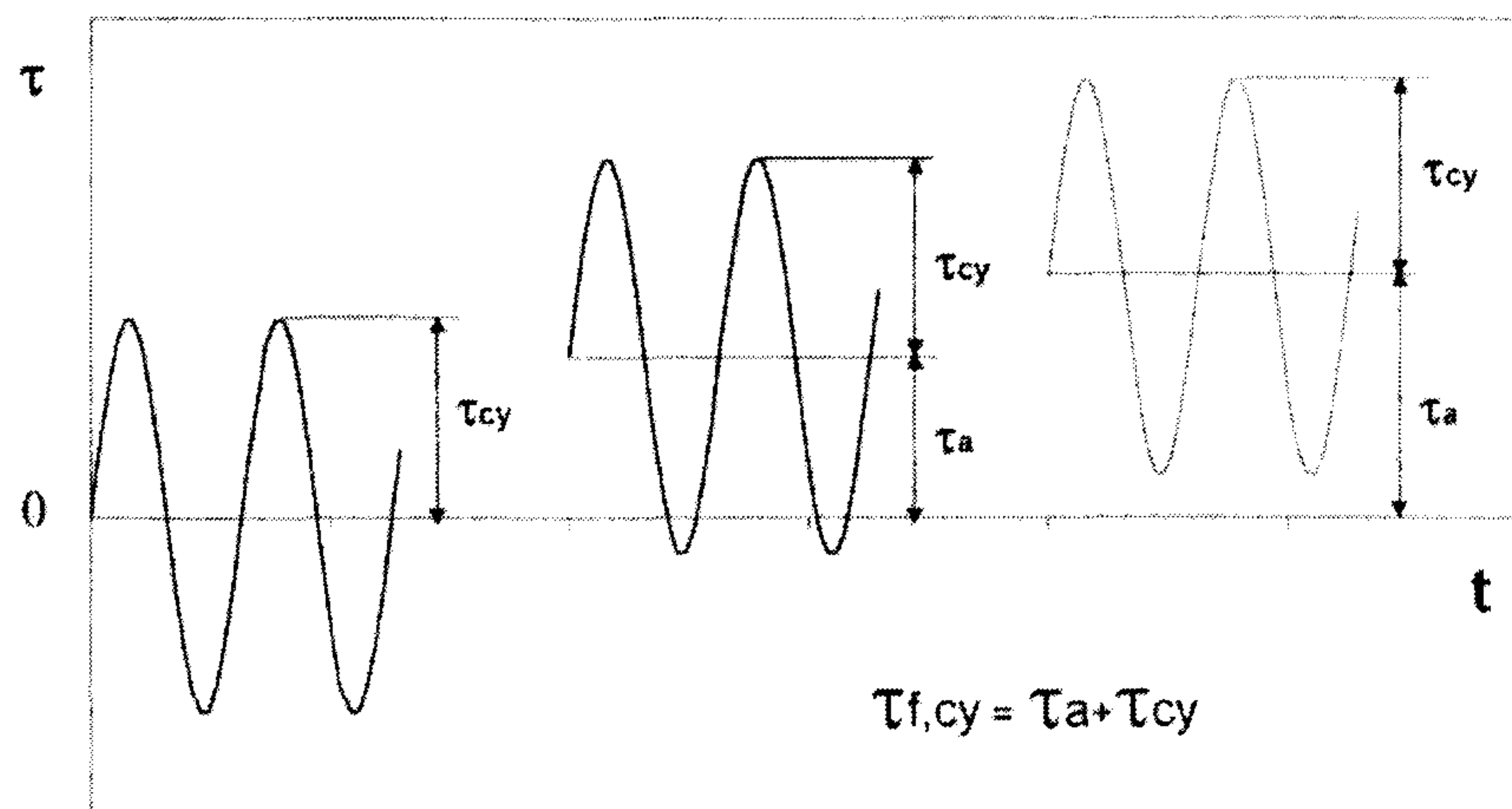
Рисунок Б.3 – Возможные соотношения циклической и статической составляющих касательных напряжений
