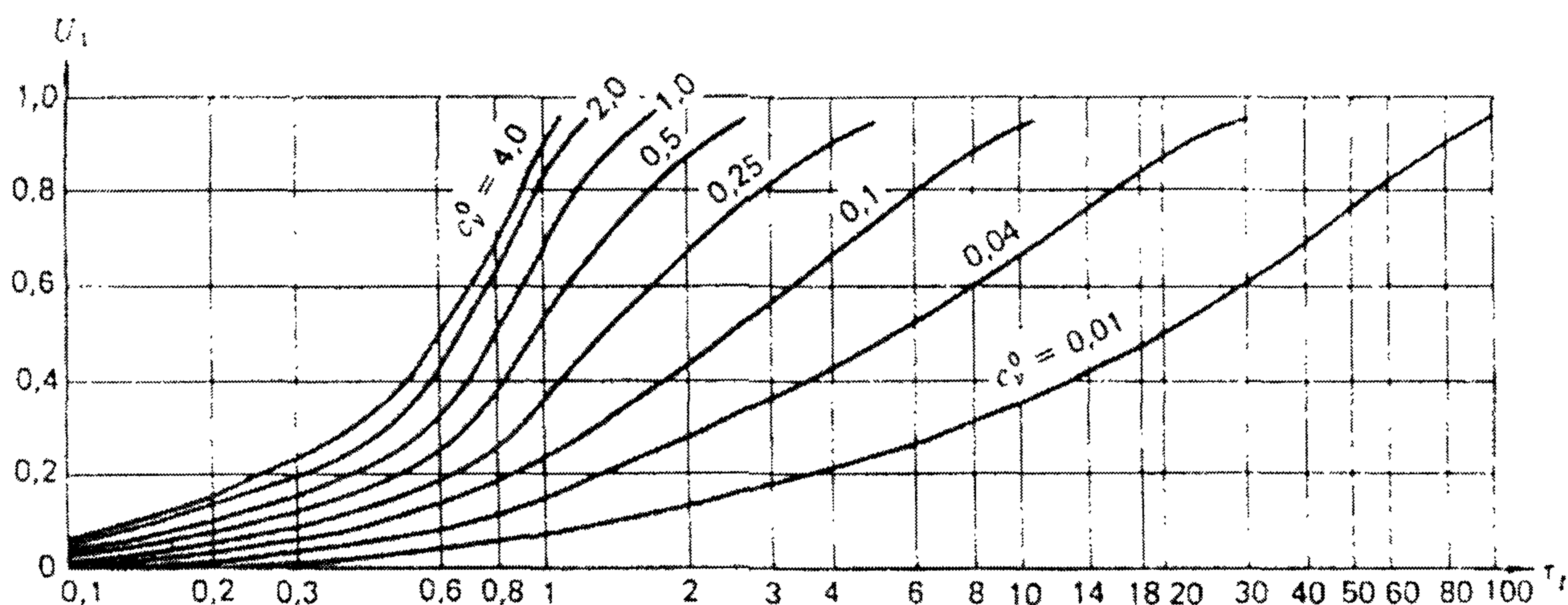
Рисунок М.1 – График зависимости степени консолидации
