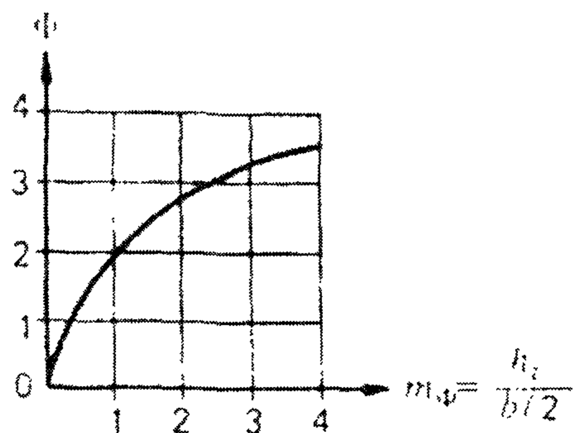
Рисунок Н.2 – График для определения коэффициента \Phi
