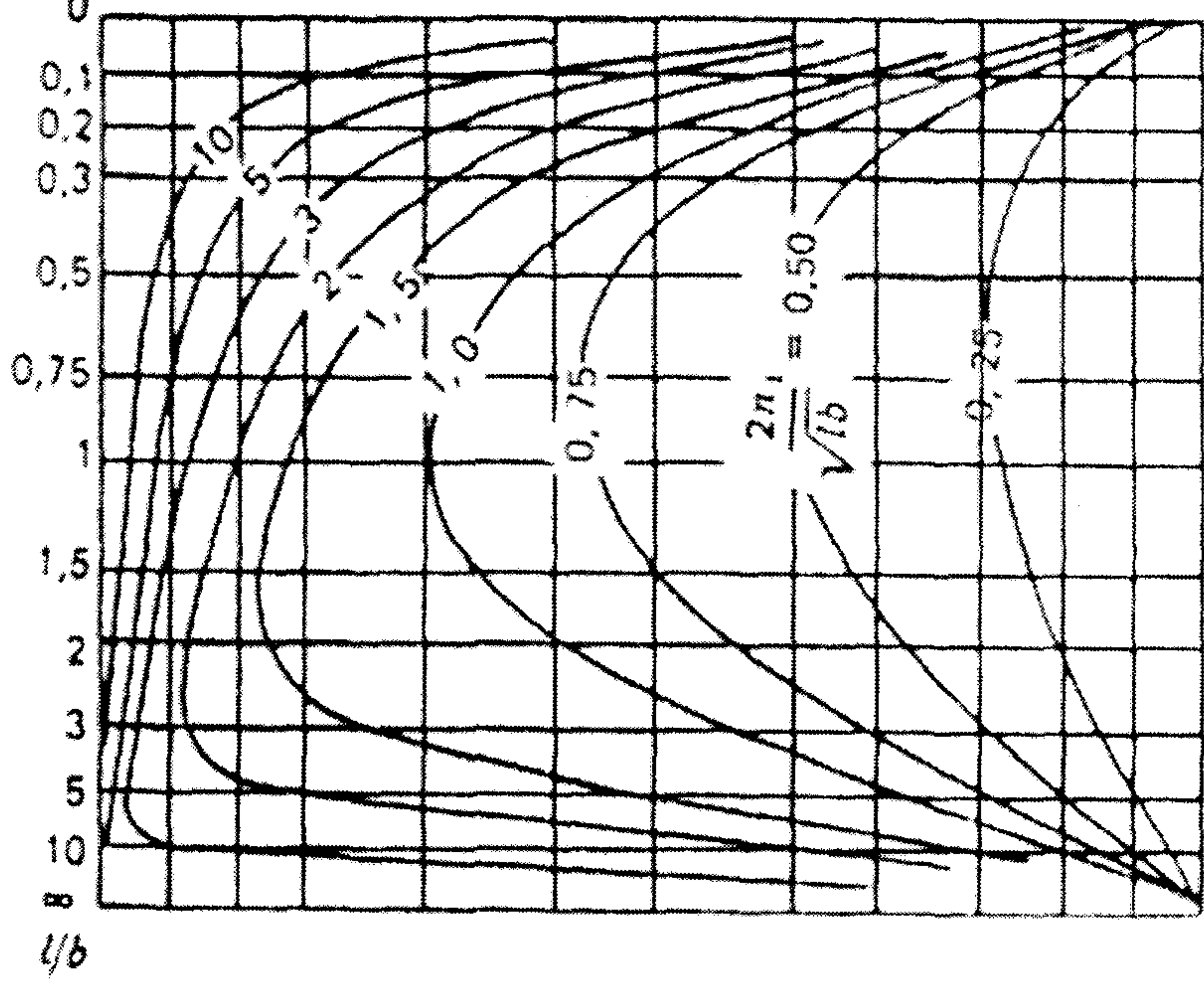
Рисунок Д.2 – Графики для определения коэффициента \alpha_1 (а) и координаты центра поворота n_1 (б)
