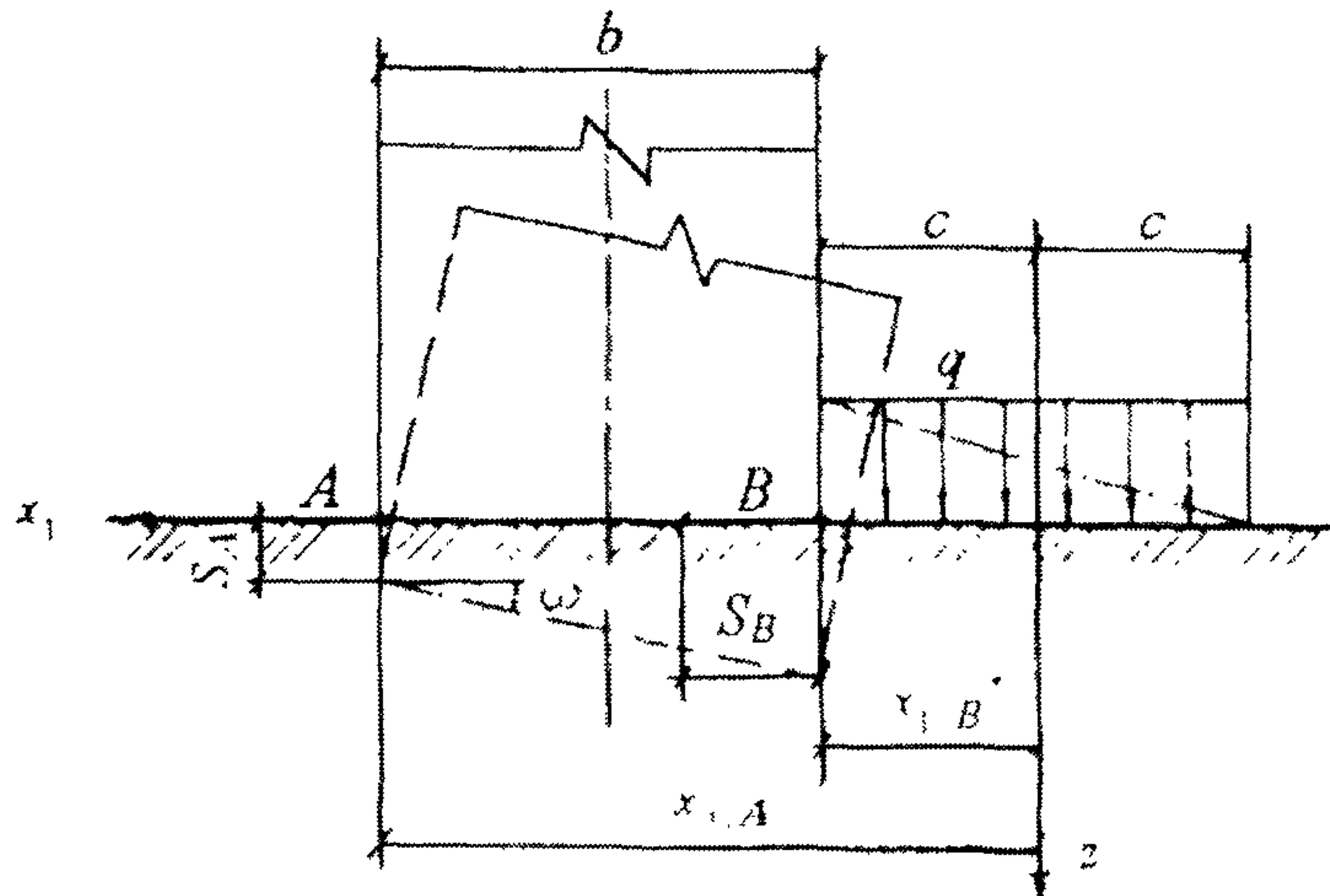
Рисунок 2 – Схема к определению крена сооружения от пригрузки
