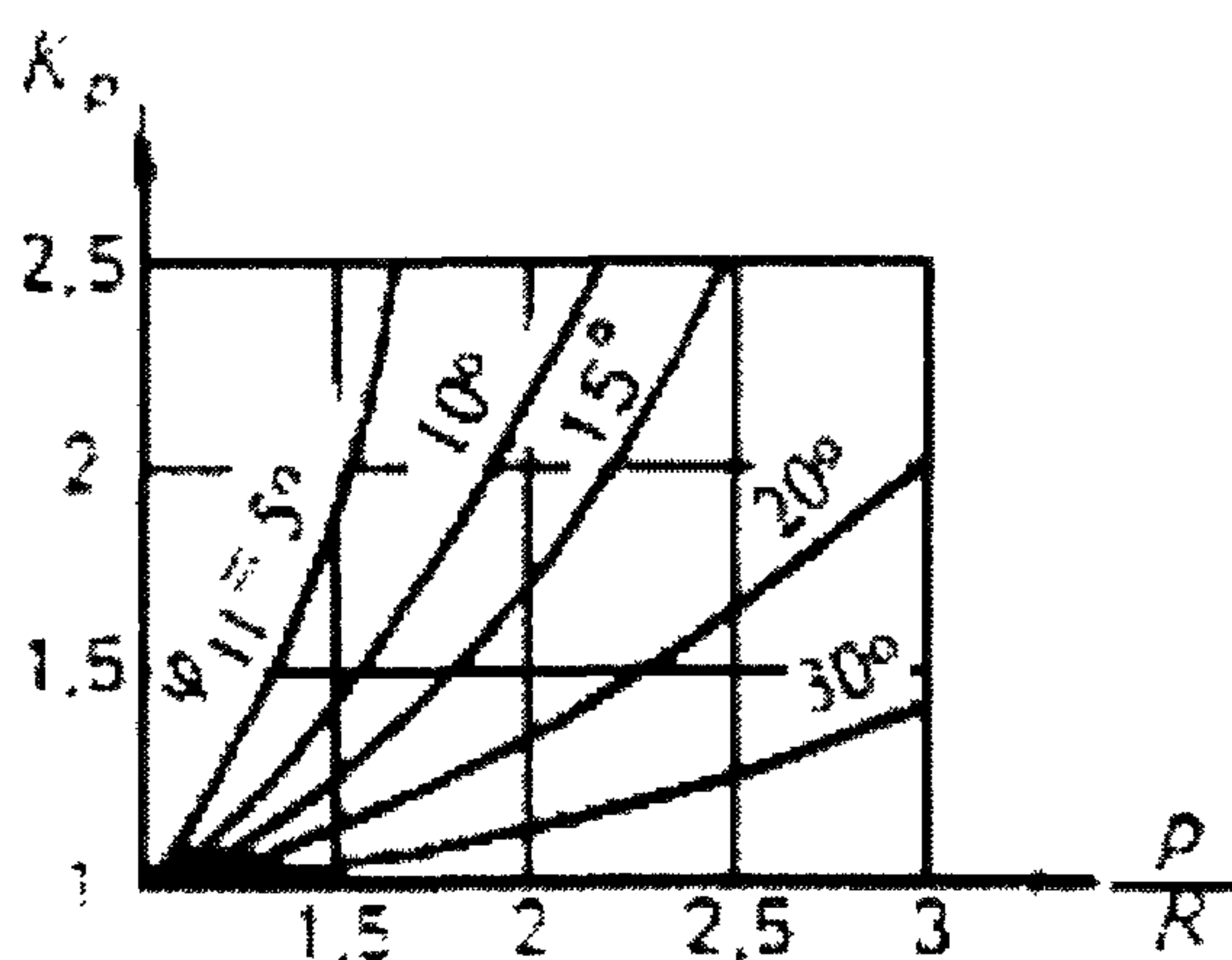
Рисунок Л.1 – График для определения коэффициента K_p
