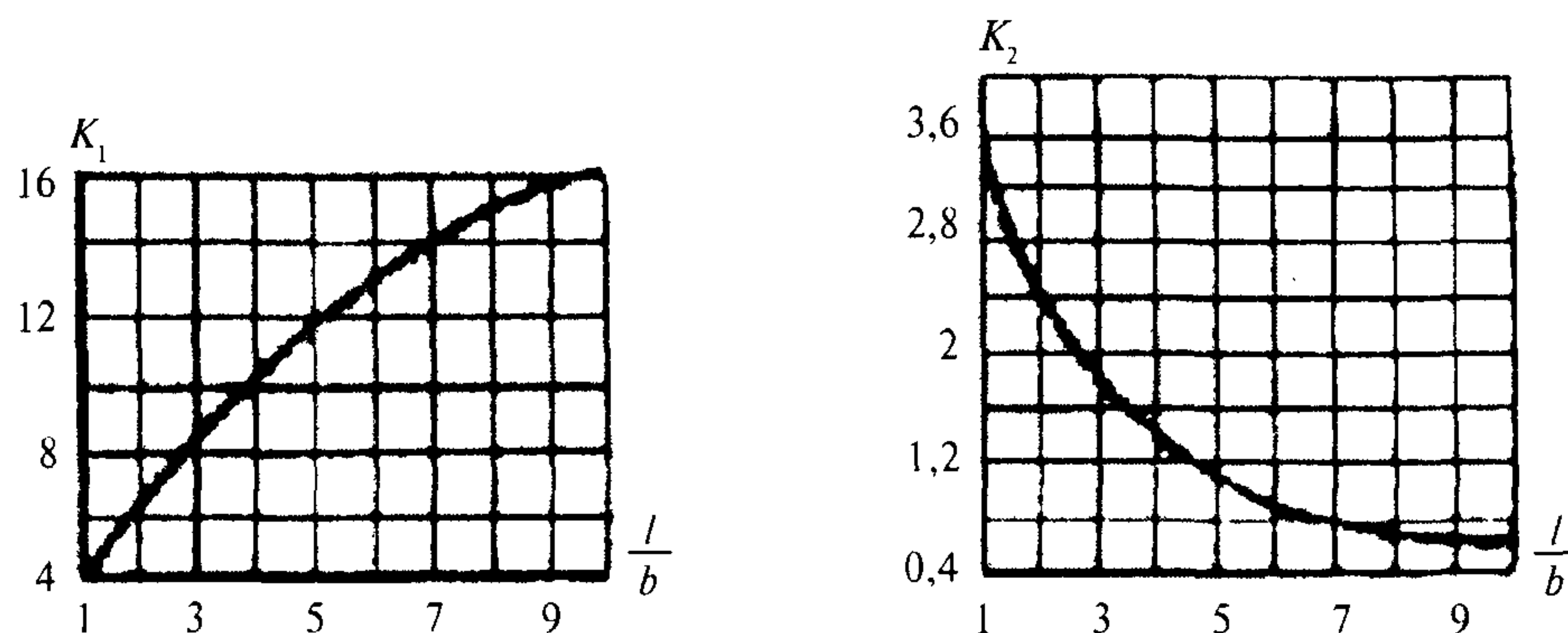
Рисунок 1 – Графики для определения коэффициентов K_1 и K_2
