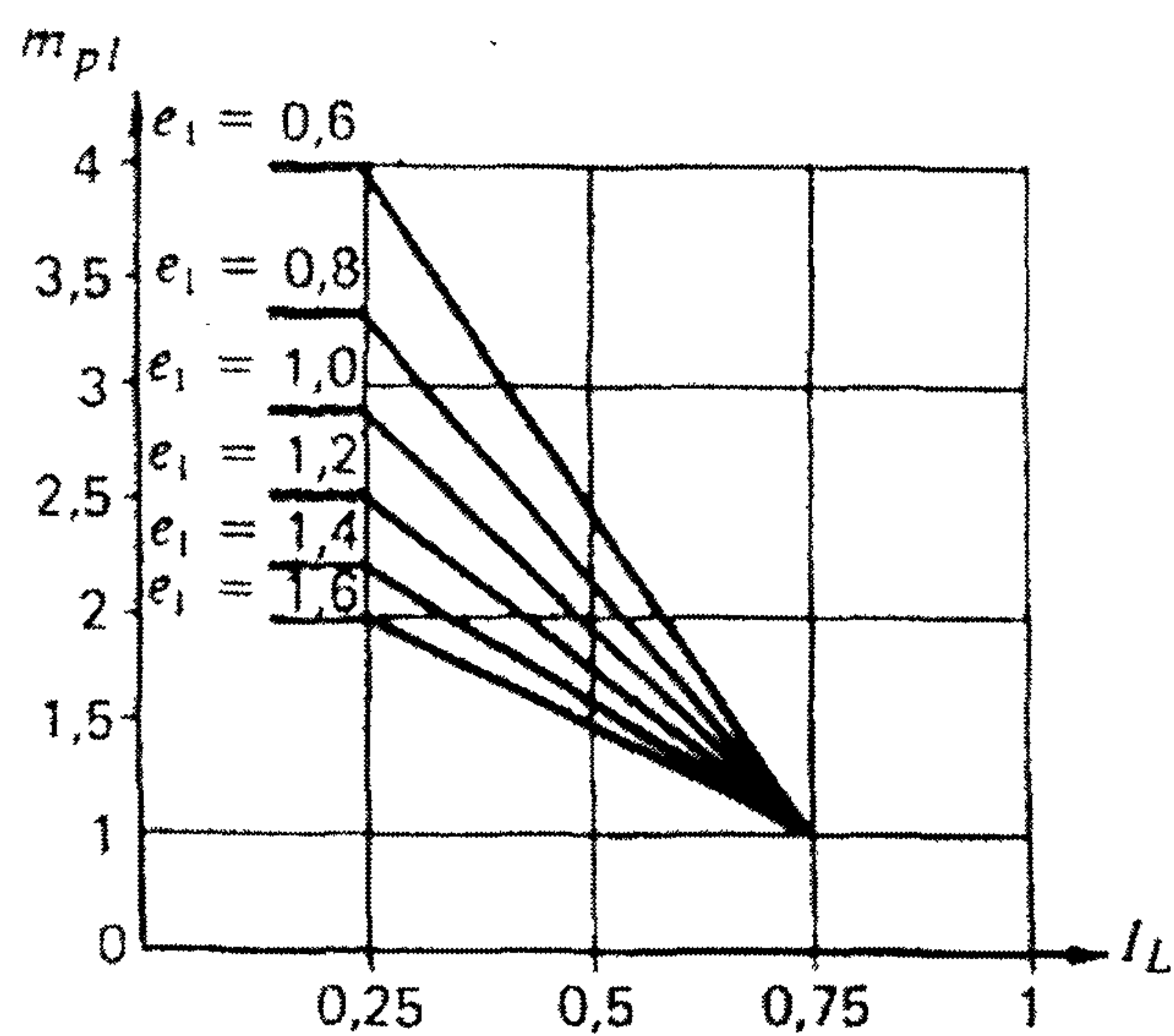
Рисунок В.1 – График для определения коэффициента m_{pl}
