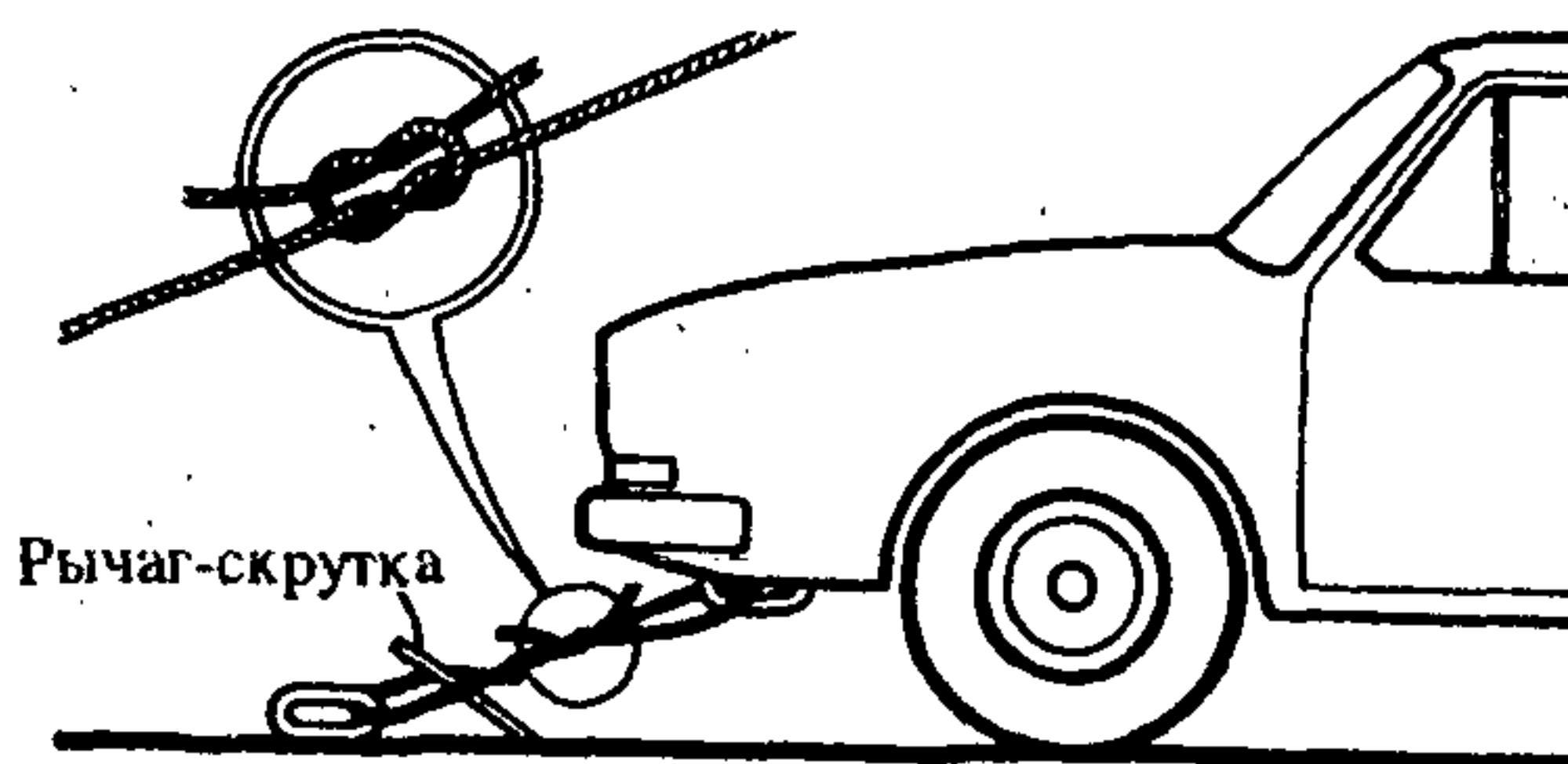
Рис. П.3.4. Крепление автомашин с помощью найтовов из синтетического или растительного каната
