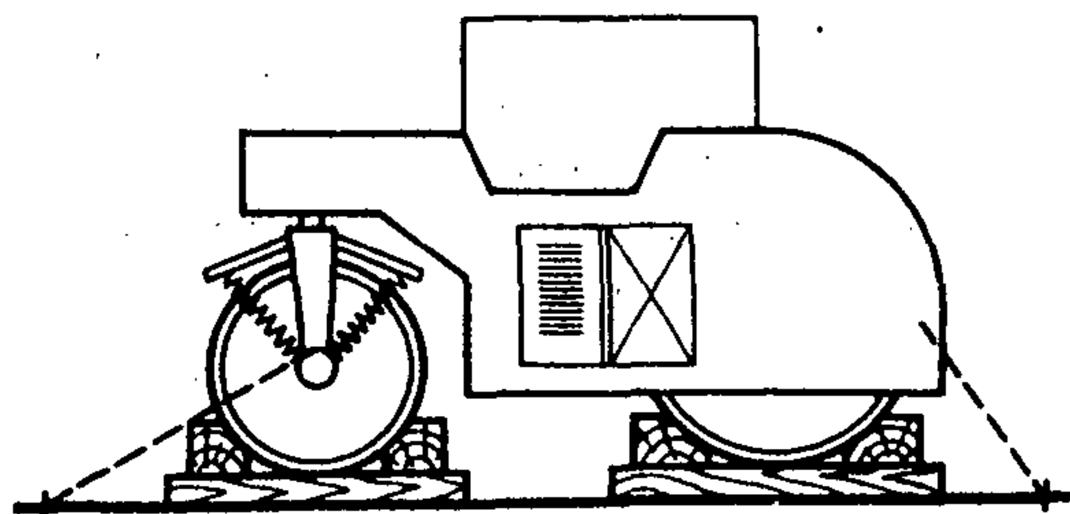
Рис. П.3.9. Дорожный мотокаток, масса 8 т
