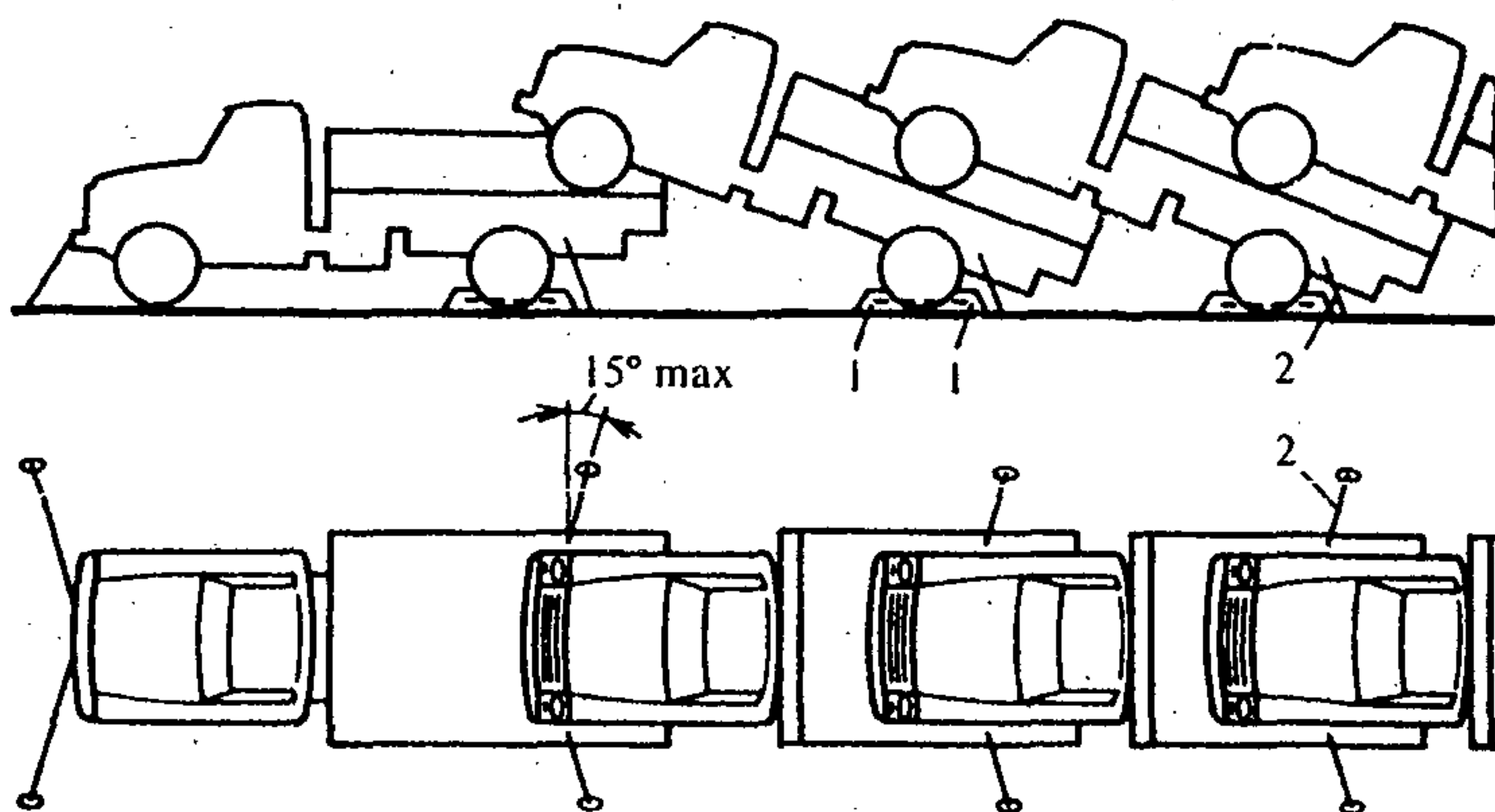
Рис. 5.1. Схема крепления автомашин: 1 - колодки; 2 - найтовы
