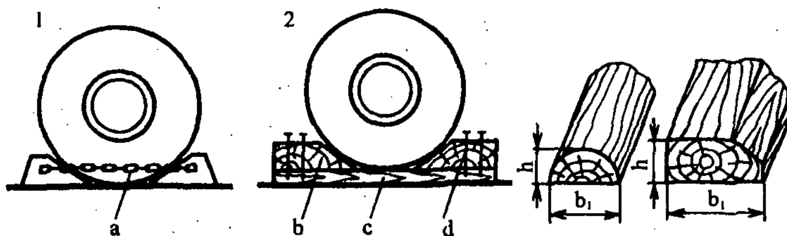
Рис. П.3.3. Установка упоров под колеса:
