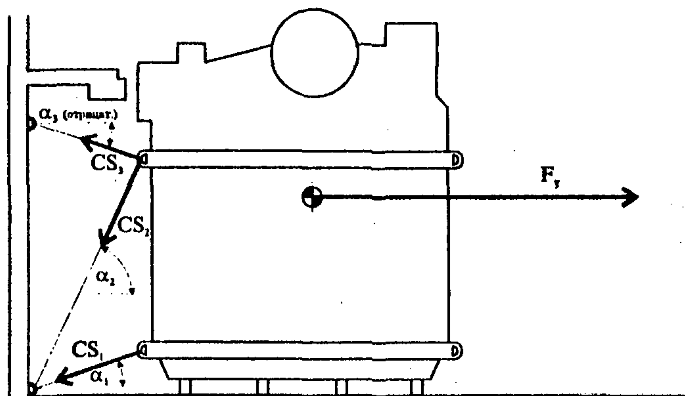
Рис. П.8.1. Равенство поперечных сил
