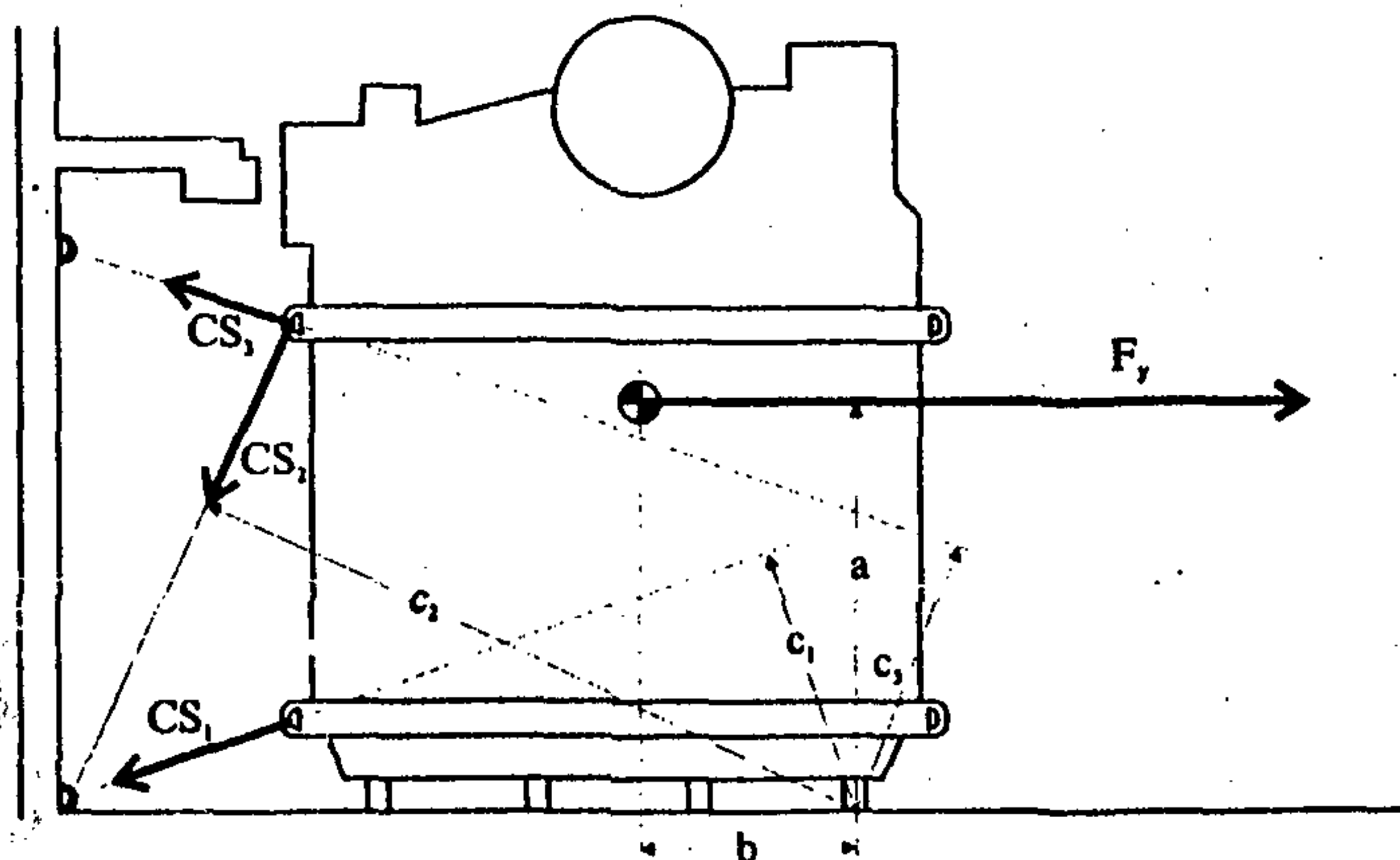
Рис. П.8.2. Равенство поперечных моментов
