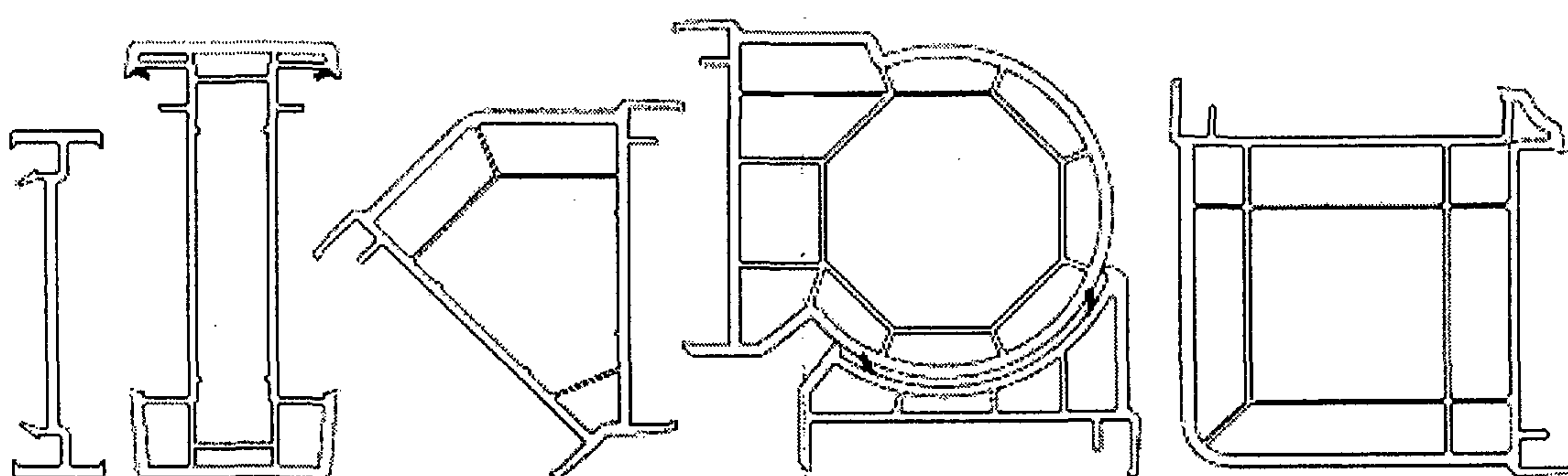
Сечения соединительных профилей
