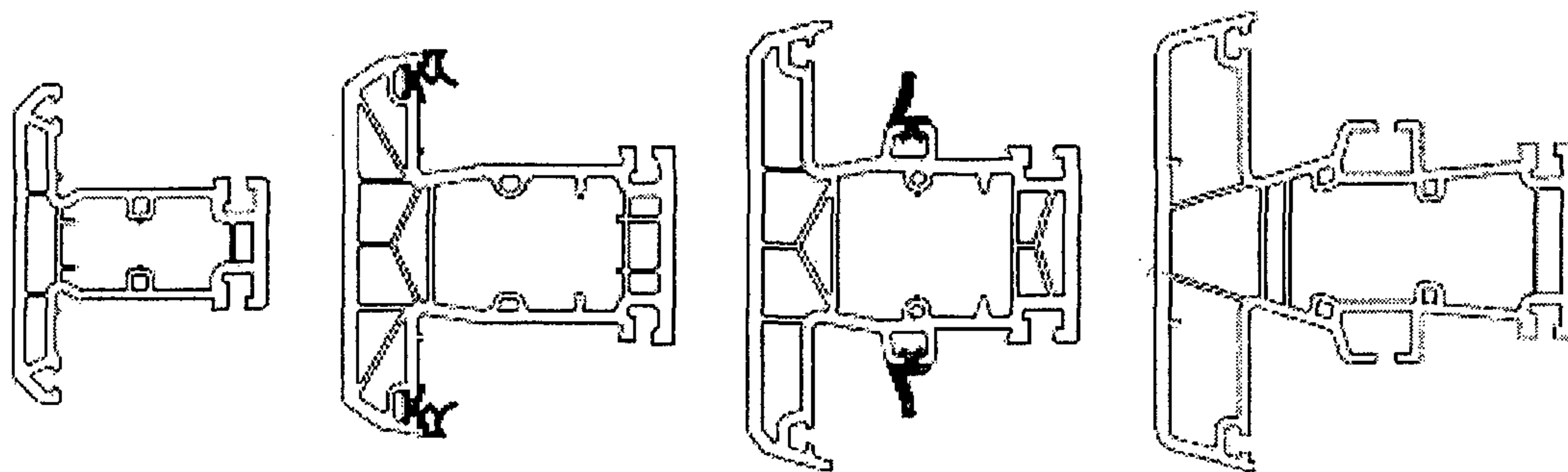
Сечения профилей импостов
