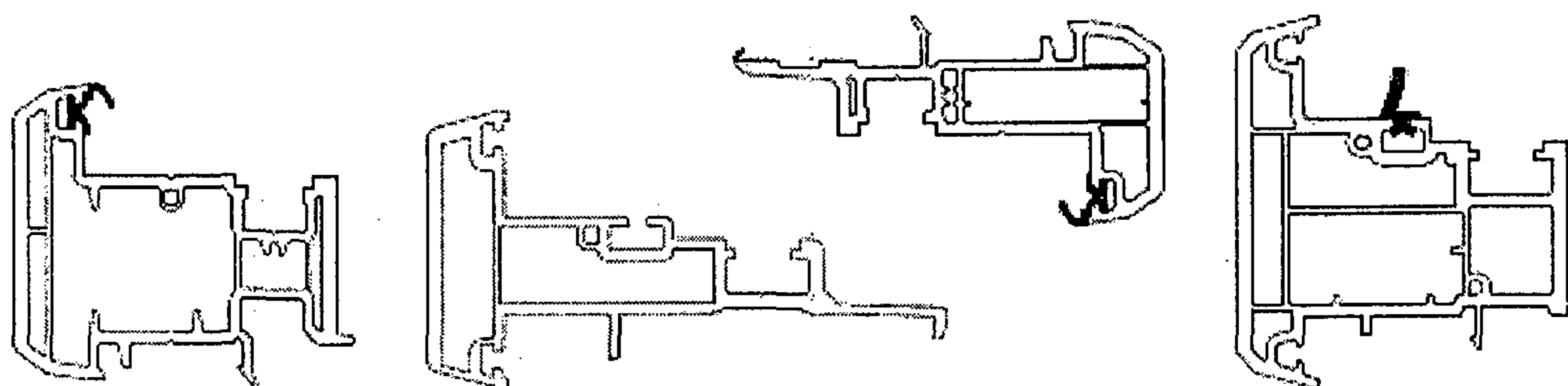
Сечения профилей штульпов
