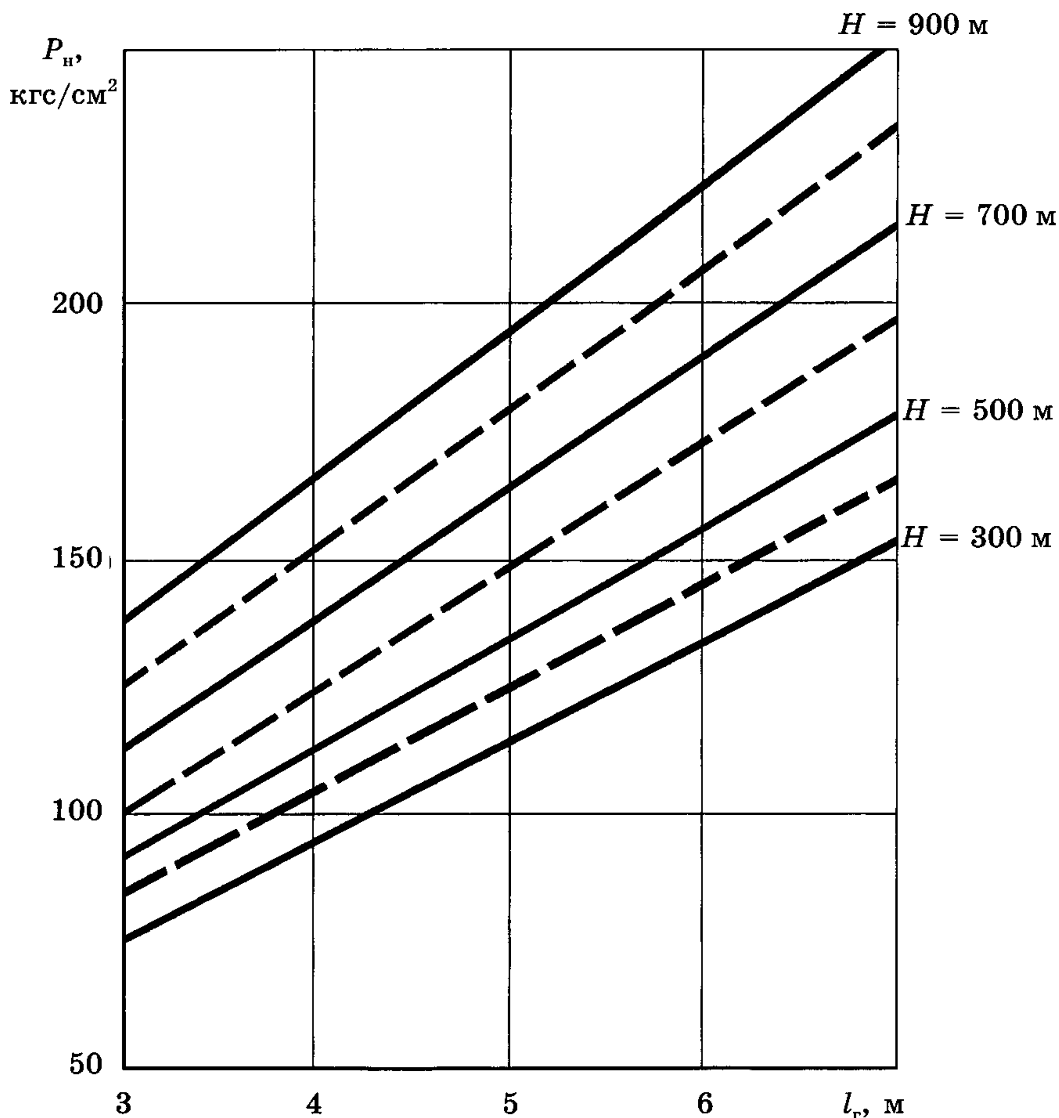
Рис. 5.2. Расчетное давление нагнетания P_n без учета потерь напора в гидросети P_c при различных значениях глубины герметизации l_r и глубины горных работ H
