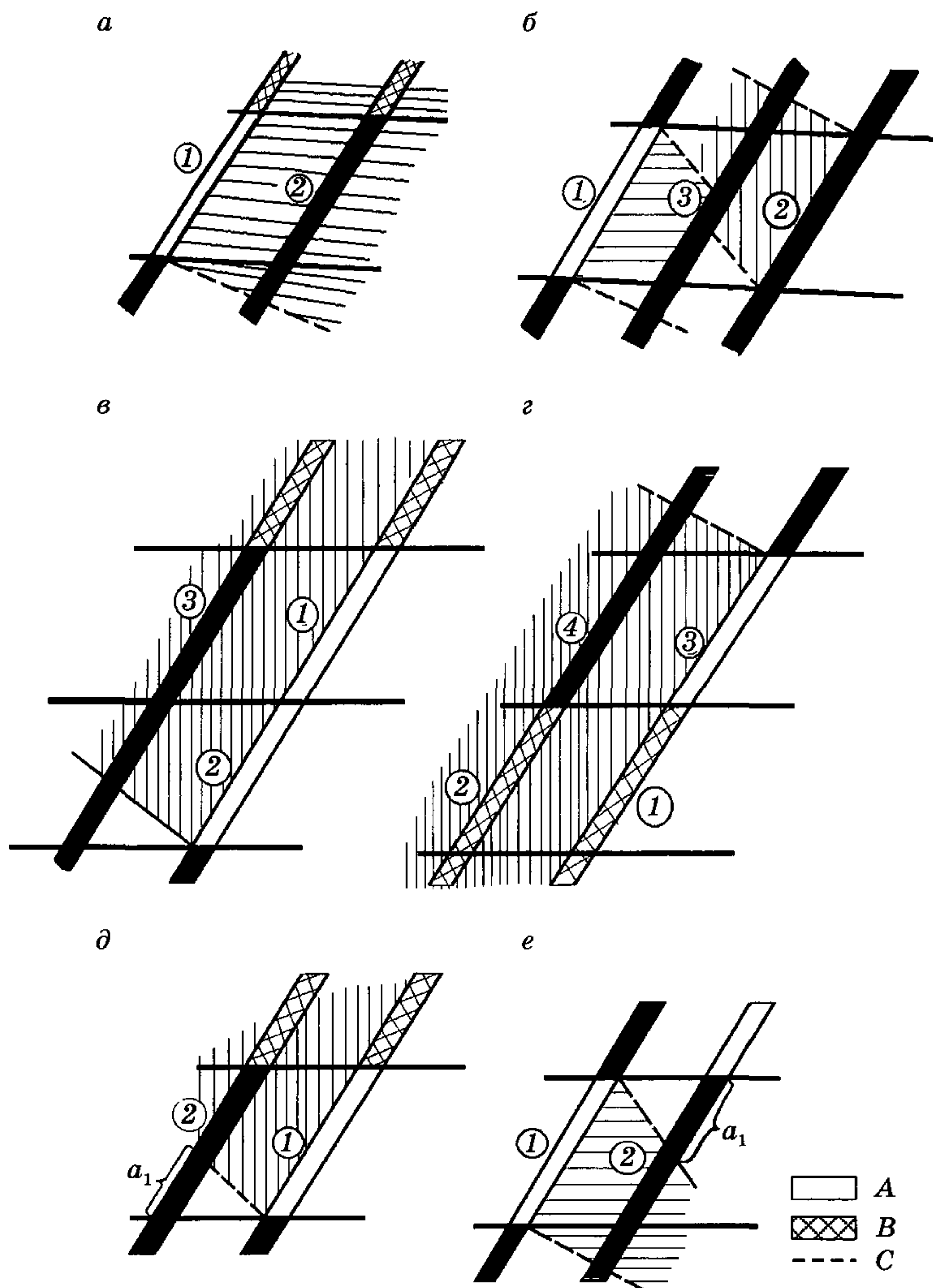
Рис. 3.1. Основные схемы использования защитных пластов:
