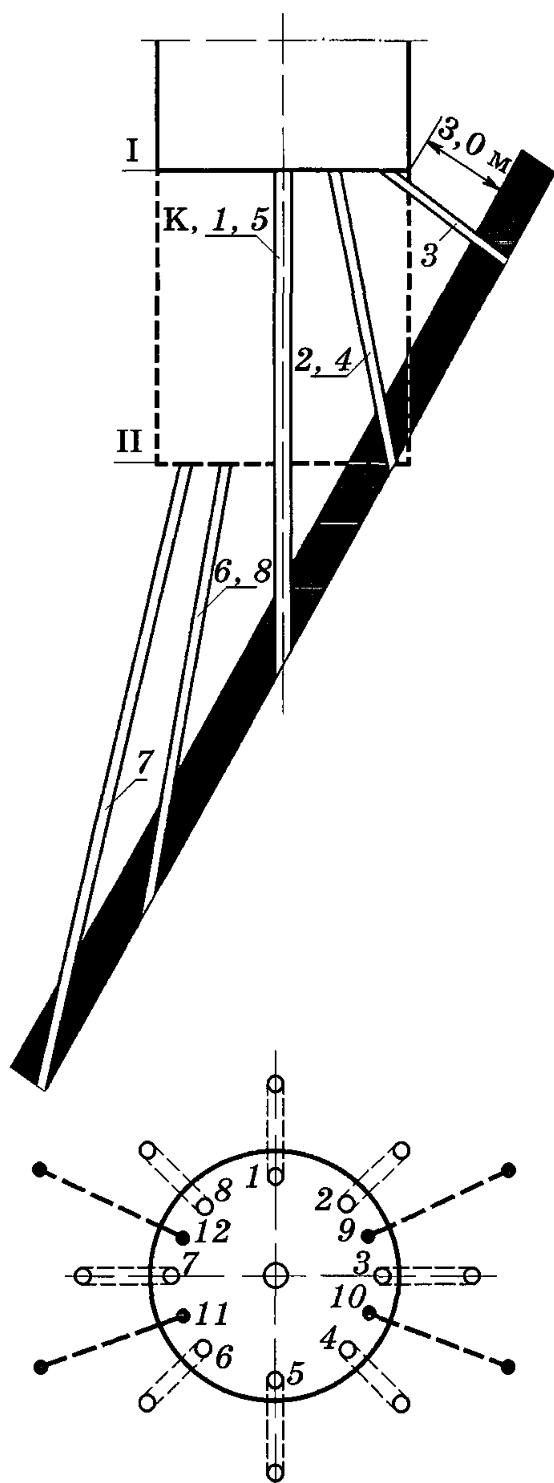
Рис. 4.5. Схема расположения скважин для гидрообработки крутого пласта из забоя выработки : 1, 2, 3, 4, 5, 6, 7, 8 — скважины для гидрорыхления угольного массива; 9, 10, 11, 12 — шпуров для замера давления газа; К — контрольная скважина; I, II — циклы обработки пласта
