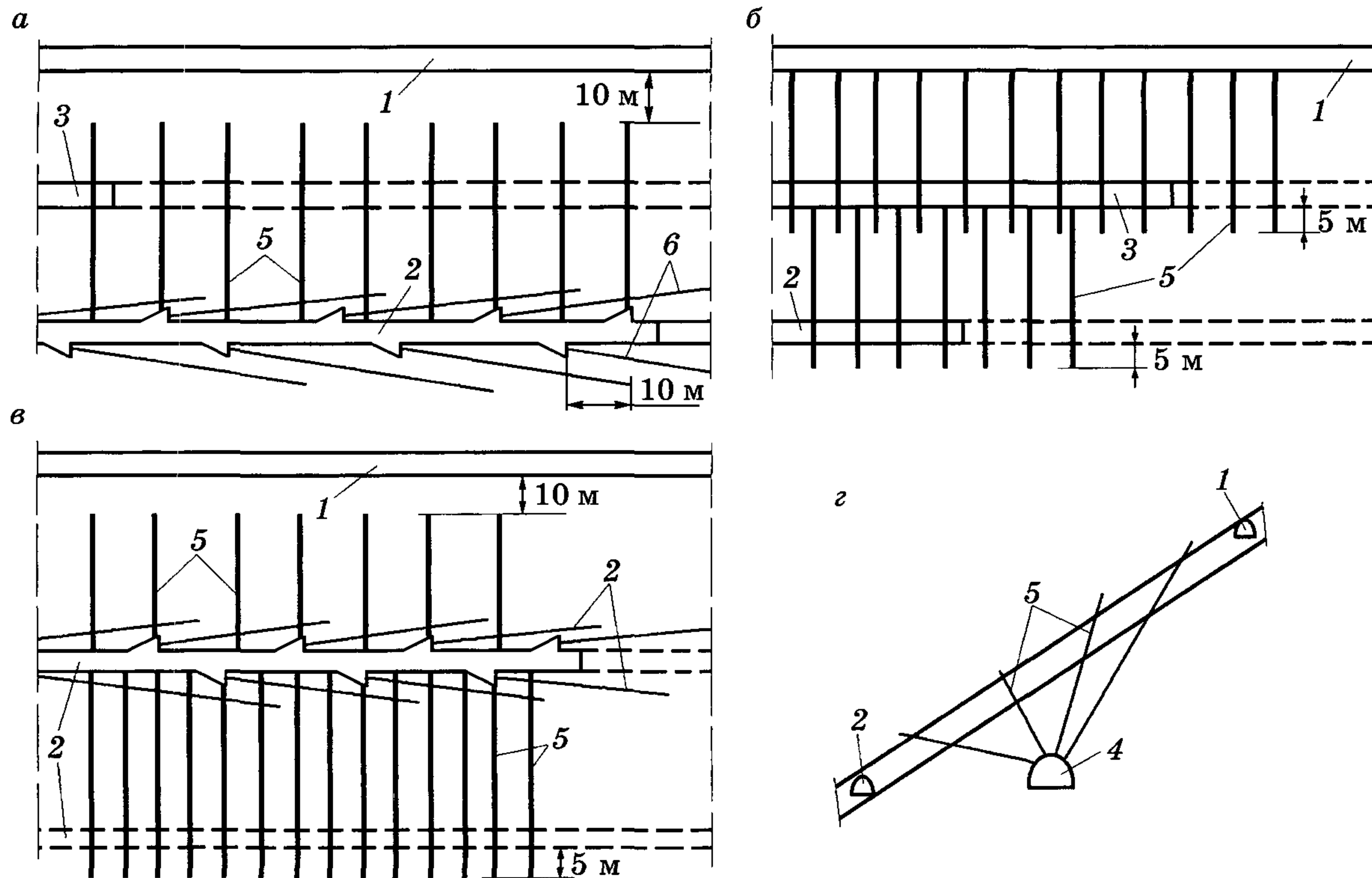
Рис. 3.3. Схемы дегазации угольного пласта:
