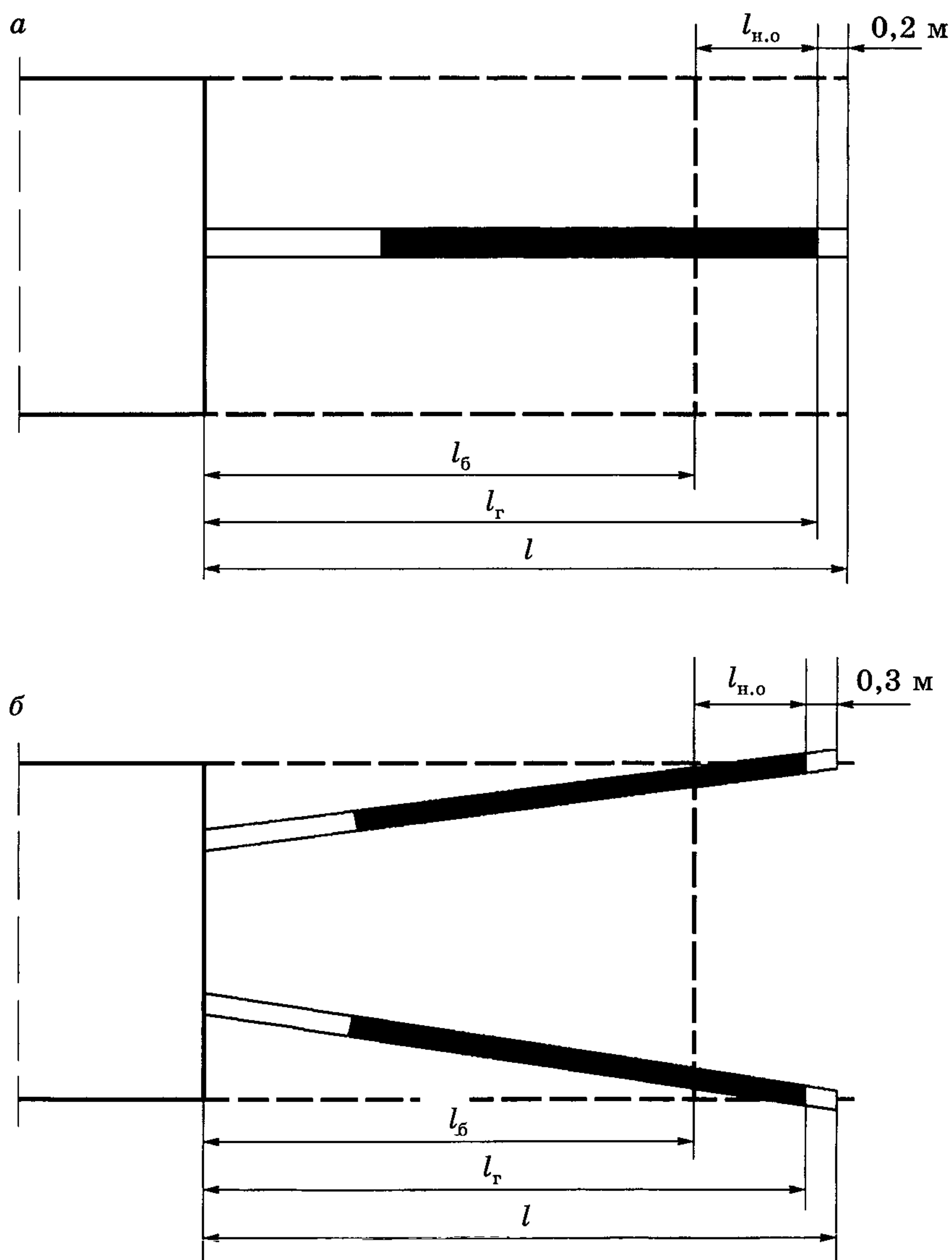
Рис. 5.1. Технологические схемы регулируемого гидроотжима: а — при мощности пачки прочного угля не менее 1 м; б — при любых условиях
