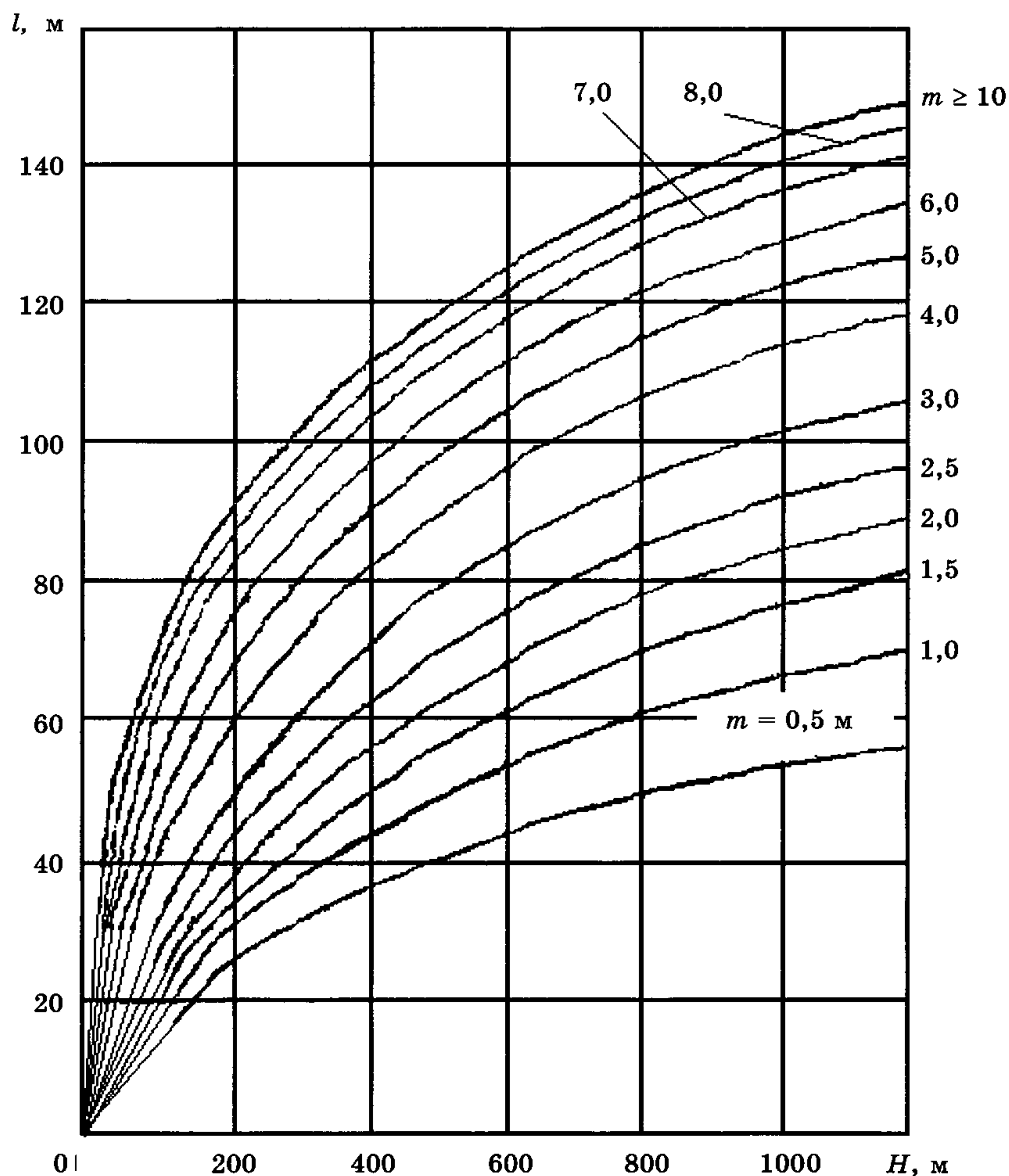
Рис. 3.2. Номограмма для определения ширины зоны опорного давления
