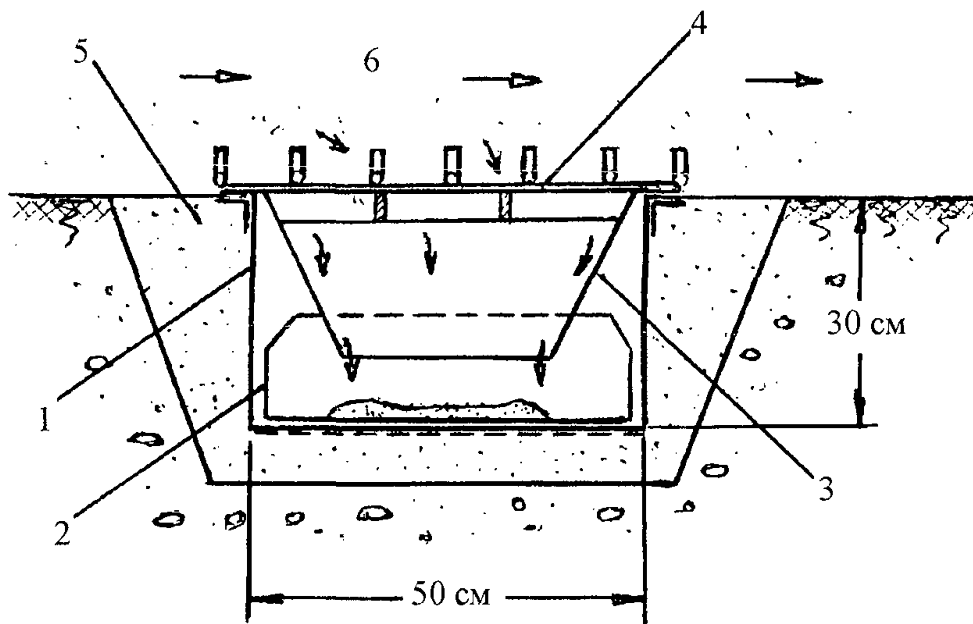
Рис.4. Конструкция наземного золоуловителя:
