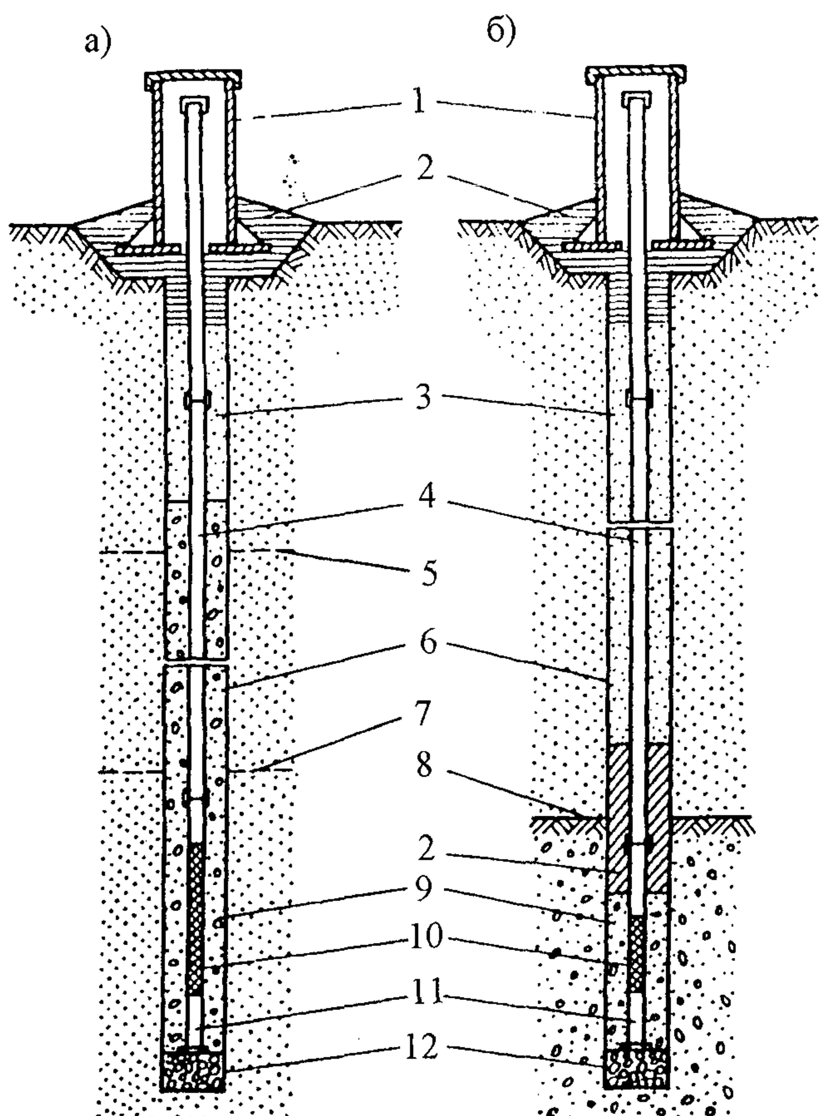
Рис.2. Опускные пьезометры
