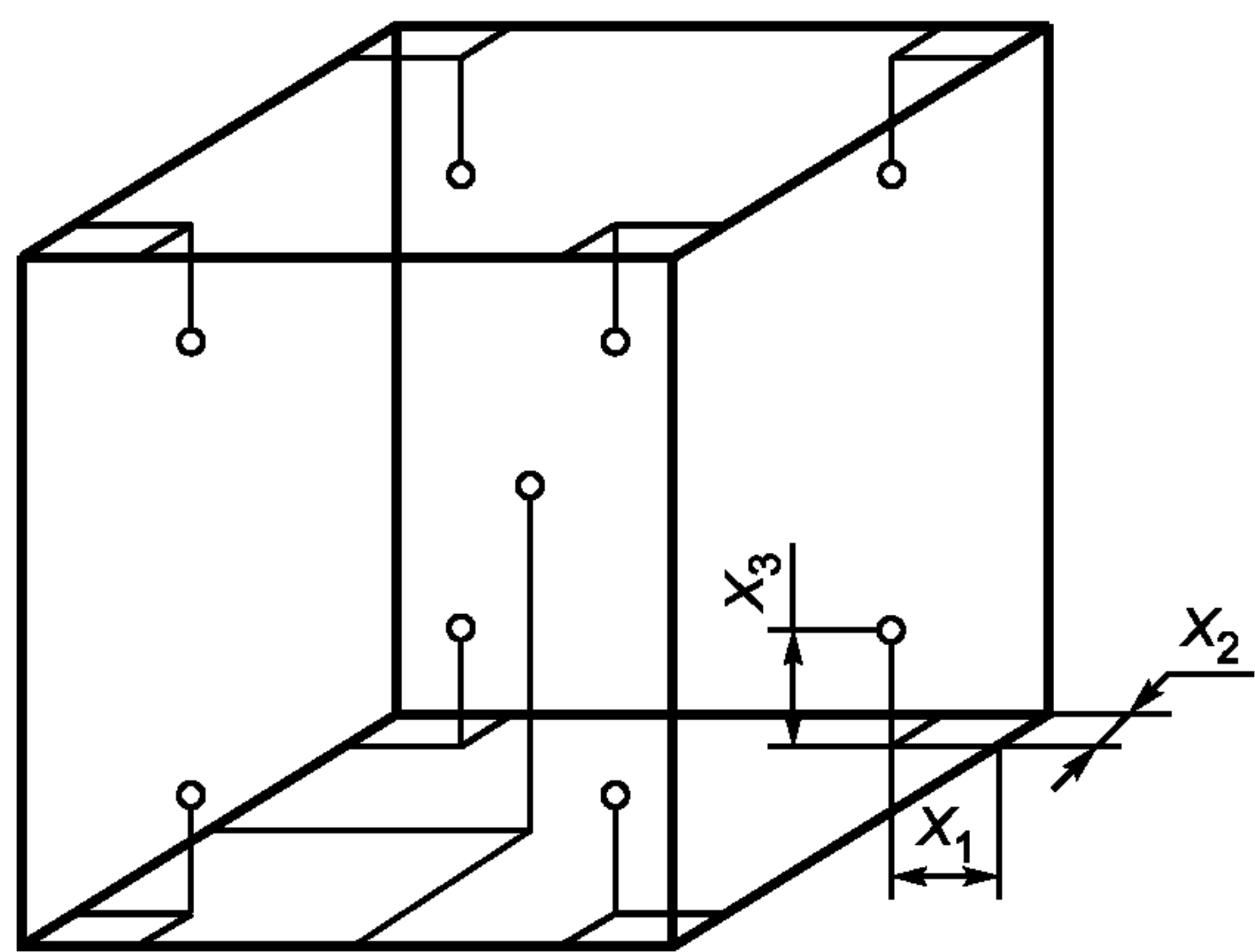
Рисунок 3 — Размещение датчиков температуры воздуха для камер объемом до 2000 л
