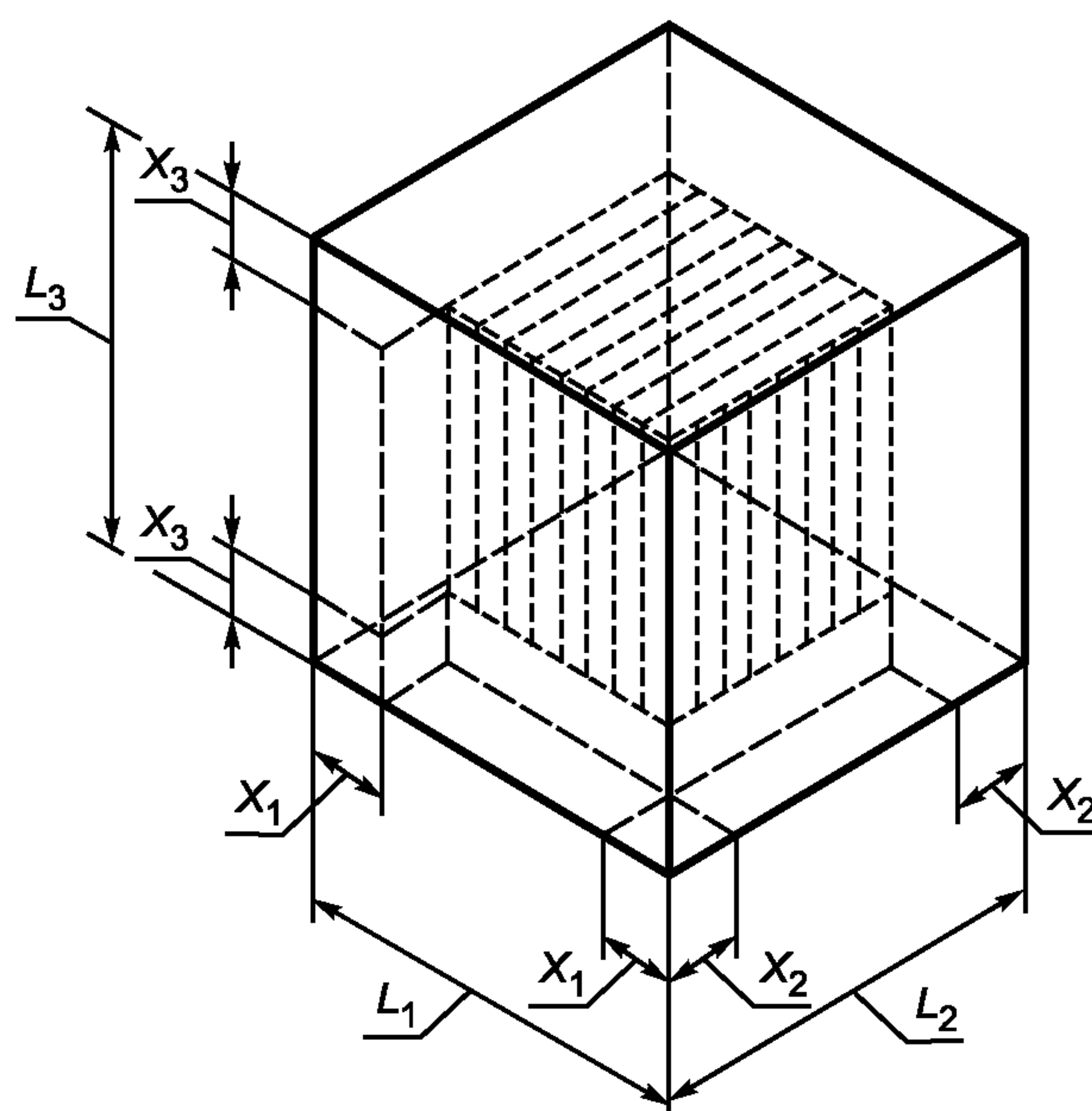
Рисунок 1 — Полезный объем
